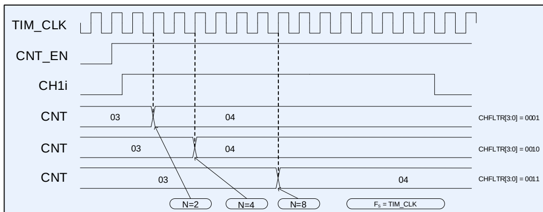
Рисунок 42 – Диаграмма внешнего тактирования с разными вариантами фильтра
