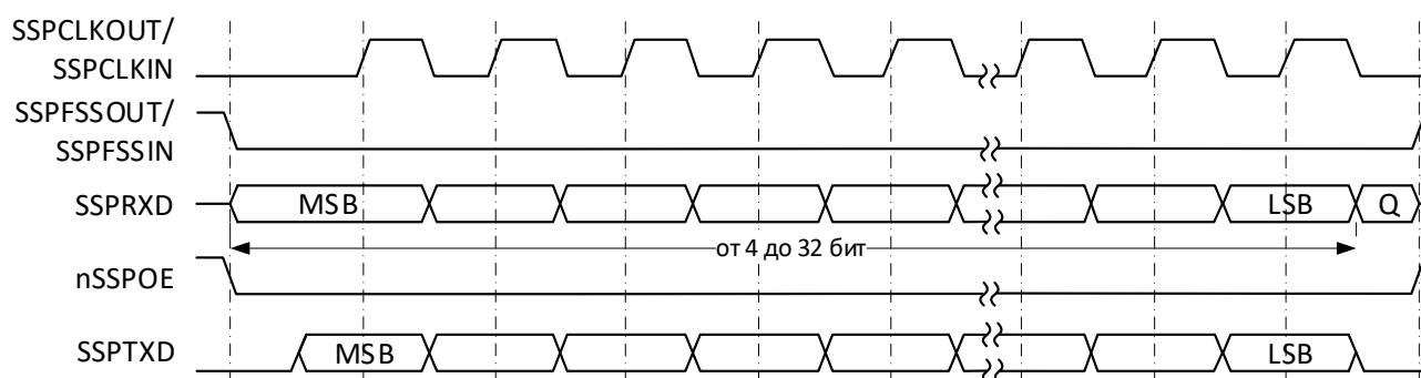
Рисунок 66 – Формат синхронного обмена протокола SPI, SPO=0, SPH=0 (одиночный обмен)
