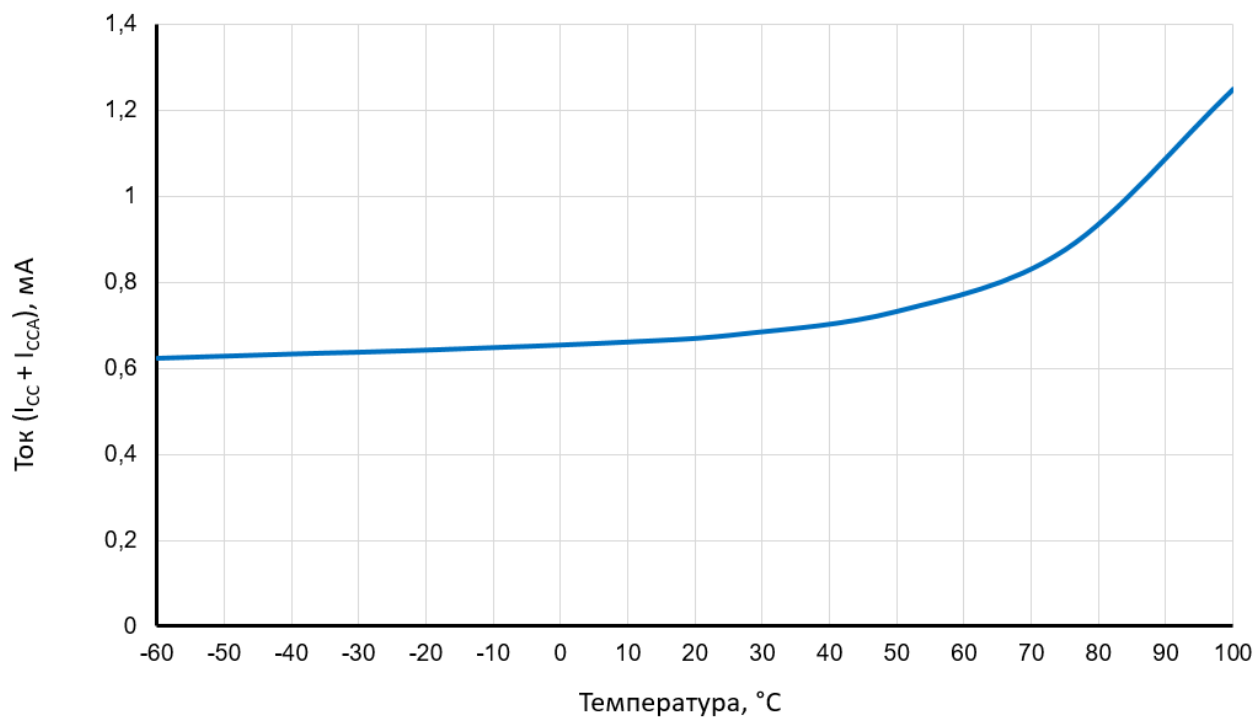
Рисунок 128 – Зависимость суммарного статического тока ( n\text{RESET} = 0 ) I_{CC} и I_{CCA} от температуры при U_{CC} = U_{CCA} = 3,3 В
