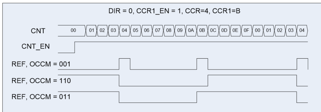
Рисунок 49 – Диаграмма работы в режиме ШИМ, CCR1_EN = 1
