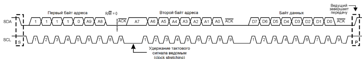
Рисунок 62 – Передача по I2C в 10-битном режиме
