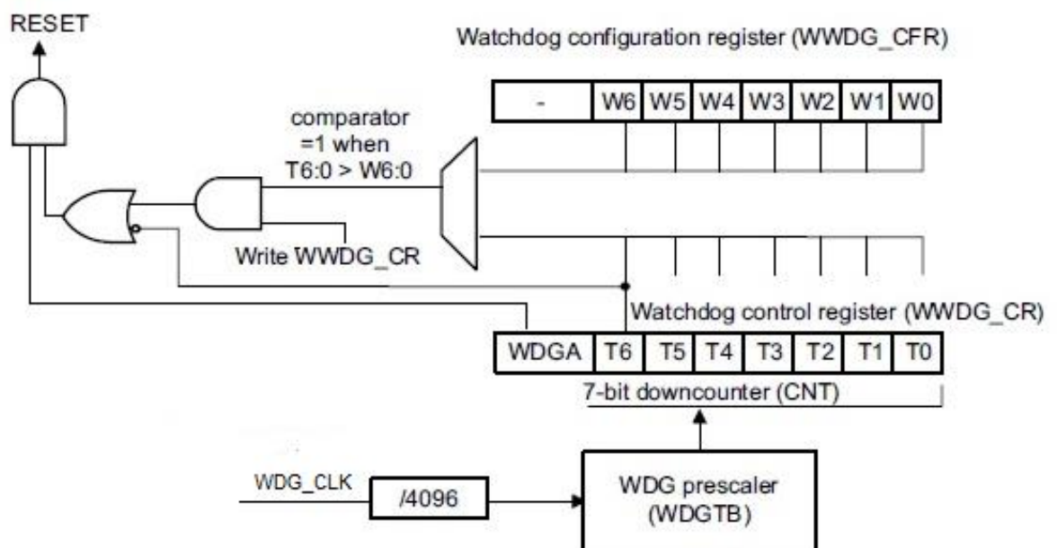
Рисунок 102 – Блок-схема оконного сторожевого таймера
