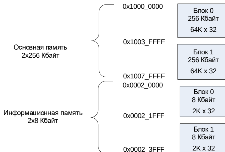
Рисунок 11 – Структура памяти
