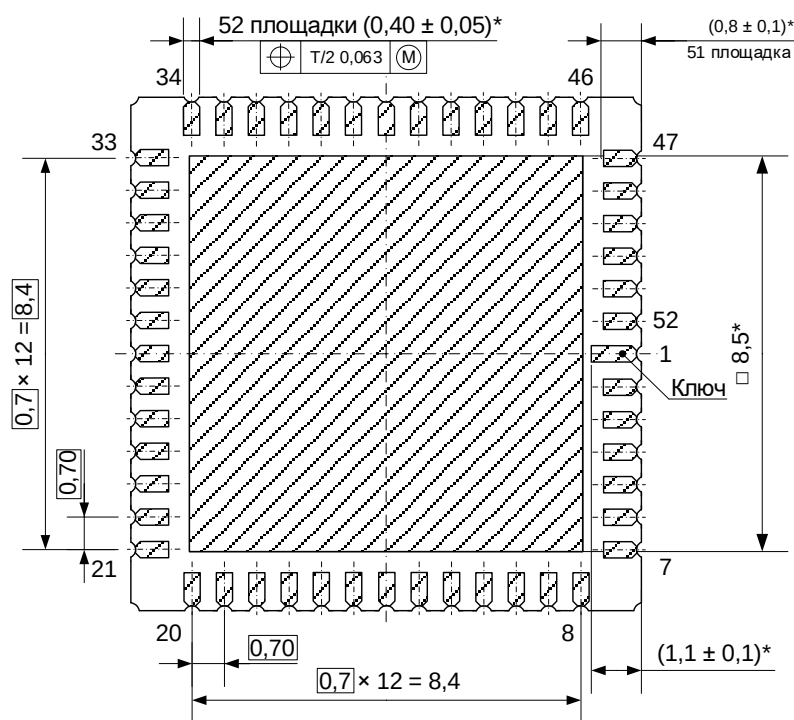
Рисунок 129 – Микросхема в корпусе 5152.52-3 К
