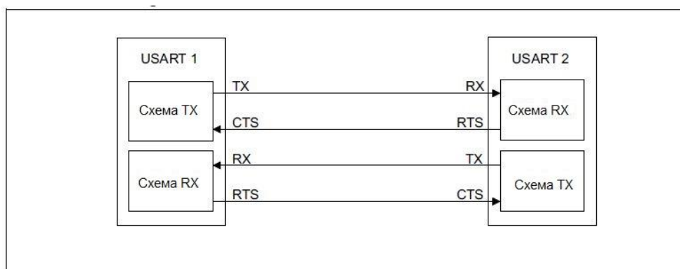
Рисунок 120 – Аппаратное управление потоком данных между двумя устройствами USART
