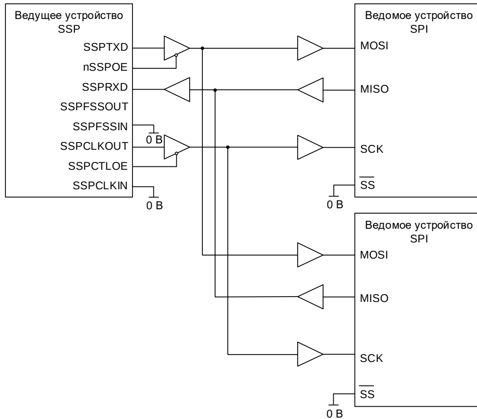
Рисунок 76 – Ведущее устройство SSP подключено к двум ведомым, поддерживающим SPI
