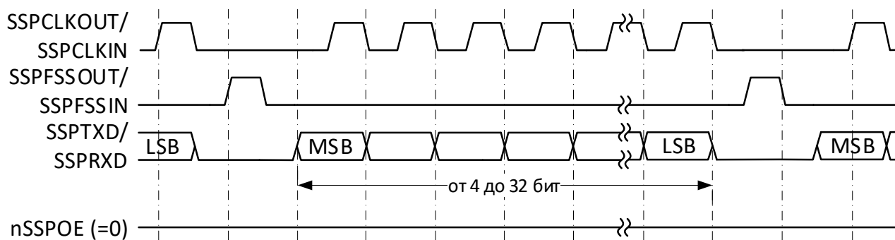
Рисунок 67 – Формат синхронного обмена протокола SPI, SPO=0, SPH=0 (непрерывный обмен)
