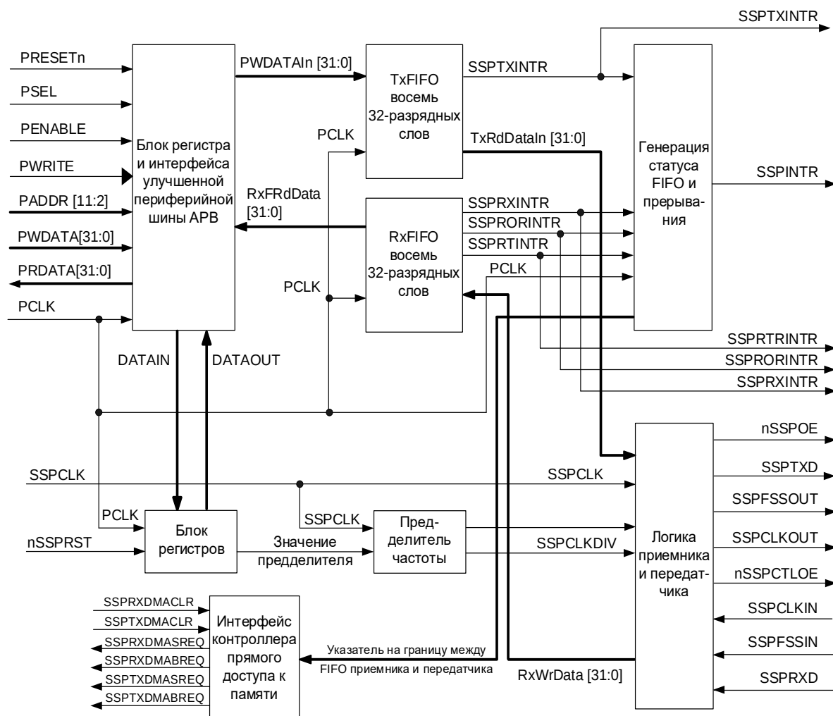
Рисунок 63 – Структурная схема модуля SSP
