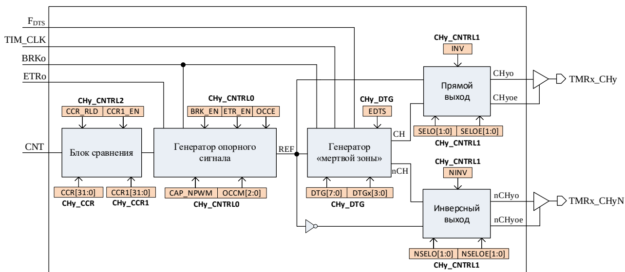
Рисунок 47 – Структурная схема блока формирования ШИМ
