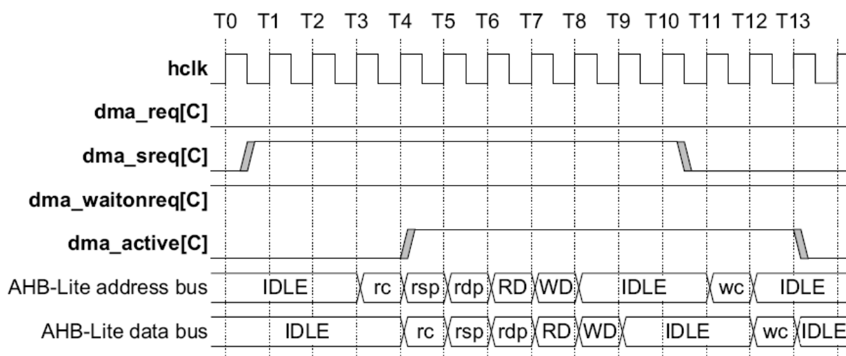
Рисунок 91 – Работа DMA при использовании dma_waitonreq совместно с dma_sreq
