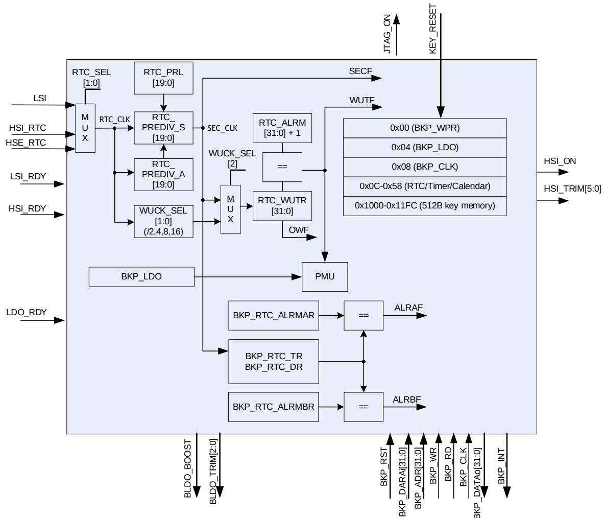
Рисунок 27 – Структурная блок-схема батарейного домена и часов реального времени
