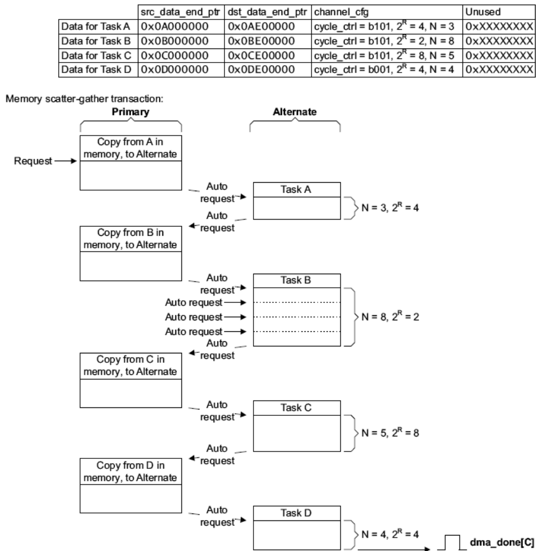
Рисунок 94 – Пример работы DMA в режиме с «Исполнением с изменением конфигурации»
