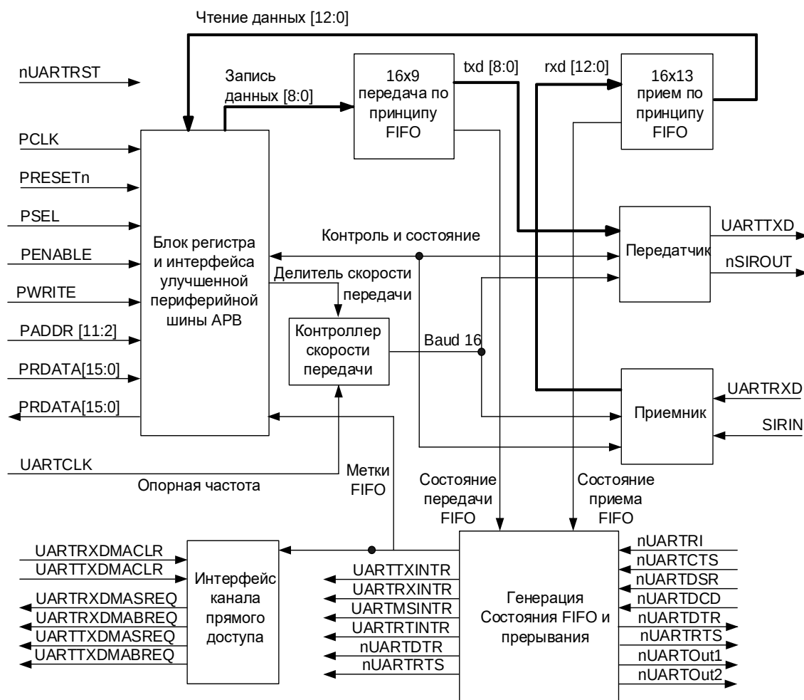
Рисунок 79 – Блок-схема универсального асинхронного приёмопередатчика (UART)
