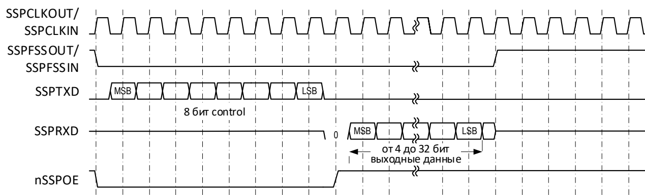
Рисунок 72 – Формат синхронного обмена протокола Microwire (одиночный обмен)
