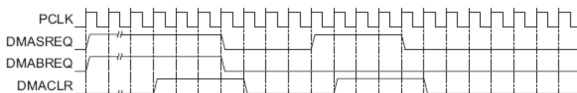
Рисунок 78 – Временные диаграммы обмена в режиме DMA
