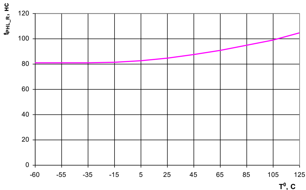
Рисунок 12 – Зависимость времени задержки распространения сигнала приемника при включении t_{PHL\_R} от температуры для микросхем K5559ИИ10АSI, K5559ИИ10БSI
