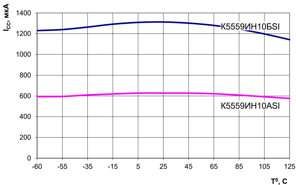
Рисунок 4 – Зависимость тока потребления I_{CC} от температуры для микросхем K5559ИH10ASI, K5559ИH10BSI при: U_{DE} = U_{CC}
