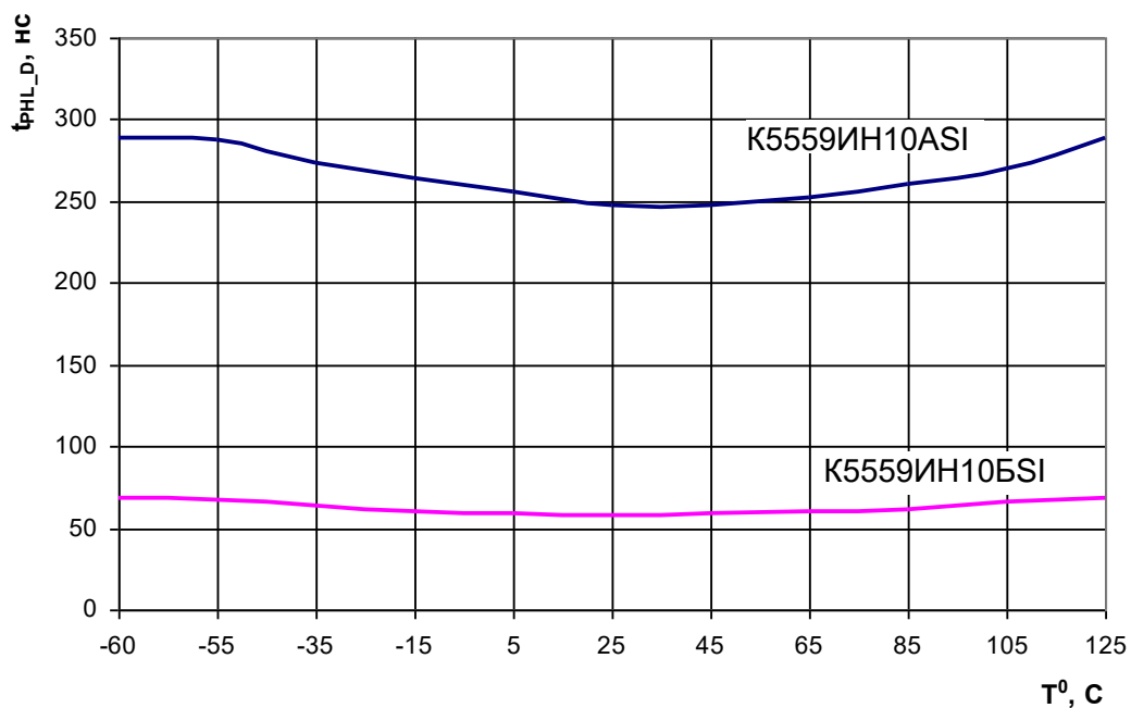
Рисунок 10 – Зависимость времени задержки распространения сигнала передатчика при выключении t_{PHL\_D} от температуры для микросхем K5559ИИ10АСI, K5559ИИ10БСИ
