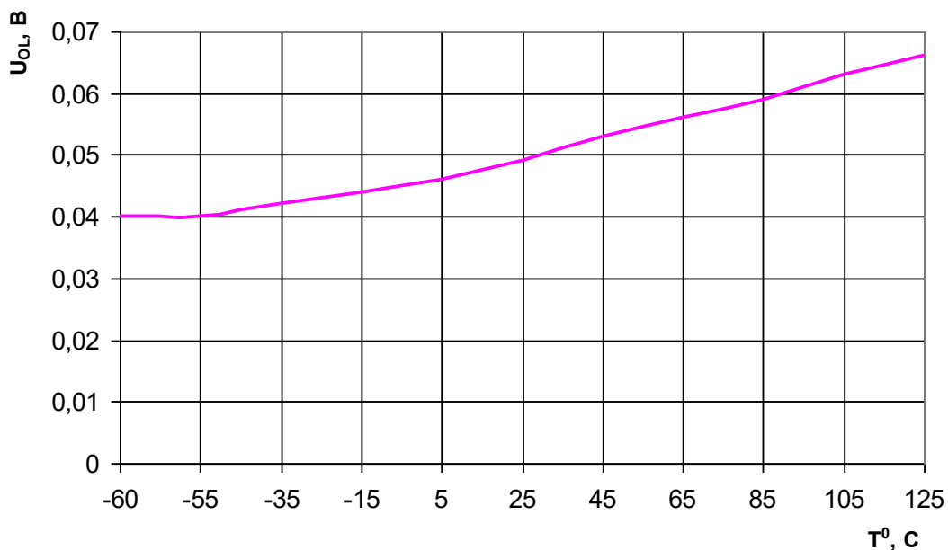
Рисунок 14 – Зависимость выходного напряжения низкого уровня приемника U_{OL} от температуры для микросхем K5559ИИ10АSI, K5559ИИ10БSI
