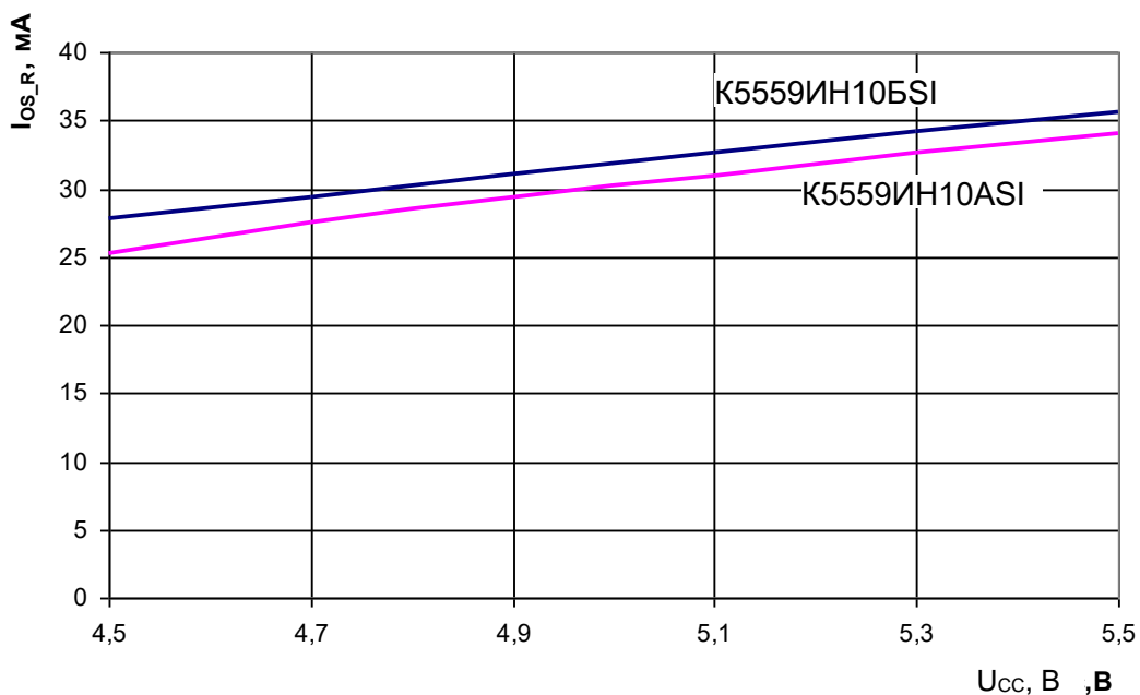
Рисунок 6 – Зависимость тока короткого замыкания выхода приемника I_{os\_R} от напряжения источника питания для микросхем K5559ИИ10АSI, K5559ИИ10БSI
