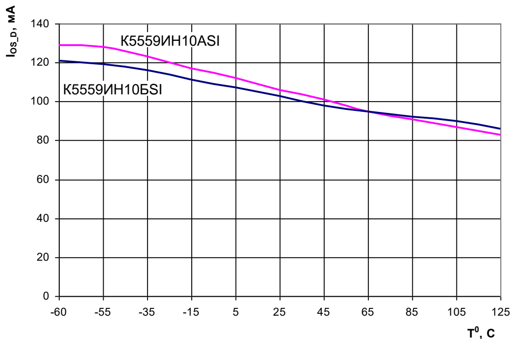
Рисунок 15 – Зависимость тока короткого замыкания передатчика I_{0S\_D} от температуры для микросхем K5559ИИ10АSI, K5559ИИ10БSI
