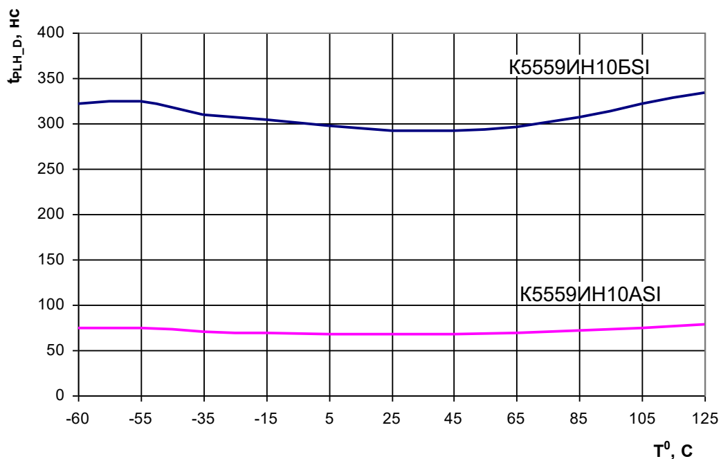
Рисунок 9 – Зависимость времени задержки распространения сигнала передатчика при включении t_{PLH\_D} от температуры для микросхем K5559ИИ10АSI, K5559ИИ10БSI
