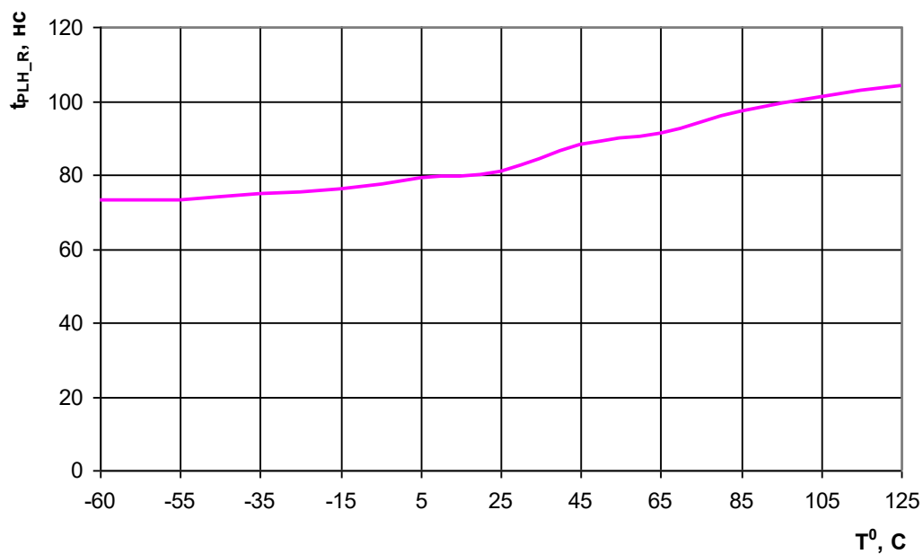
Рисунок 11 – Зависимость времени задержки распространения сигнала приемника при выключении t_{PLH\_R} от температуры для микросхем K5559ИИ10АСI, K5559ИИ10БСИ
