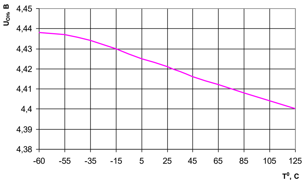
Рисунок 13 – Зависимость выходного напряжения высокого уровня приемника U_{OH} от температуры для микросхем K5559ИИ10АSI, K5559ИИ10БSI
