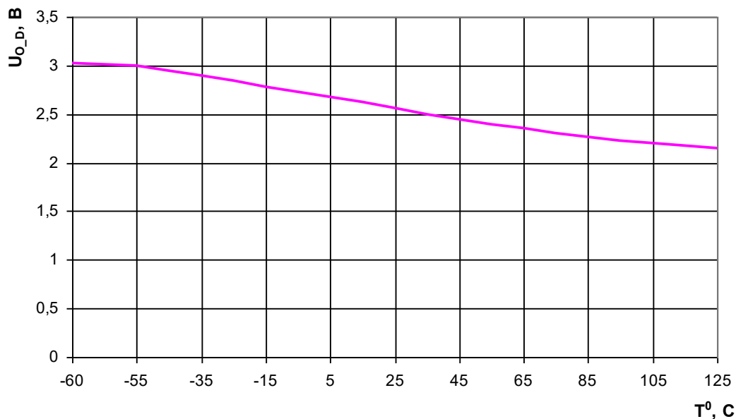
Рисунок 8 – Зависимость выходного дифференциального напряжения передатчика U_{O\_D} от температуры для микросхем K5559ИИ10АSI, K5559ИИ10БSI
