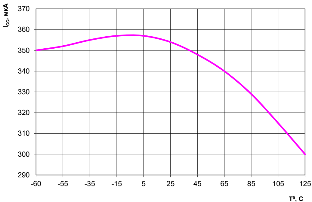
Рисунок 5 – Зависимость тока потребления I_{CC} от температуры для микросхем K5559ИH10ASI, K5559ИH10BSI при: U_{DE} = 0 В, без нагрузки
