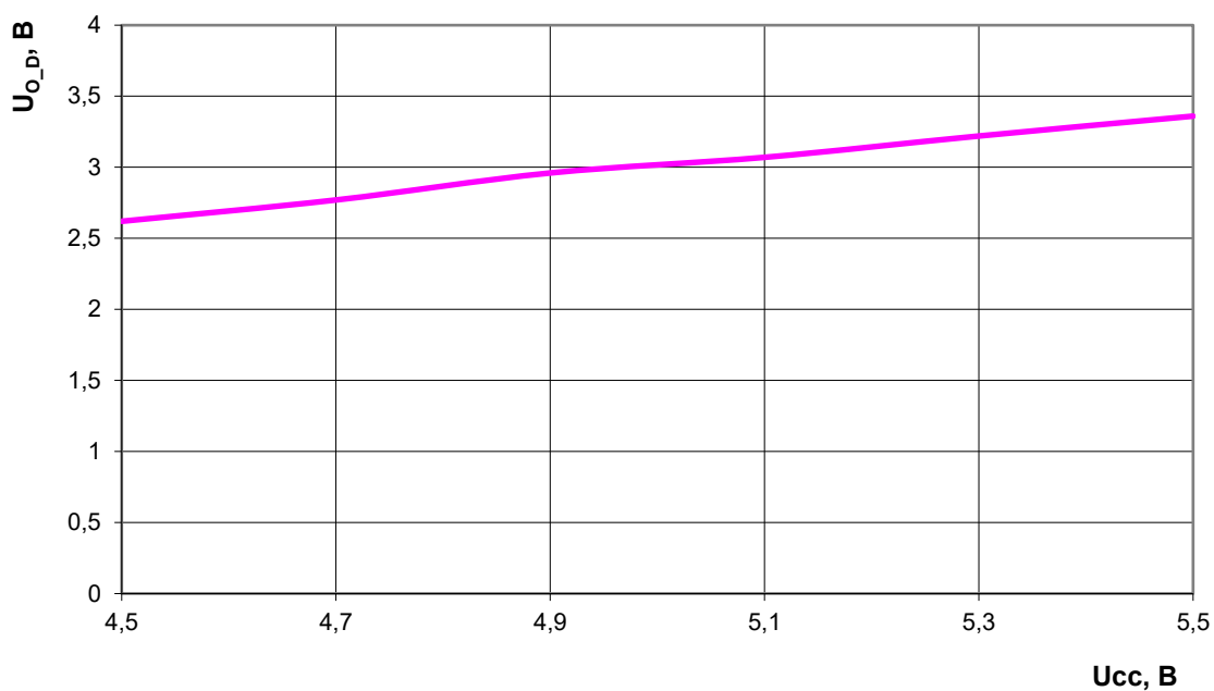
Рисунок 7 – Зависимость выходного дифференциального напряжения передатчика U_{o\_D} от напряжения источника питания для микросхем K5559ИИ10АSI, K5559ИИ10БSI
