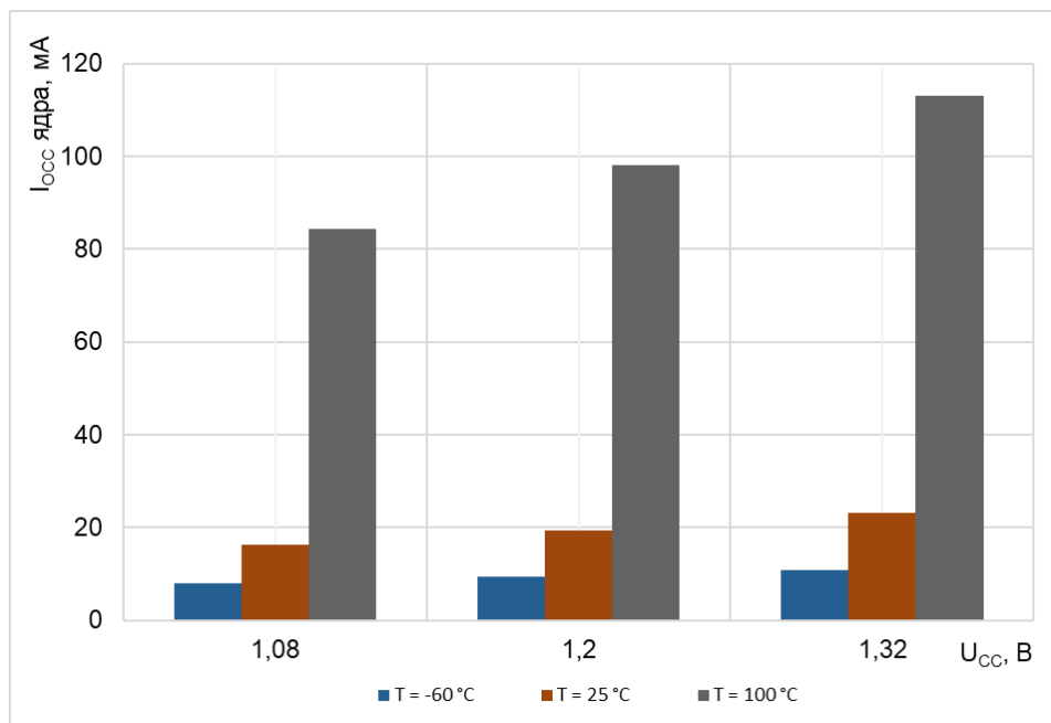
Рисунок 188 – Зависимость тока потребления I_{OSS} ядра от температуры и напряжения U_{CC} в режиме SLEEP
