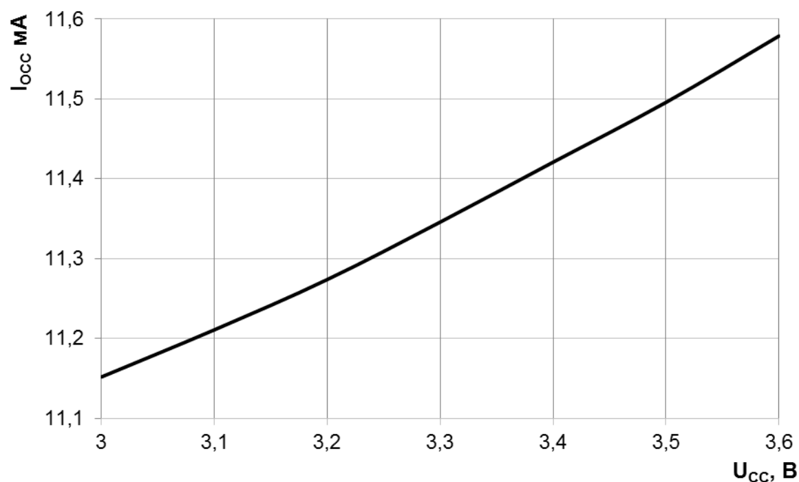
Рисунок 182 – Зависимость динамического тока потребления I_{OSS} аналоговых блоков от напряжения питания при f_C = 230 МГц, T = 25 °С
