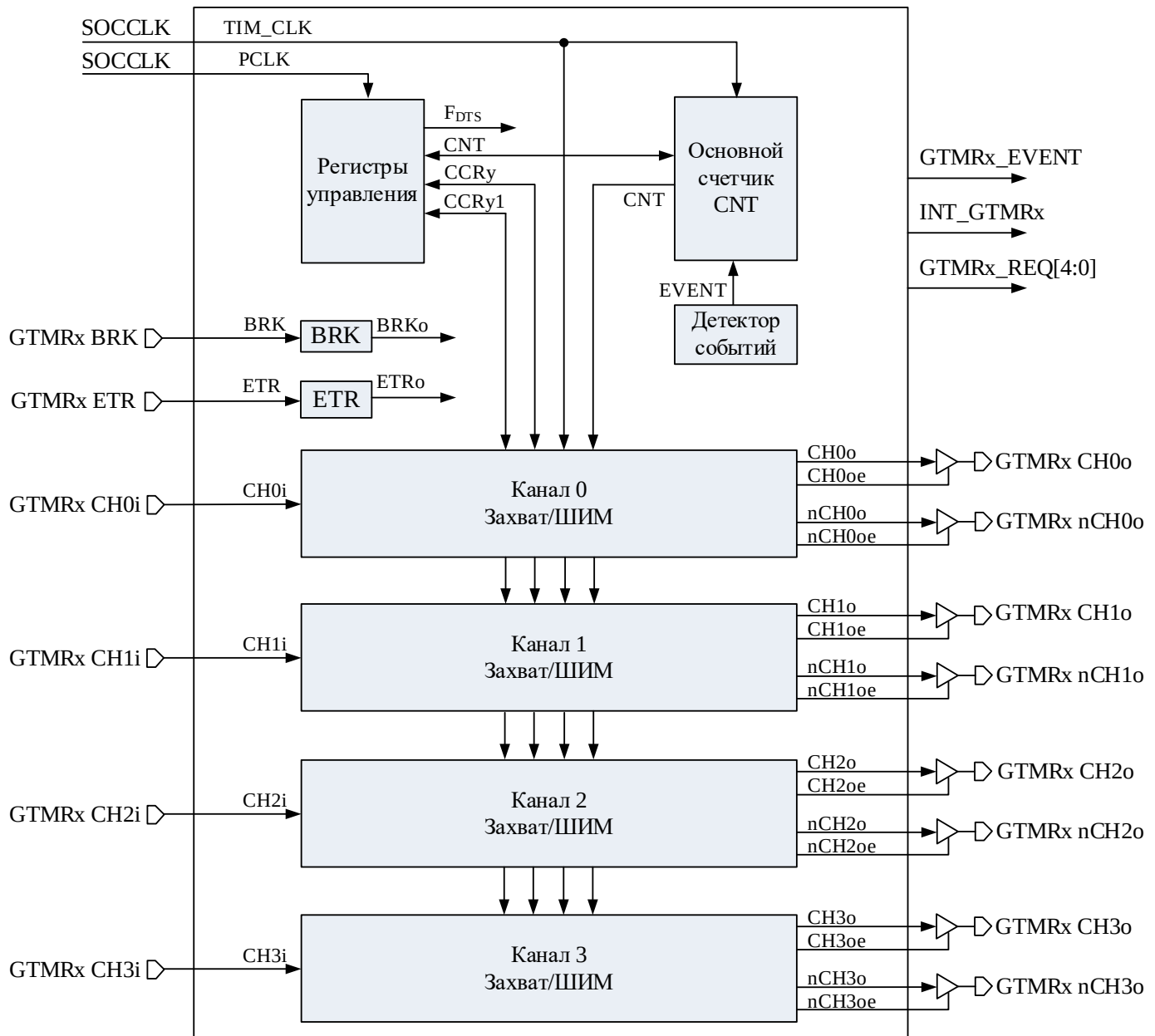
Рисунок 19 – Структурная схема блока «Таймер»
