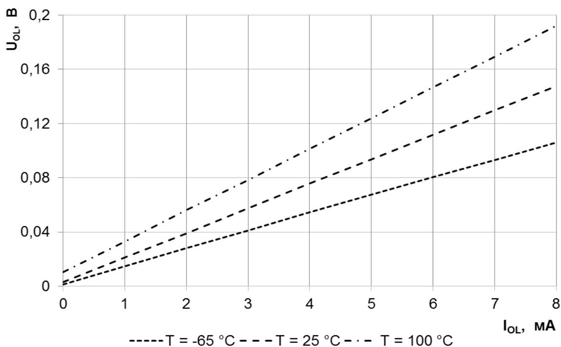
Рисунок 176 – Зависимость выходного напряжения низкого уровня U_{OL} от выходного тока низкого уровня при U_{CC} = 1,08\text{ В} , U_{CCIO} = 3,0\text{ В}
