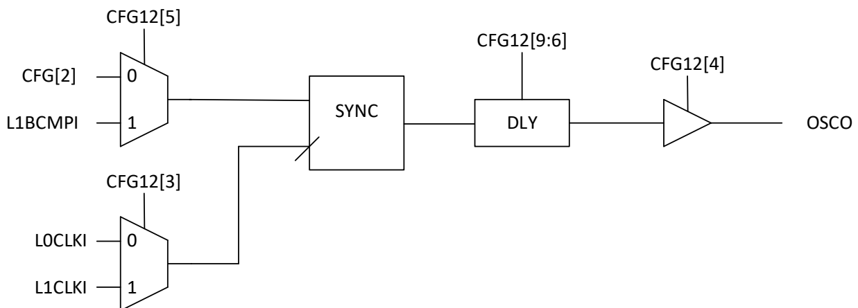
Рисунок 171 – Схема формирования внешнего импульса синхронизации
