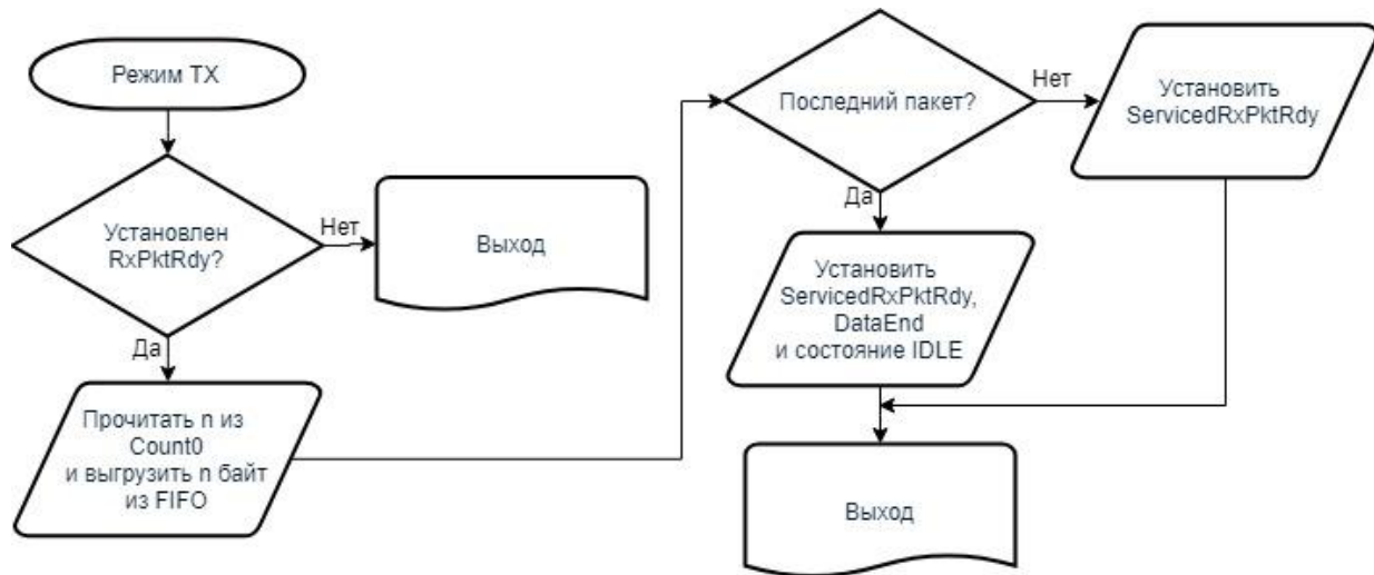
Рисунок 113 – Алгоритм режима RX
