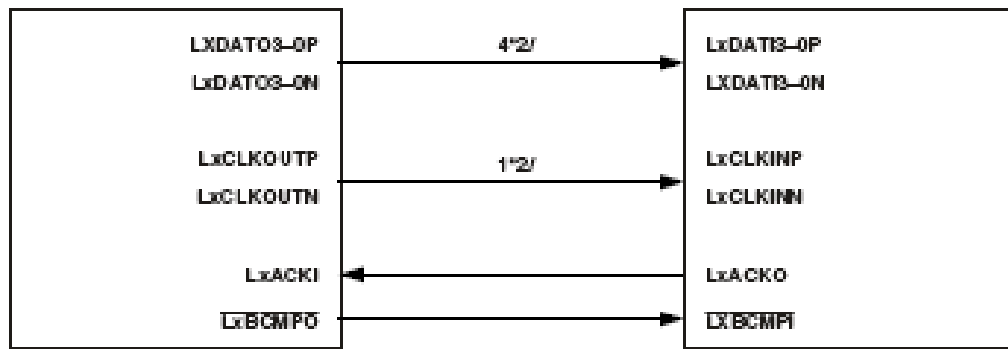
Рисунок 72 – Конфигурация порта связи (четырёхразрядный режим)
