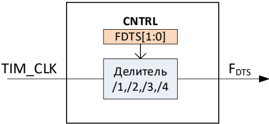
Рисунок 24 – Схема формирования тактовой частоты F DTS
