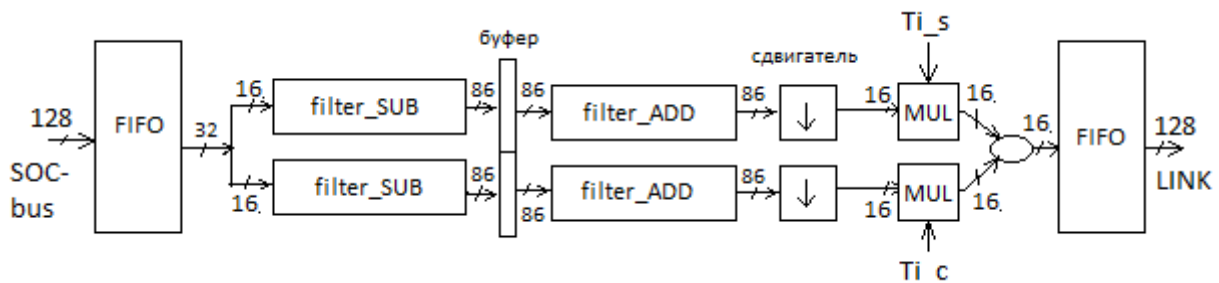
Рисунок 155 – Структура модуля в режиме UP
