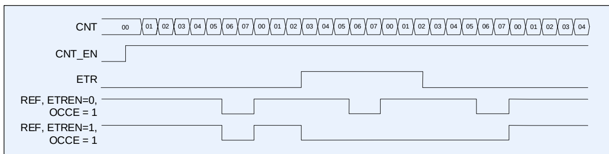
Рисунок 40 – Диаграмма сброса сигнала REF по выводу ETR
