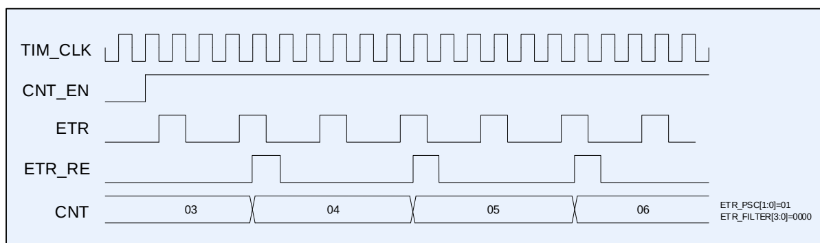
Рисунок 34 – Диаграмма тактирования со входа ETR, EVENT\_SEL[3:0] = 1000
