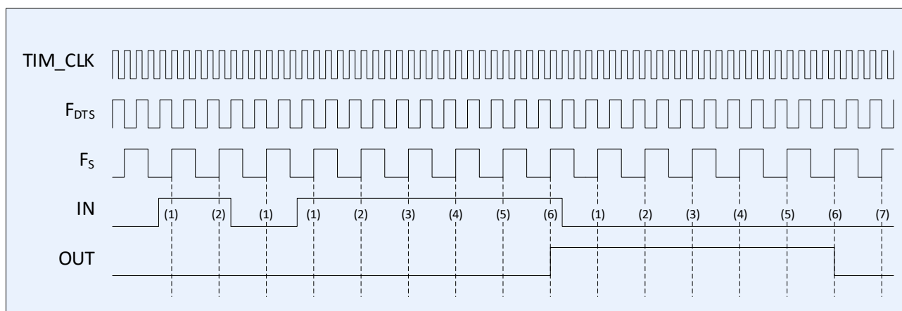
Рисунок 44 – Диаграмма работы фильтра, F_S = F_{DTS}/2 , N = 6
