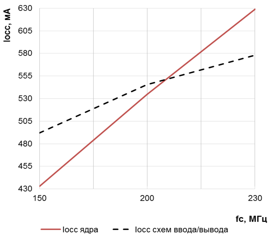
Рисунок 184 – Зависимость динамического тока потребления I_{OCC} ядра и схем ввода/вывода от тактовой частоты процессора f_C при U_{CC} = 1,32 \text{ В} , U_{CCIO} = U_{CCA} = 3,6 \text{ В} , T = 25 \text{ °C}
