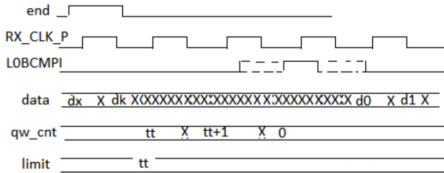
Рисунок 89. Временная диаграмма завершения приёма, инициированного по сигналу события (вход L0BCMPI).
