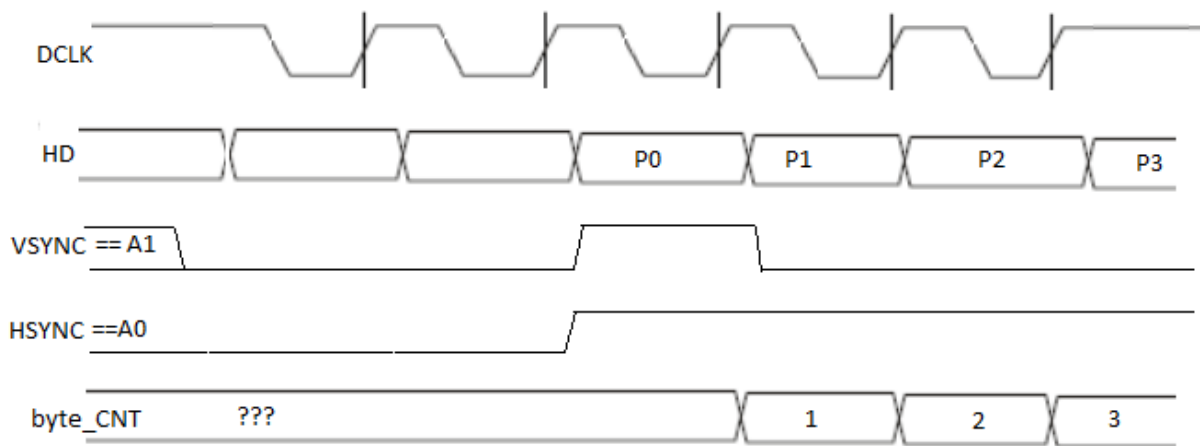
Рисунок 95 – Начало приема данных в режиме «ведущее устройство»
