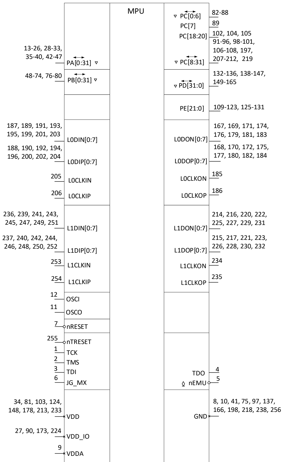
Рисунок 2 – Условное графическое обозначение
