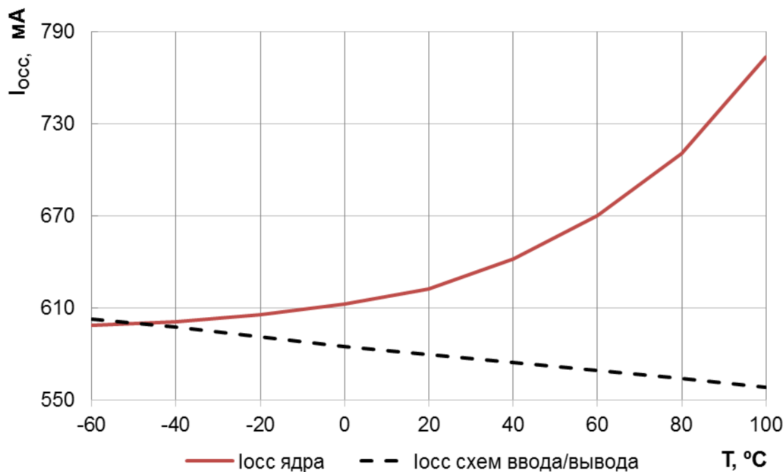
Рисунок 179 – Зависимость динамического тока потребления I_{\text{осс}} ядра и схем ввода/вывода от температуры при U_{\text{CC}} = 1,32 \text{ В} , U_{\text{CCIO}} = U_{\text{CCA}} = 3,6 \text{ В} , f_{\text{C}} = 230 \text{ МГц}
