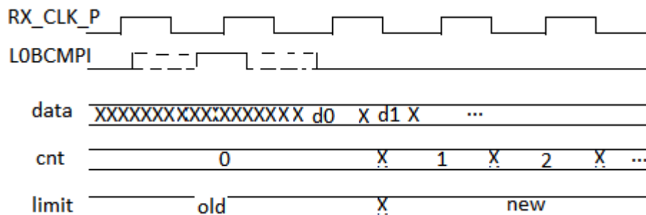
Рисунок 88. Временная диаграмма старта приёма по внешнему событию (импульс на L0BCMPI ).
