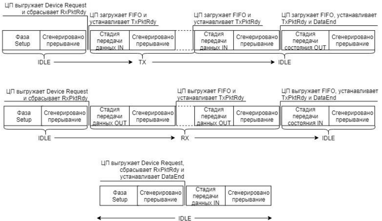
Рисунок 110 – Диаграмма передачи данных
