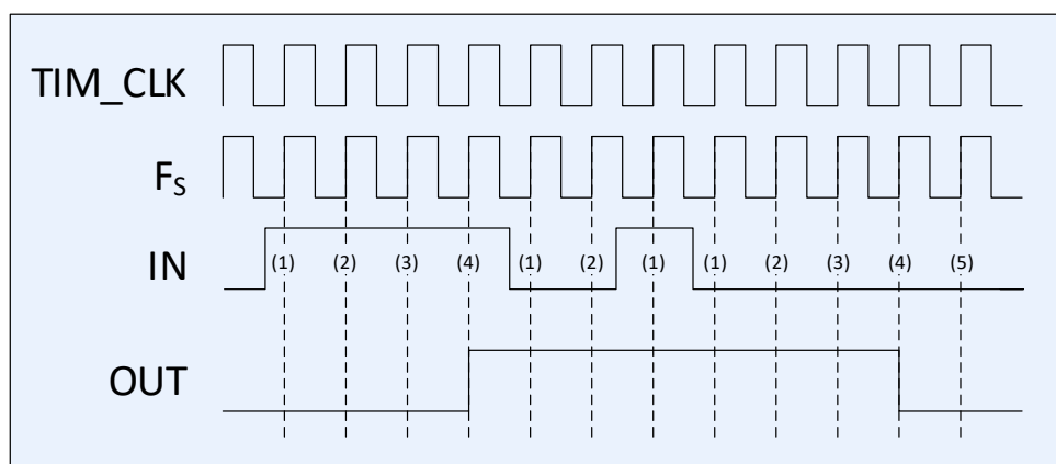
Рисунок 43 – Диаграмма работы фильтра, F_S = \text{TIM\_CLK} , N = 4
