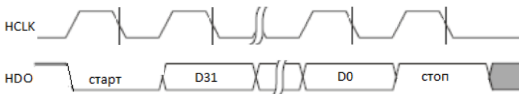
Рисунок 69 – Передача информации контроллером интерфейса
