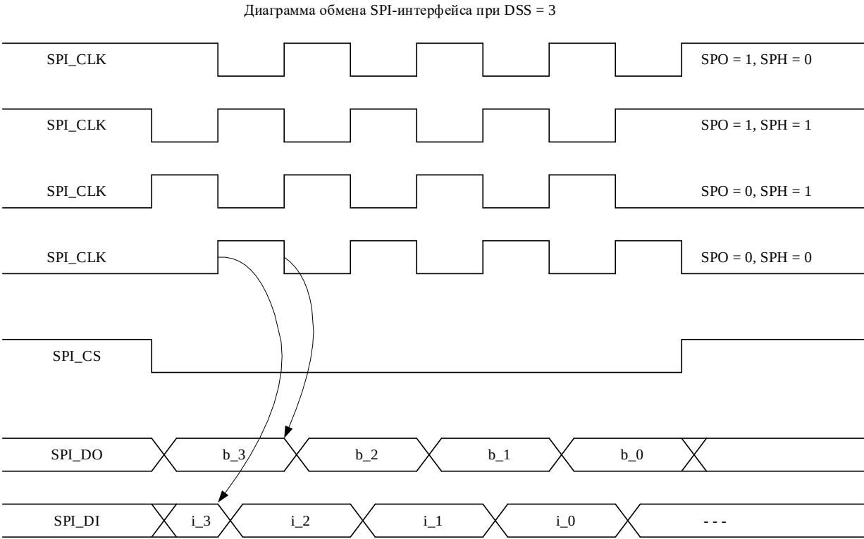
Рисунок 91 – Диаграмма обмена в режиме master
