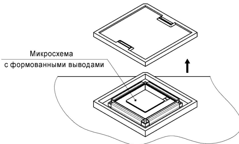
Рисунок 193 – Схема открытия крышки контейнера
