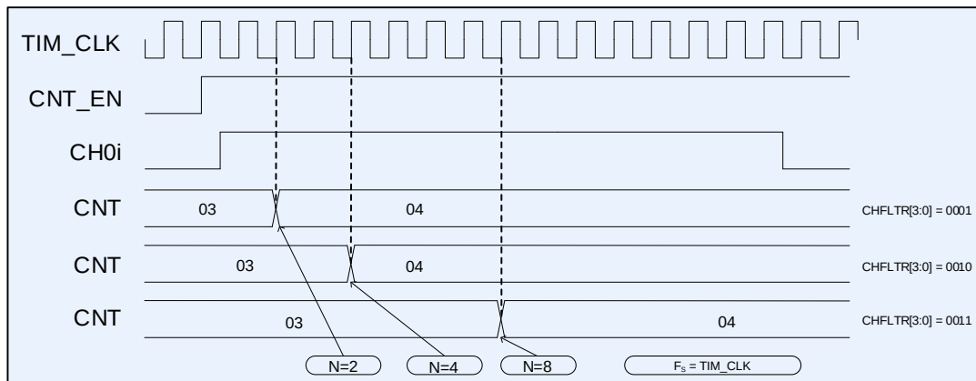
Рисунок 32 – Диаграмма внешнего тактирования с разными вариантами фильтра
