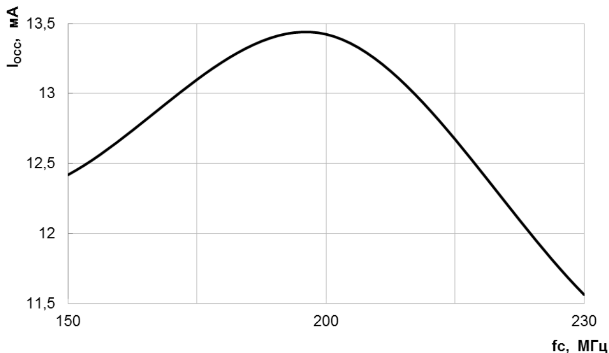
Рисунок 185 – Зависимость динамического тока потребления аналоговых блоков I_{OCC} от тактовой частоты процессора f_C при U_{CC} = 1,32 В, U_{CCIO} = U_{CCA} = 3,6 В, T = 25 °С
