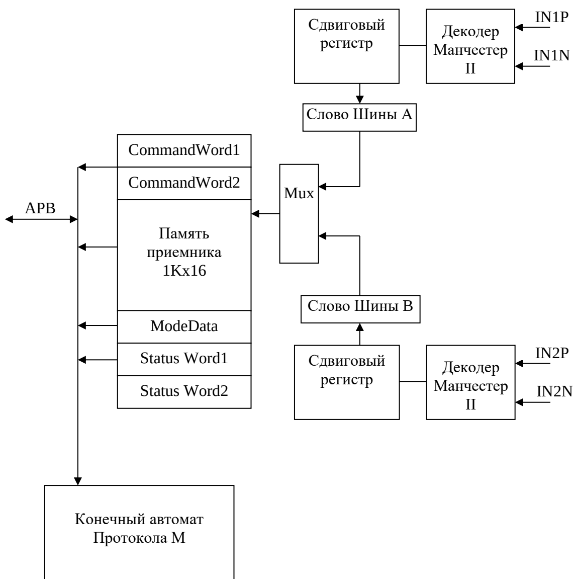
Рисунок 152 – Структурная схема работы в режиме М
