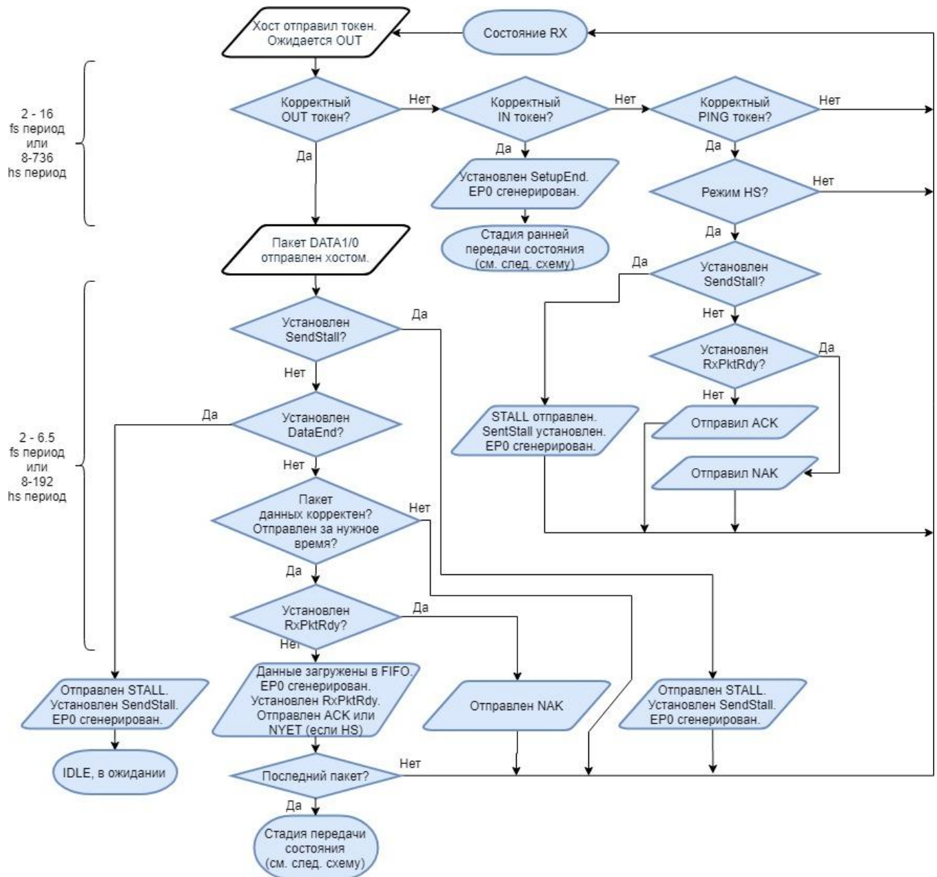
Рисунок 117 – Фаза передачи данных OUT
