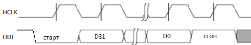
Рисунок 68 – Прием информации контроллером интерфейса
