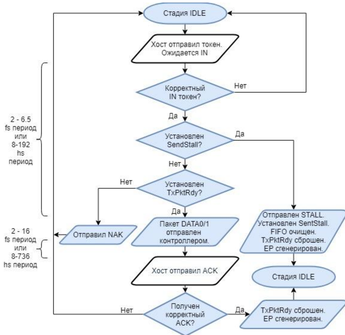
Рисунок 119 – Передача транзакций IN
