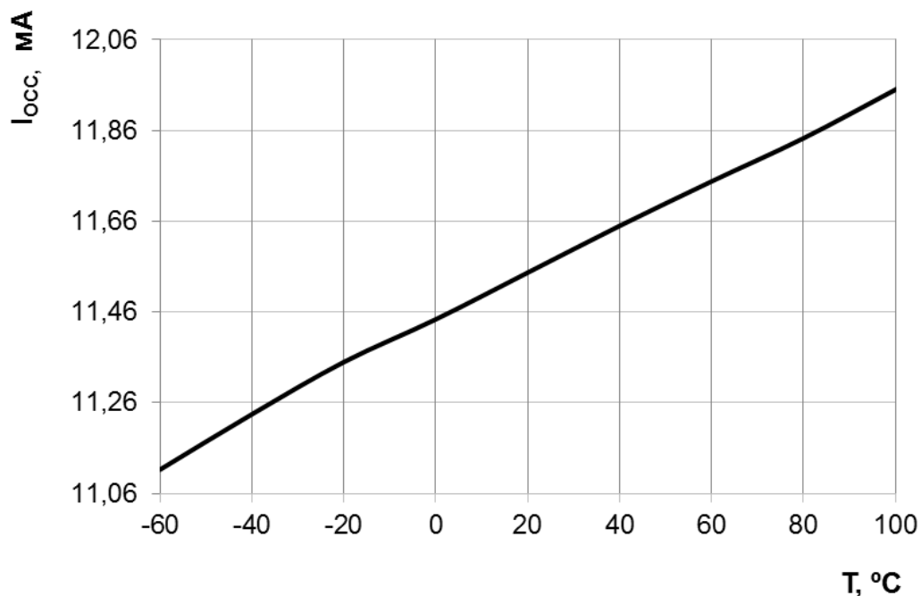
Рисунок 180 – Зависимость динамического тока потребления I_{\text{осс}} аналоговых блоков от температуры при U_{\text{CC}} = 1,32 \text{ В} , U_{\text{CCIO}} = U_{\text{CCA}} = 3,6 \text{ В}
