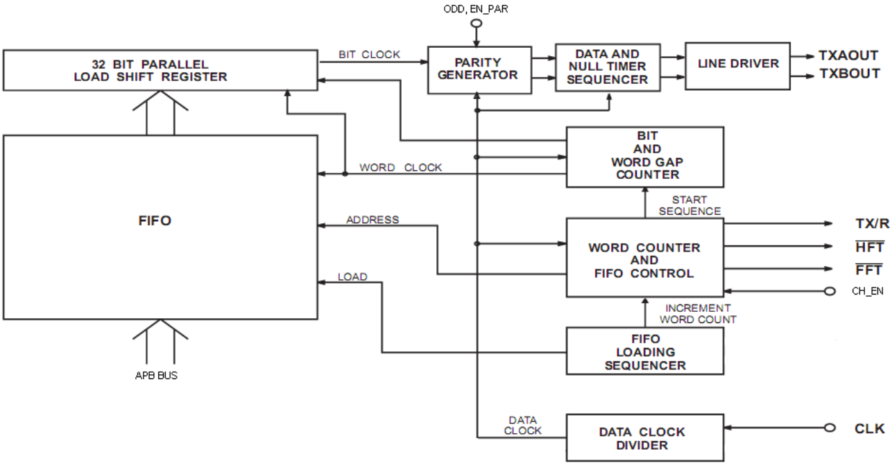
Рисунок 145 – Структурная схема канала передачи
