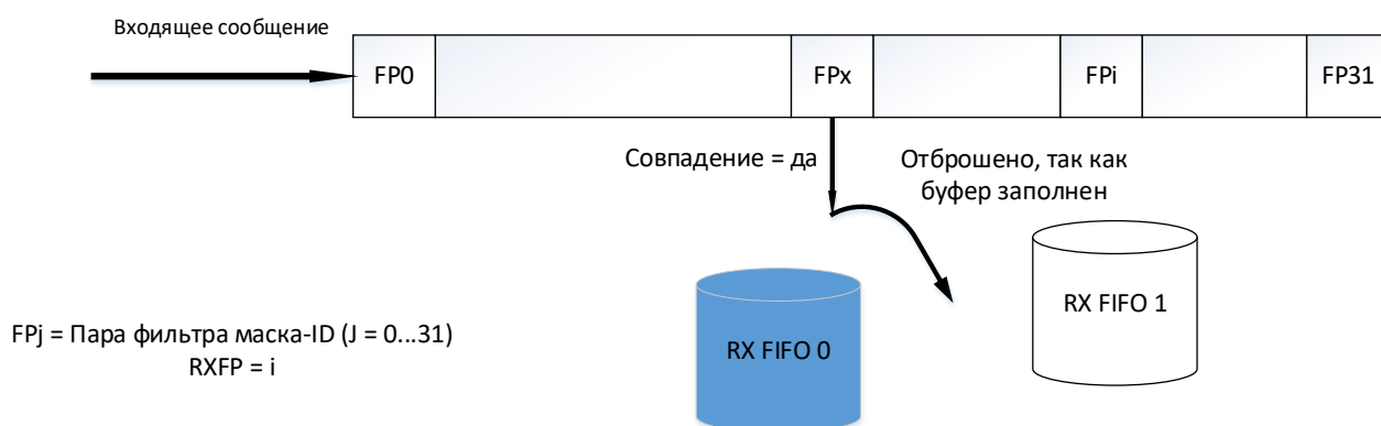
Рисунок 140 – отбрасывание сообщения (RX FIFO 0 заполнен, но совпадение)
