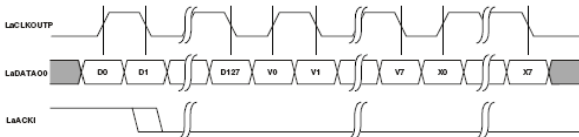
Рисунок 81 – Порт связи «a» передает порту связи «b» с верификацией
