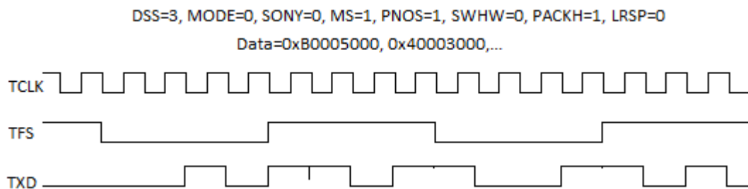
Рисунок 104 – Выдача информации по срезу TCLK
