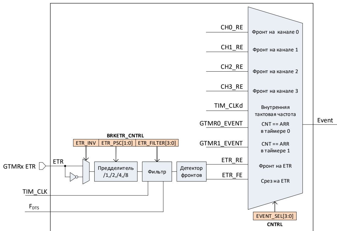
Рисунок 33 – Схема тактирования сигналом со входа ETR
