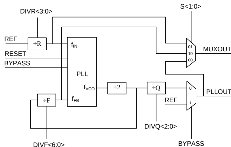
Рисунок 170 – Структура PLL
