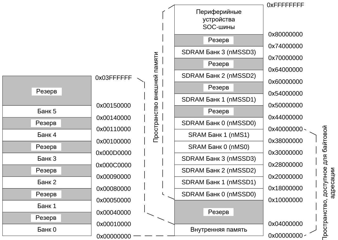
Рисунок 9 – Карта памяти с включенной дополнительной областью
