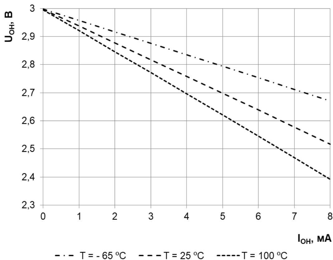
Рисунок 175 – Зависимость выходного напряжения высокого уровня U_{OH} от выходного тока высокого уровня при U_{CC} = 1,08\text{ В} , U_{CCIO} = 3,0\text{ В}
