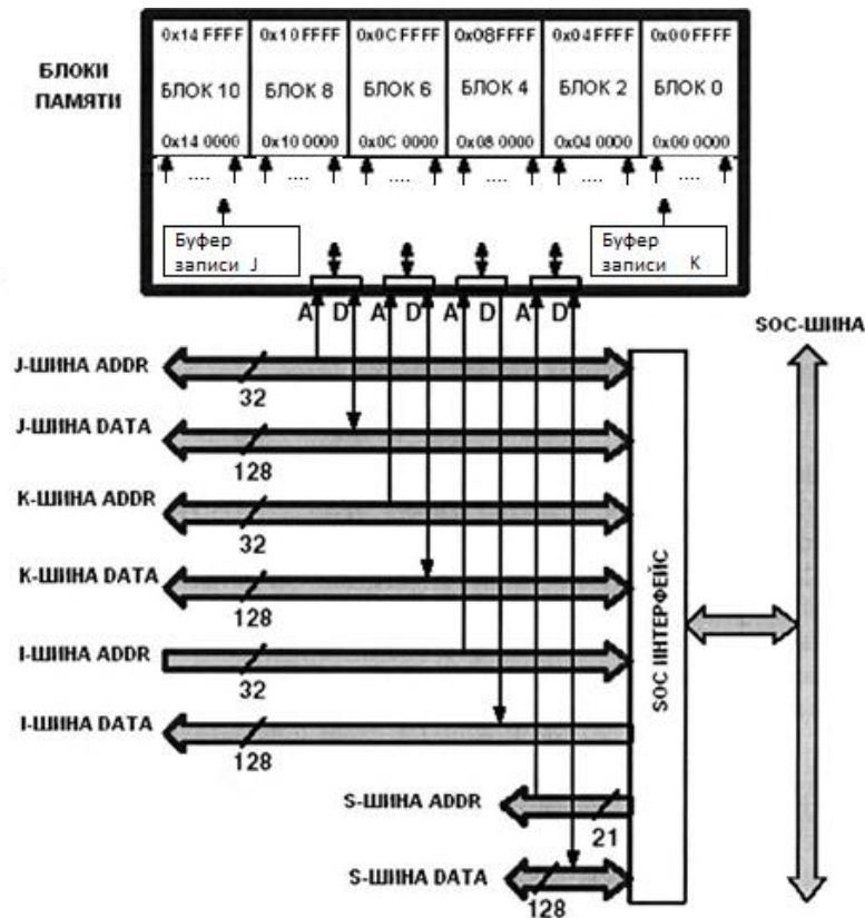
Рисунок 4 – Подключение внутренней памяти к ядру процессора
