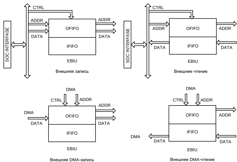
Рисунок 53 – Передача данных через интерфейс внешней шины (EBIU)
