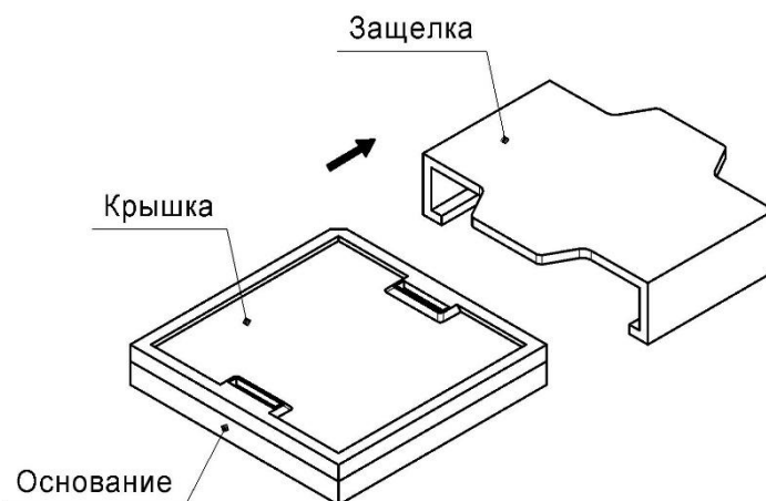
Рисунок 192 – Схема сдвига защелки контейнера
