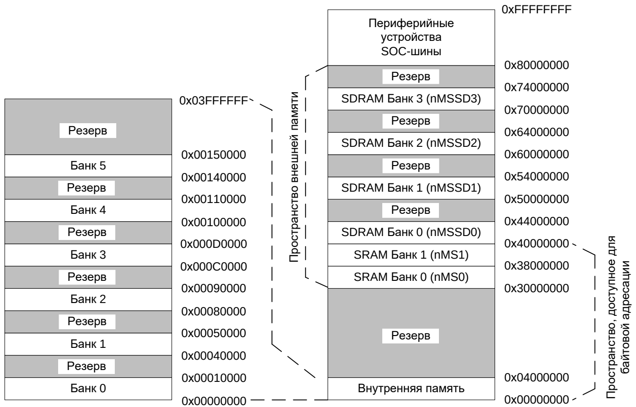
Рисунок 8 – Базовая карта памяти
