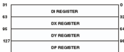
Рисунок 52 – Регистры блока управления передачей
