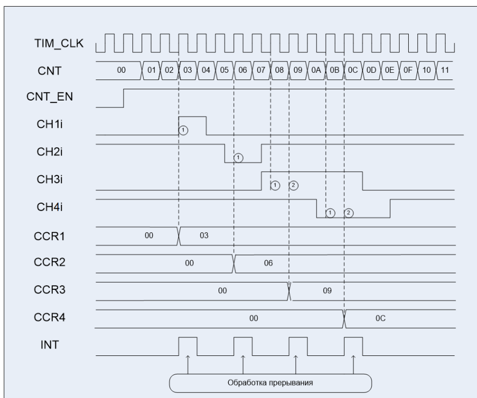
Рисунок 87 – Диаграммы примера работы в режиме захвата
