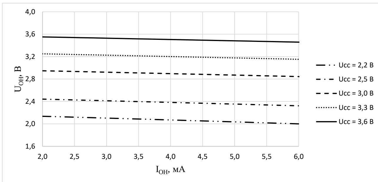
Рисунок 145 – Зависимость выходного напряжения высокого уровня U_{OH} от выходного тока высокого уровня I_{OH} при разном напряжении питания при T = -60^\circ\text{C}
