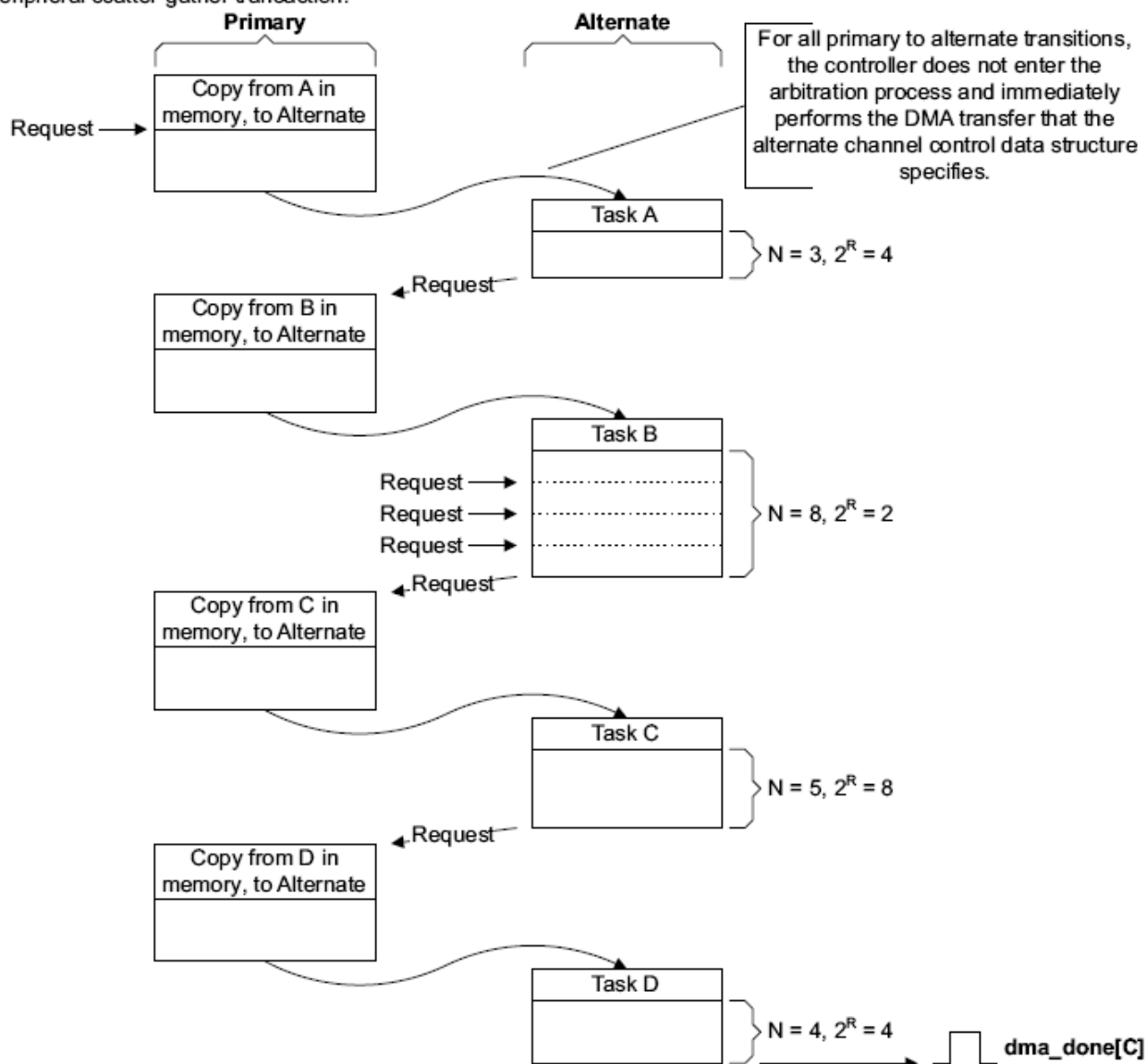
Рисунок 130 – Пример работы DMA в режиме с «Исполнением с изменением конфигурации»
