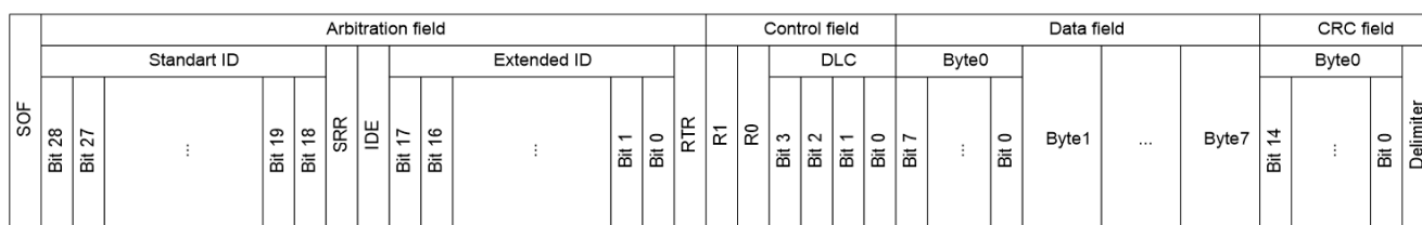
Рисунок 49 – Структура расширенного пакета данных
