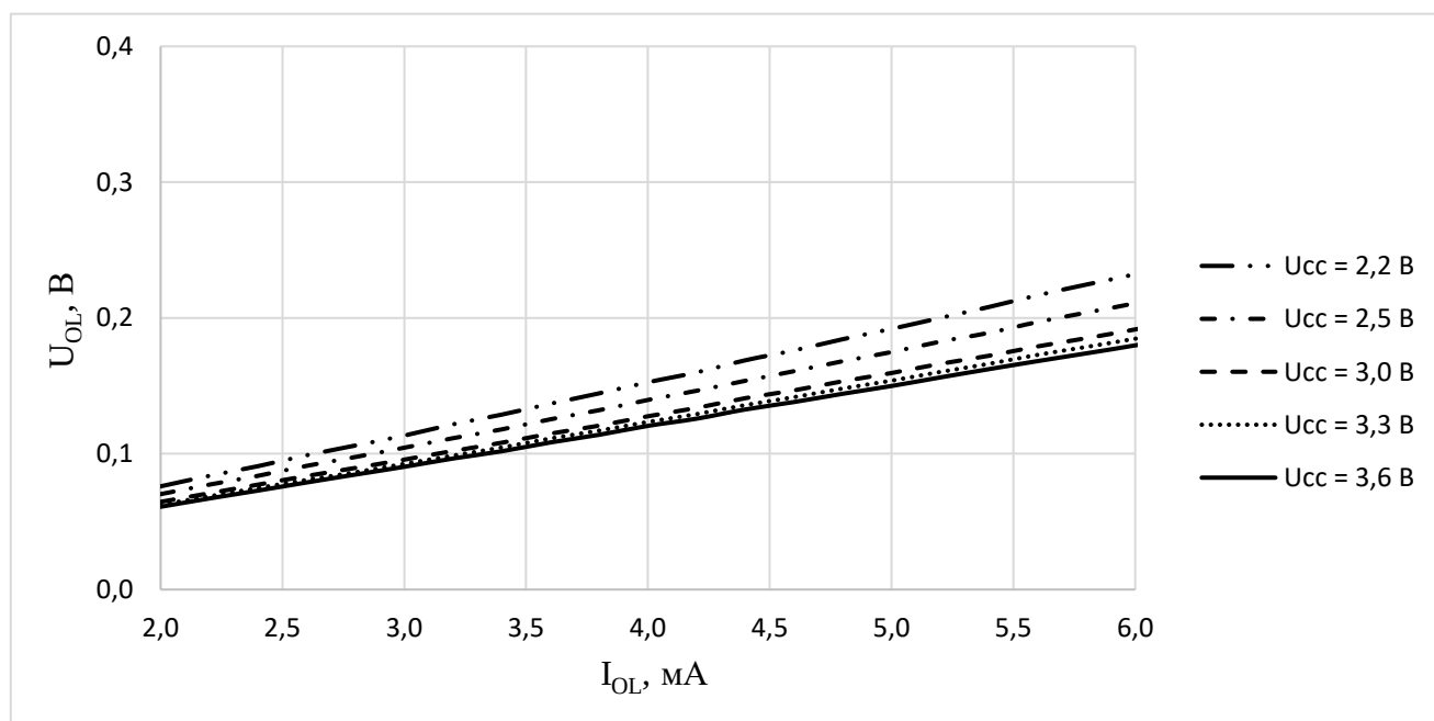
Рисунок 147 – Зависимость выходного напряжения низкого уровня U_{OL} от выходного тока низкого уровня I_{OL} при разном напряжении питания при T_a = (25 \pm 10)^\circ\text{C}
