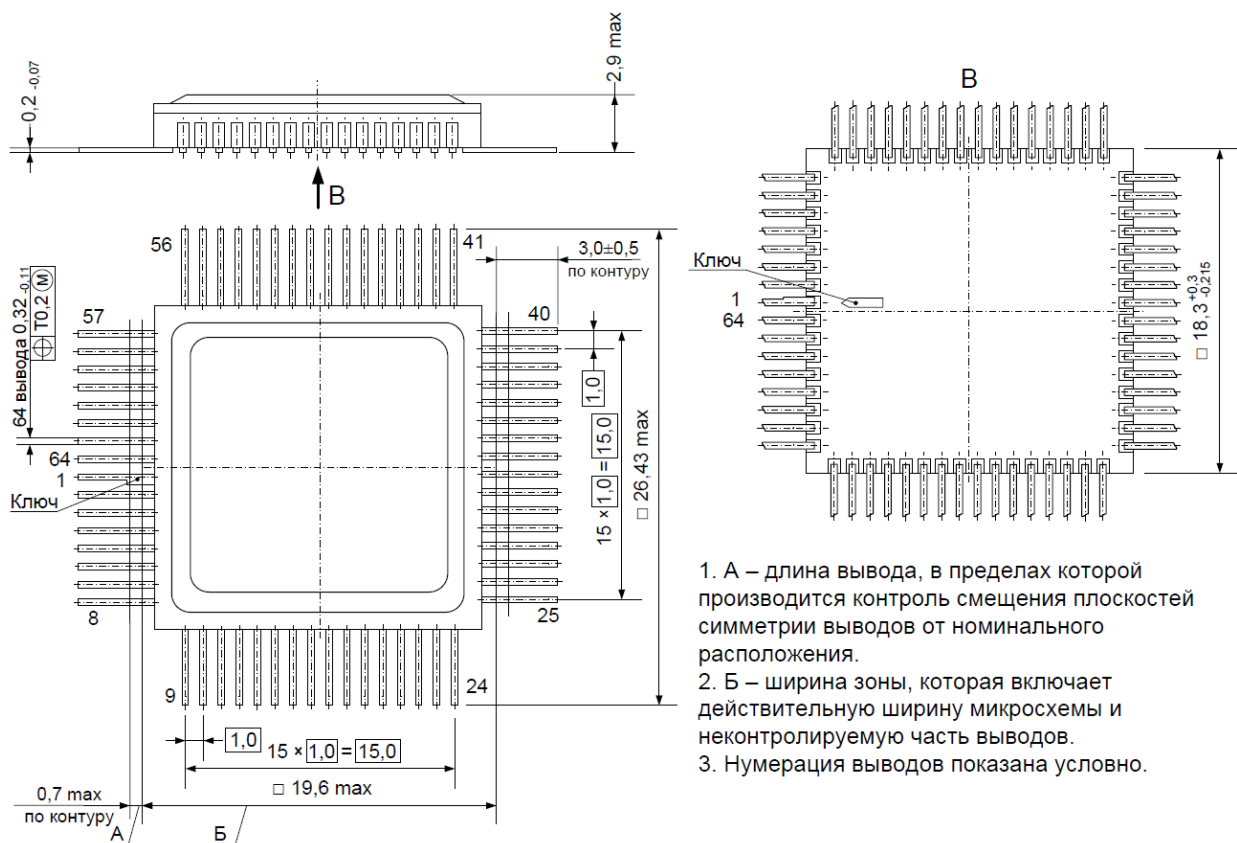
Рисунок 152 – Габаритный чертеж микросхемы в корпусе N18.64-1B
