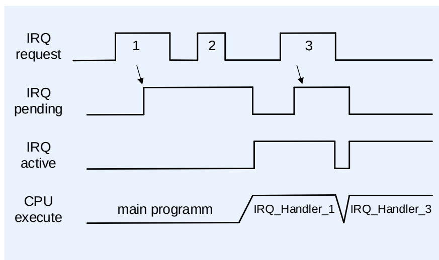
Рисунок 140 – Повторная установка запроса на прерывание в момент выполнения обработчика исключения
