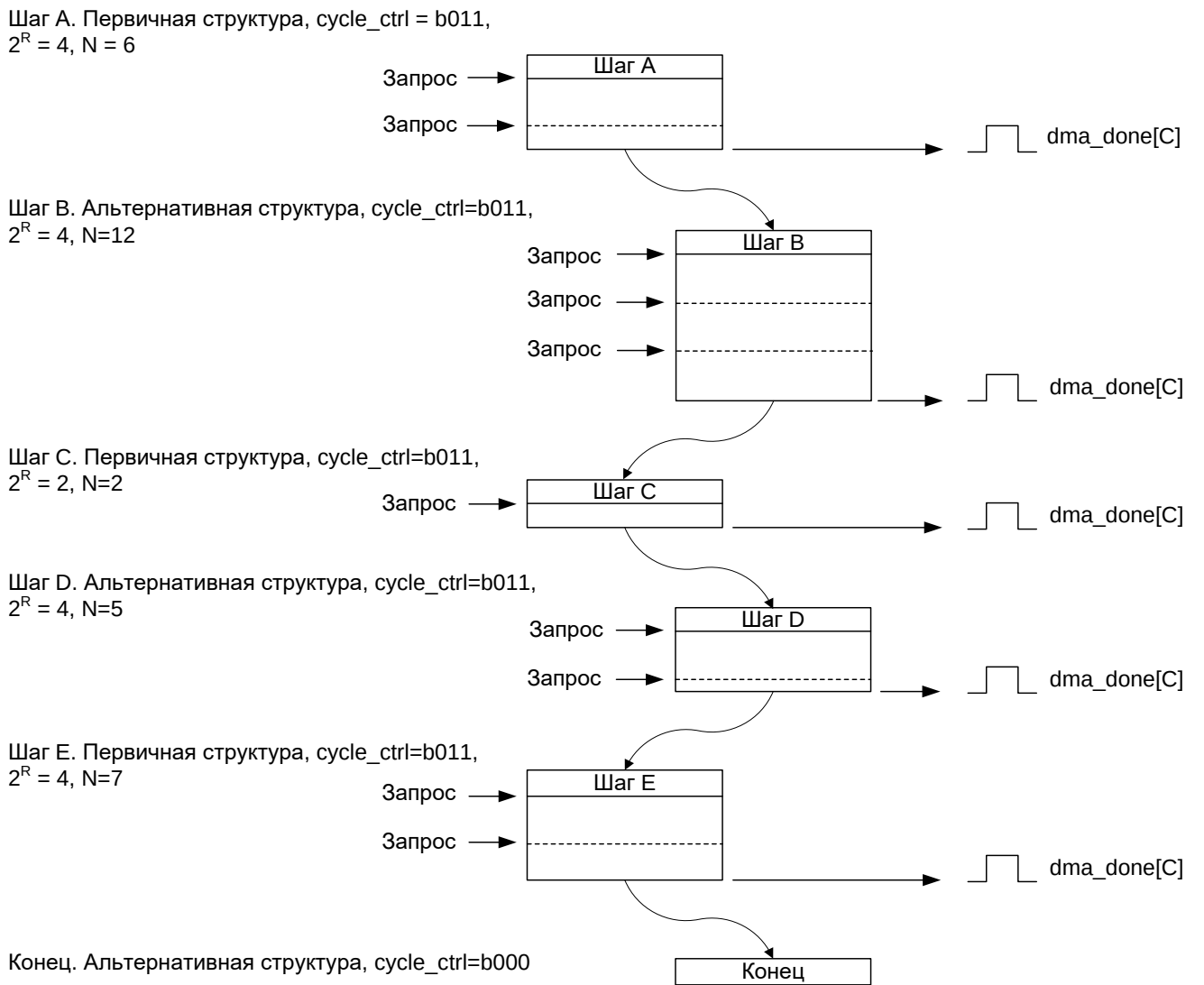
Рисунок 128 – Пример функционирования контроллера в режиме «пинг-понг»
