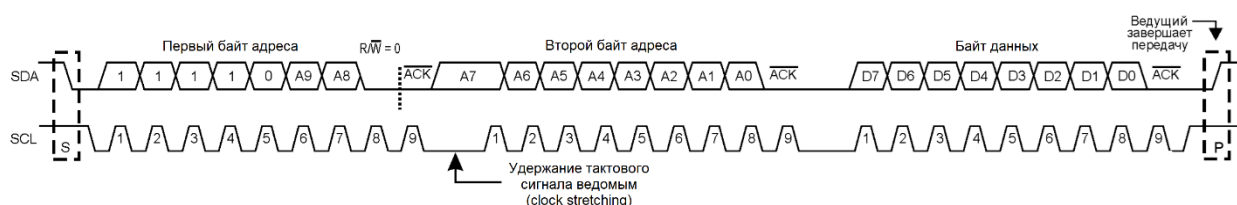
Рисунок 97 – Передача по I2C в 10-битном режиме
