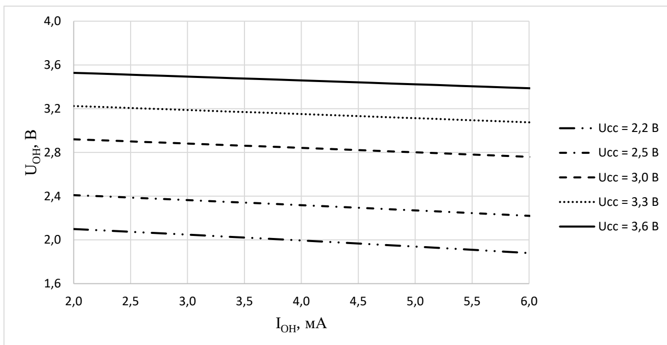
Рисунок 146 – Зависимость выходного напряжения высокого уровня U_{OH} от выходного тока высокого уровня I_{OH} при разном напряжении питания при T = 125^\circ\text{C}
