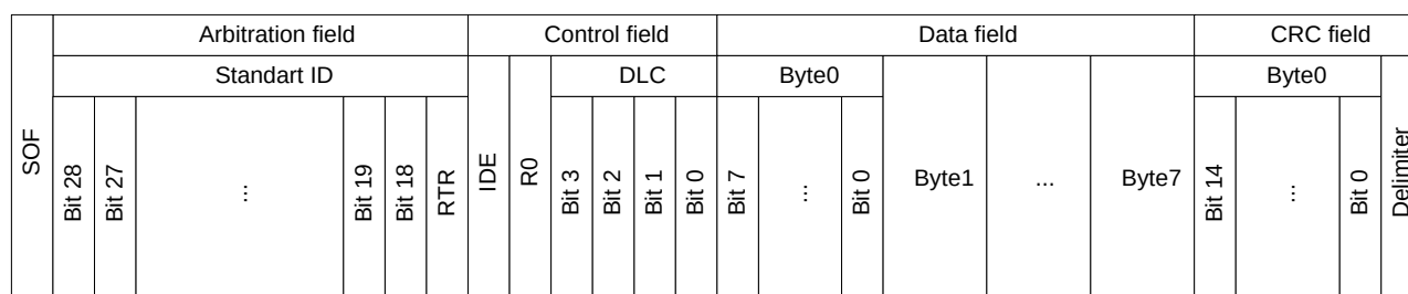
Рисунок 48 – Структура стандартного пакета данных
