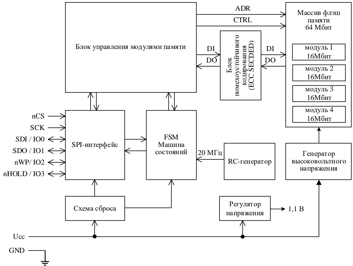
Рисунок 1 – Структурная блок-схема
