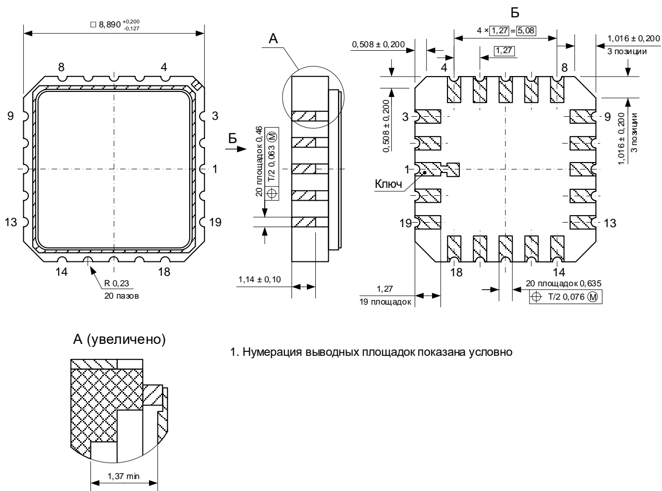
Рисунок 39 – Микросхема в корпусе МК 5121.20-А
