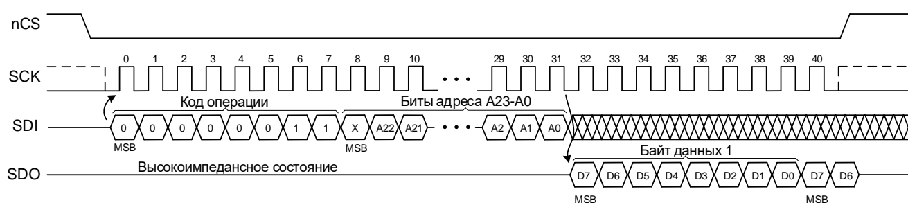
Рисунок 5 – Операция чтения с кодом 03h
