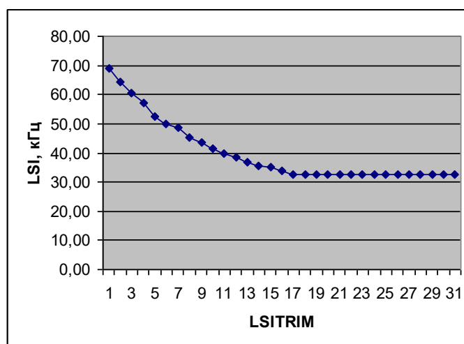
Рисунок 31 – Зависимость частоты LSI от значения LSITRIM
