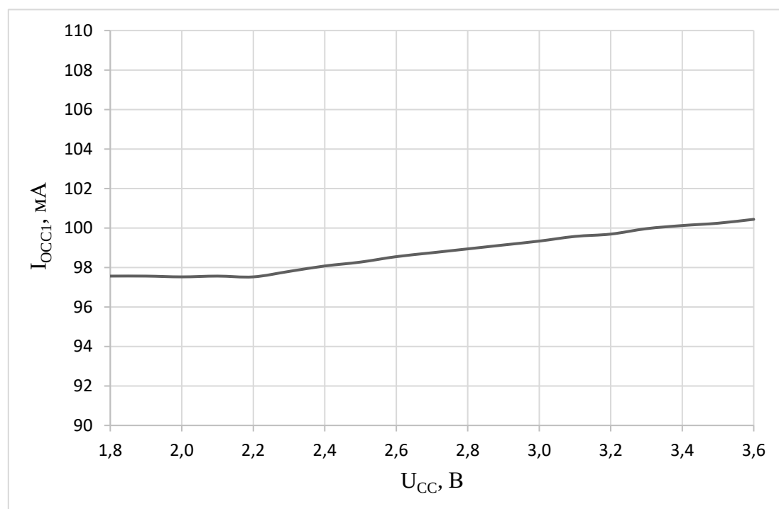
Рисунок 147 – Зависимость динамического тока потребления I_{OCC1} от напряжения питания U_{CC} при f_C = 80 МГц, T_a = (25 \pm 10) °C
