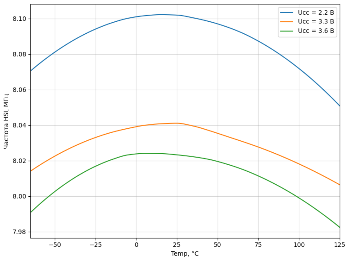
Рисунок 143 – Зависимость частоты HSI от температуры при типовом HSITRIM
