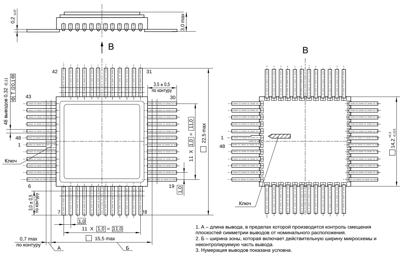
Рисунок 158 – Габаритный чертеж микросхемы в корпусе N16.48-1B
