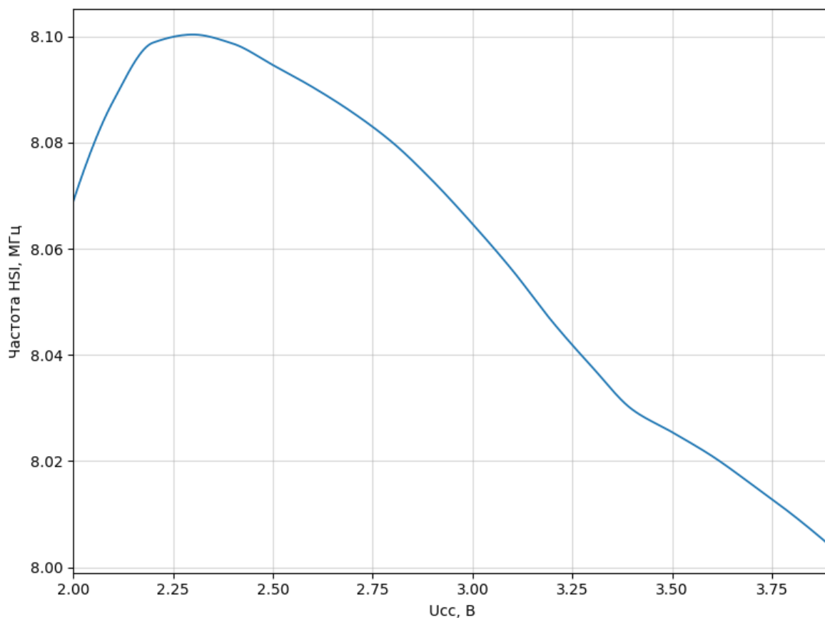
Рисунок 142 – Зависимость частоты HSI от напряжения питания при типовом HSITRIM
