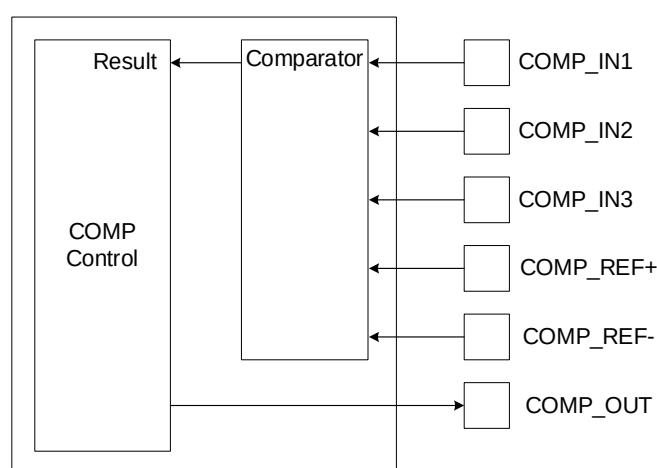
Рисунок 92 – Структура блока компаратора
