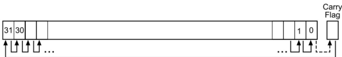
Рисунок 27 – Инструкция RRX
