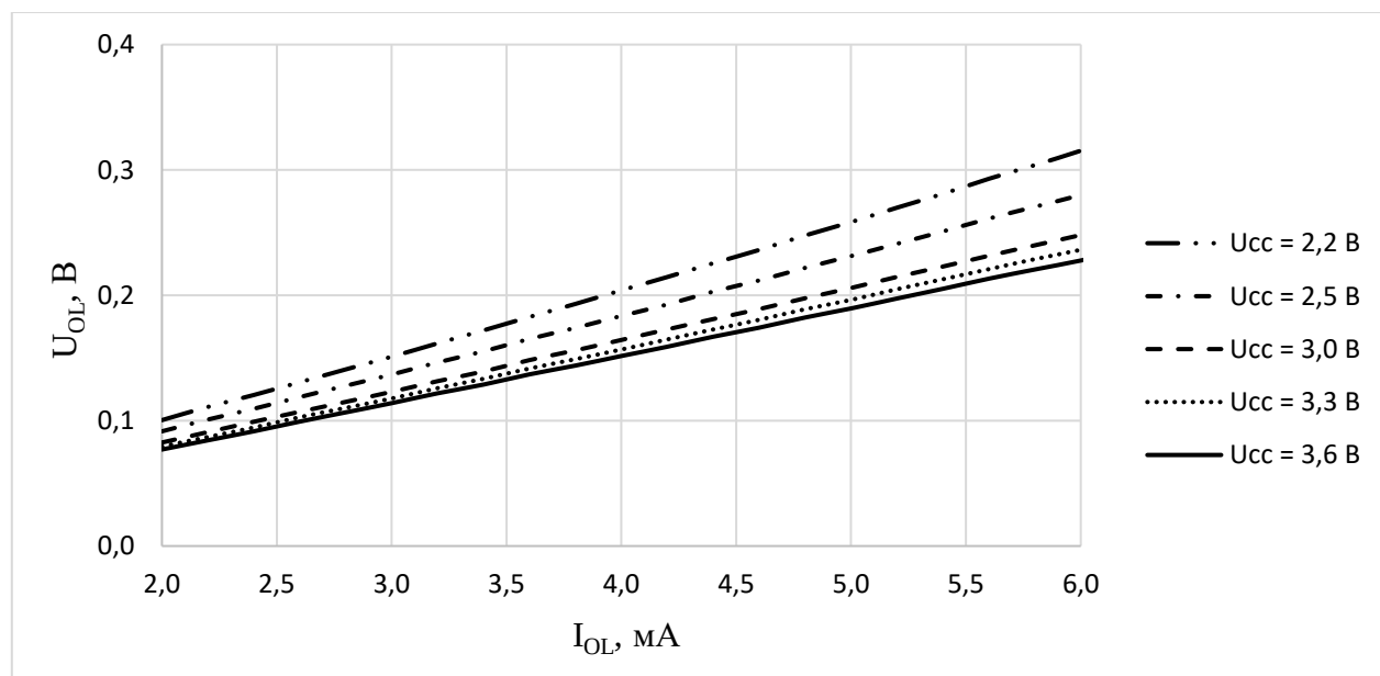
Рисунок 153 – Зависимость выходного напряжения низкого уровня U_{OL} от выходного тока низкого уровня I_{OL} при разном напряжении питания при T = 125\text{ }^{\circ}\text{C}
