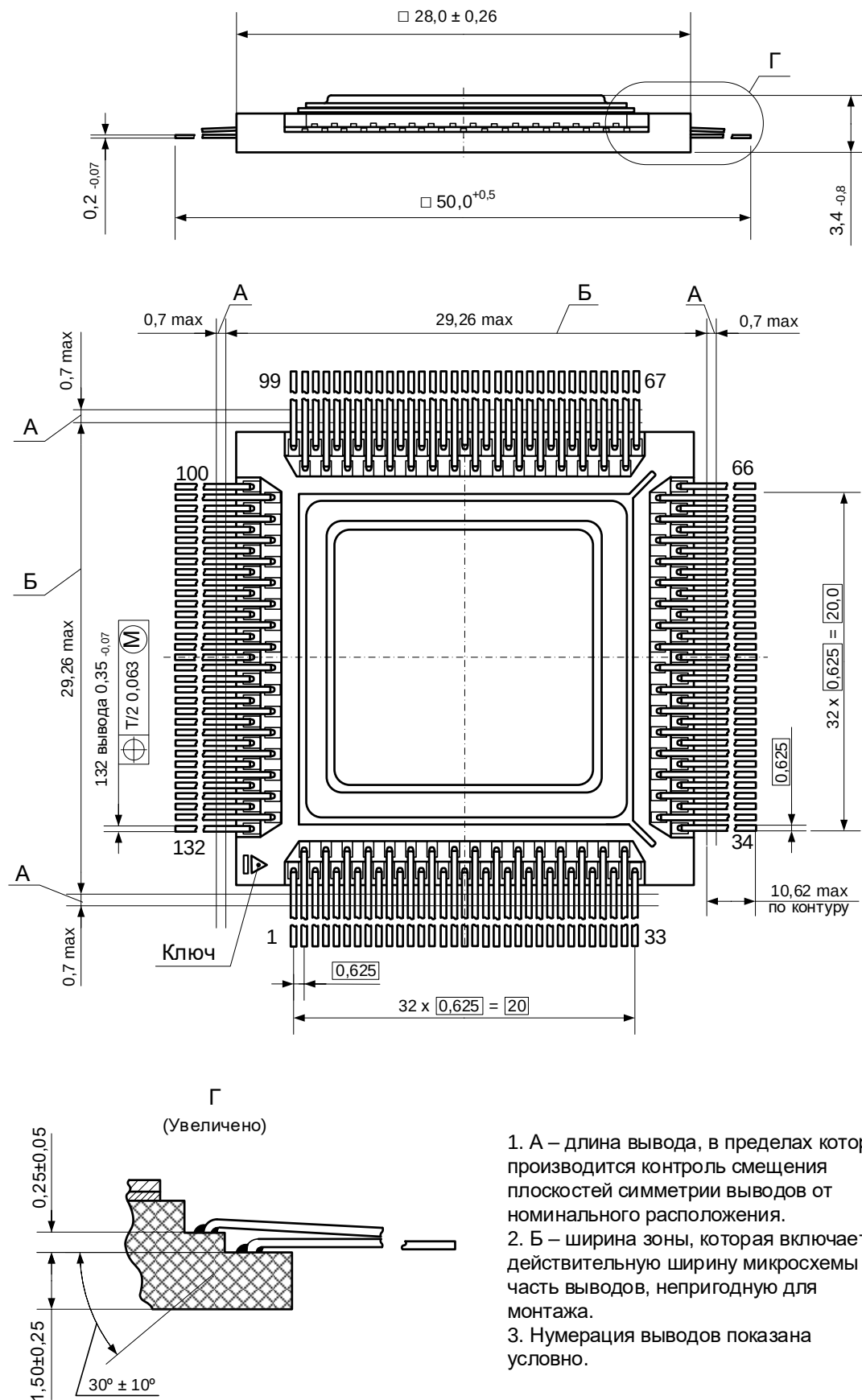
Рисунок 154 – Габаритный чертеж микросхемы в корпусе 4229.132-3
