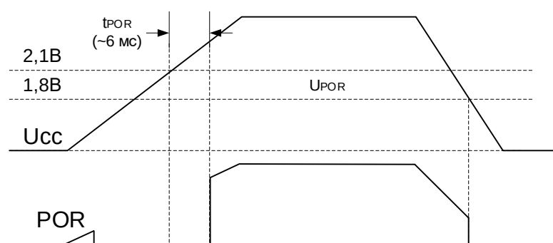
Рисунок 8 – Сигнал сброса при включении и выключении основного напряжения питания
