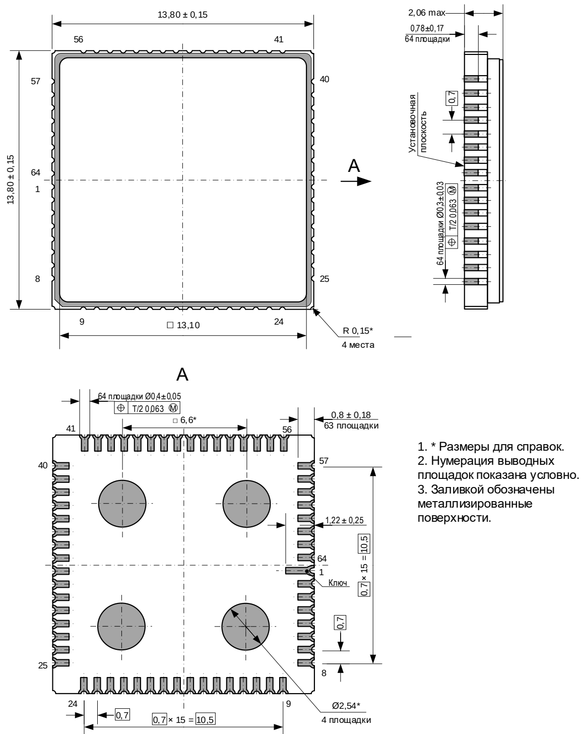
Рисунок 157 – Габаритный чертеж микросхемы в корпусе МК 5153.64-2
