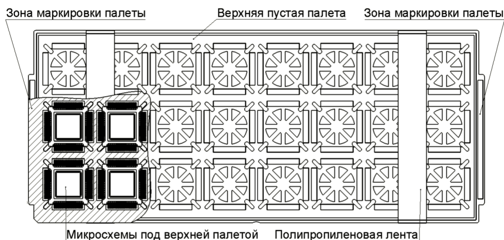
Рисунок 161 – Стопка палет. Вид сверху
