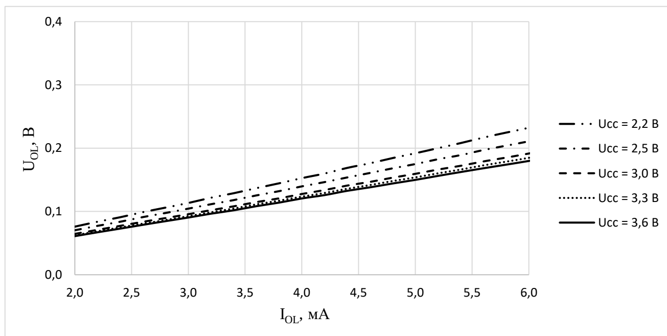
Рисунок 151 – Зависимость выходного напряжения низкого уровня U_{OL} от выходного тока низкого уровня I_{OL} при разном напряжении питания при T_a = (25 \pm 10)\text{ °C}
