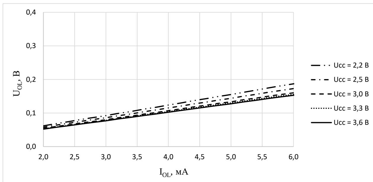
Рисунок 152 – Зависимость выходного напряжения низкого уровня U_{OL} от выходного тока низкого уровня I_{OL} при разном напряжении питания при T = -60\text{ }^{\circ}\text{C}
