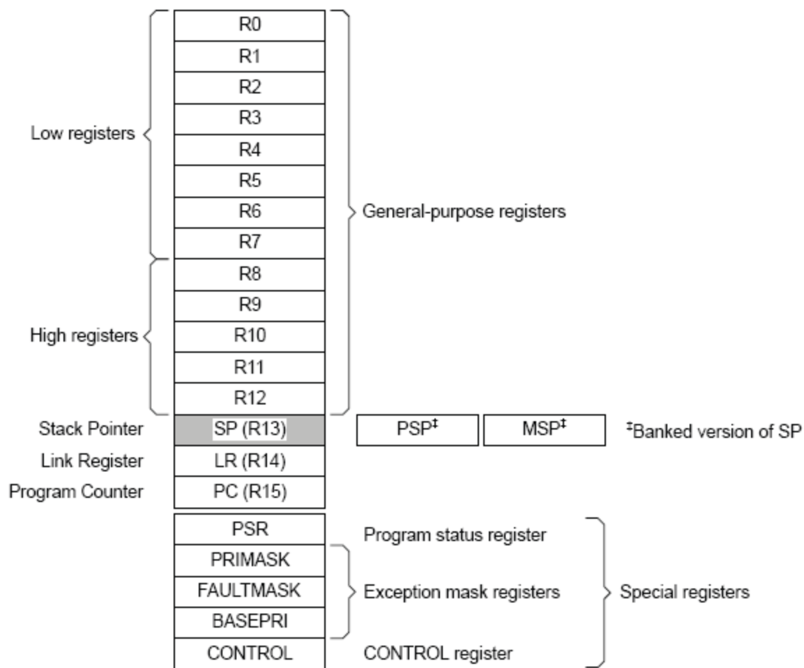
Рисунок 22 – Регистры ядра
