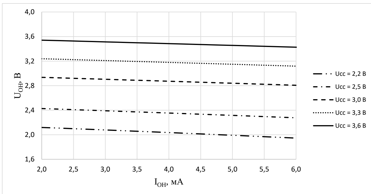
Рисунок 148 – Зависимость выходного напряжения высокого уровня U_{OH} от выходного тока высокого уровня I_{OH} при разном напряжении питания при T_a = (25 \pm 10)^\circ\text{C}
