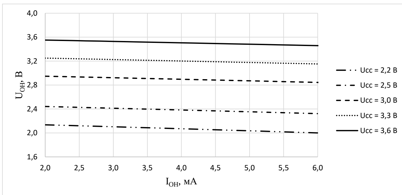
Рисунок 149 – Зависимость выходного напряжения высокого уровня U_{OH} от выходного тока высокого уровня I_{OH} при разном напряжении питания при T = -60^\circ\text{C}
