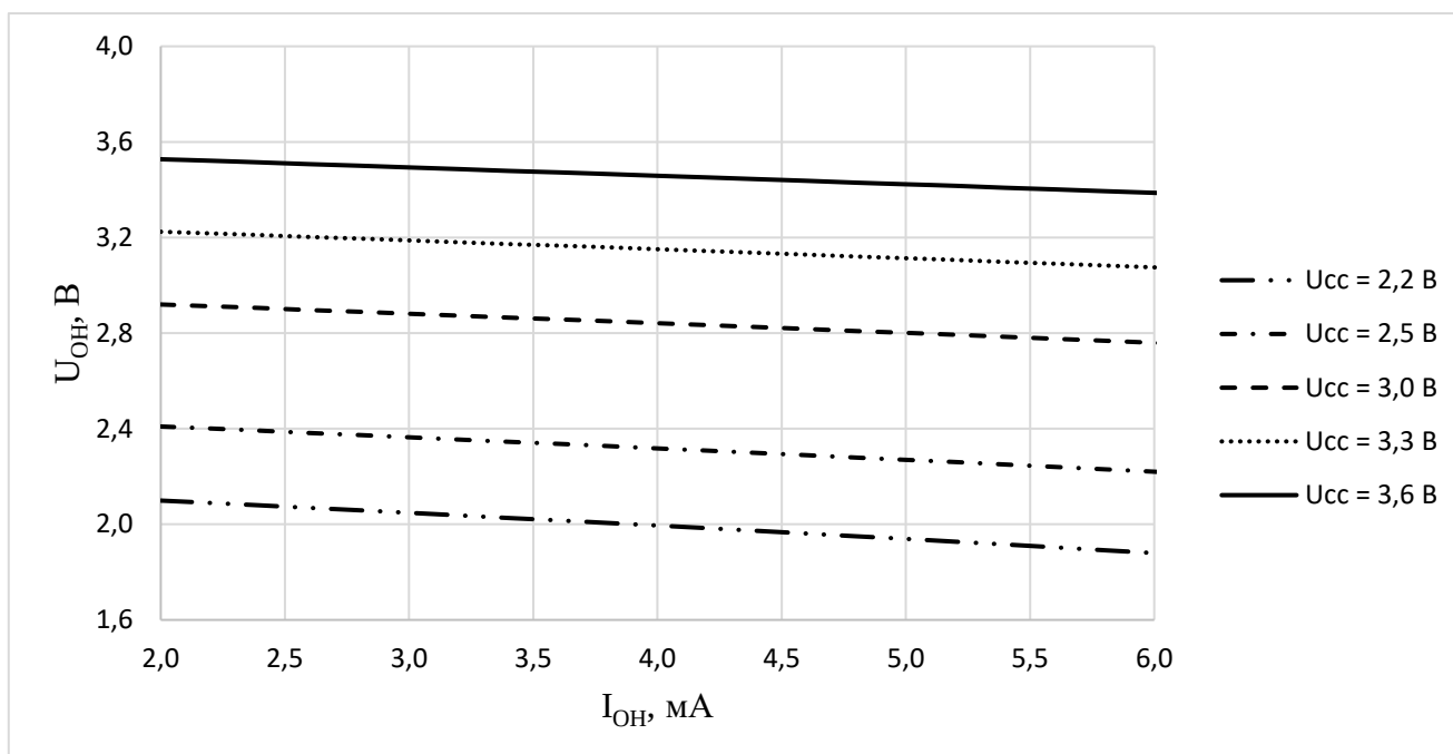
Рисунок 150 – Зависимость выходного напряжения высокого уровня U_{OH} от выходного тока высокого уровня I_{OH} при разном напряжении питания при T = 125\text{ °C}
