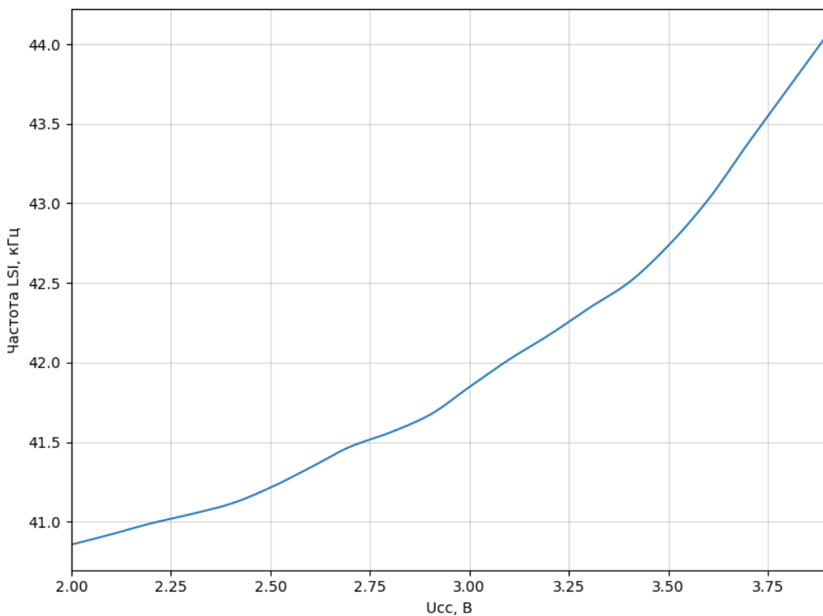
Рисунок 144 – Зависимость частоты LSI от напряжения питания при типовом LSITRIM
