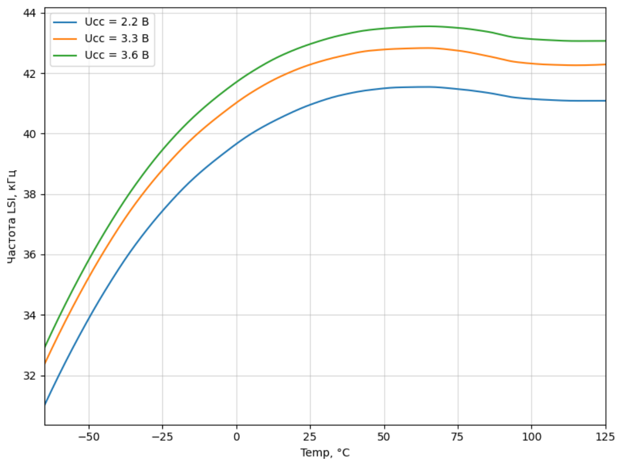
Рисунок 145 – Зависимость частоты LSI от температуры при типовом LSITRIM
