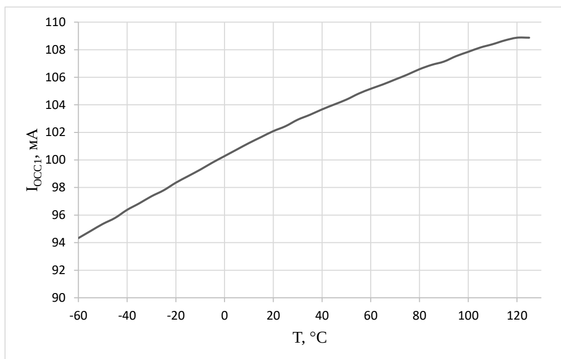
Рисунок 146 – Зависимость динамического тока потребления I_{OCC1} от температуры T при f_C = 80 МГц, U_{CC} = 3,6 В
