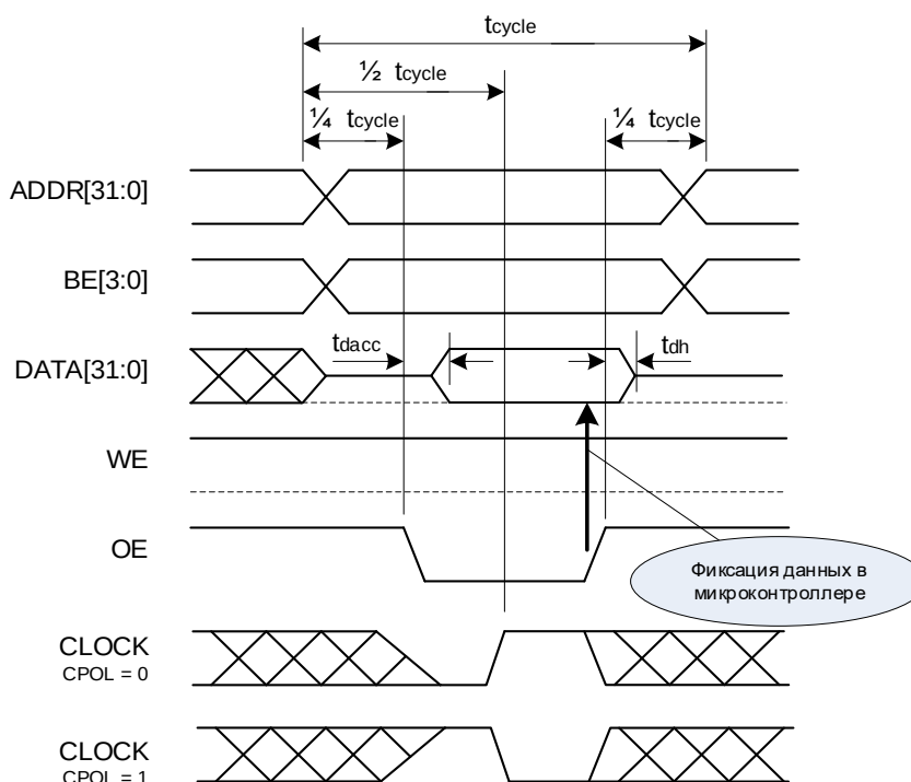
Рисунок 36 – Диаграмма чтения
