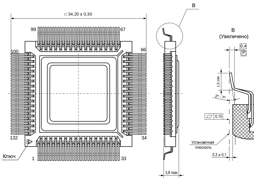
Рисунок 155 – Габаритный чертеж микросхемы в корпусе 4229.132-3 с формованными выводами
