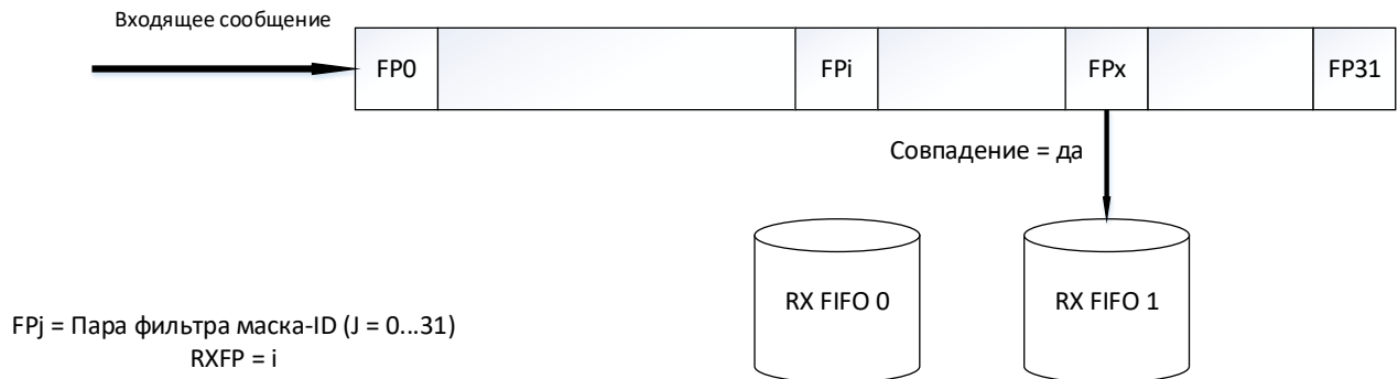
Рисунок 139 – нормальное функционирование RX FIFO 1
