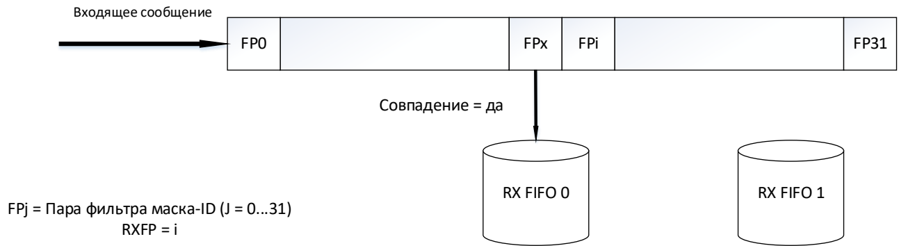
Рисунок 138 – нормальное функционирование RX FIFO 0
