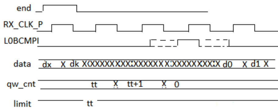
Рисунок 89. Временная диаграмма завершения приёма, инициированного по сигналу события (вход L0BCMPIO).
