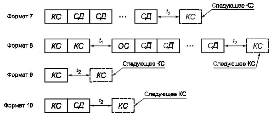
Рисунок 148 – Форматы групповых сообщений
