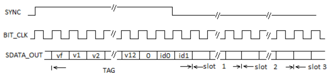
Рисунок 102 – Структура тэга
