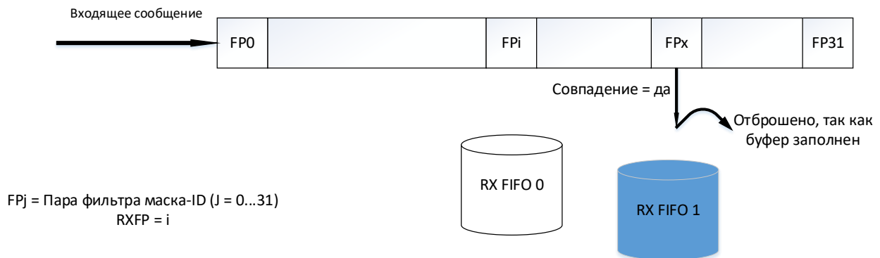
Рисунок 141 – отбрасывание сообщения (RX FIFO 1 заполнен, но совпадение)
