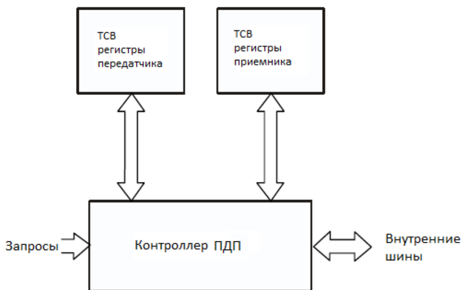
Рисунок 48 – Блок-схема DMA
