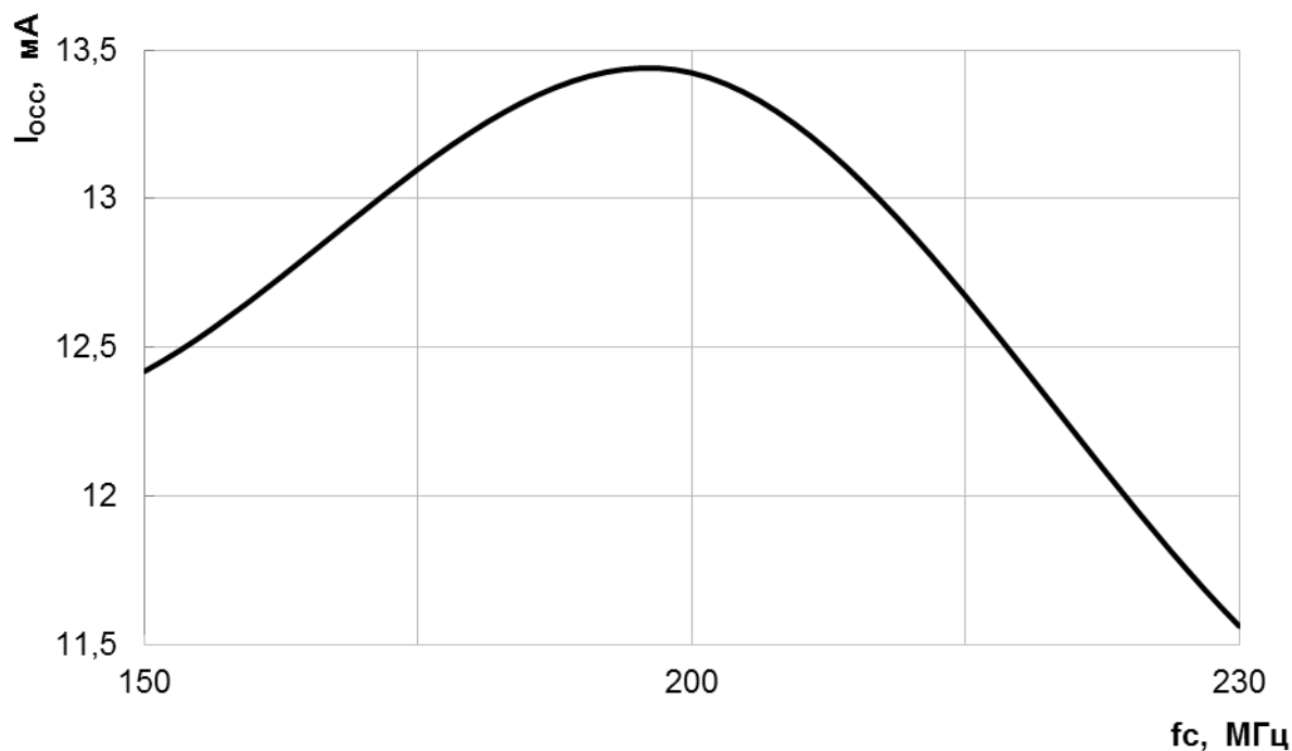
Рисунок 185 – Зависимость динамического тока потребления аналоговых блоков I_{OSS} от тактовой частоты процессора f_C при U_{CC} = 1,32 В, U_{CCIO} = U_{CCA} = 3,6 В, T = 25 °С
