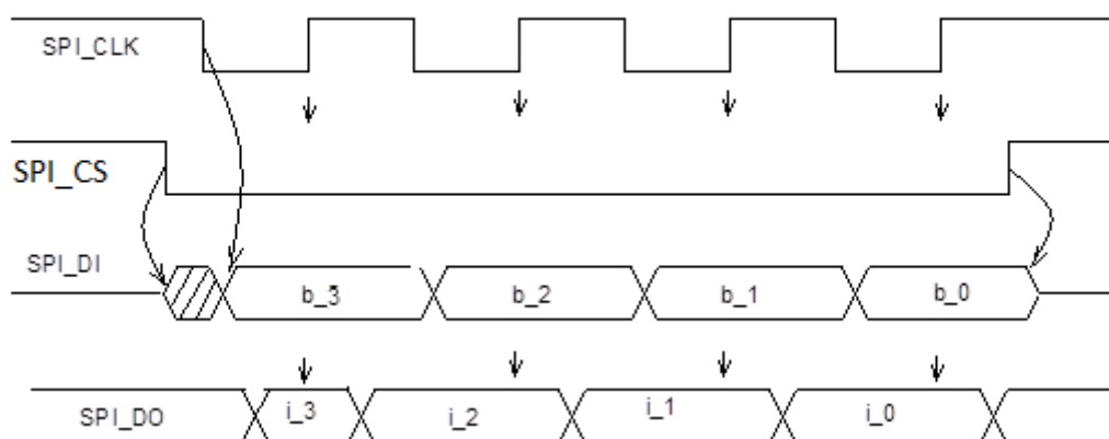
Рисунок 92 – Диаграмма обмена в режиме slave
