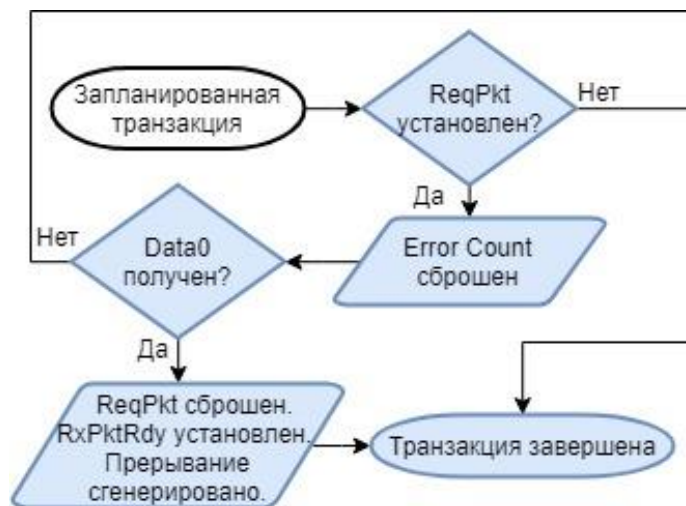
Рисунок 132 – Передача транзакций IN
