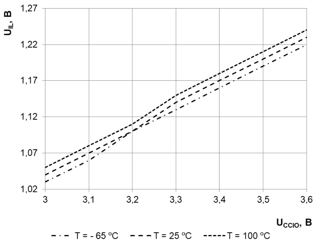
Рисунок 187 – Зависимость входного напряжения низкого уровня U_{IL} от напряжения питания схем ввода/вывода U_{ССЮ} при U_{СС} = 1,08 \text{ В}
