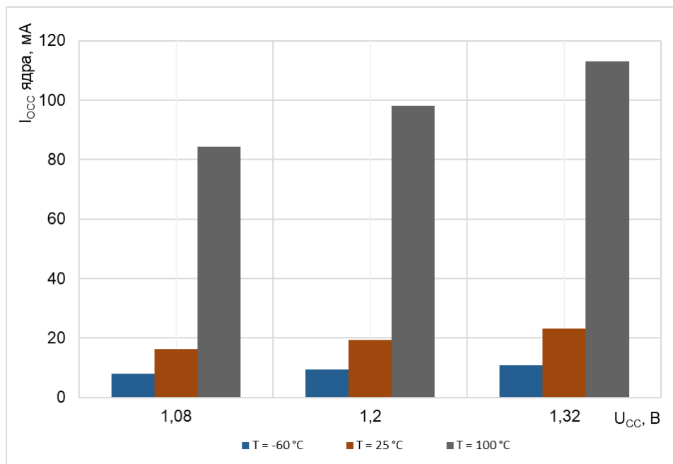
Рисунок 188 – Зависимость тока потребления I_{СС} ядра от температуры и напряжения U_{СС} в режиме SLEEP
