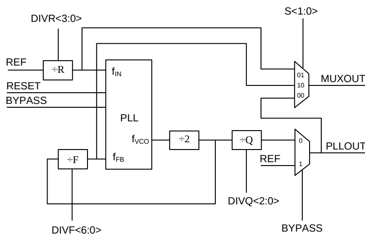
Рисунок 170 – Структура PLL
