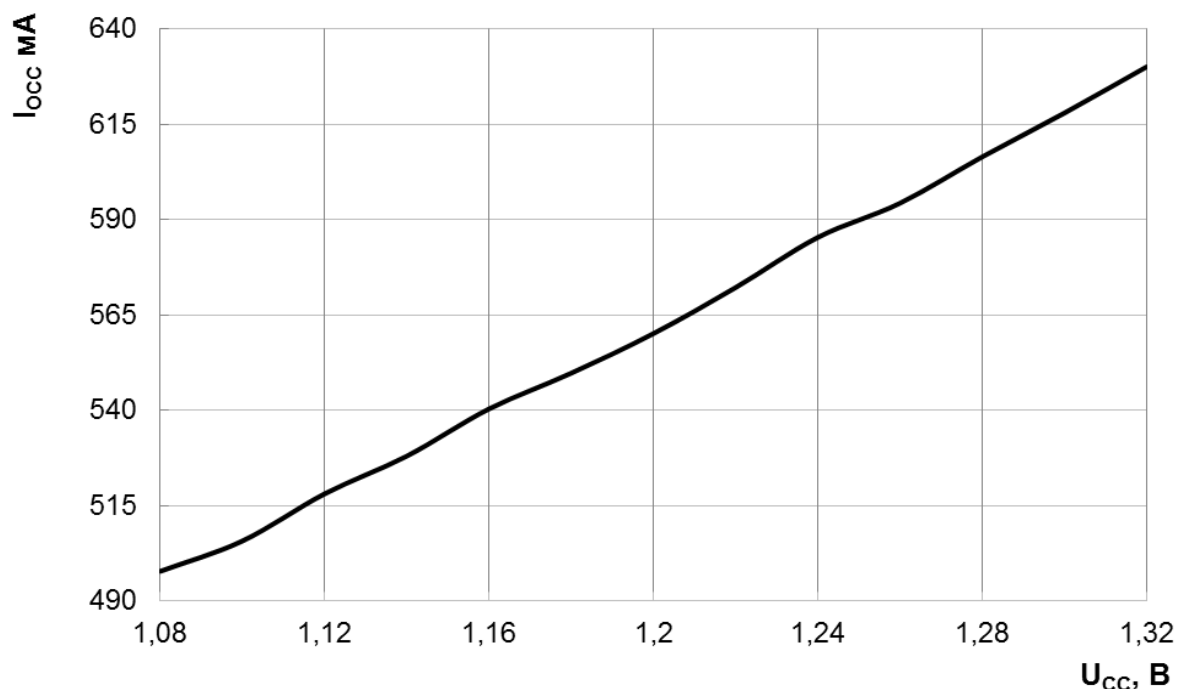
Рисунок 183 – Зависимость динамического тока потребления I_{oss} ядра от напряжения питания при f_c = 230 МГц, T = 25 °C
