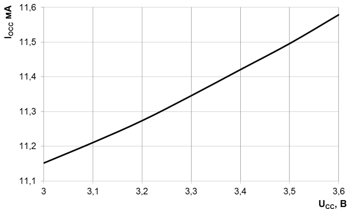
Рисунок 182 – Зависимость динамического тока потребления I OCC аналоговых блоков от напряжения питания при f C = 230 МГц, T = 25 °C
