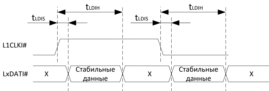
Рисунок 86 – Временная диаграмма входных данных порта связи при тактировании от L1CLKI#
