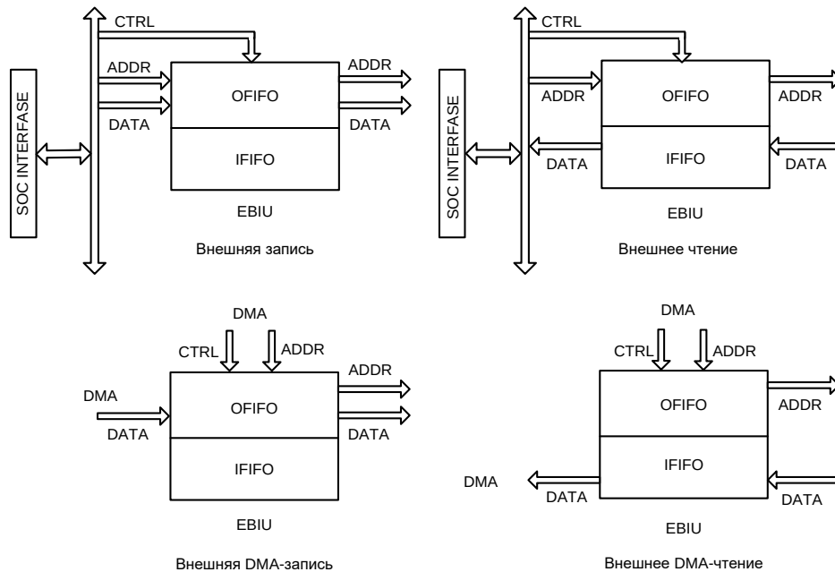
Рисунок 53 – Передача данных через интерфейс внешней шины (EBIU)
