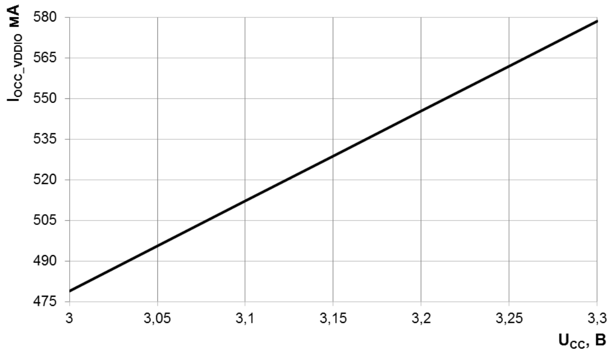
Рисунок 181 – Зависимость динамического тока потребления I OCC схем ввода/вывода от напряжения питания при f C = 230 МГц, T = 25 °C
