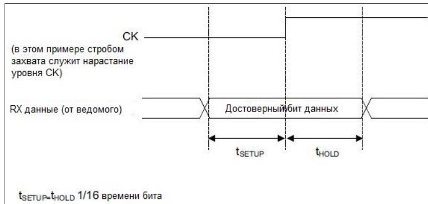
Рисунок 125 – Время установки/удержания RX
