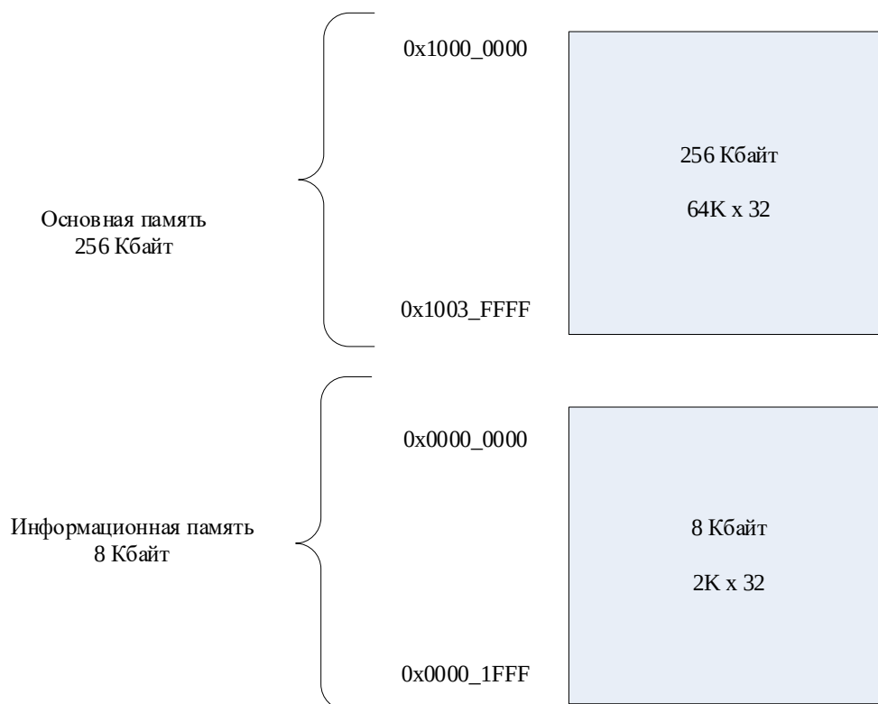
Рисунок 11 – Структура FLASH-памяти
