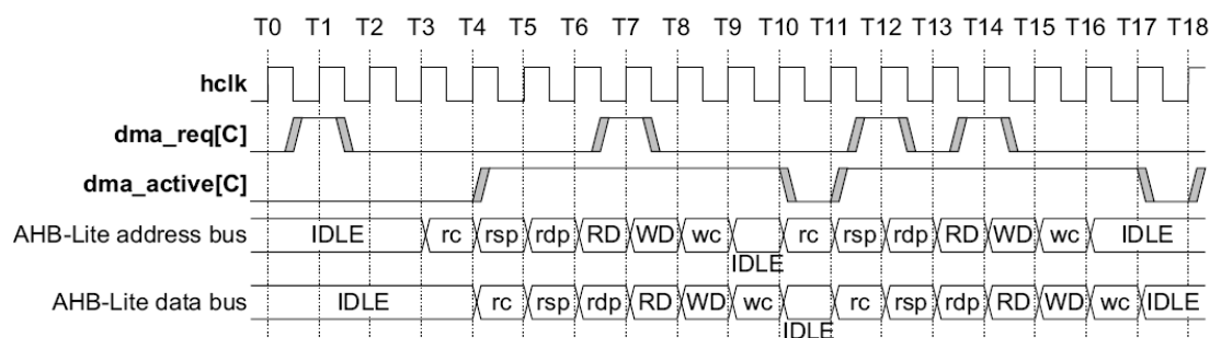
Рисунок 86 – Диаграмма работы при получении импульсного запроса от периферийного блока
