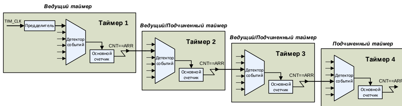
Рисунок 41 – Пример каскадного соединения таймеров
