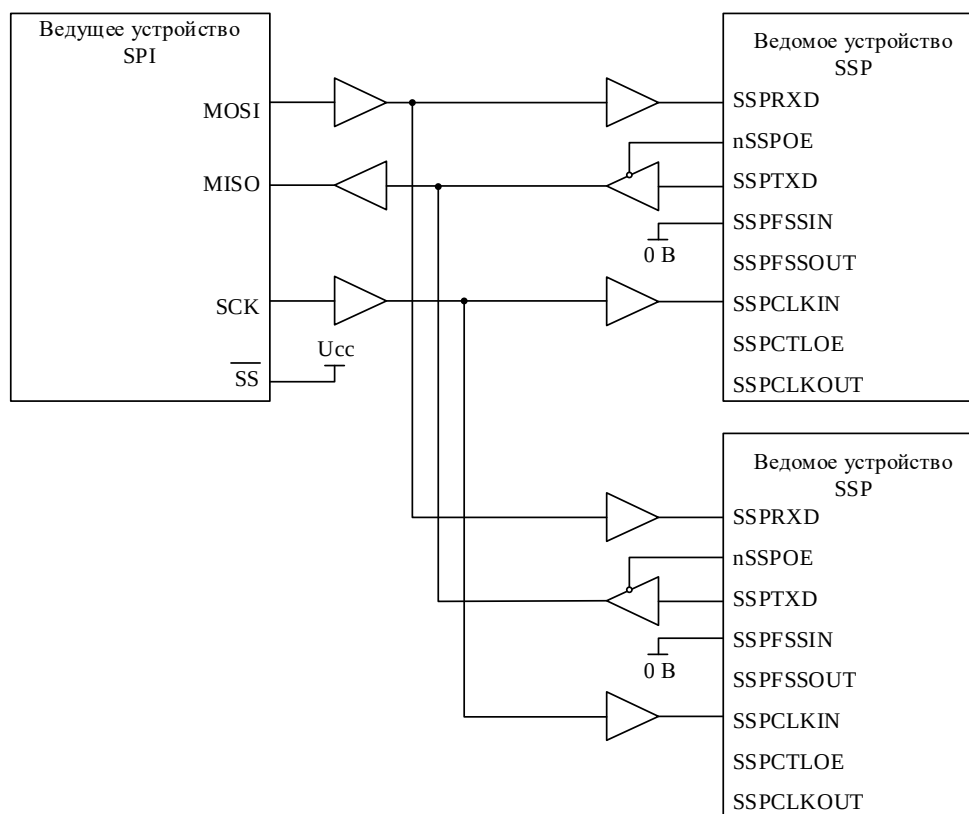
Рисунок 76 – Ведущее устройство, протокол SPI, подключено к двум ведомым модулям SSP
