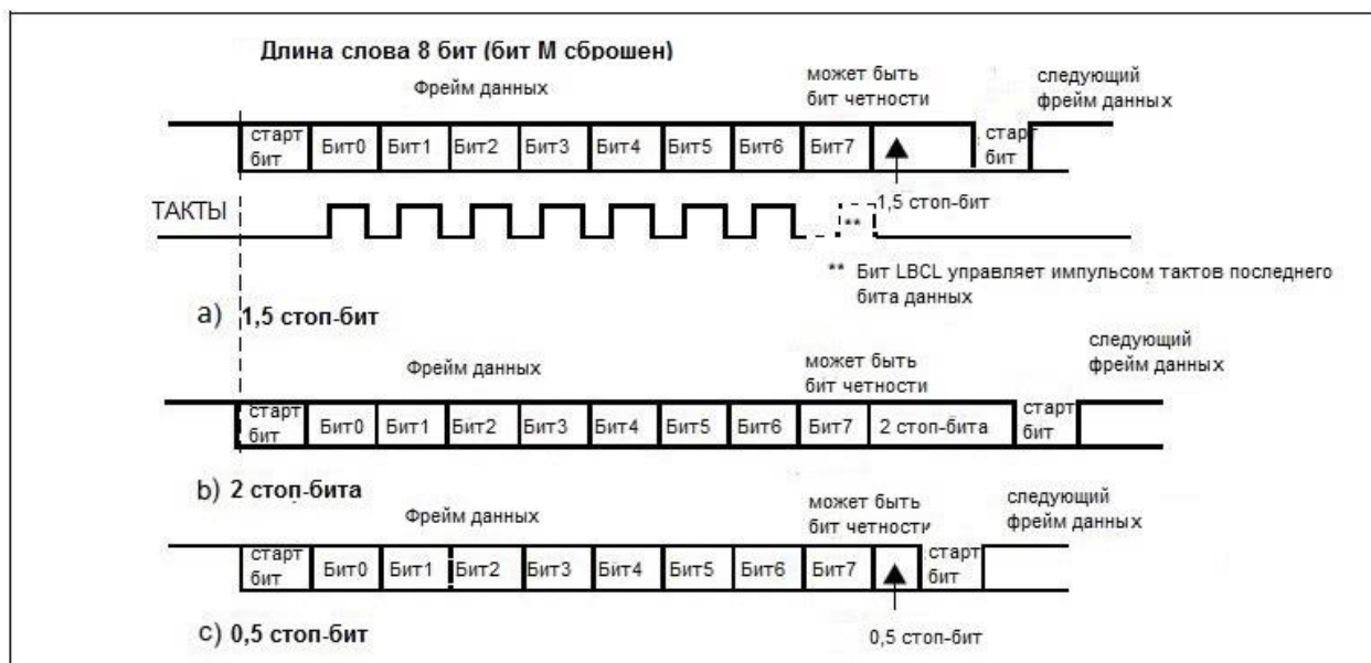
Рисунок 115 – Конфигурируемые стоп-биты
