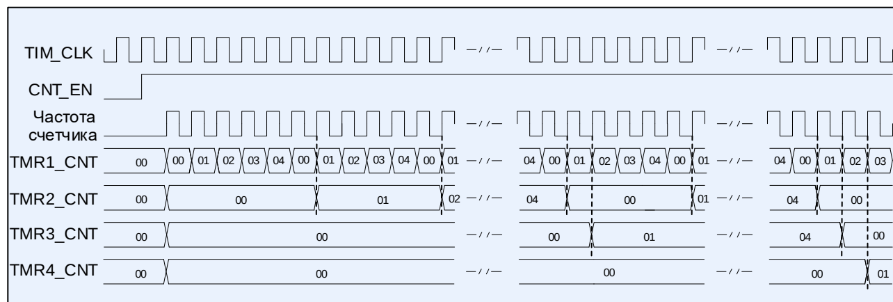
Рисунок 42 – Диаграммы работы четырех таймеров в каскаде
