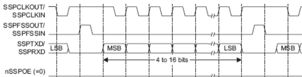
Рисунок 69 – Формат синхронного обмена протокола SPI, SPO=1, SPH=0 (непрерывный обмен)
