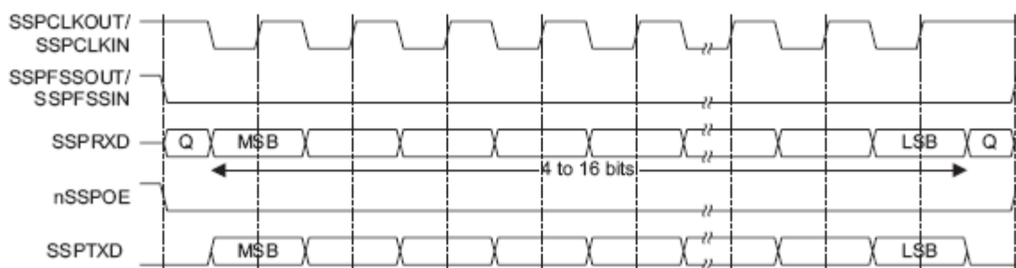
Рисунок 70 – Формат синхронного обмена протокола SPI, SPO=1, SPH=1
