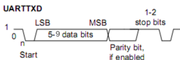
Рисунок 81 – Кадр передачи данных
