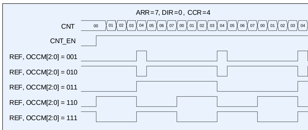
Рисунок 50 – Диаграмма работы в режиме ШИМ, CCR1_EN=0
