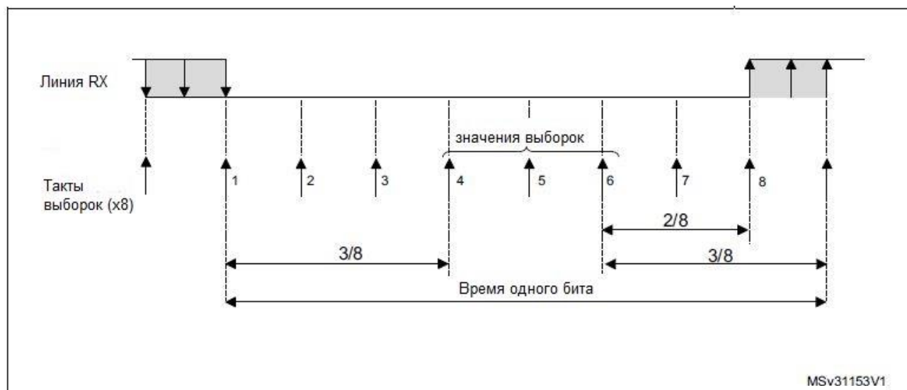
Рисунок 119 – Выборка данных при передискретизации на 8
