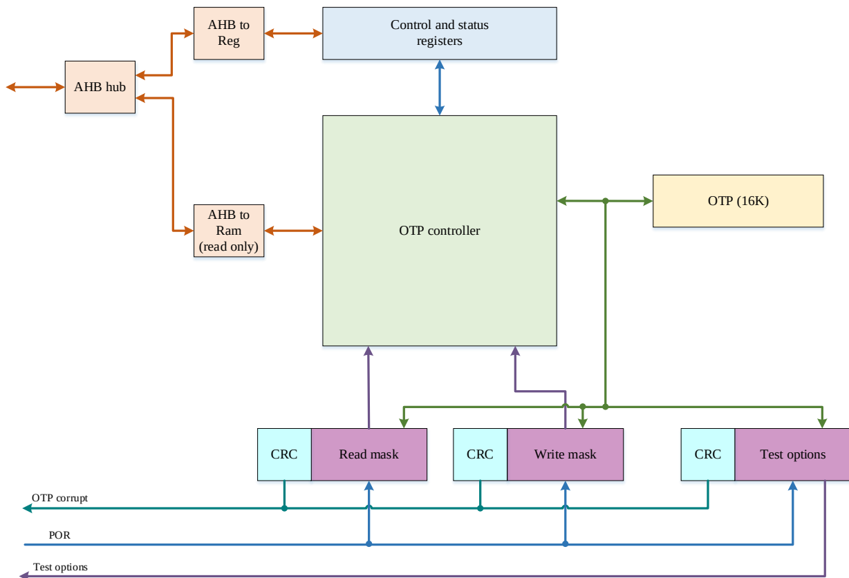
Рисунок 132 – Структурная схема модуля ОТР
