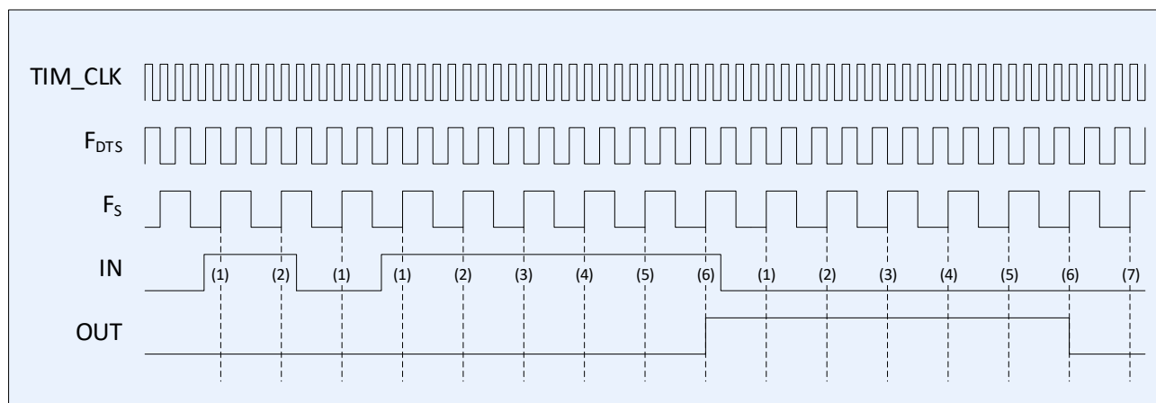
Рисунок 56 – Диаграмма работы фильтра, F_S = F_{DTS}/2 , N = 6
