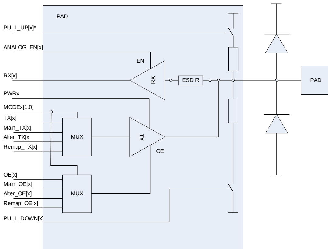
Рисунок 30 – Блок схема разряда порта ввода-вывода
