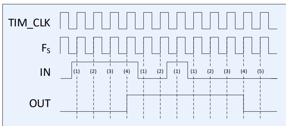
Рисунок 55 – Диаграмма работы фильтра, F_S = \text{TIM\_CLK} , N = 4
