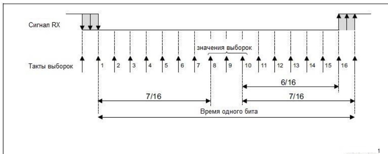
Рисунок 118 – Выборка данных при передискретизации на 16
