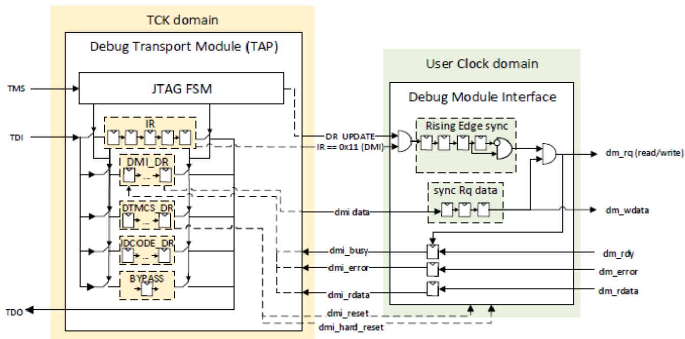
Рисунок 101 – Интерфейс DM
