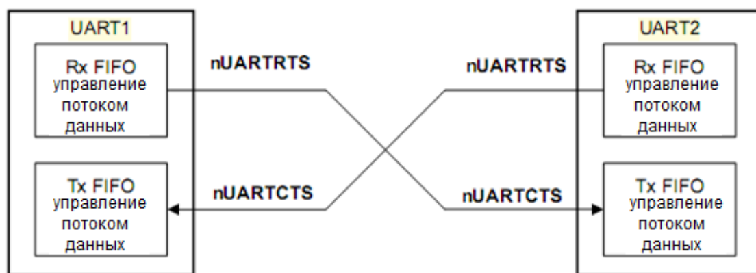
Рисунок 83 – Взаимодействие двух устройств последовательной связи с аппаратным управлением потоком данных
