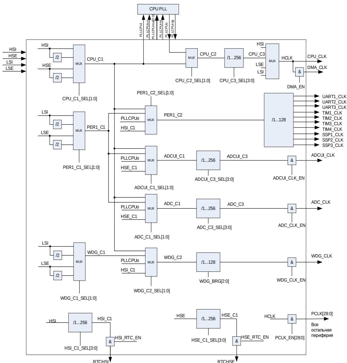
Рисунок 28 – Структурная блок-схема формирования тактовой частоты
