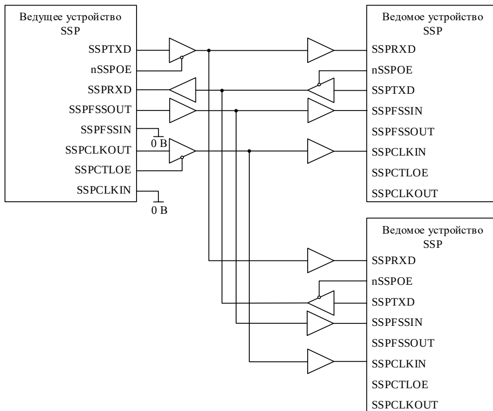
Рисунок 74 – Ведущее устройство SSP подключено к двум ведомым
