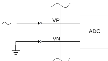
Рисунок 20 – Недифференциальное включение
