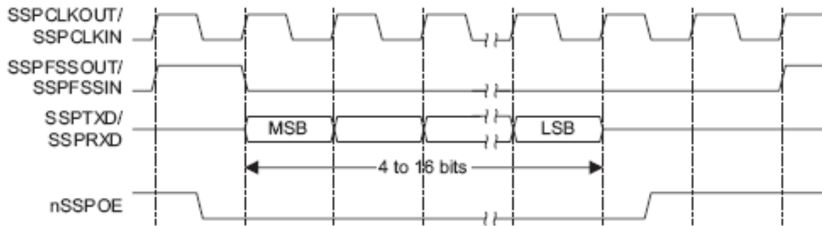
Рисунок 63 – Формат синхронного обмена протокола SSI (единичный обмен)
