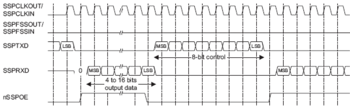
Рисунок 72 – Формат синхронного обмена протокола Microwire (непрерывный обмен)
