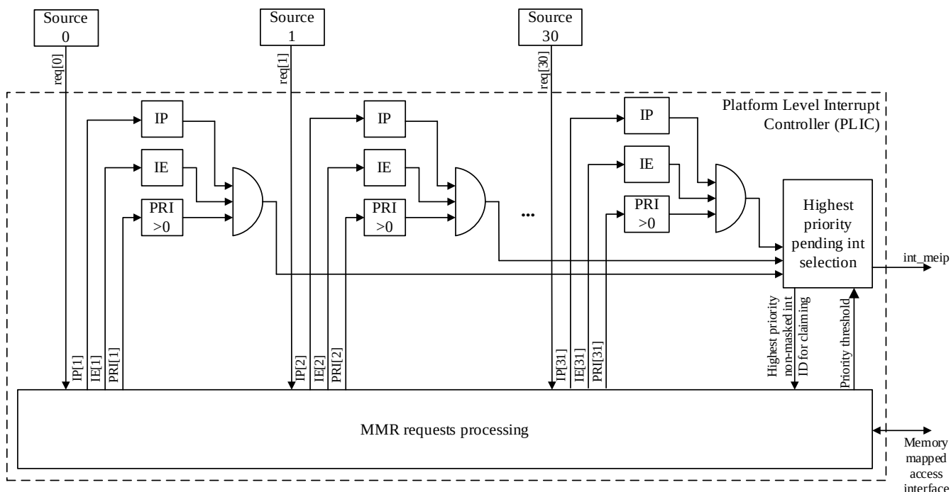
Рисунок 98 – Структурная схема PLIC
