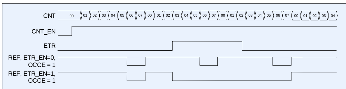
Рисунок 52 – Диаграмма сброса сигнала REF по выводу ETR
