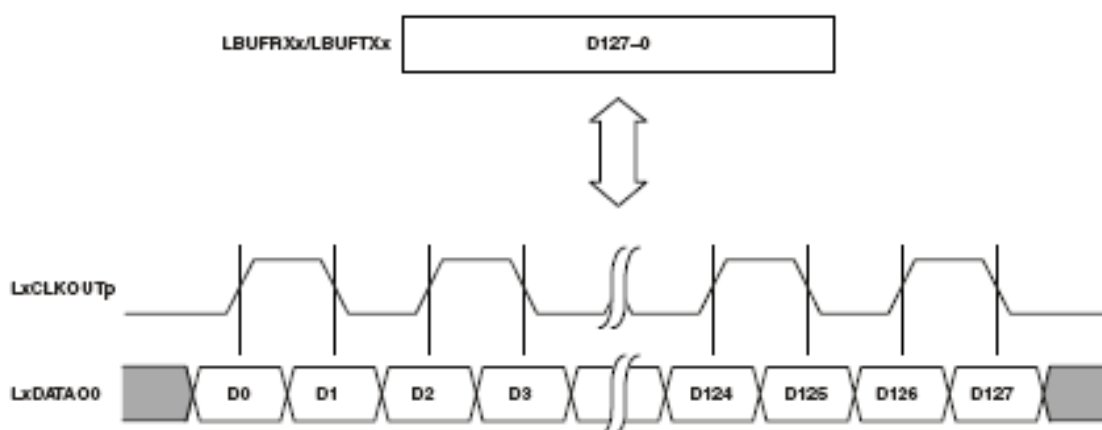
Рисунок 54 – Шина данных 1 разряда
