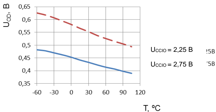
Рисунок 85 – Зависимость дифференциального выходного напряжения LINK-портов U_{OD} от температуры при R_L=100 Ом
