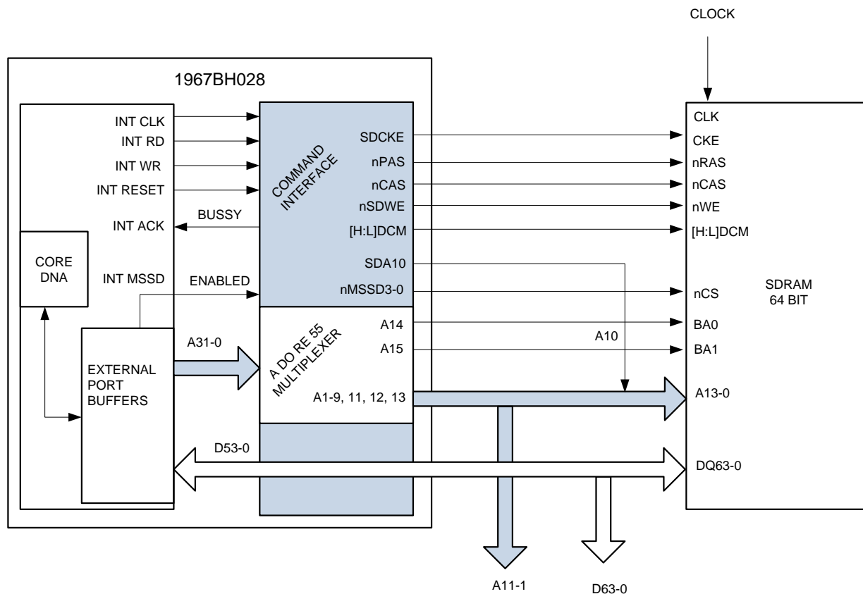
Рисунок 35 – Интерфейс контроллера SDRAM (для конфигурации с 64-разрядной шиной)
