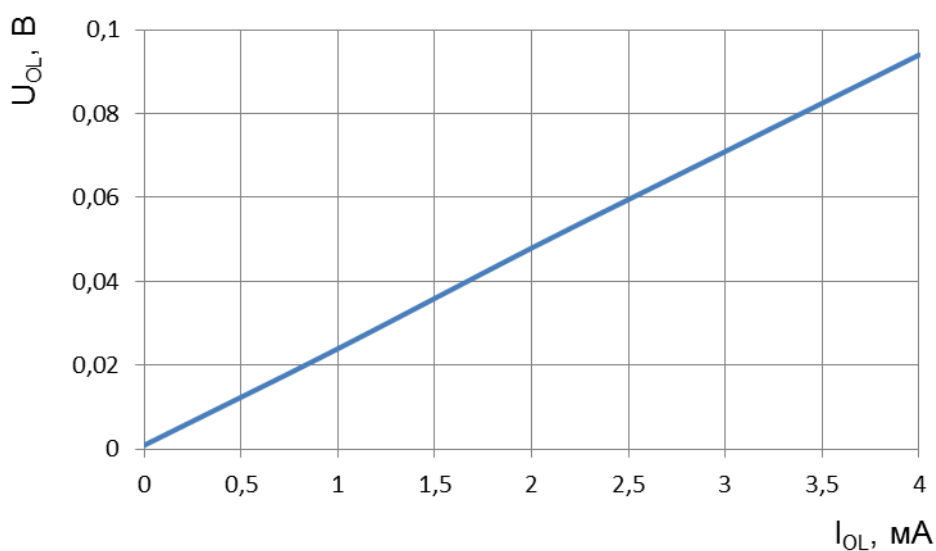
Рисунок 84 – Зависимость выходного напряжения низкого уровня U_{OL} от тока нагрузки при U_{CC} = 0,9 \text{ В} , U_{CCA} = U_{CCIO} = 2,25 \text{ В} , T = 25 \text{ °С}
