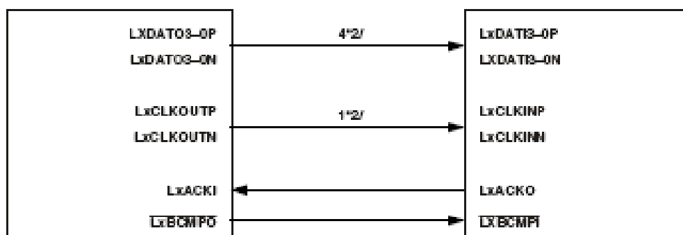
Рисунок 50 – Конфигурация порта связи (4-разрядный режим)
