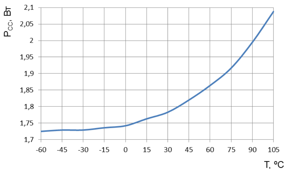
Рисунок 87 – Зависимость потребляемой мощности P_{CC} от температуры при U_{CC} = 1,1 В, U_{CCA} = U_{CCIO} = 2,75 В, f_C = 450 МГц, f_{C\_PLL} = 100 МГц
