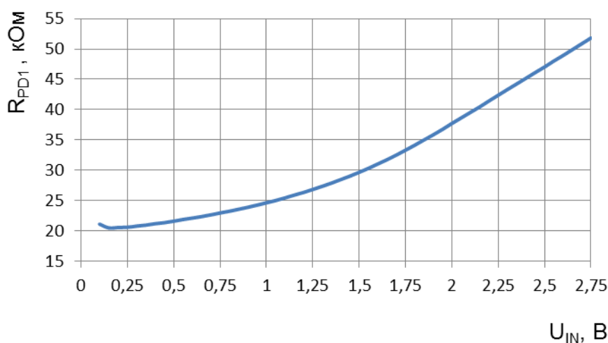
Рисунок 92 – Зависимость сопротивления подтягивающего к земле резистора R_{PD1} от входного напряжения U_{IN} при U_{CC} = 1,1 В, U_{CCA} = U_{CCIO} = U_{IN} = 2,75 В, T = 25 °С
