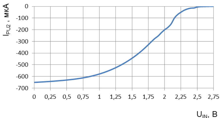
Рисунок 93 – Зависимость тока I_{PU2} от входного напряжения U_{IN} при температуре 25 °С
