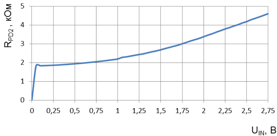
Рисунок 95 – Зависимость сопротивления подтягивающего к земле резистора R PD2 от входного напряжения U IN при U CC = 1,1 В, U CCA = U CCIO = U IN = 2,75 В, T = 25 °C
