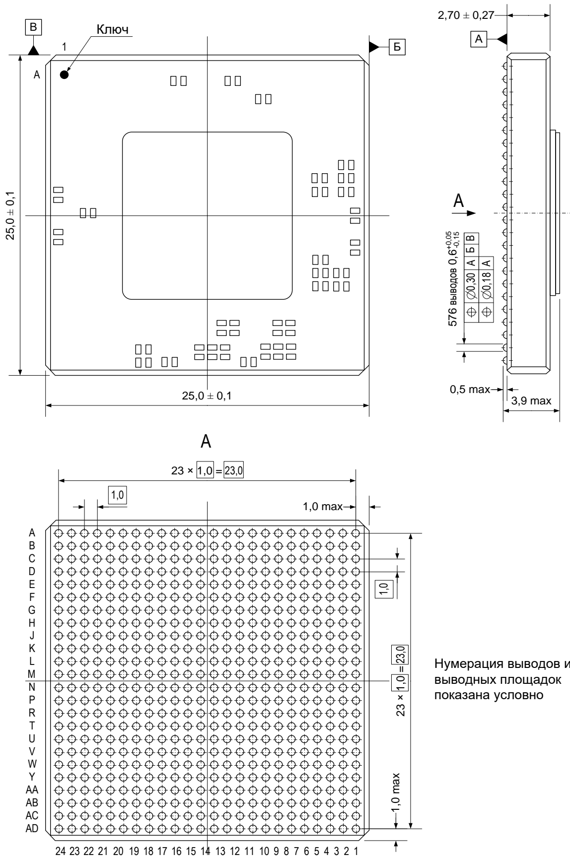
Рисунок 96 – Микросхема в корпусе МК8303.576-1
