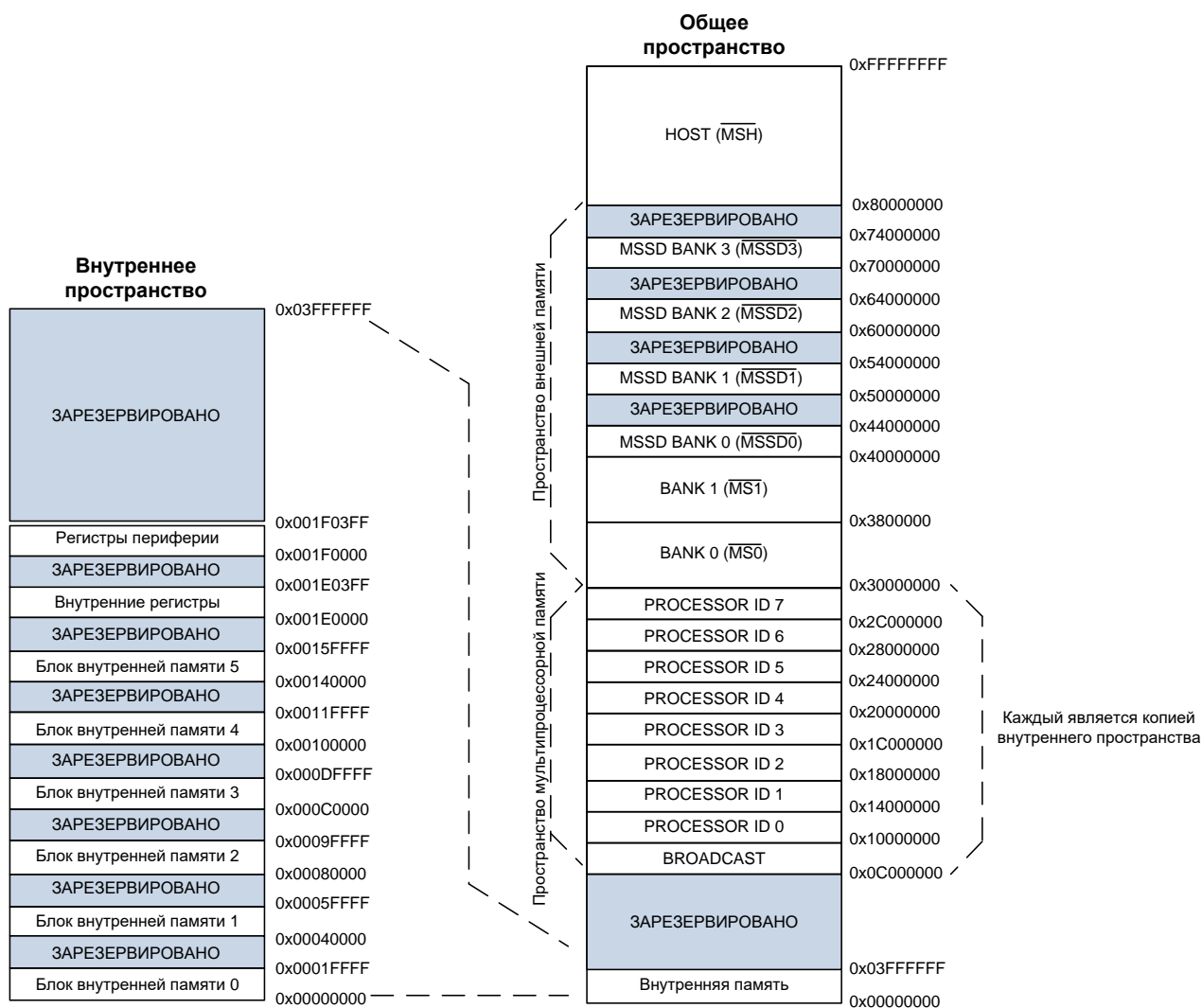
Рисунок 12 – Карта памяти 1967BH028
