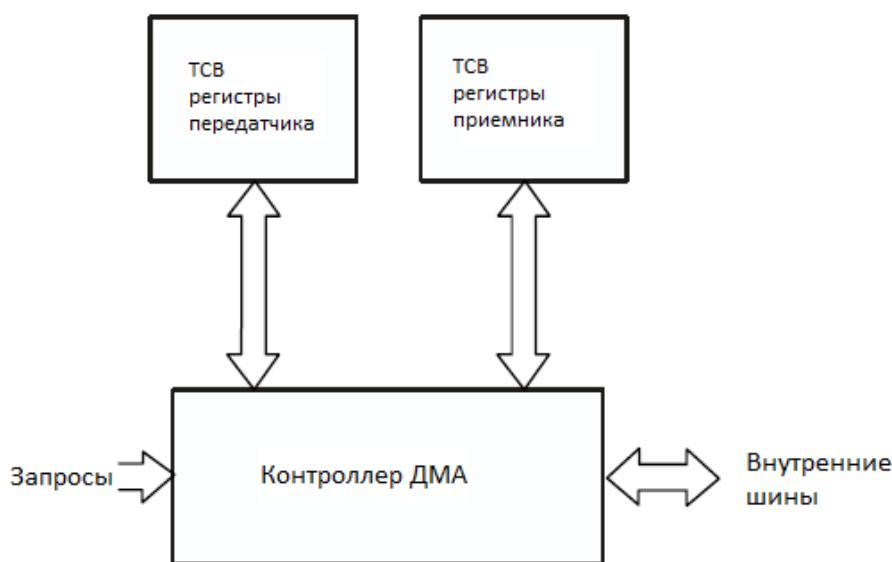
Рисунок 45 – Блок-схема DMA
