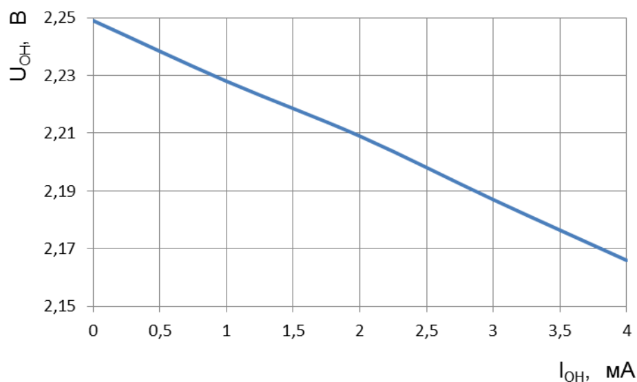
Рисунок 83 – Зависимость выходного напряжения высокого уровня U_{OH} от тока нагрузки при U_{CC} = 0,9 \text{ В} , U_{CCA} = U_{CCIO} = 2,25 \text{ В} , T = 25 \text{ °С}
