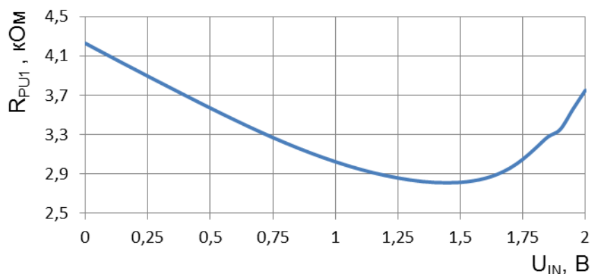
Рисунок 91 – Зависимость сопротивления подтягивающего к питанию резистора R_{PU1} от входного напряжения U_{IN} при U_{CC} = 1,1 В, U_{CCA} = U_{CCIO} = 2,75 В, U_{IL} = 0 В, T = 25 °С
