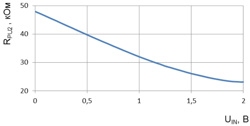
Рисунок 94 – Зависимость сопротивления подтягивающего к питанию резистора R PU2 от входного напряжения U IN при U CC = 1,1 В, U CCA = U CCIO = 2,75 В, U IL = 0 В, T = 25 °C
