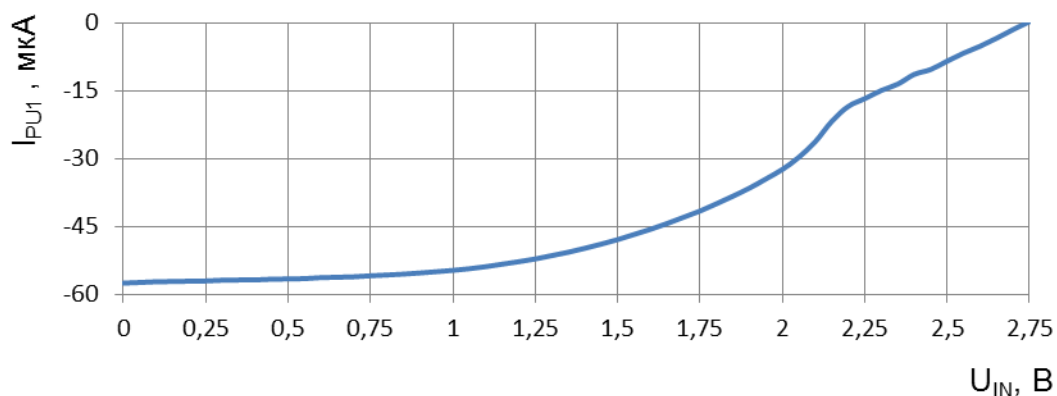
Рисунок 90 – Зависимость тока I_{PU1} от входного напряжения U_{IN} при T = 25 °С
