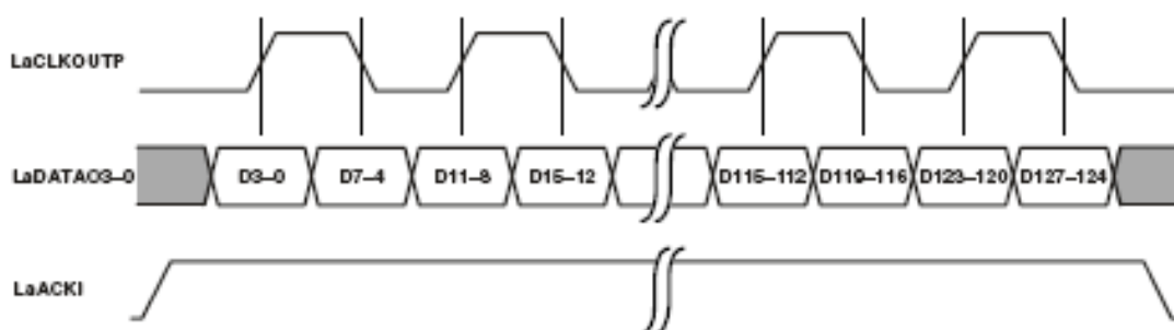
Рисунок 55 – Порт связи “а” передает одно счетверенное слово порту связи “b”
