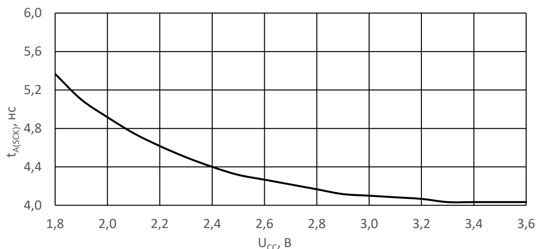
Рисунок 55 – Зависимость времени выборки данных по спаду сигнала SCK t_{A(SCK)} от напряжения питания U_{CC} при T = 25 °С
