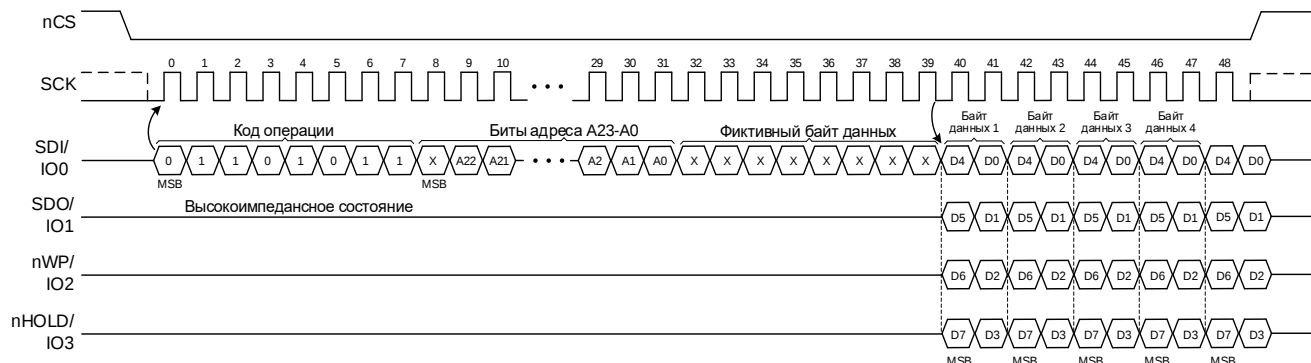
Рисунок 8 – Операция чтения с кодом 6Bh
