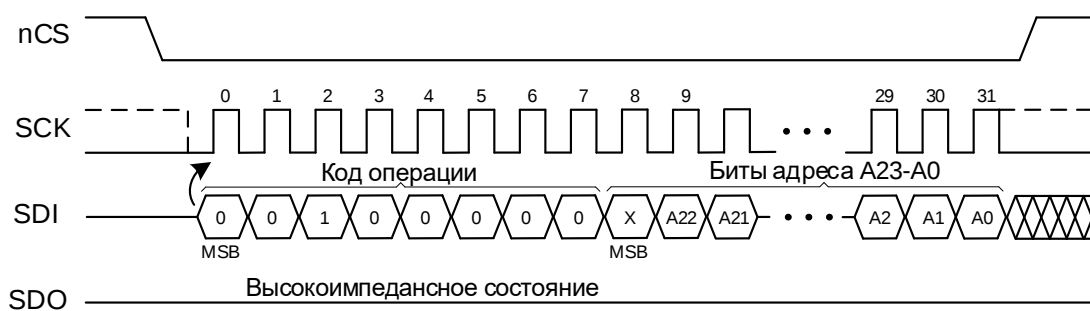
Рисунок 12 – Операция стирания сектора с кодом 20h
