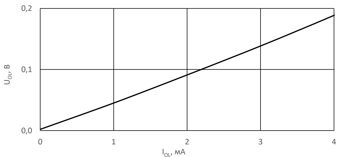
Рисунок 44 – Зависимость выходного напряжения низкого уровня U_{OL} от тока нагрузки I_{OL} при U_{CC} = 1,8 \text{ В} , T = 25^\circ\text{C}
