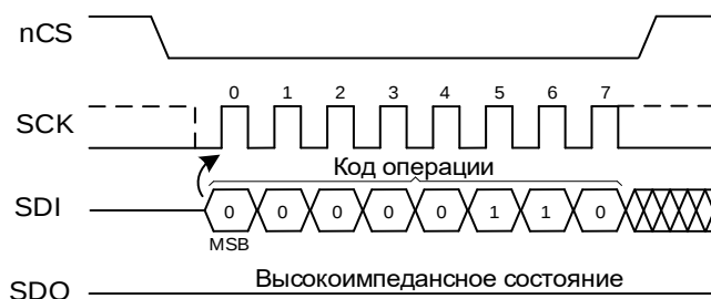
Рисунок 17 – Операция разрешения записи
