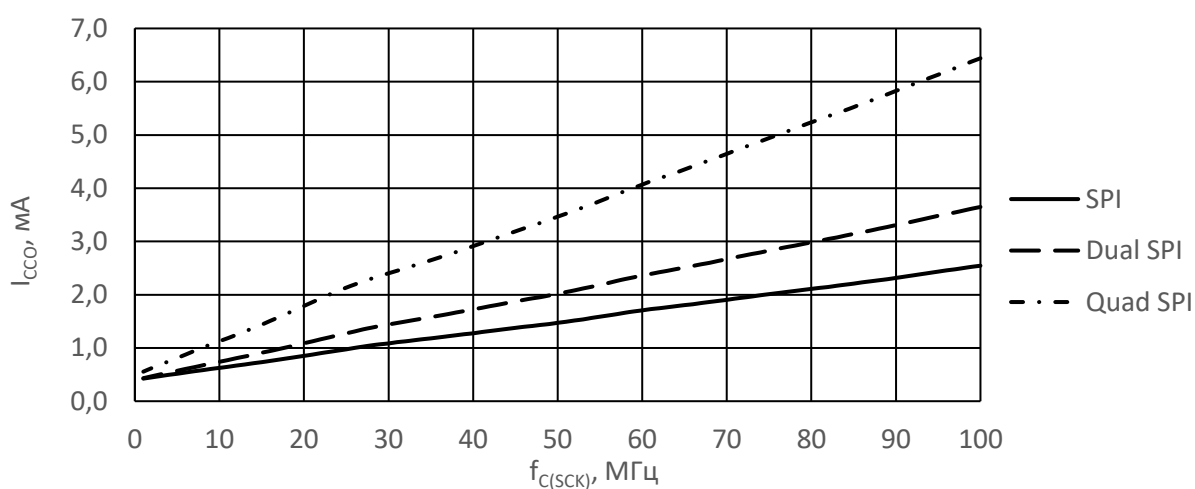
Рисунок 50 – Зависимость динамического тока потребления I_{CCO} при чтении в режимах SPI, Dual SPI и Quad SPI от частоты тактового сигнала SPI интерфейса f_{C(SCK)} при U_{CC} = 3,6 В, T = 25 °C
