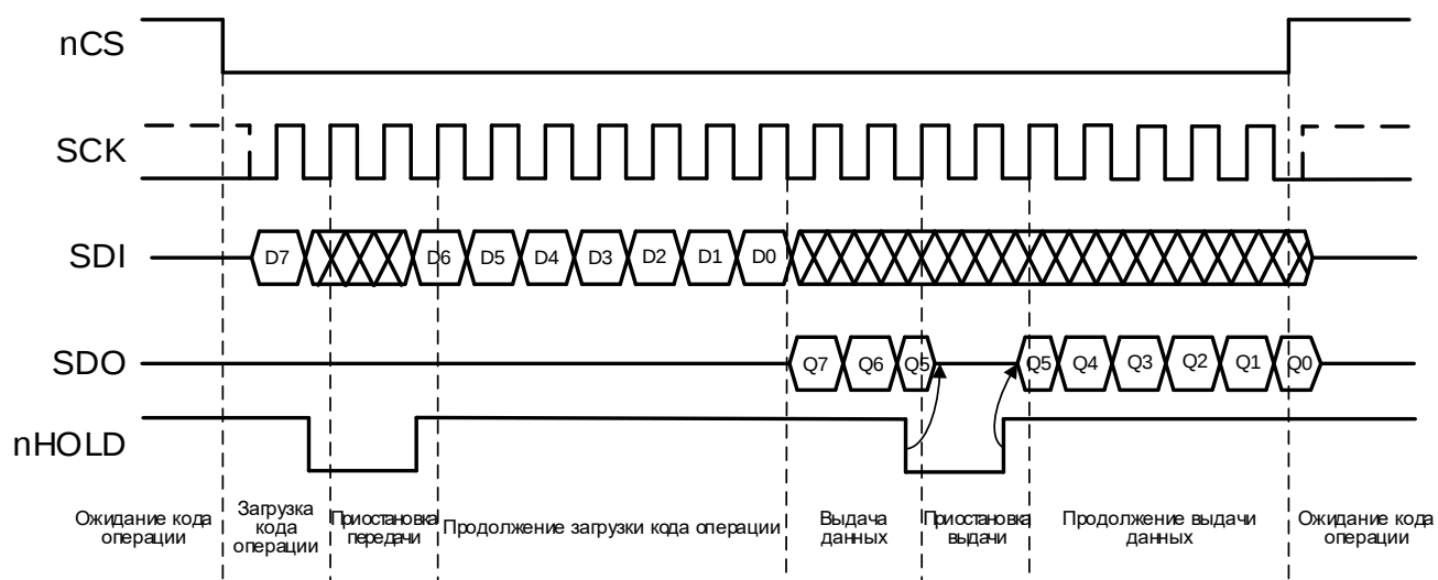
Рисунок 4 – Приостановка передачи по шине SPI
