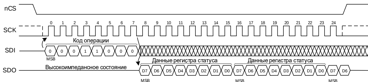
Рисунок 24 – Операция чтения регистра статуса помехоустойчивого кодирования
