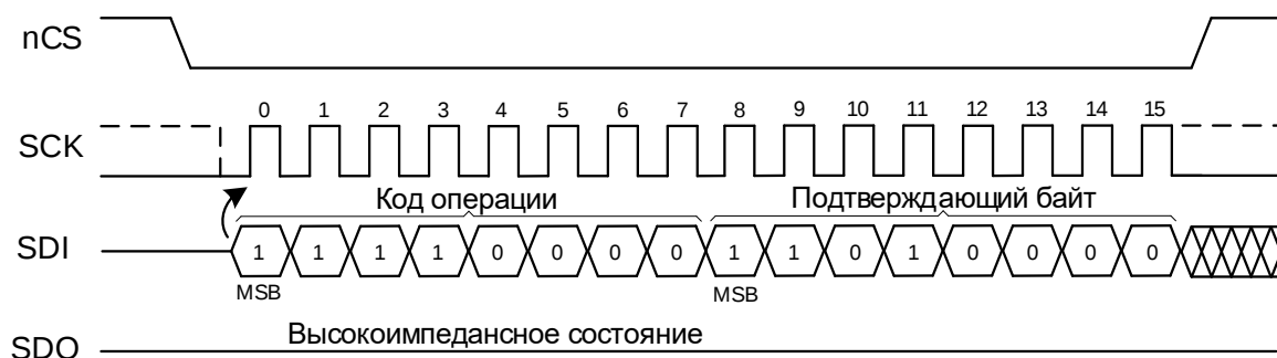
Рисунок 25 – Операция сброса
