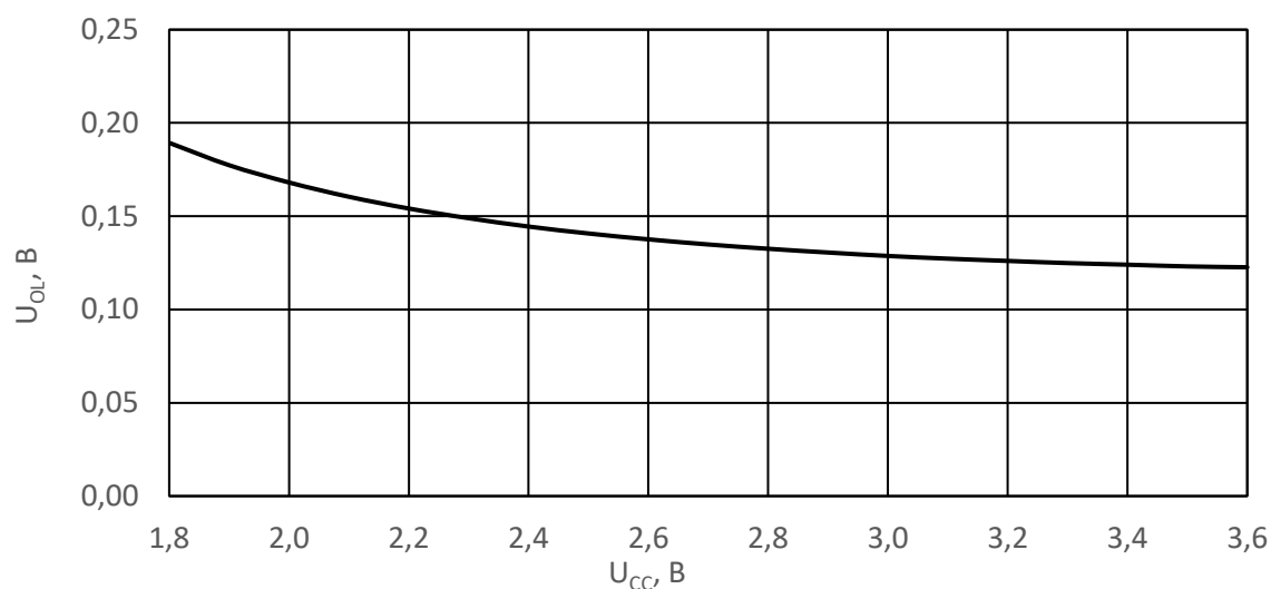
Рисунок 42 – Зависимость выходного напряжения низкого уровня U_{OL} от напряжения питания U_{CC} при T = 25^\circ\text{C} и I_{OL} = 4 \text{ мА}
