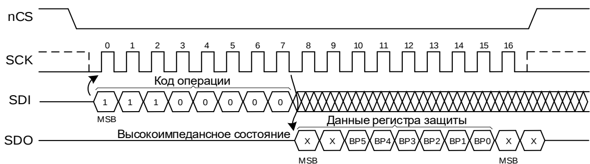
Рисунок 21 – Операция чтения регистра защиты секторов
