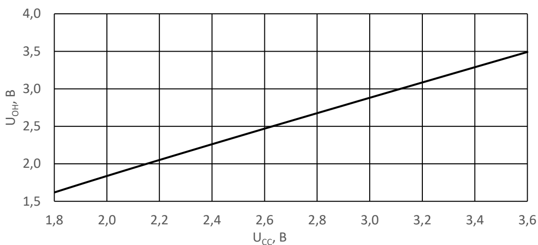
Рисунок 39 – Зависимость выходного напряжения высокого уровня U_{OH} от напряжения питания U_{CC} при T = 25\text{ }^{\circ}\text{C} и I_{OH} = -4\text{ мА}
