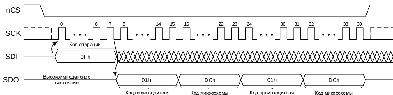
Рисунок 26 – Операция чтения идентификационной информации микросхемы
