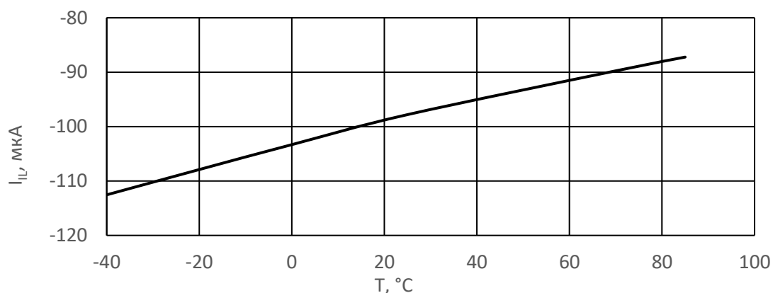
Рисунок 46 – Зависимость входного тока низкого уровня I_{IL} , от температуры T при U_{CC} = 3,6 В, U_{IL} = 0 В, U_{IH} = U_{CC}
