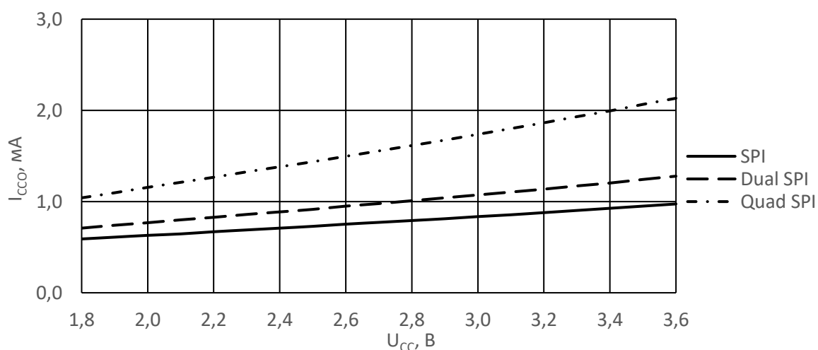
Рисунок 49 – Зависимость динамического тока потребления I_{CCO} при чтении в режимах SPI, Dual SPI и Quad SPI от напряжения питания U_{CC} при T = 25 °C, f_{C(SCK)} = 25 МГц
