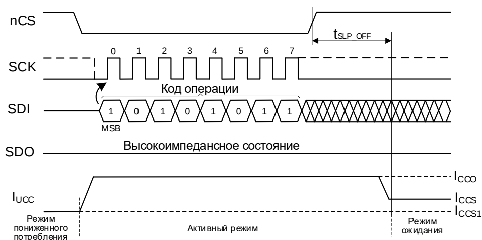
Рисунок 29 – Операция выхода из режима пониженного потребления
