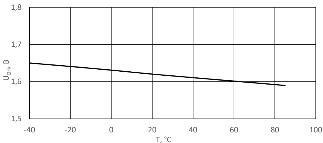
Рисунок 40 – Зависимость выходного напряжения высокого уровня U_{OH} от температуры T при U_{CC} = 1,8\text{ В} и I_{OH} = -4\text{ мА}
