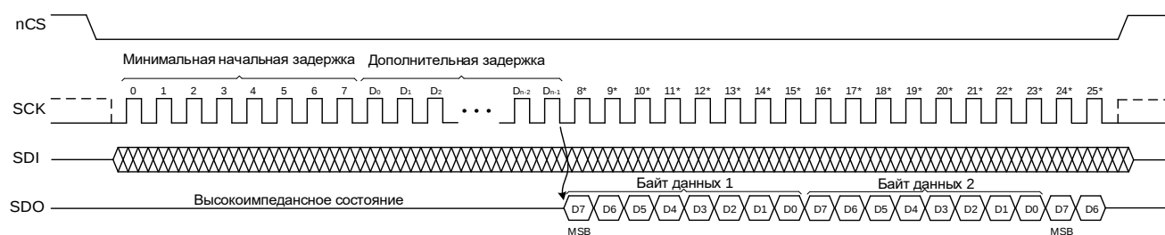
Рисунок 30 – Чтение в режиме автоматической загрузки, бит QE=0
