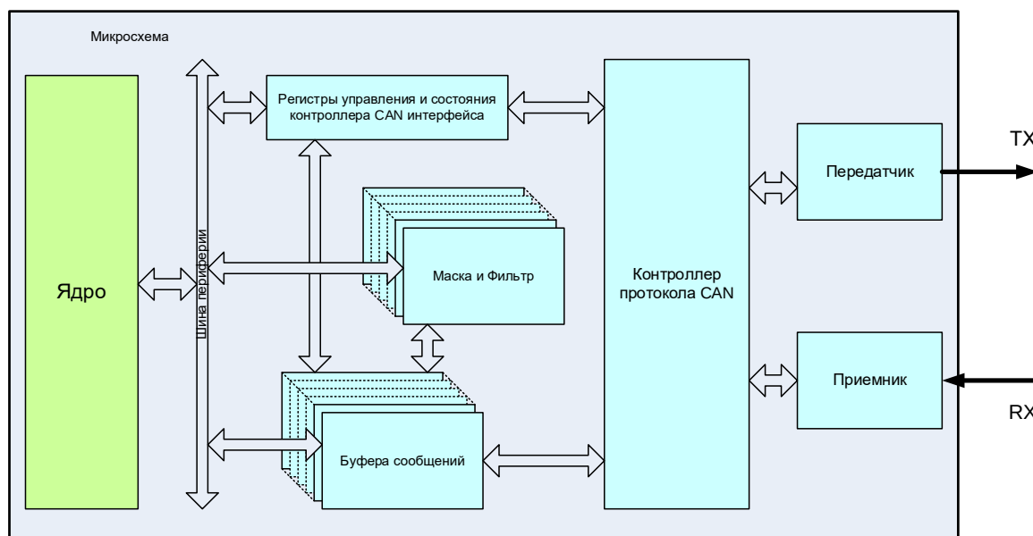
Рисунок 47 – Структурная блок-схема контроллера CAN
