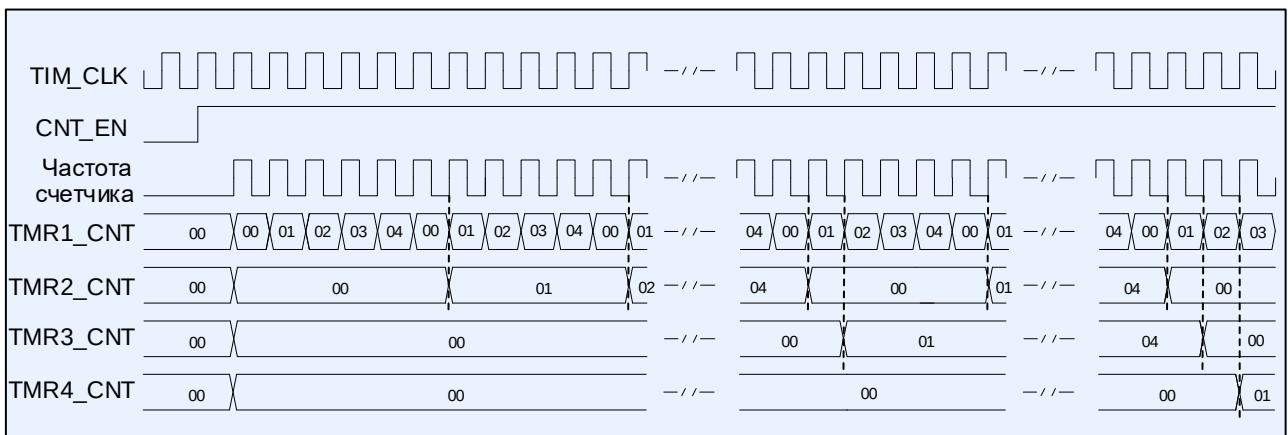
Рисунок 74 – Диаграммы работы четырех таймеров в каскаде
