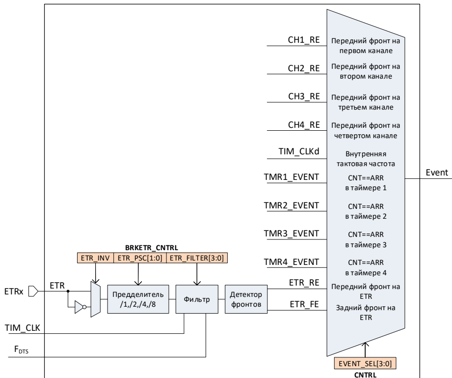
Рисунок 77 – Схема тактирования сигналом со входа ETR
