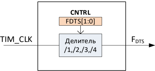
Рисунок 68 – Схема формирования тактовой частоты F DTS
