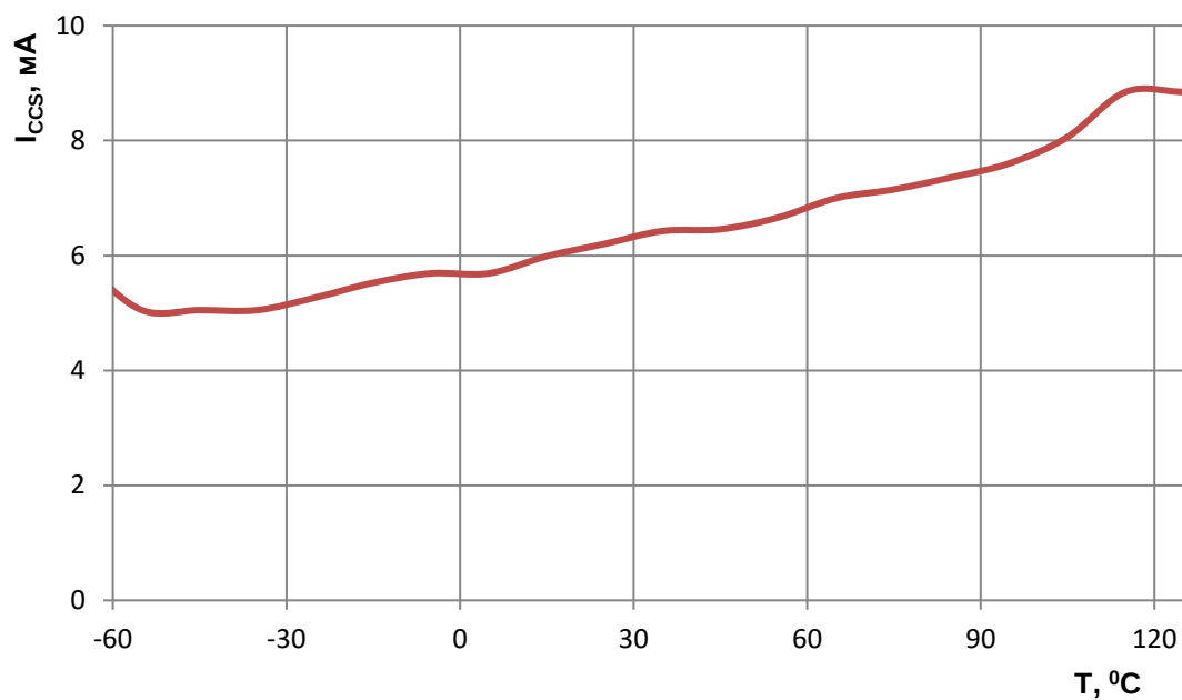
Рисунок 146 – Зависимость статического тока потребления в режиме покоя (регулятор напряжения выключен) от температуры при напряжении U_{cc}=3.6V
