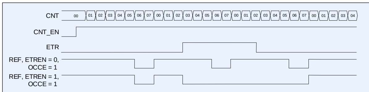
Рисунок 84 – Диаграмма сброса сигнала REF по выводу ETR
