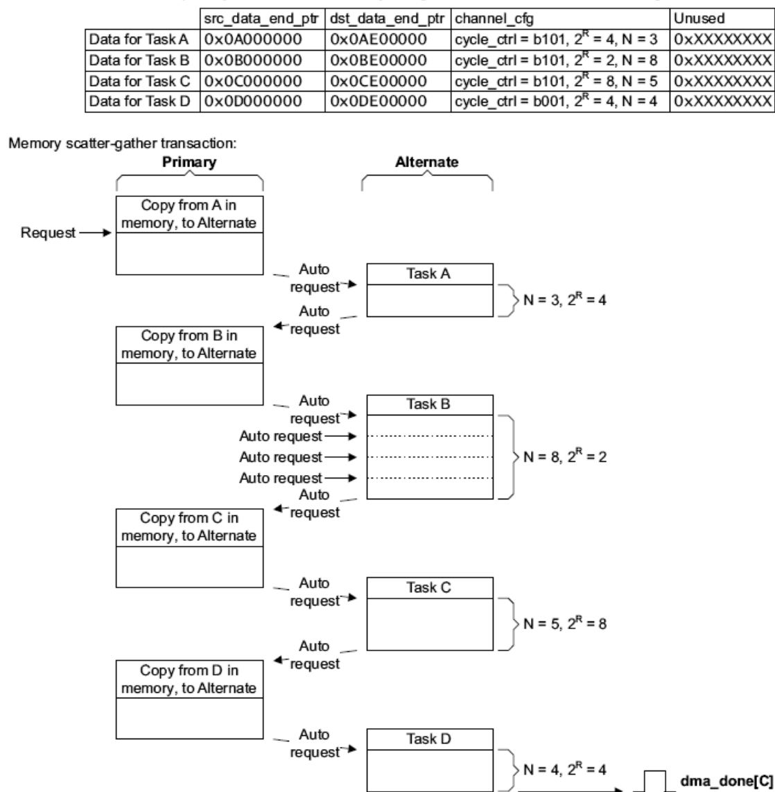
Рисунок 129 – Пример работы DMA в режиме с «Исполнением с изменением конфигурации»
