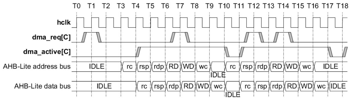
Рисунок 122 – Диаграмма работы при получении импульсного запроса от периферийного блока
