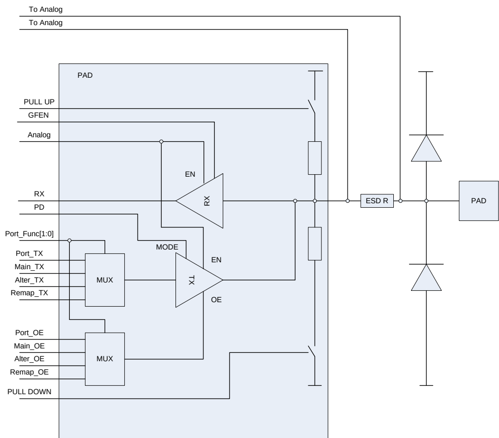
Рисунок 26 – Порты ввода/вывода
