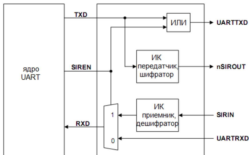
Рисунок 115 – Структурная схема кодака IrDA
