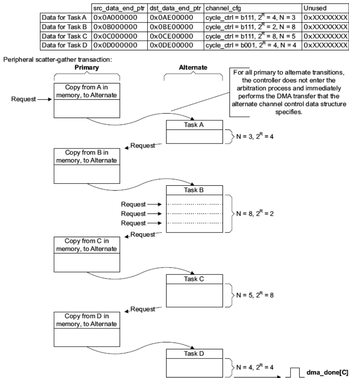
Рисунок 130 – Пример работы DMA в режиме с «Исполнением с изменением конфигурации»
