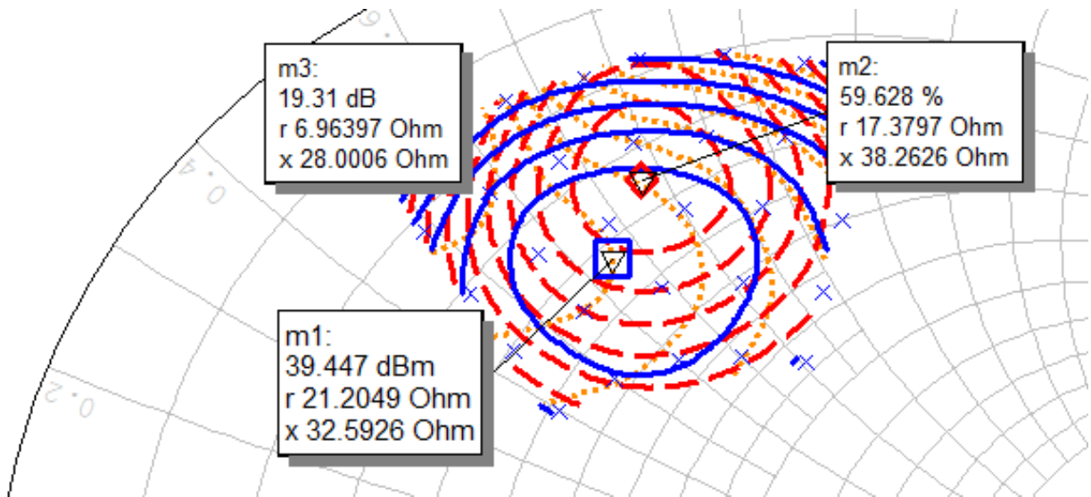
а) f_{ТЕСТ} = 2,6 ГГц
