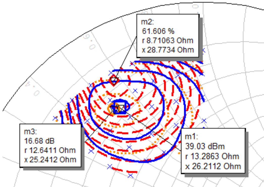
г) f_{\text{ТЕСТ}} = 3,2 \text{ ГГц}
