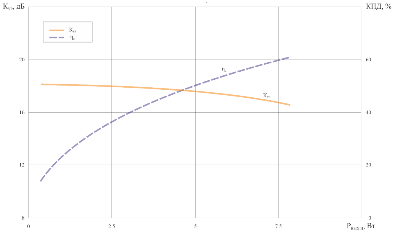
г) f_{\text{ТЕСТ}} = 3,2 ГГц
