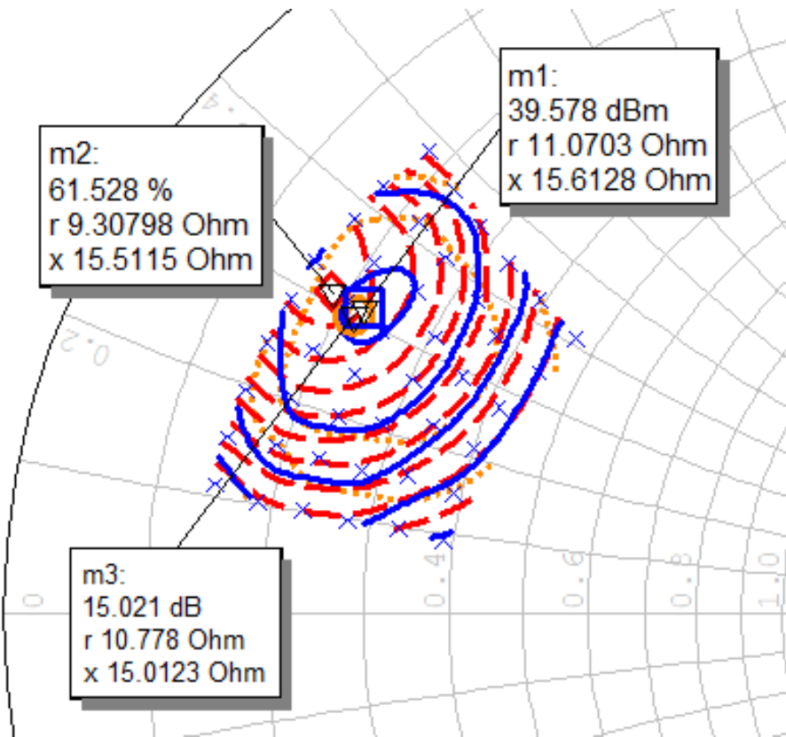
к) f_{\text{ТЕСТ}} = 5,0 \text{ ГГц}
