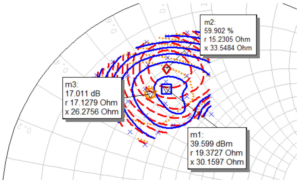
б) f_{ТЕСТ} = 2,8 ГГц
