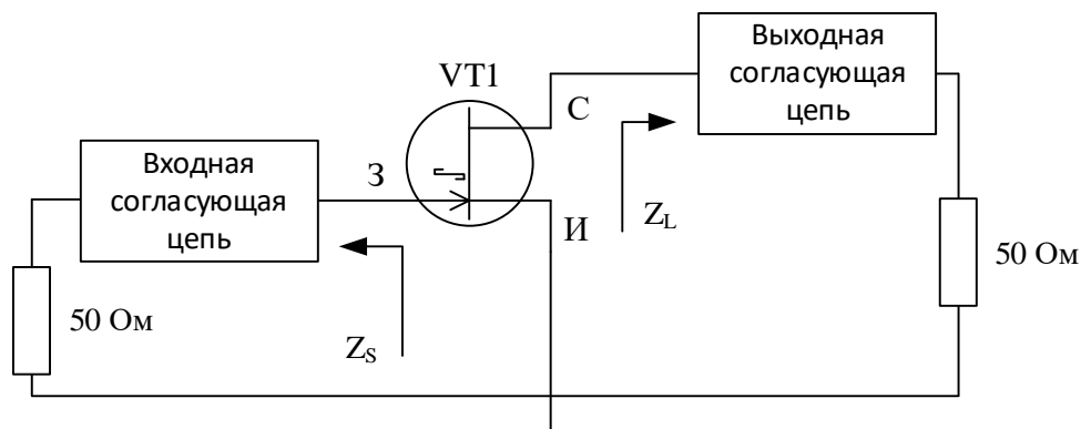
Рисунок 1 – Схема теста для определения импедансов источника и нагрузки
