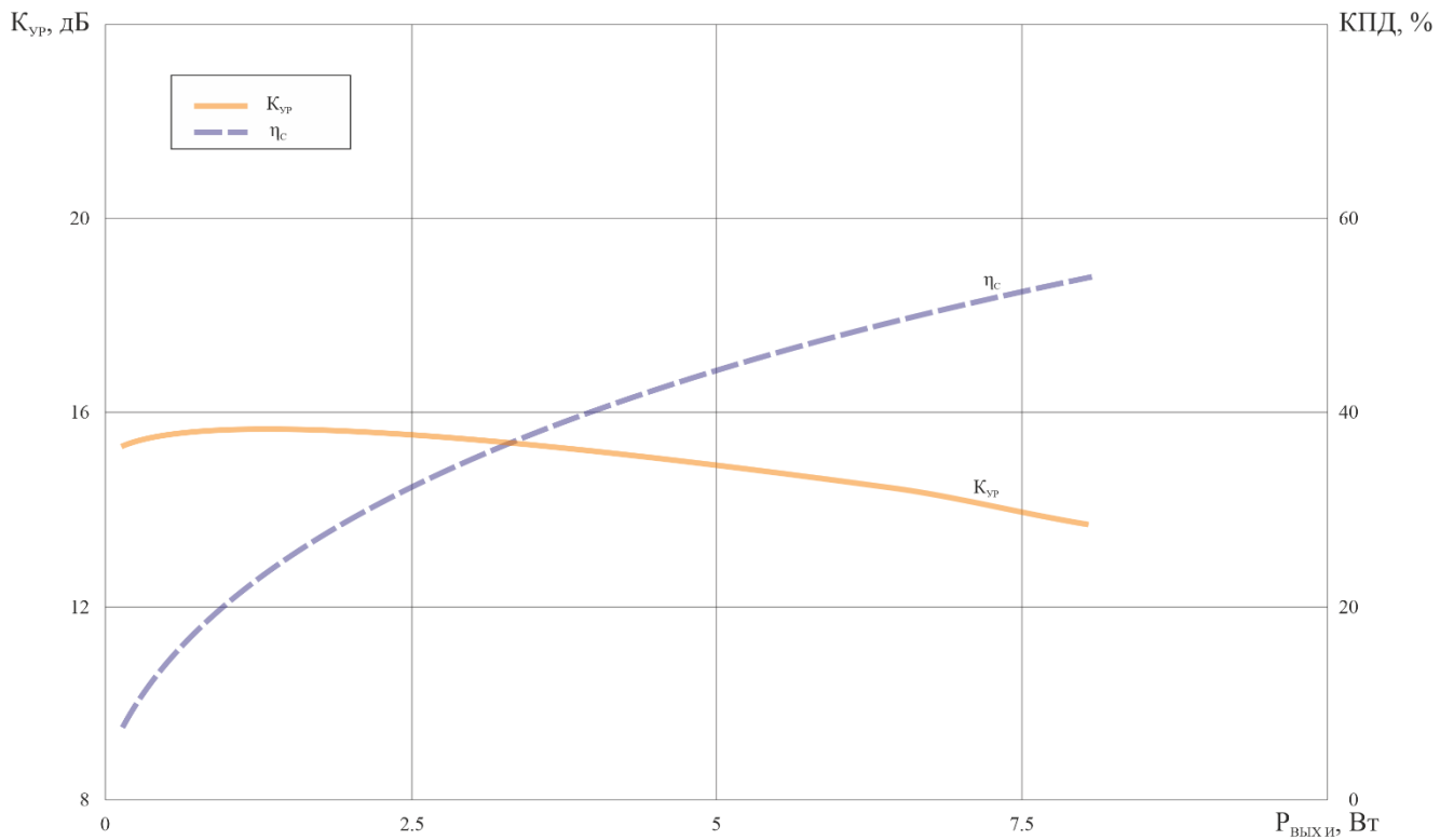
л) f_{\text{ТЕСТ}} = 5,5 \text{ ГГц}
