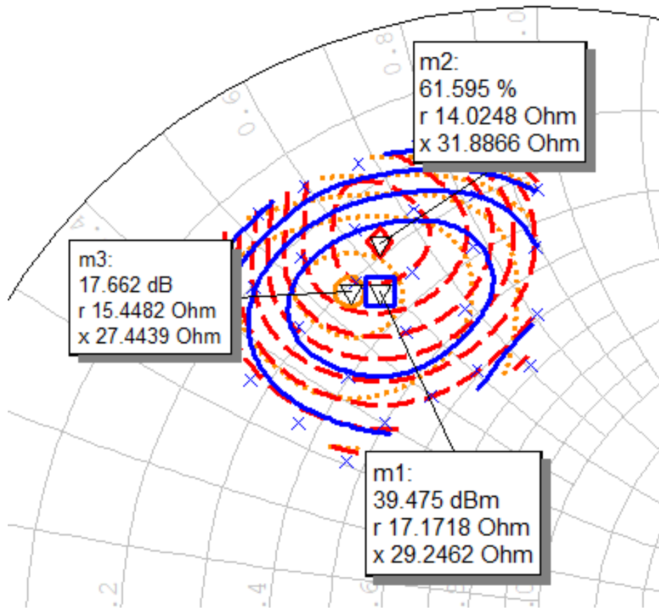
в) f_{\text{ТЕСТ}} = 3,0 \text{ ГГц}
