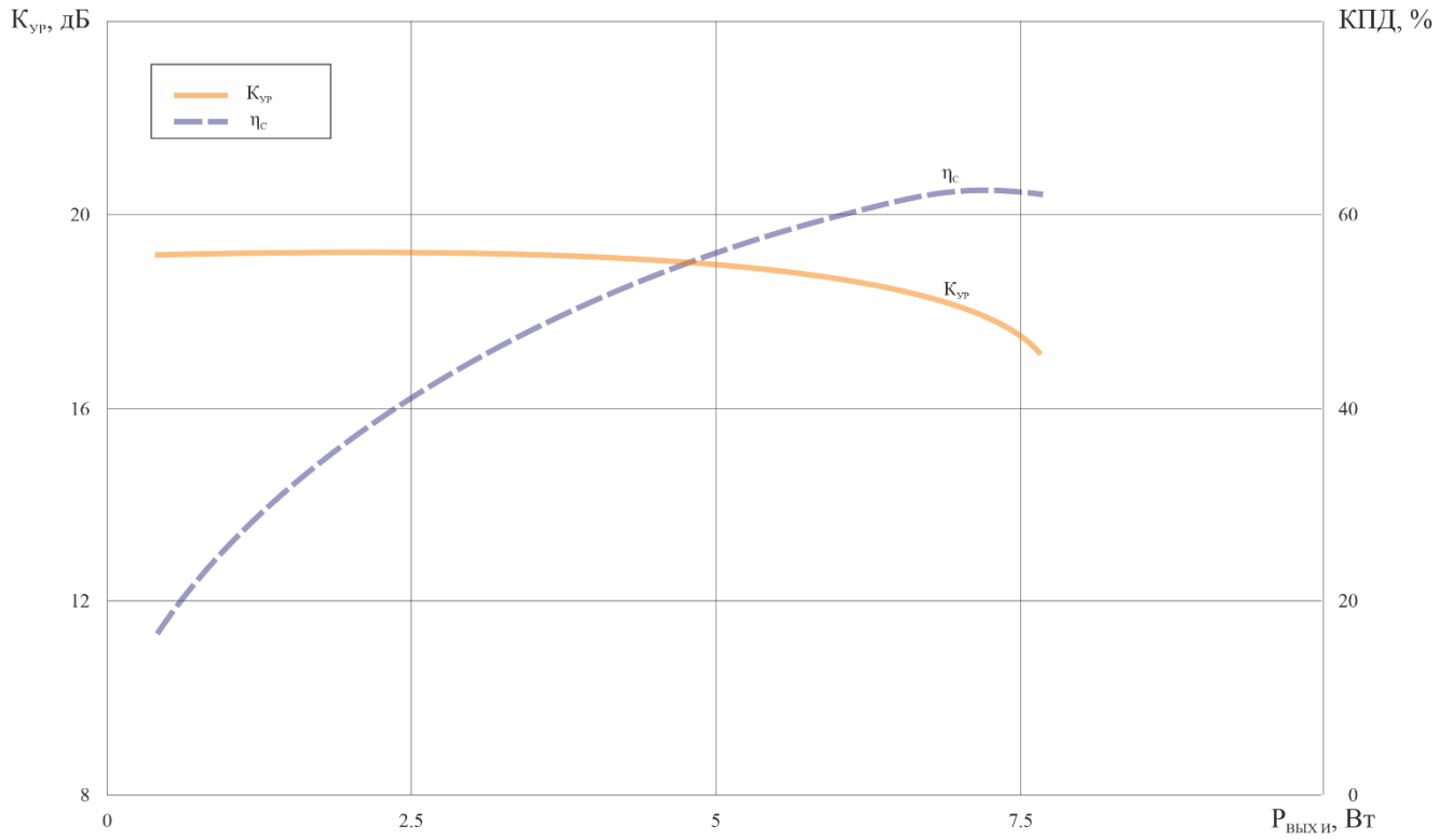
в) f_{\text{ТЕСТ}} = 3,0 ГГц
