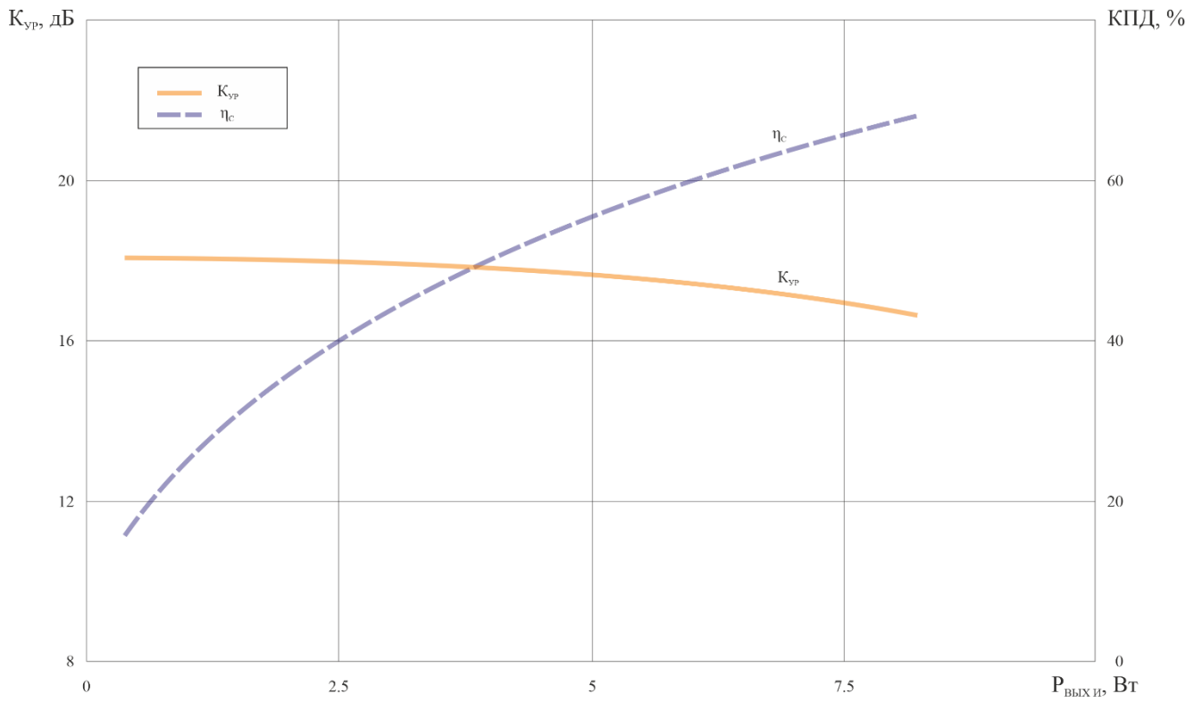
д) f_{\text{ТЕСТ}} = 3,4 \text{ ГГц}
