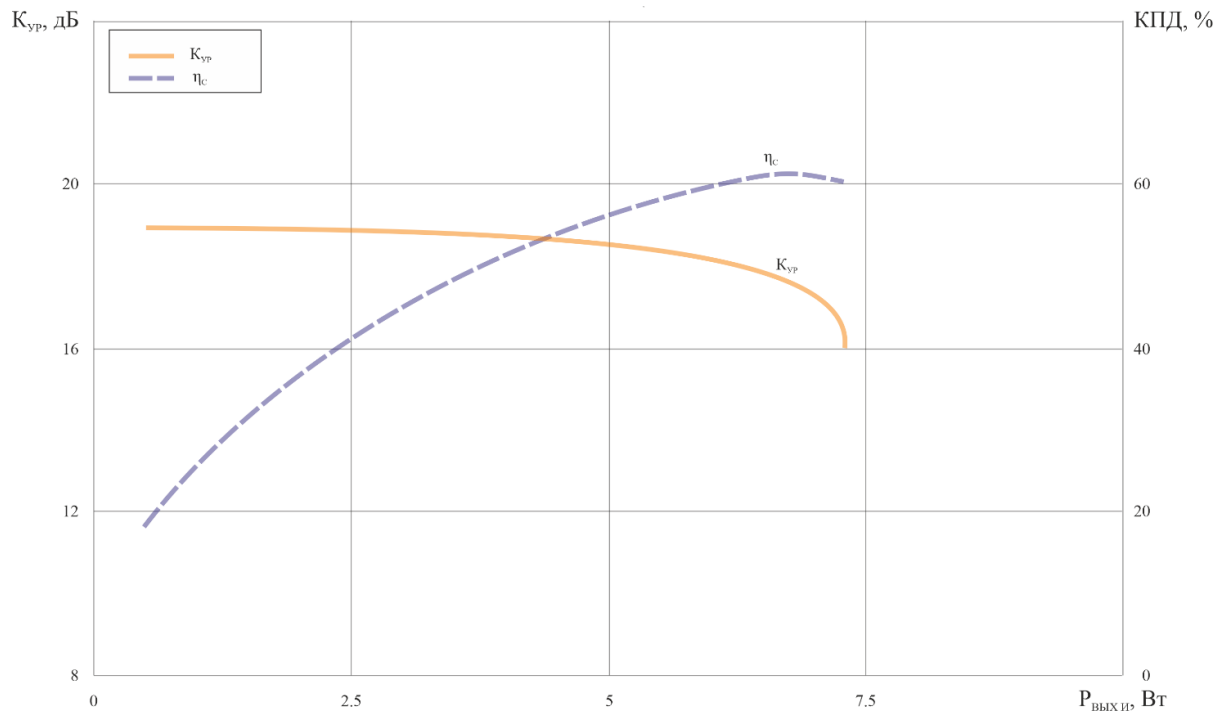
а) f_{ТЕСТ} = 2,8 ГГц
