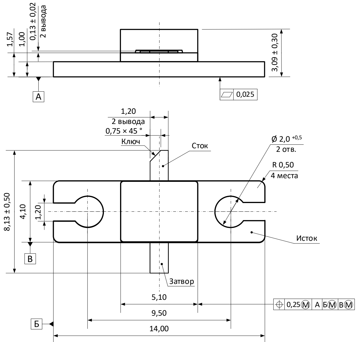
Рисунок 4 – Габаритный чертеж транзисторов MGN1643-5A
