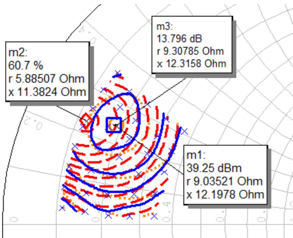
л) f_{\text{ТЕСТ}} = 5,5 \text{ ГГц}
