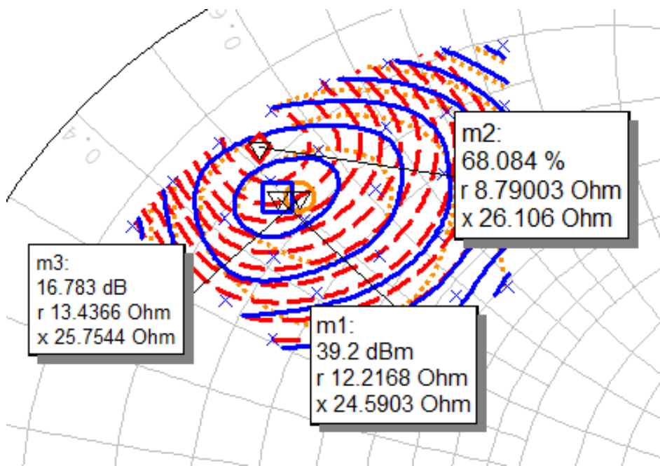
д) f_{\text{ТЕСТ}} = 3,4 \text{ ГГц}
