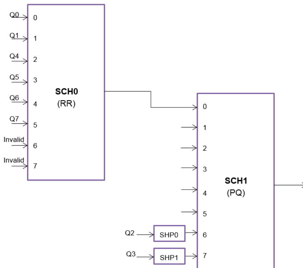
Рисунок 43 – Конфигурация TMU по умолчанию
