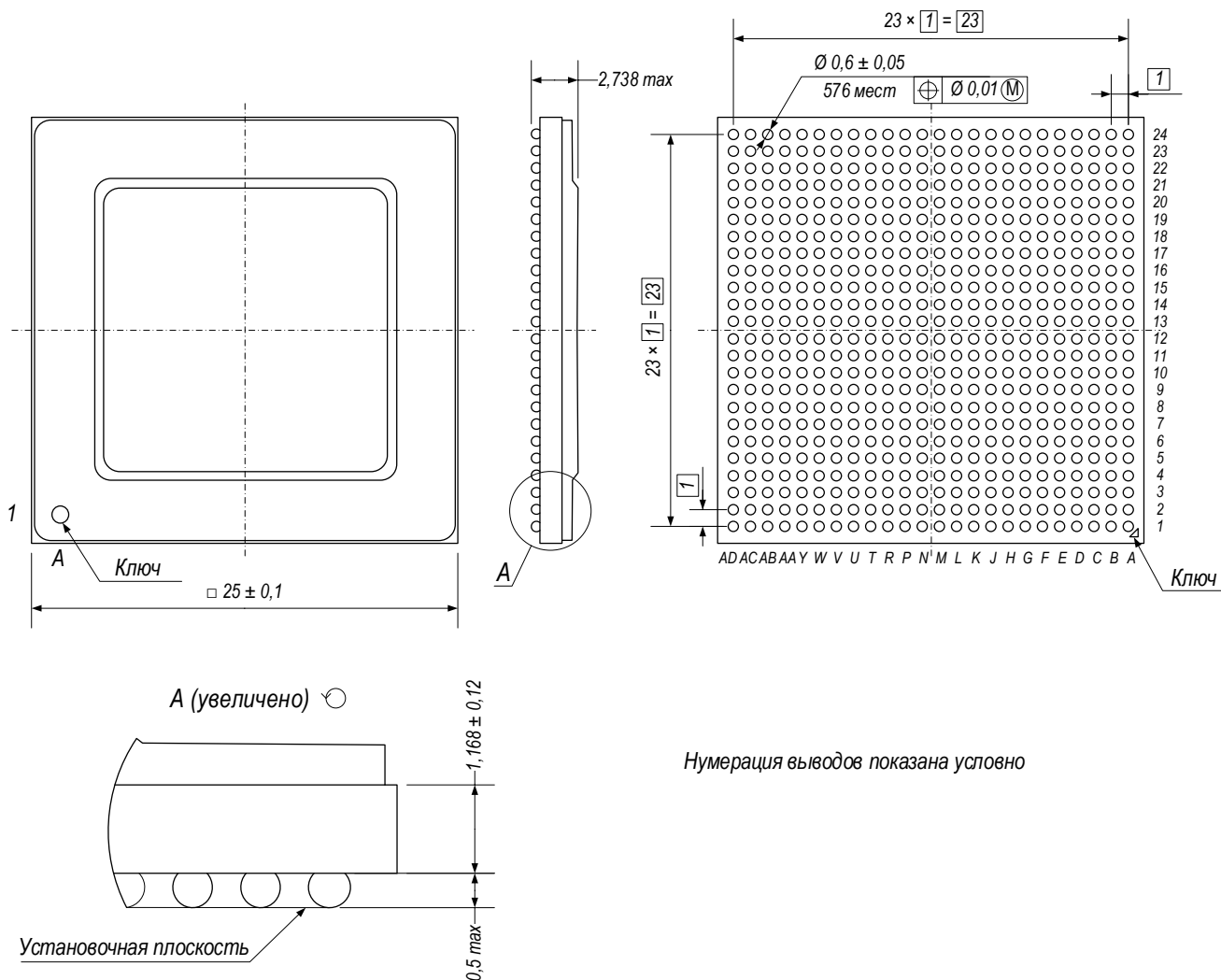
Рисунок 60 – Микросхема в корпусе BGA576 25×25×2,238 (1,0)
