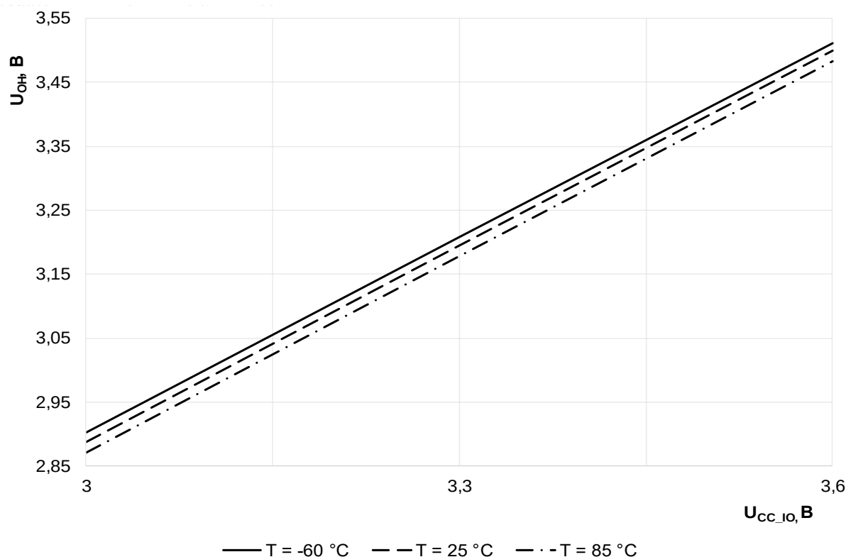
Рисунок 52 – Зависимость выходного напряжения высокого уровня U_{OH} на цифровых входах от напряжения питания на площадках ввода/вывода U_{CC\_IO} при низковольтном питании U_{CC} = 0.99 В и температурах T = 85 °C, T = 25 °C, T = -60 °C
