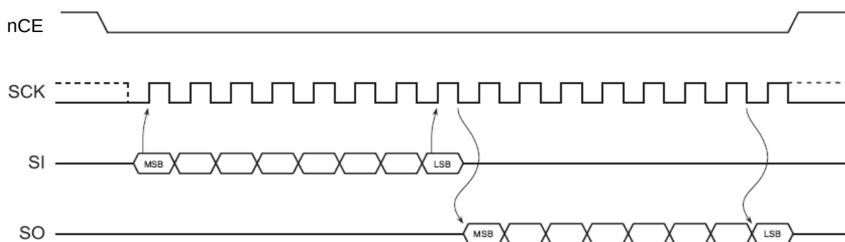
Рисунок 37 – Временная диаграмма режимов SPI 0 и 3
