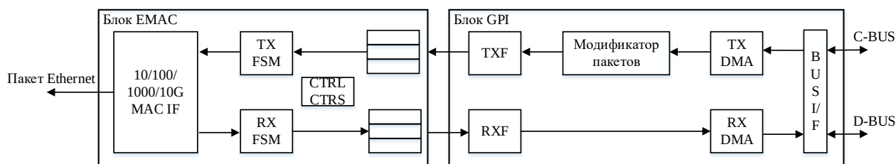
Рисунок 5 – Периферия Ethernet
