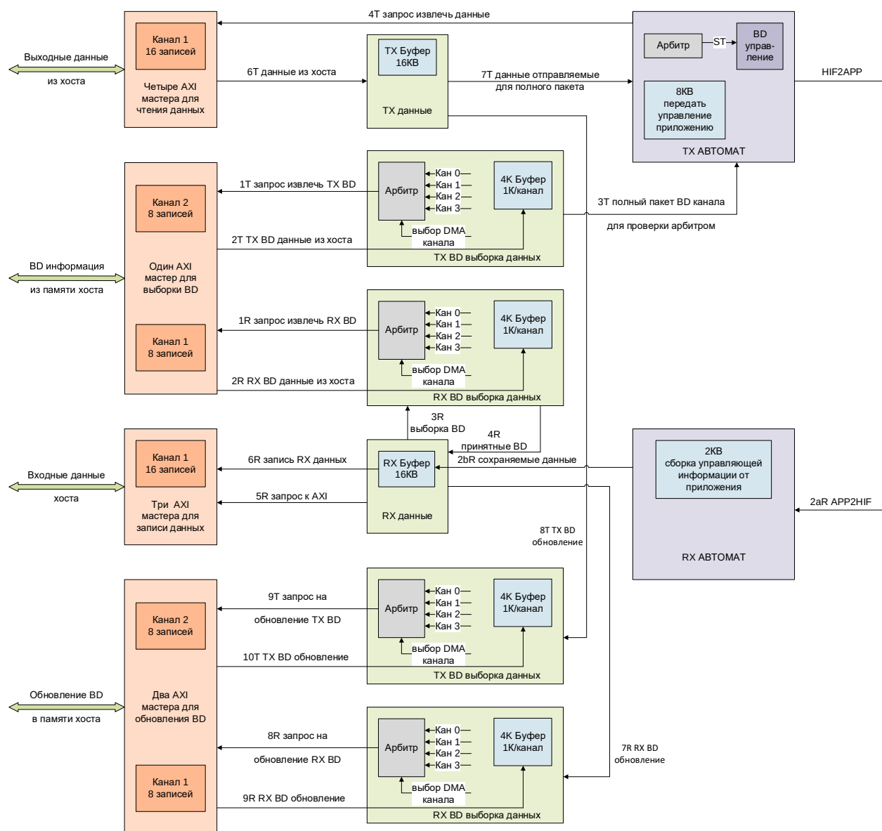
Рисунок 13 – Поток приема и передачи
