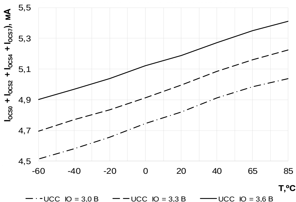
Рисунок 57 – Зависимость суммарного статического тока потребления выводов высоковольтного питания ( I_{OCS0} + I_{OCS2} + I_{OCS4} + I_{OCS7} ) от температуры при U_{CC\_IO} = 3,0\text{ V} , U_{CC\_IO} = 3,3\text{ V} , U_{CC\_IO} = 3,6\text{ V}
