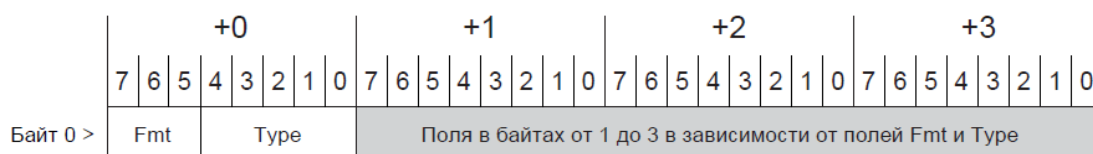
Рисунок 25 – Поля, представленные во всех TLP
