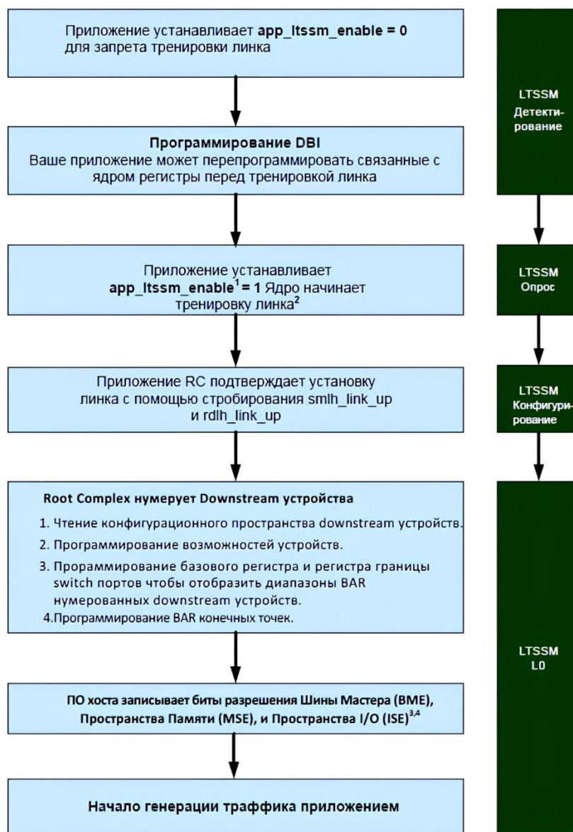
Рисунок 22 – Последовательность инициализации PCIe
