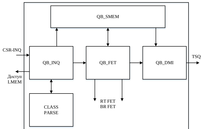
Рисунок 12 – Структура блока QB
