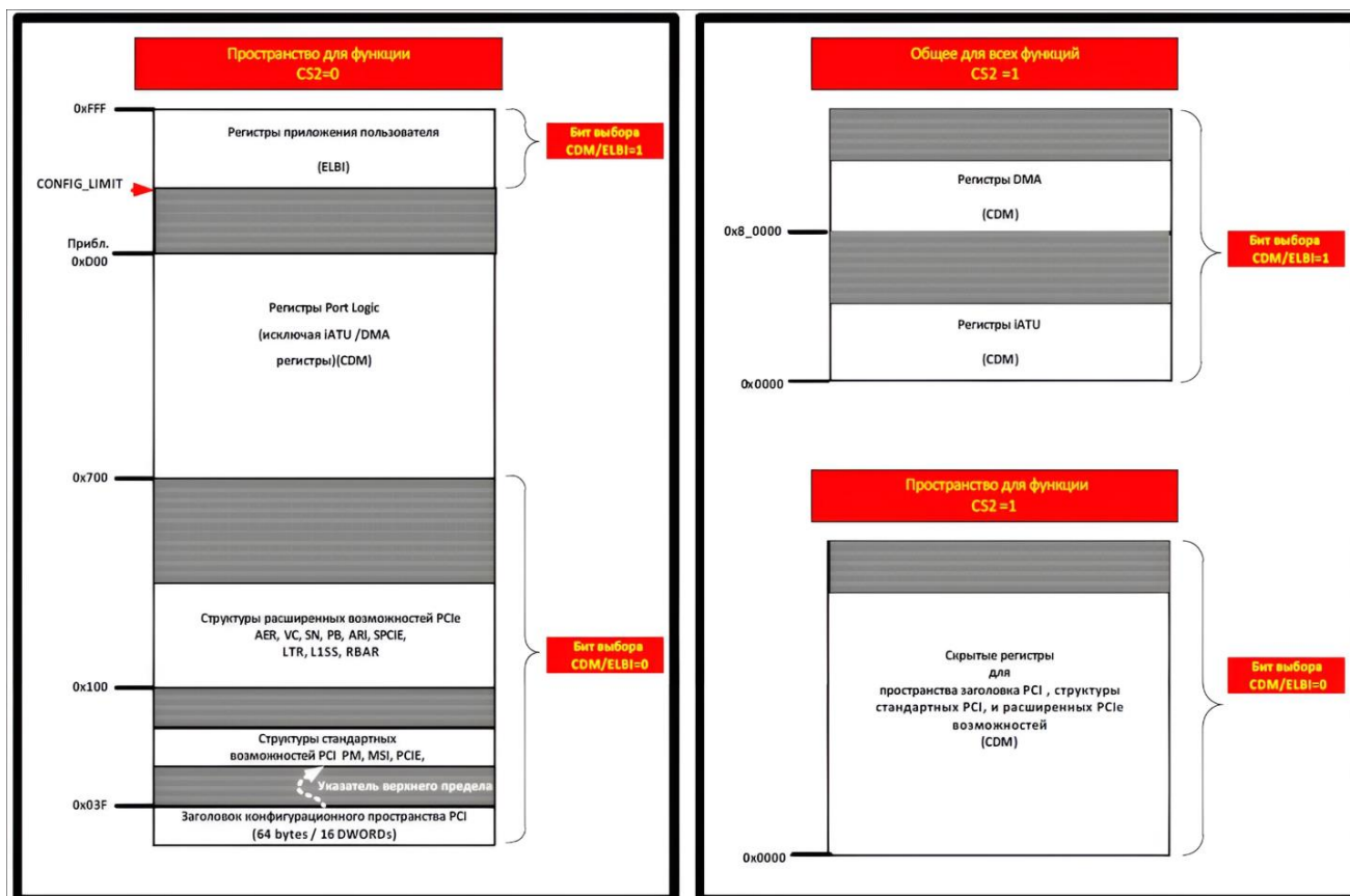
Рисунок 31 – Схема размещения пространства конфигурации контроллера
