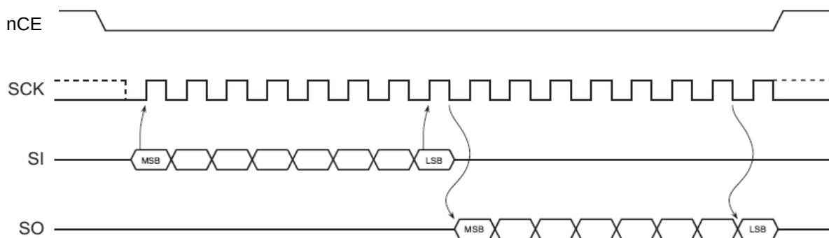
Рисунок 44 – Временная диаграмма режимов SPI 0 и 3
