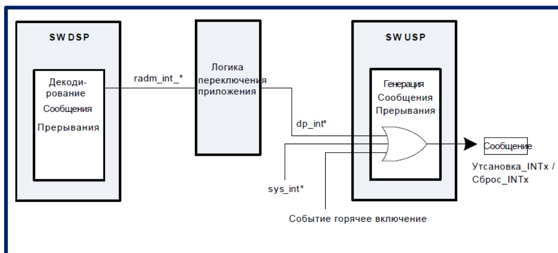
Рисунок 36 – Генерация сообщений: Установка_INTx и Сброс_INTx
