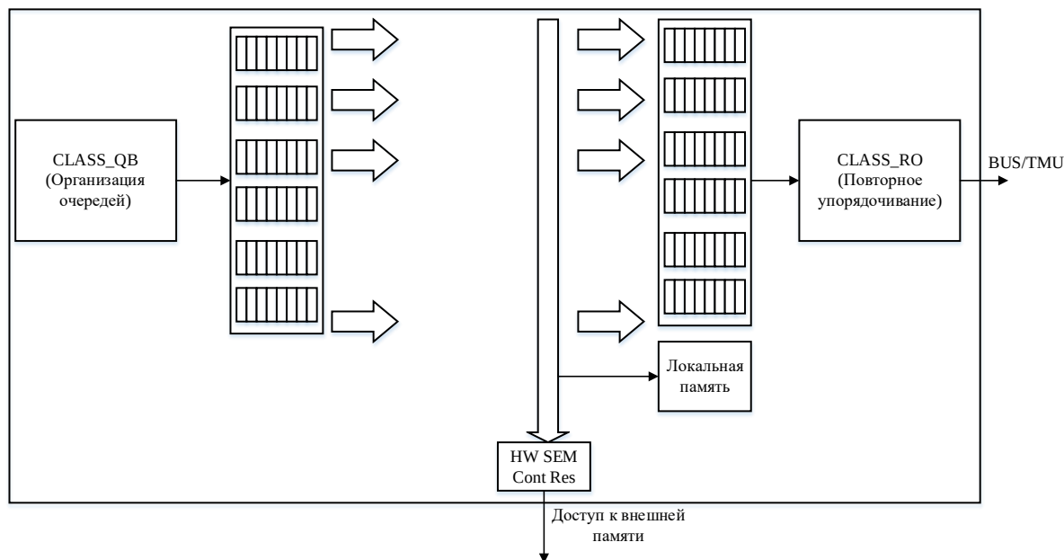
Рисунок 11 – Структурная схема классификатора
