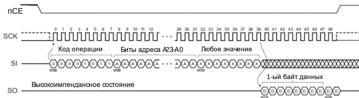
Рисунок 45 – Операция чтения с кодом 0Bh
