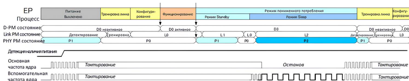
Рисунок 23 – Временная диаграмма инициализации PCIe
