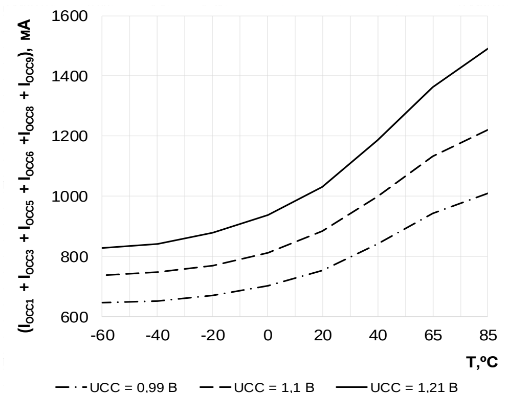
Рисунок 58 – Зависимость суммарного динамического тока потребления на выводах низковольтного питания ( I_{OCC1} + I_{OCC3} + I_{OCC5} + I_{OCC6} + I_{OCC8} + I_{OCC9} ) от температуры при U_{CC} = 0,99 В, U_{CC} = 1,1 В, U_{CC} = 1,21 В
