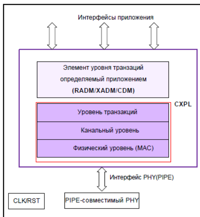
Рисунок 20 – Архитектура контроллера PCIe
