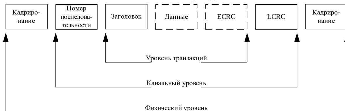
Рисунок 24 – Прохождение пакетов через уровни
