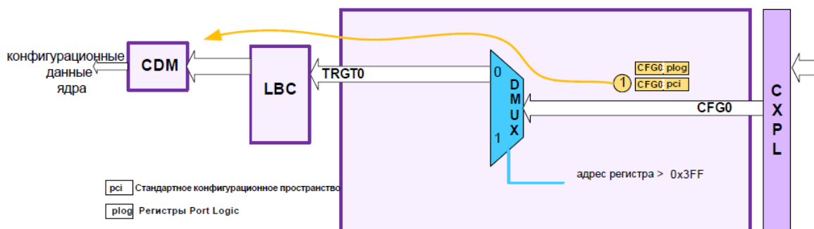
Рисунок 32 – Маршрутизация TLP-запроса: типичная модель применения
