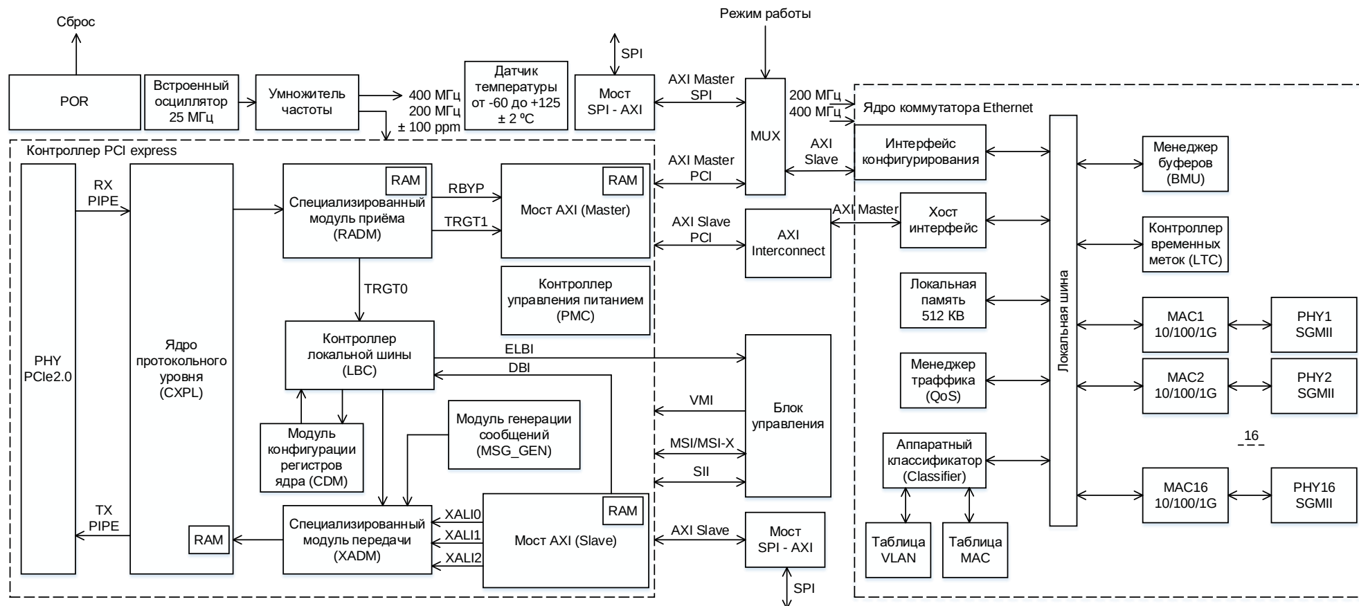
Рисунок 1 – Структурная блок-схема микросхемы
