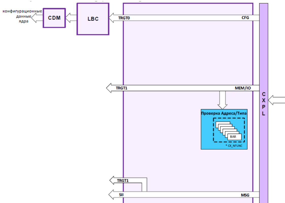
Рисунок 28 – Маршрутизация запроса TLP по умолчанию (при условии, что TLP без CA/CRS/UR ошибки статуса)
