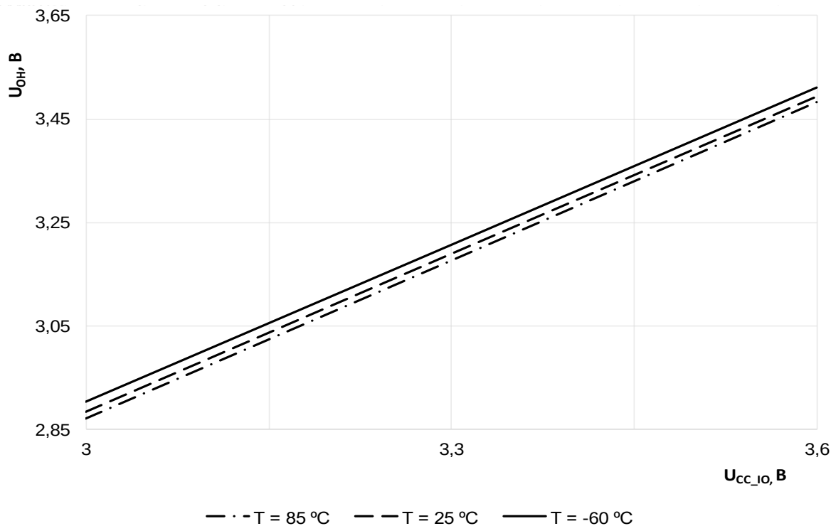
Рисунок 53 – Зависимость выходного напряжения высокого уровня U_{OH} на цифровых входах от напряжения питания на площадках ввода/вывода U_{CC\_IO} при низковольтном питании U_{CC} = 1.21 В и температурах T = 85 °C, T = 25 °C, T = -60 °C
