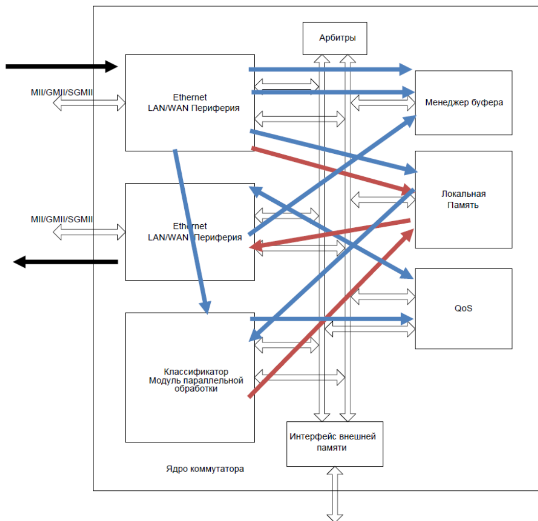
Рисунок 18 – Архитектура потока данных
