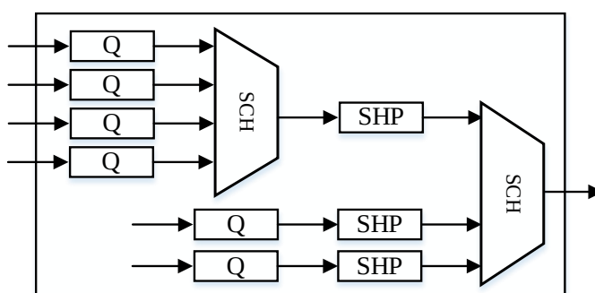
Рисунок 7 – Пример формирователя с планировщиком
