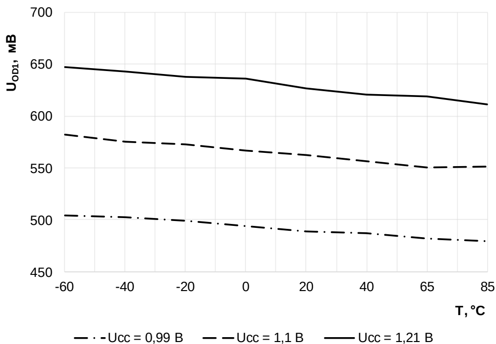
Рисунок 49 – Зависимость дифференциального выходного напряжения на выходах SGMII U_{OD1} от температуры при U_{CC\_IO} = 3,6 В, R_L = 100 Ом \pm 1 %
