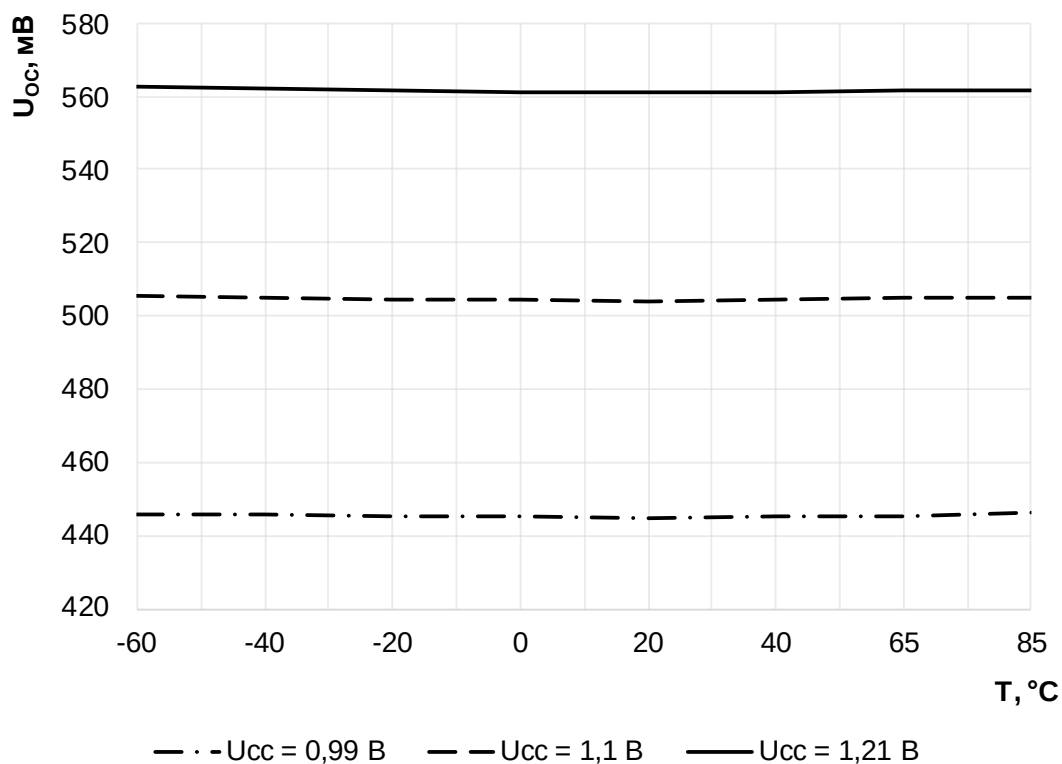
Рисунок 50 – Зависимость синфазного выходного напряжения U_{oc} на выходах PCIE от температуры при U_{CC\_IO} = 3,6 В, R_L = 100 Ом \pm 1 %
