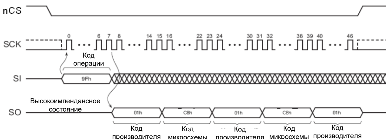
Рисунок 41 – Операция чтения ID-кодов
