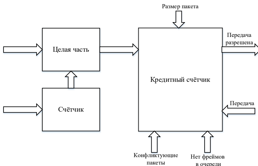
Рисунок 8 – Структурная схема формирователя
