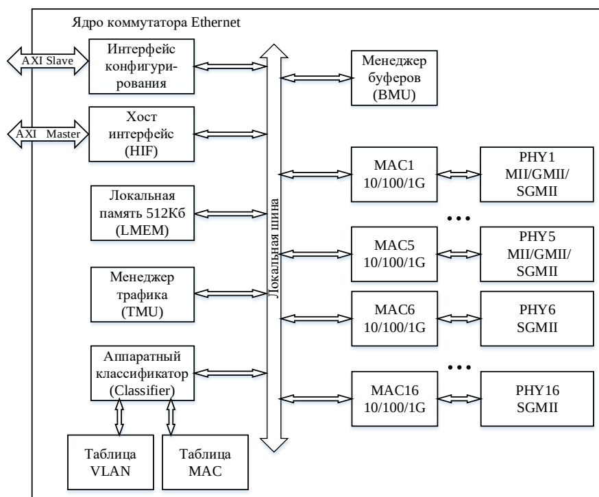
Рисунок 4 – Аппаратная архитектура
