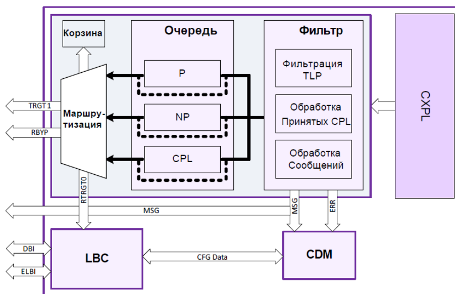
Рисунок 27 – Структурная схема блока RADM
