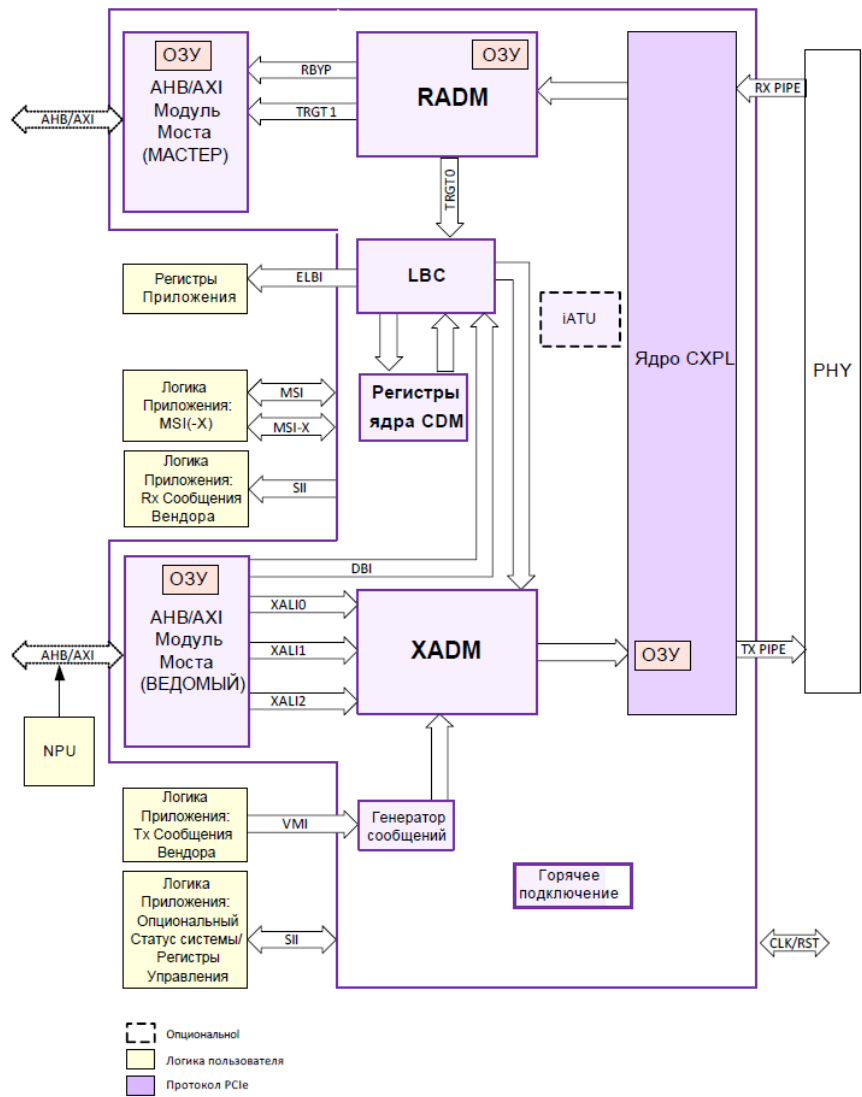
Рисунок 21 – Структурная схема ядра Endpoint (с модулем моста АНВ/АХІ)
