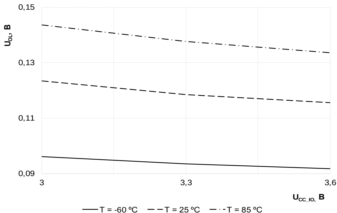
Рисунок 54 – Зависимость выходного напряжения низкого уровня U_{OL} на цифровых входах от напряжения питания на площадках ввода/вывода U_{CC\_IO} при низковольтном питании U_{CC} = 0.99 В и температурах T = 85 °C, T = 25 °C, T = -60 °C
