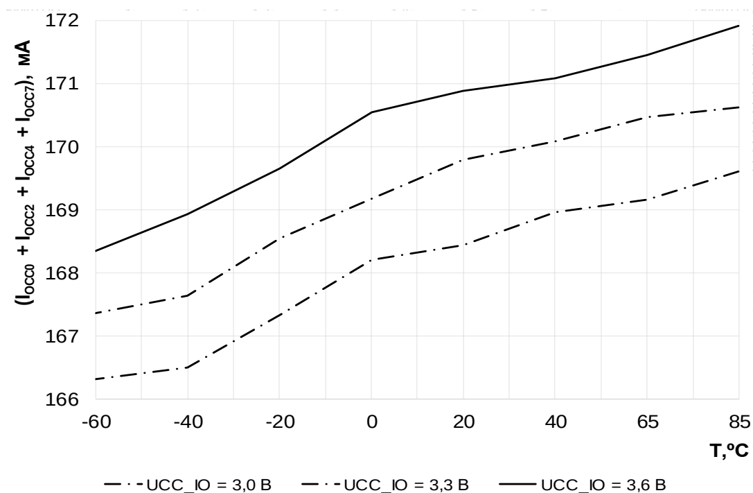
Рисунок 59 – Зависимость суммарного динамического тока потребления в выводах высоковольтного питания ( I_{OCC0} + I_{OCC2} + I_{OCC4} + I_{OCC7} ) от температуры при U_{CC\_IO} = 3,0 В, U_{CC\_IO} = 3,3 В, U_{CC\_IO} = 3,6 В
