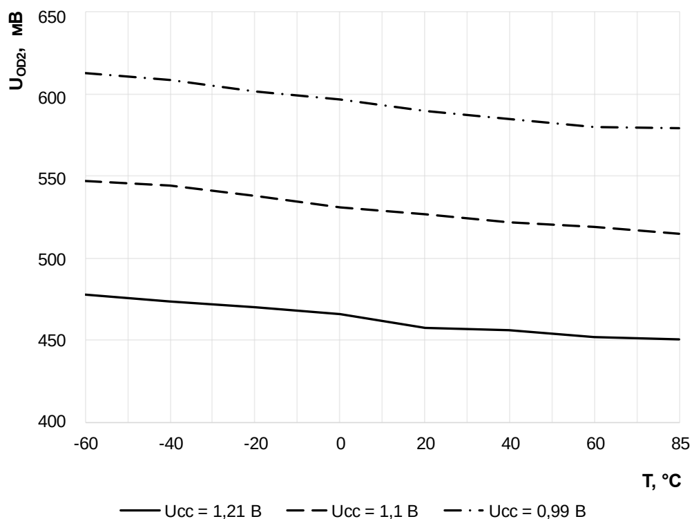
Рисунок 48 – Зависимость дифференциального выходного напряжения на выходах PCIE U_{OD2} от температуры при U_{CC\_IO} = 3,6 В, R_L = 100 Ом \pm 1 %
