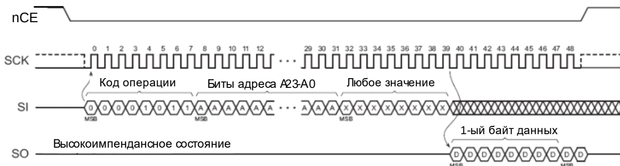
Рисунок 38 – Операция чтения с кодом 0Bh
