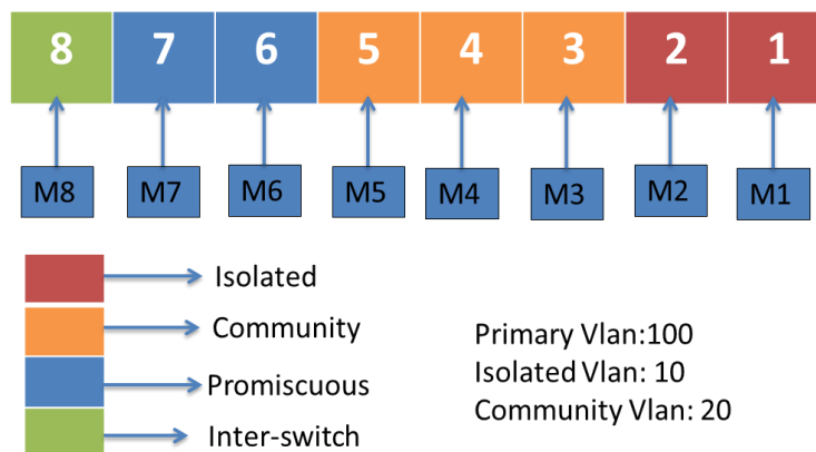
Рисунок 46 – Подключение коммутатора к устройствам
