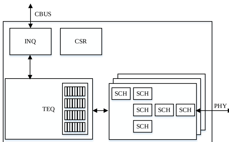
Рисунок 6 – Структурная схема блока TMU
