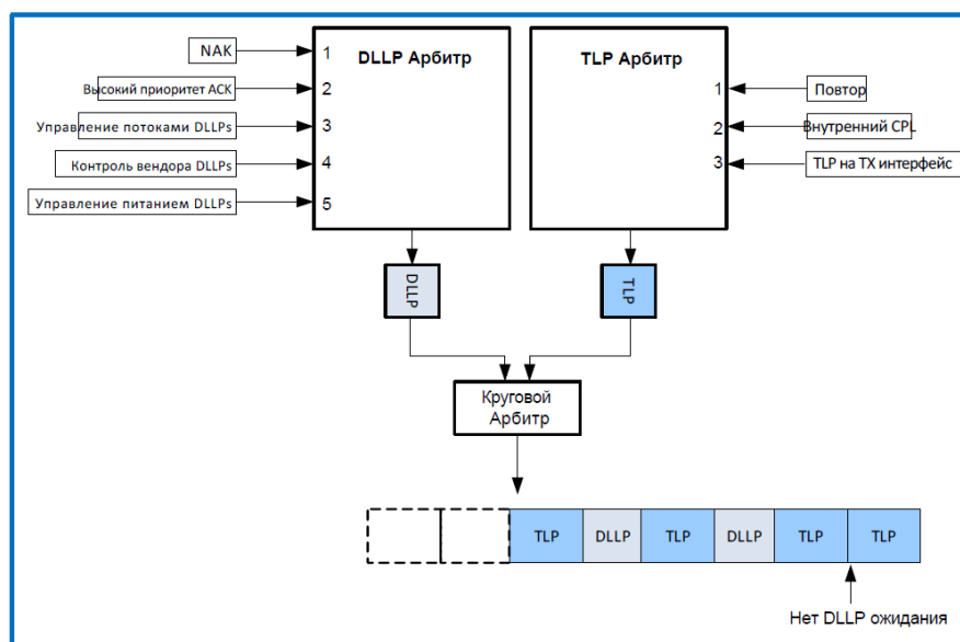
Рисунок 26 – Арбитраж передаваемых TLP/DLLP
