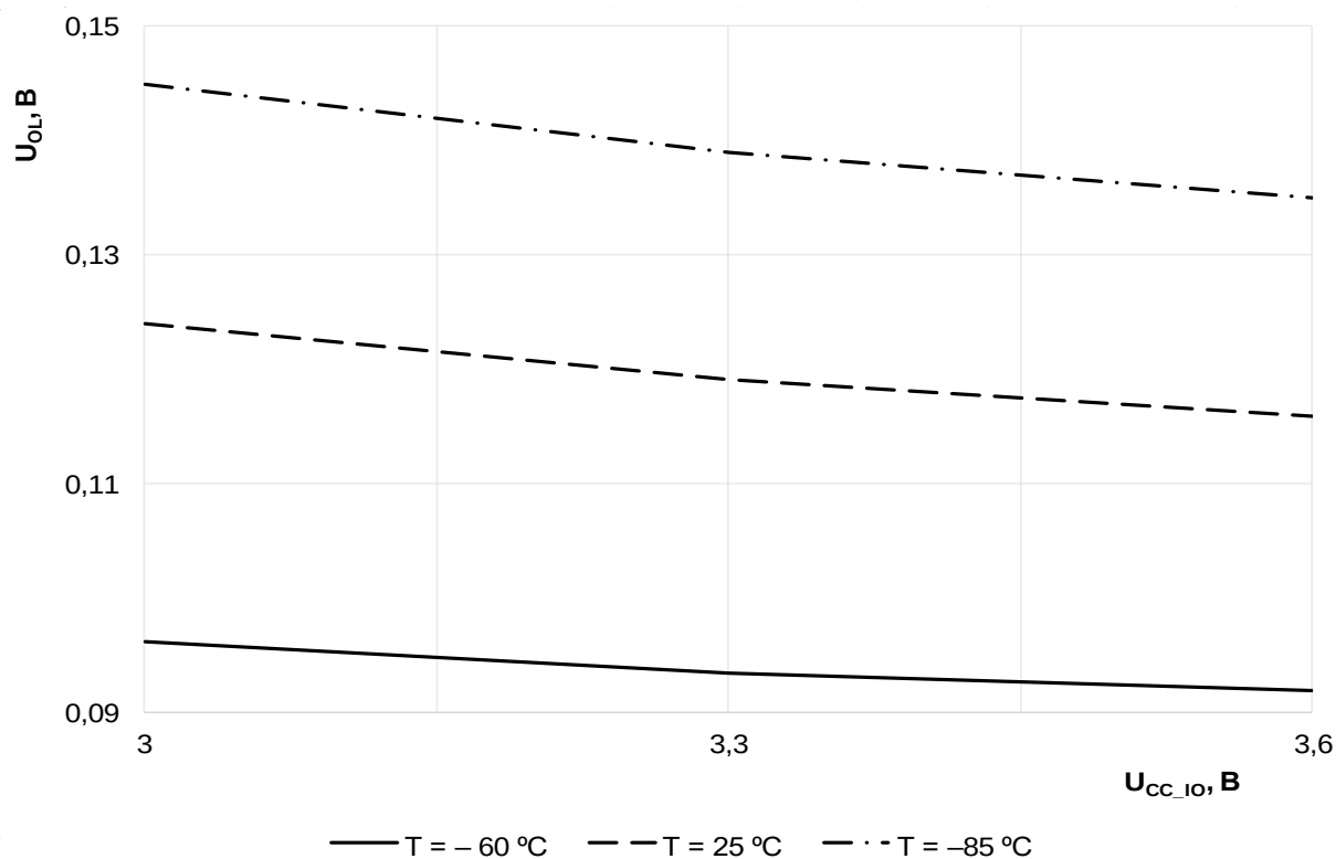
Рисунок 55 – Зависимость выходного напряжения низкого уровня U_{OL} на цифровых входах от напряжения питания на площадках ввода/вывода U_{CC\_IO} при низковольтном питании U_{CC} = 1.21 В и температурах T = 85 °C, T = 25 °C, T = -60 °C
