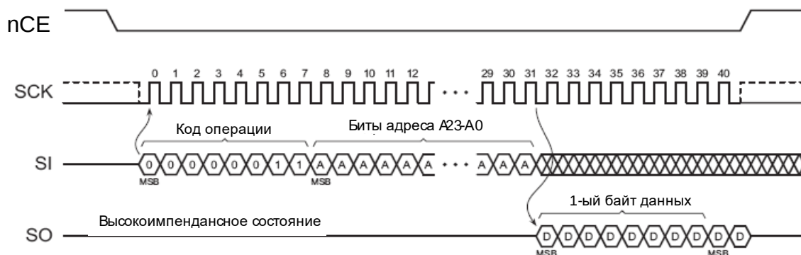
Рисунок 39 – Операция чтения с кодом 05h
