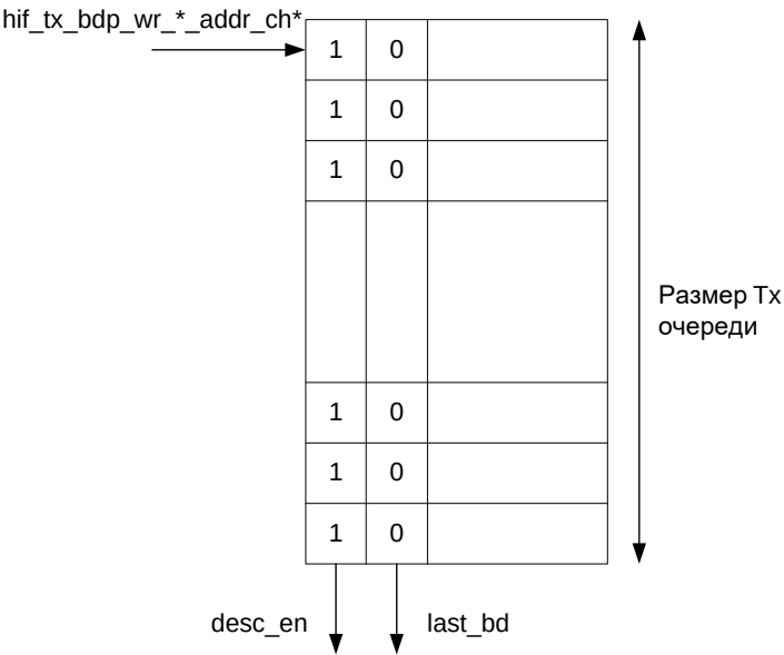
Рисунок 16 – Очередь буфера дескриптора
