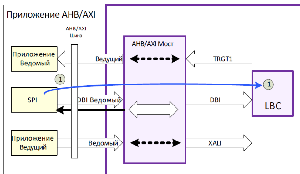
Рисунок 33 – Доступ AXI DBI через выделенный слэив интерфейс
