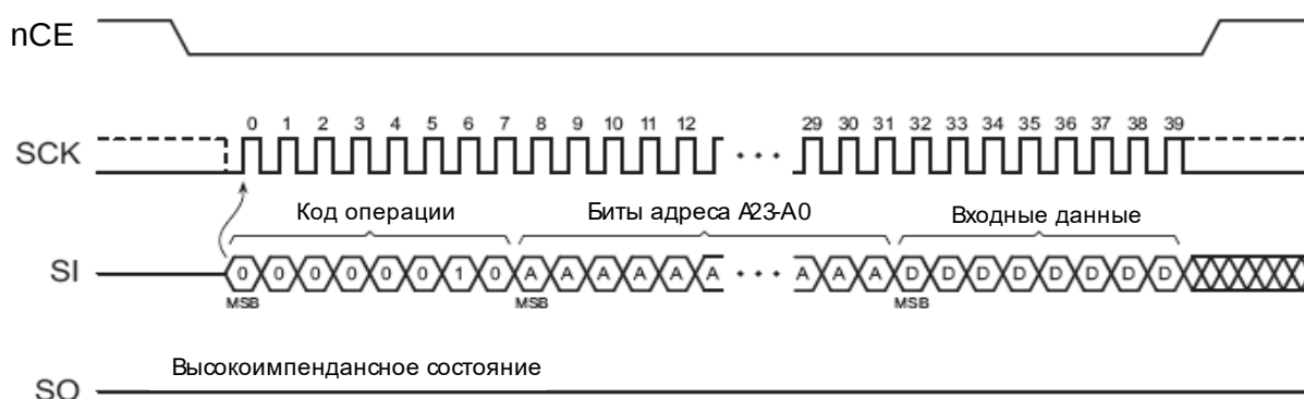
Рисунок 40 – Операция программирования 32-разрядного слова
