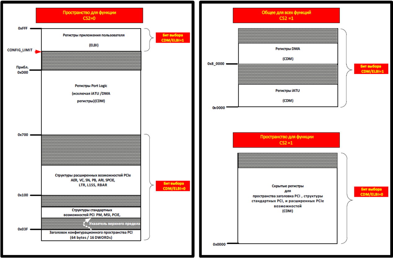
Рисунок 42 – Конфигурационное пространство PCI Express
