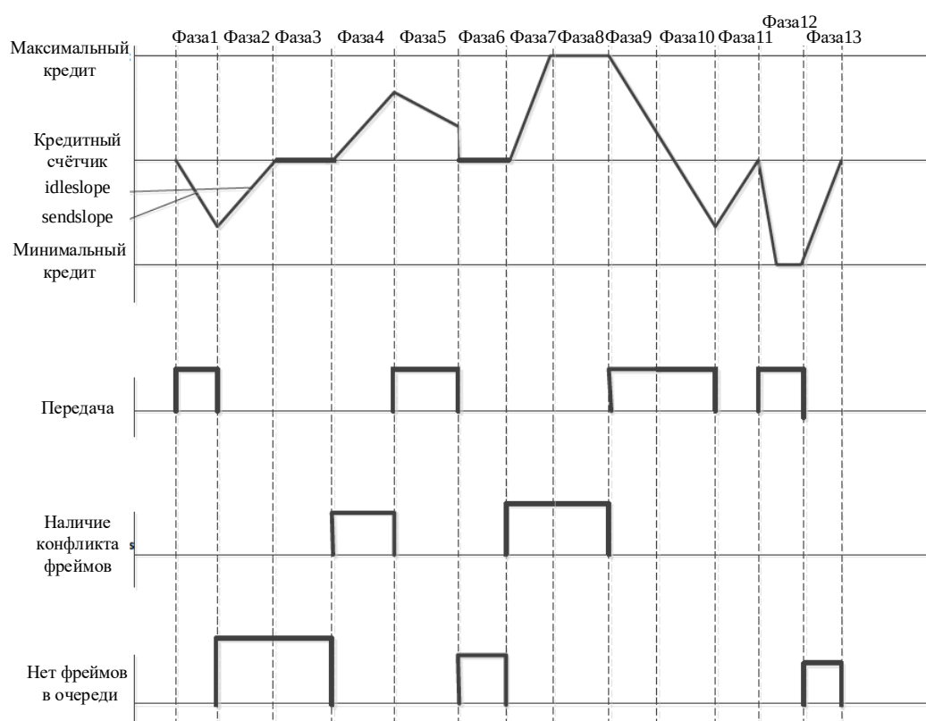
Рисунок 9 – Поведение формирователя в зависимости от входов
