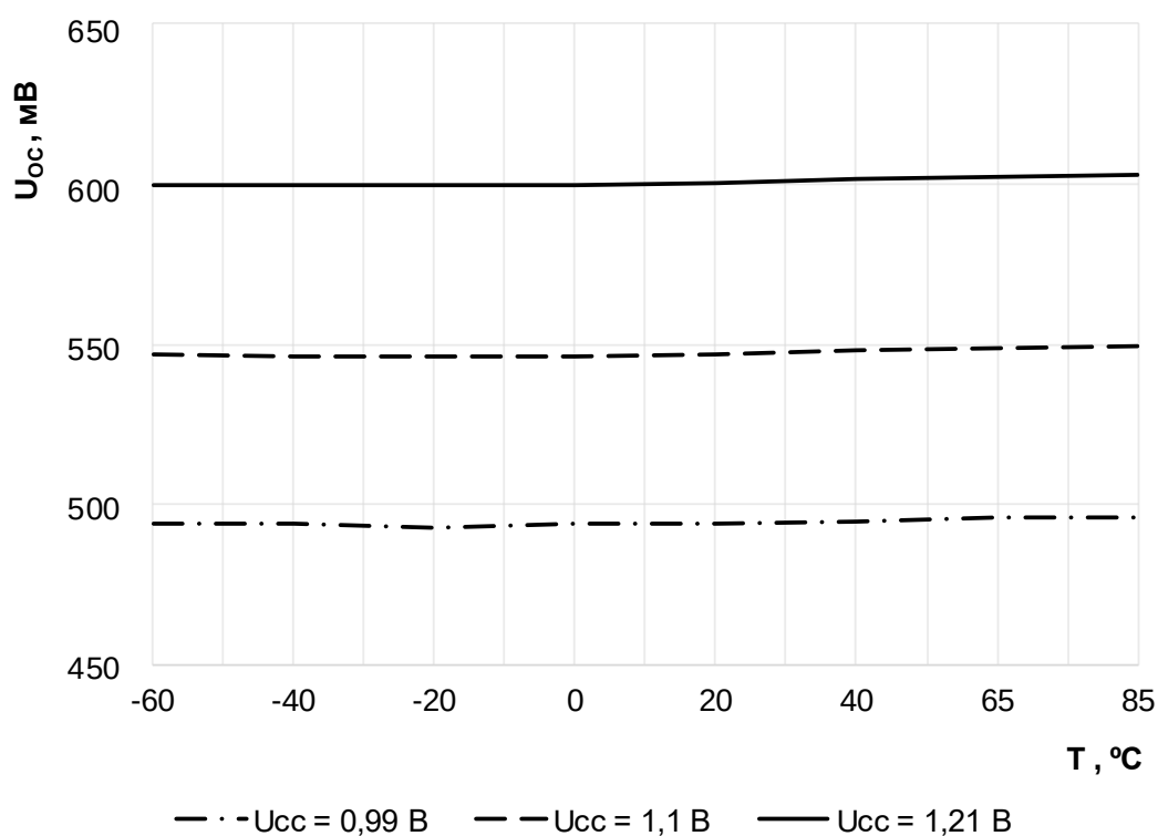
Рисунок 51 – Зависимость синфазного выходного напряжения U_{oc} на выходах SGMII от температуры при U_{CC\_IO} = 3,6 В, R_L = 100 Ом \pm 1 %
