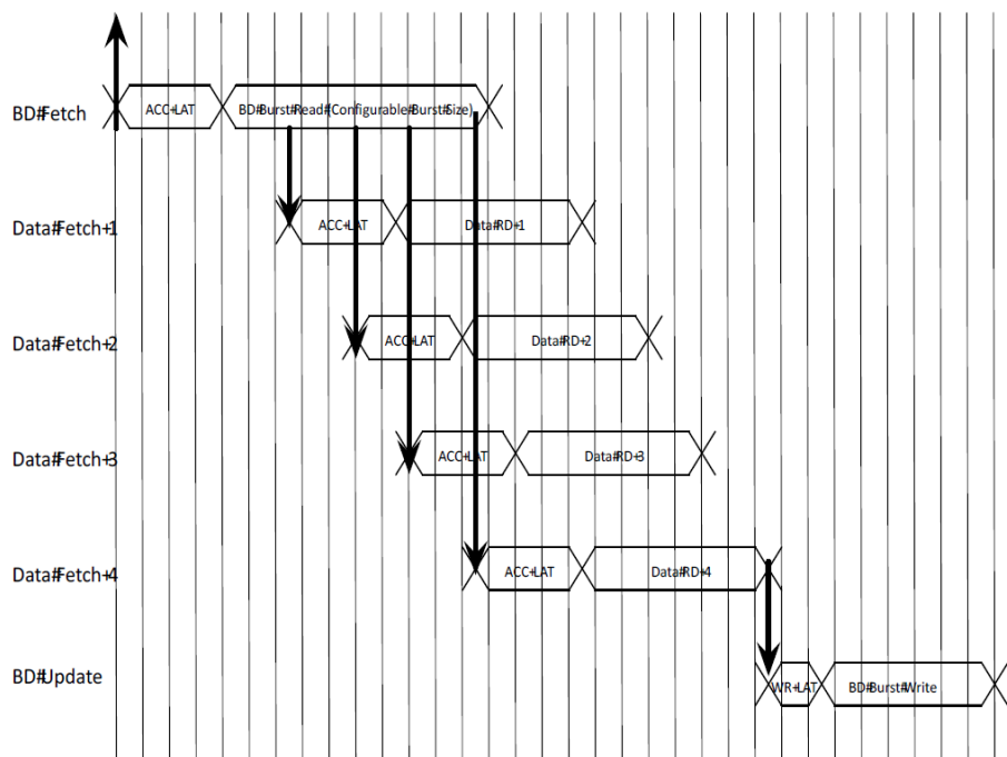
Рисунок 14 – Временная диаграмма потока данных
