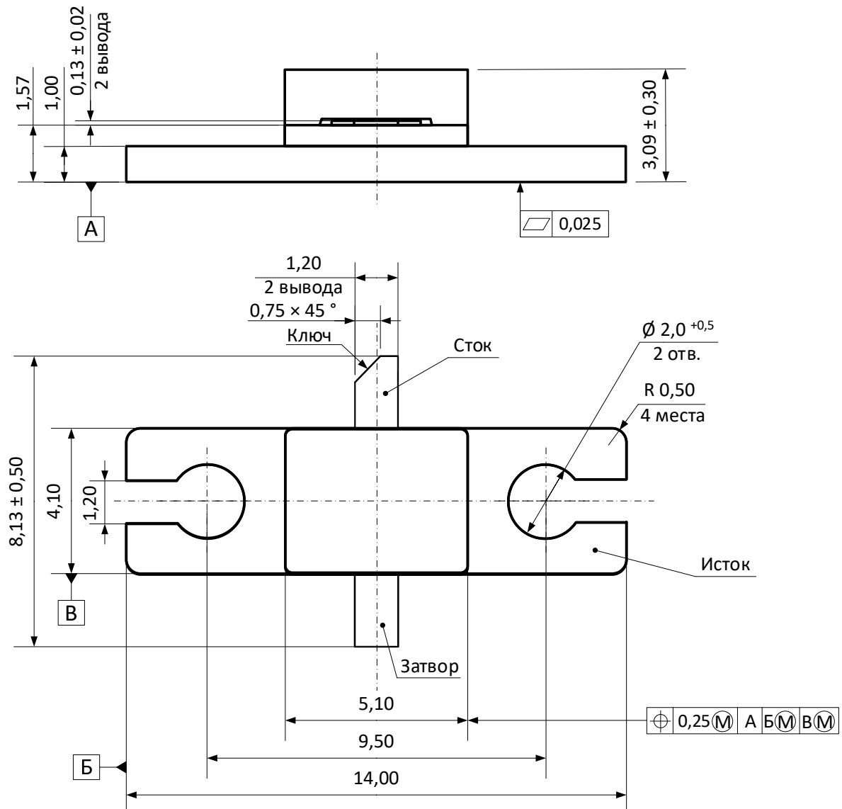
Рисунок 4 – Габаритный чертеж транзисторов MGN1643-25A
