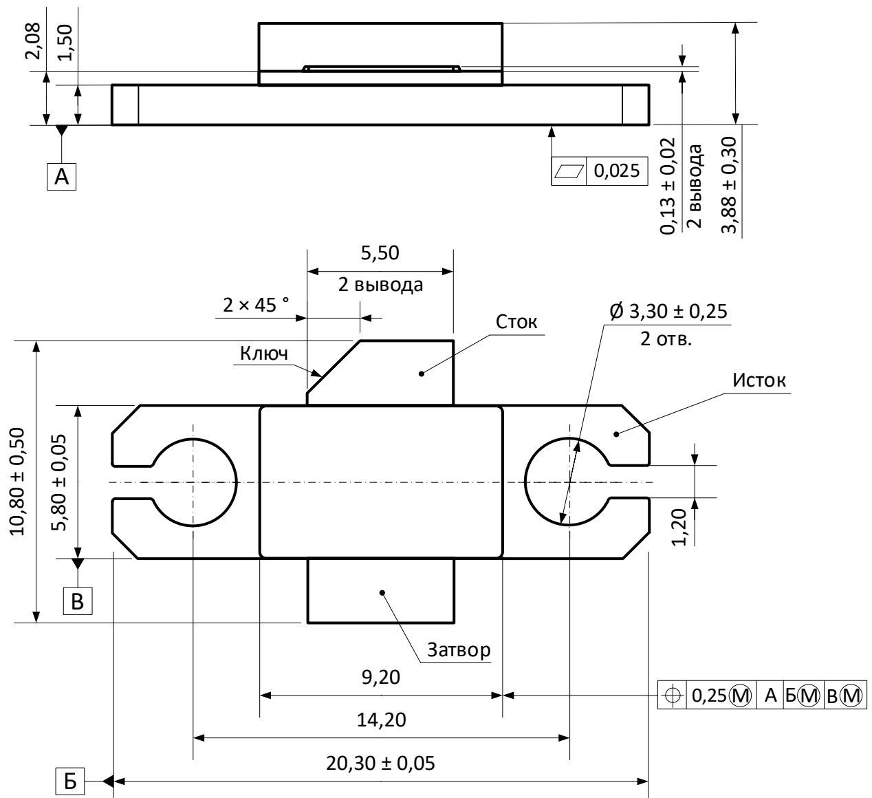
Рисунок 2 – Габаритный чертеж транзисторов MGN16-250A
