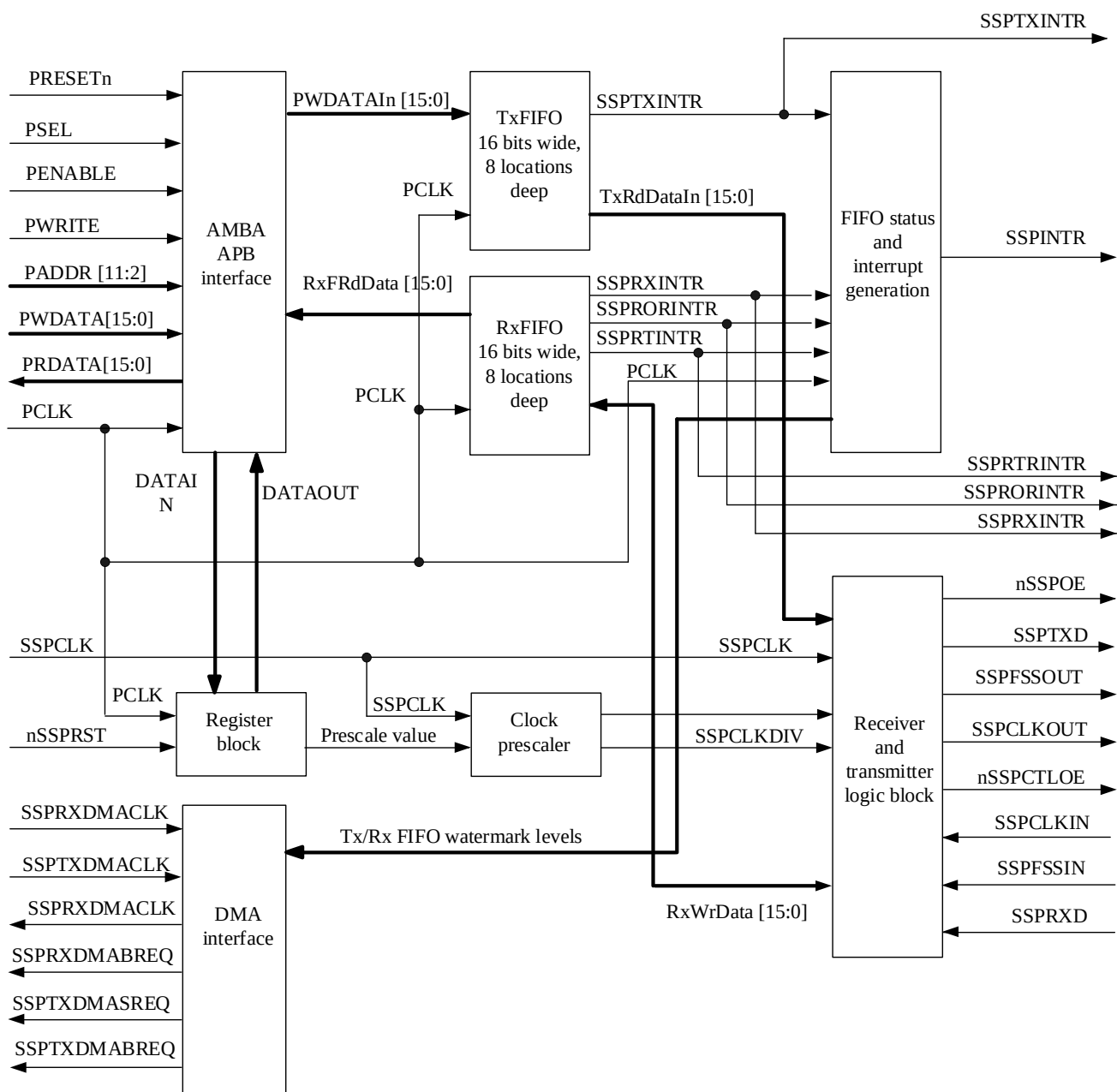
Рисунок 95 – Структурная схема модуля SSP
