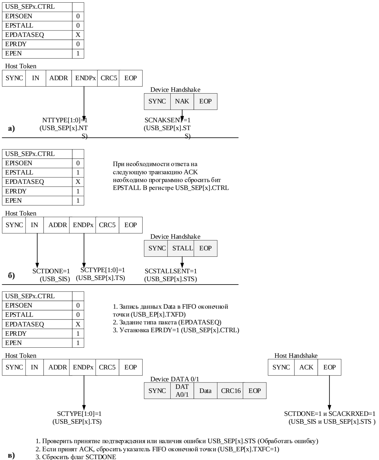
Рисунок 35 – Транзакция IN (USB Device)
