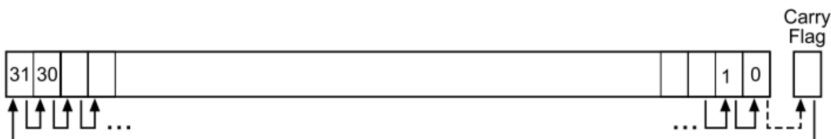
Рисунок 24 – Инструкция RRX
