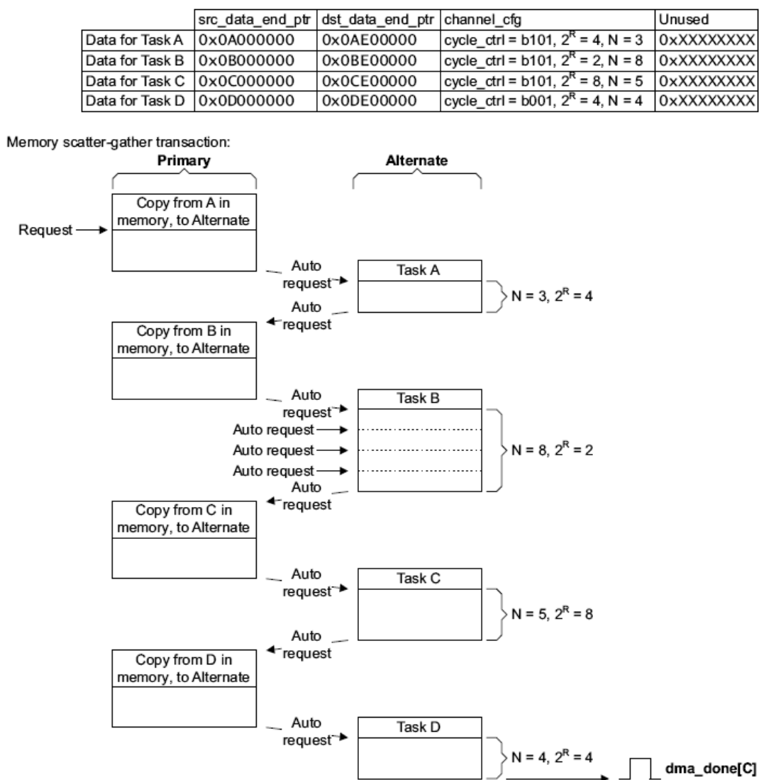
Рисунок 126 – Пример работы DMA в режиме с «Исполнением с изменением конфигурации»
