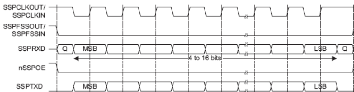
Рисунок 103 – Формат синхронного обмена протокола SPI, SPO=1, SPH=1
