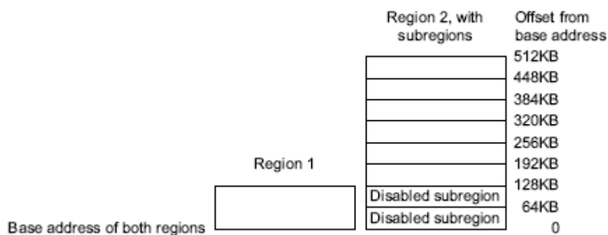
Рисунок 25 – Применение SRD
