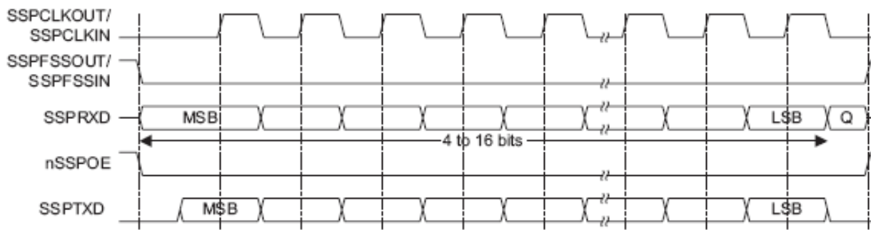
Рисунок 98 – Формат синхронного обмена протокола SPI, SPO=0, SPH=0 (одиночный обмен)
