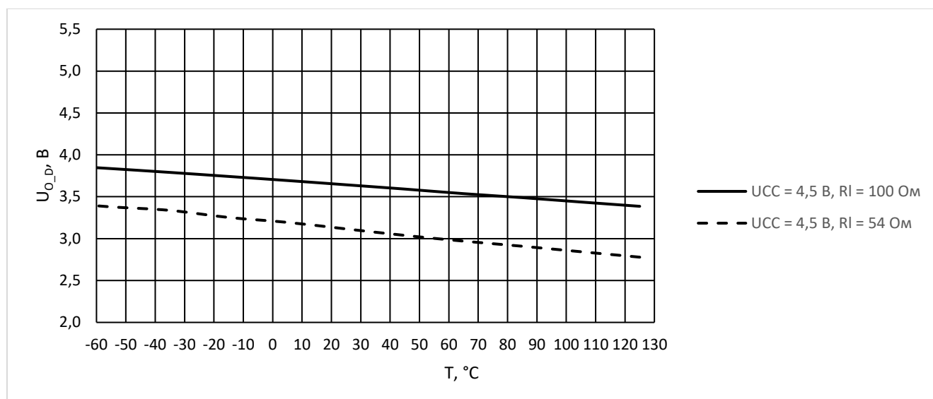
Рисунок 12 – Зависимость выходного дифференциального напряжения передатчика U_{O\_D} от температуры при U_{CC} = 4,5 \text{ В}
