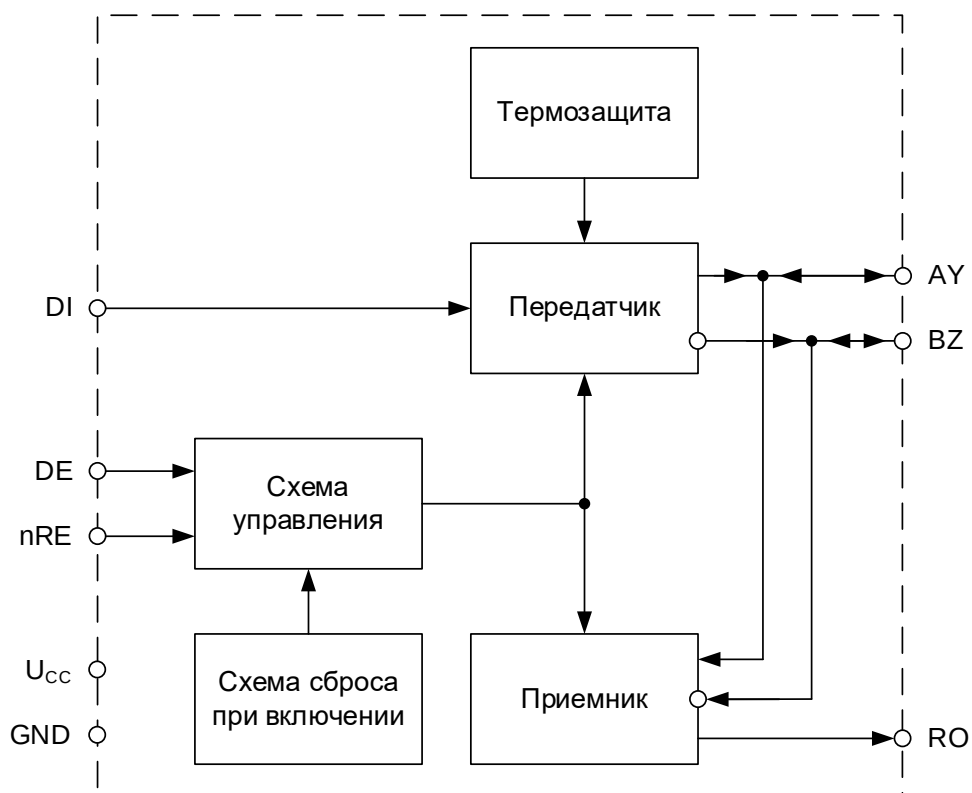
Рисунок 1 – Структурная блок-схема
