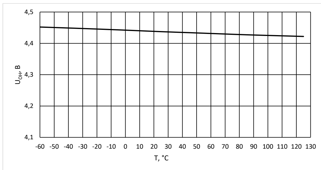
Рисунок 17 – Зависимость выходного напряжения высокого уровня приемника U_{OH} от температуры при U_{CC} = 4,5 \text{ В} , I_{OH} = -1 \text{ мА}
