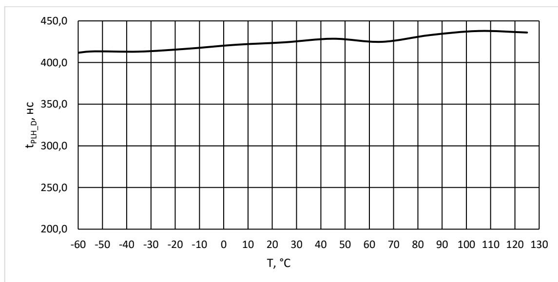
Рисунок 13 – Зависимость времени задержки распространения сигнала передатчика при включении t_{PLH\_D} от температуры при U_{CC} = 4,5 \text{ В}
