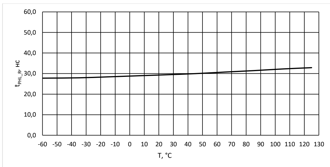
Рисунок 16 – Зависимость времени задержки распространения сигнала приемника при включении t_{PHL\_R} от температуры при U_{CC} = 4,5 \text{ В}
