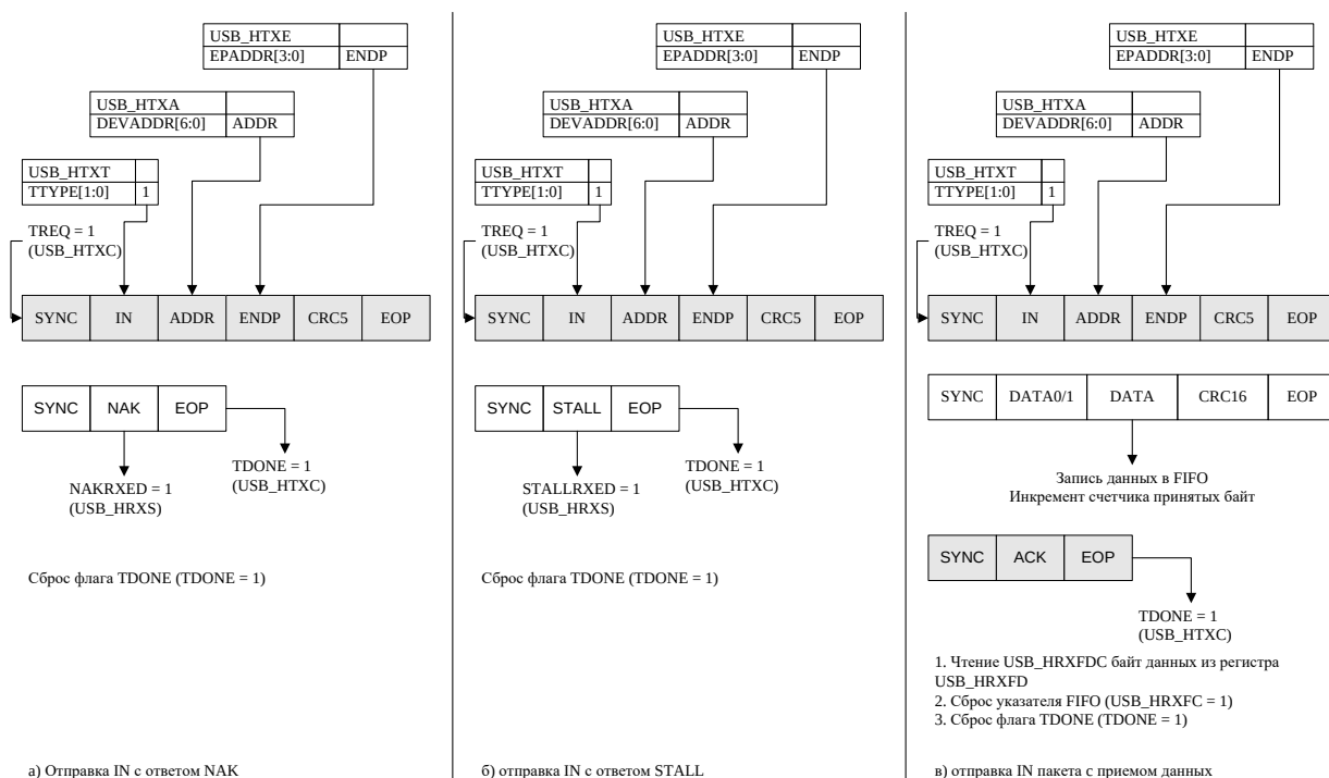
Рисунок 38 (а, б, в) – Транзакция IN (USB Host)
