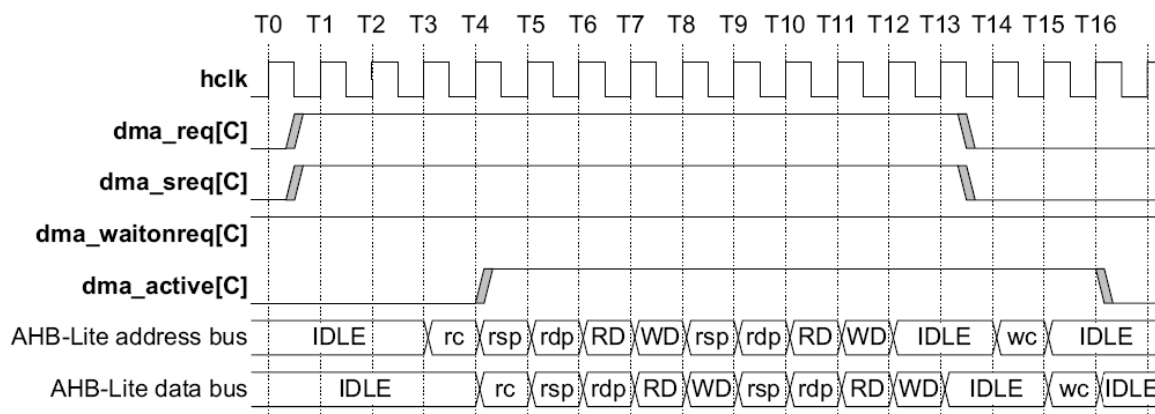
Рисунок 122 – Диаграмма работы контроллера DMA при использовании dma_waitonreq
