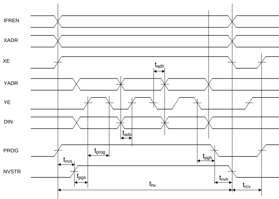
Рисунок 16 – Временная диаграмма записи памяти
