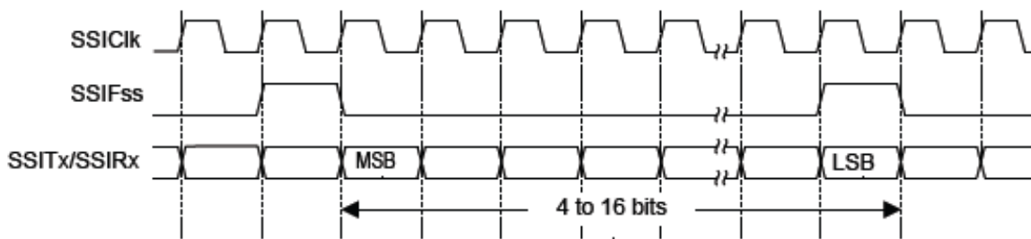
Рисунок 97 – Формат синхронного обмена протокола SSI (непрерывный обмен)
