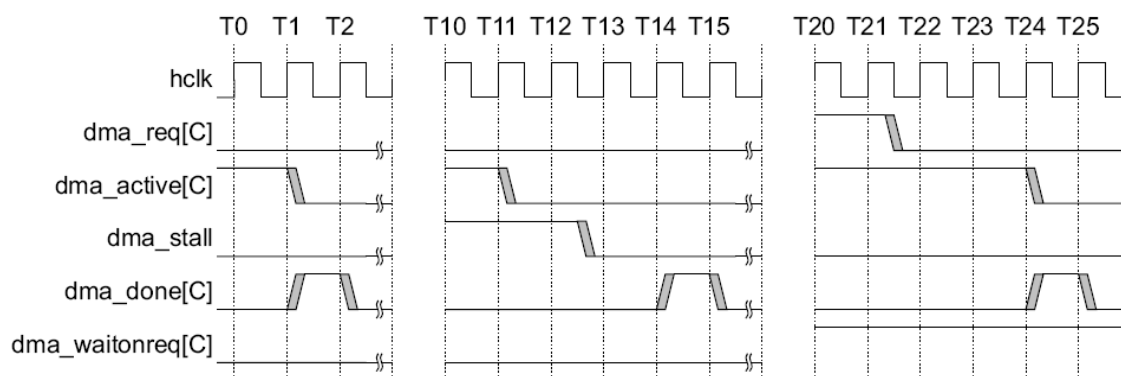
Рисунок 121 – Диаграммы функционирования dma_done
