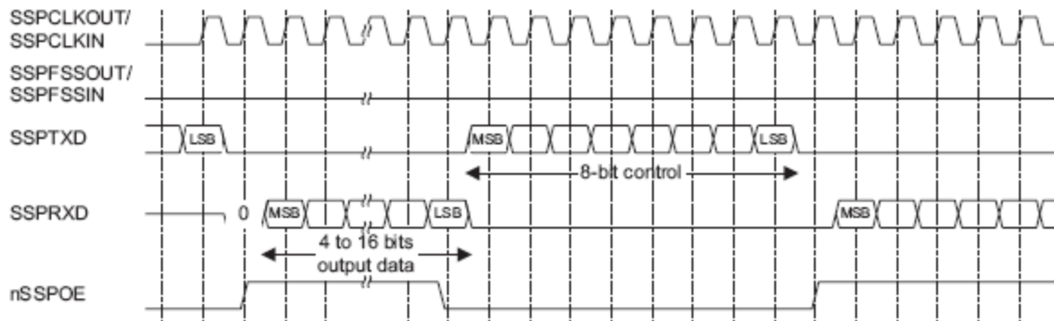
Рисунок 105 – Формат синхронного обмена протокола Microwire (непрерывный обмен)
