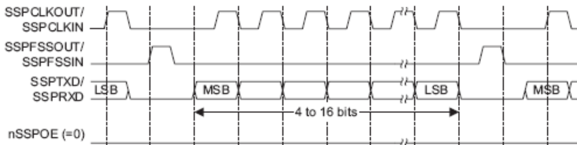
Рисунок 99 – Формат синхронного обмена протокола SPI, SPO=0, SPH=0 (непрерывный обмен)
