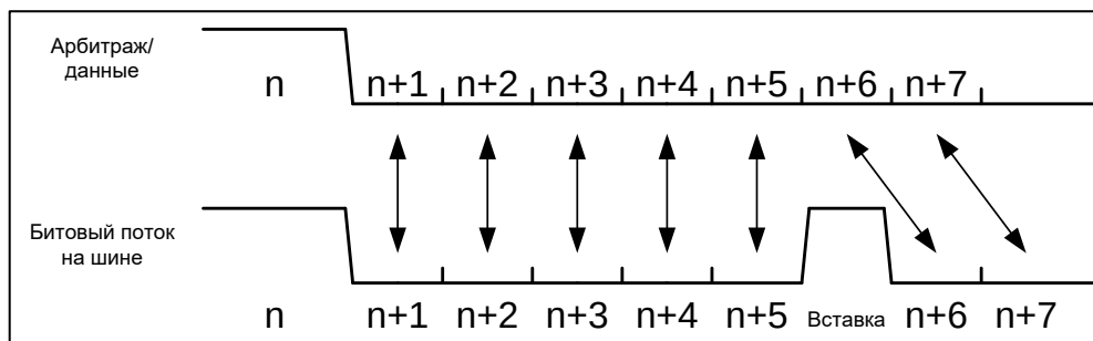
Рисунок 54 – Битстаффинг
