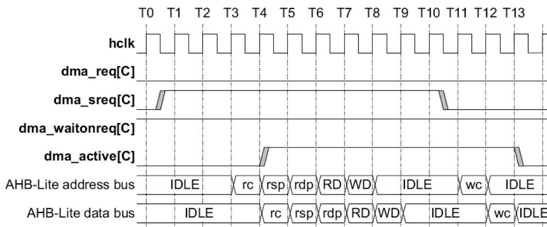
Рисунок 123 – Работа DMA при использовании dma_waitonreq совместно с dma_sreq
