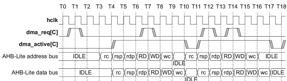
Рисунок 119 – Диаграмма работы при получении импульсного запроса
