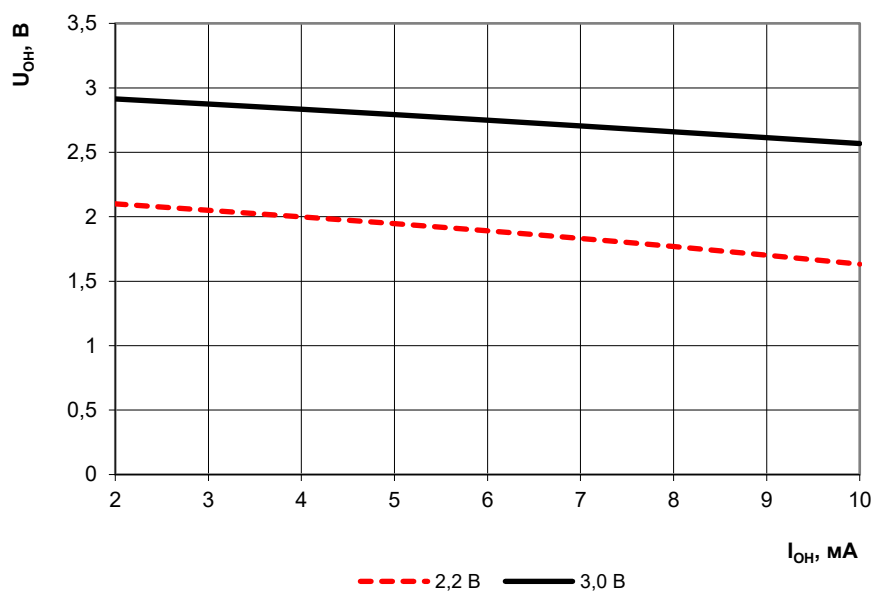
Рисунок 144 – Зависимость выходного напряжения высокого уровня от выходного тока высокого уровня при напряжении питания 2,2 и 3,0 В
