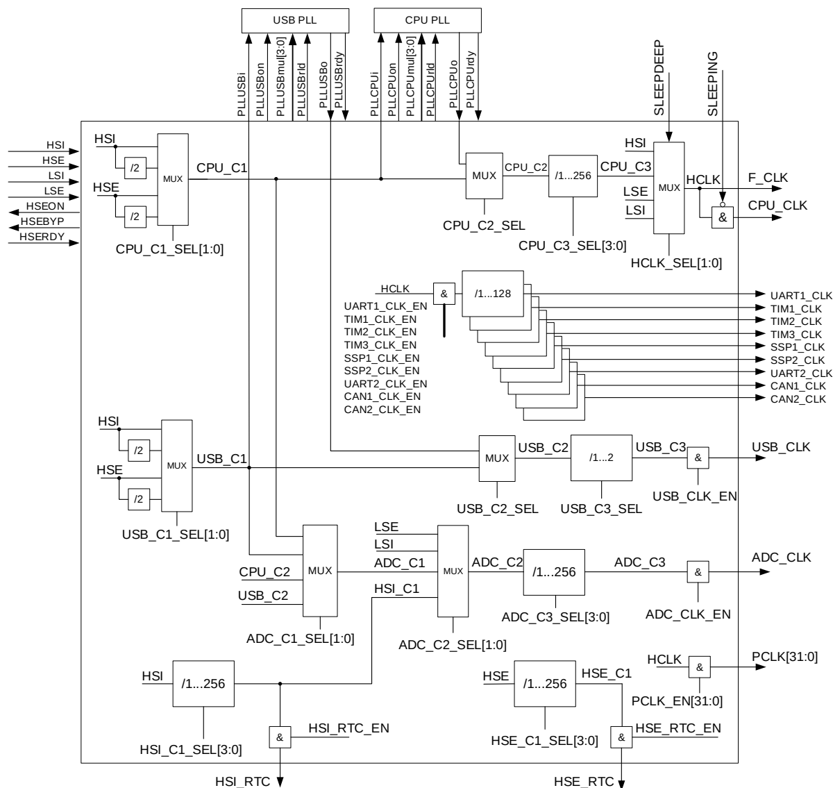
Рисунок 26 – Структурная блок-схема формирования тактовой частоты
