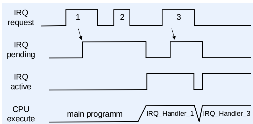
Рисунок 137 – Повторная установка запроса на прерывание в момент выполнения обработчика исключения
