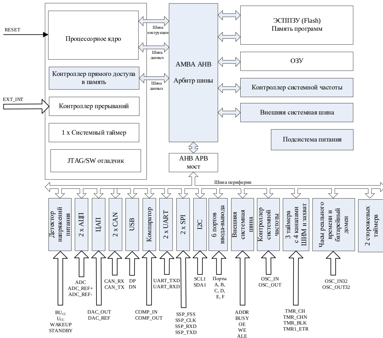
Рисунок 1 – Структурная блок-схема
