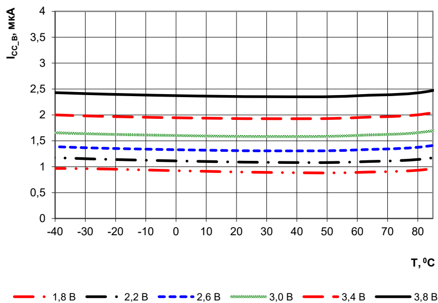
Рисунок 142 – Зависимость тока потребления батарейного домена от температуры при разном напряжении
