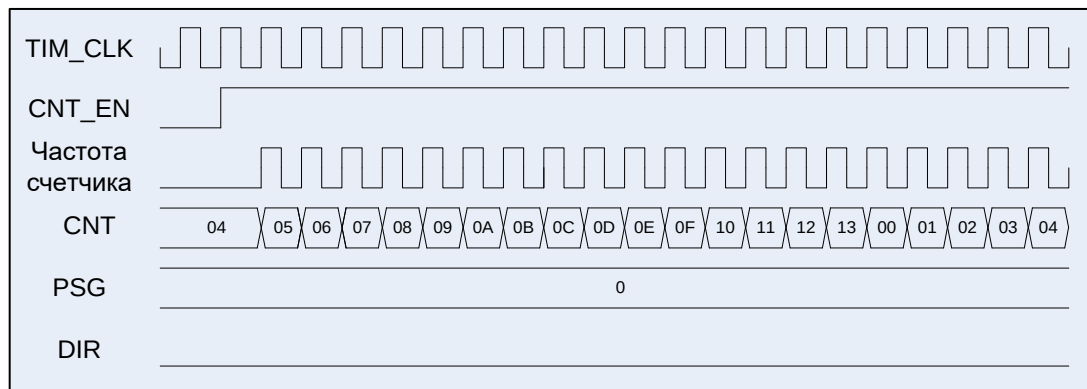
Рисунок 58 – Диаграммы работы таймера, счет прямой от 0 до 0x13, стартовое значение 0x04
