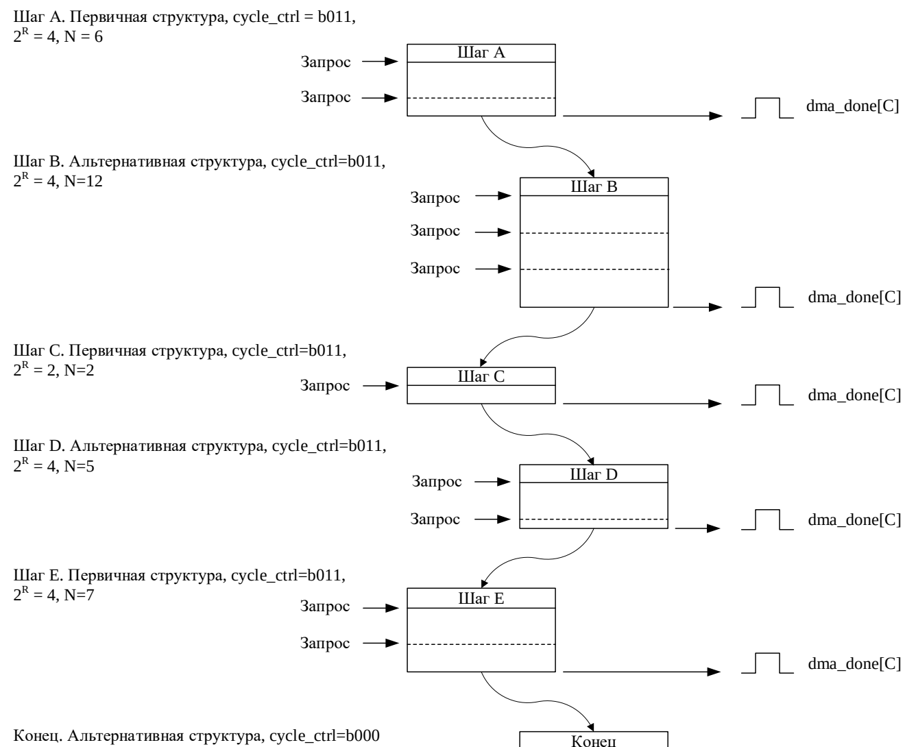
Рисунок 125 – Пример функционирования контроллера в режиме «пинг-понг»
