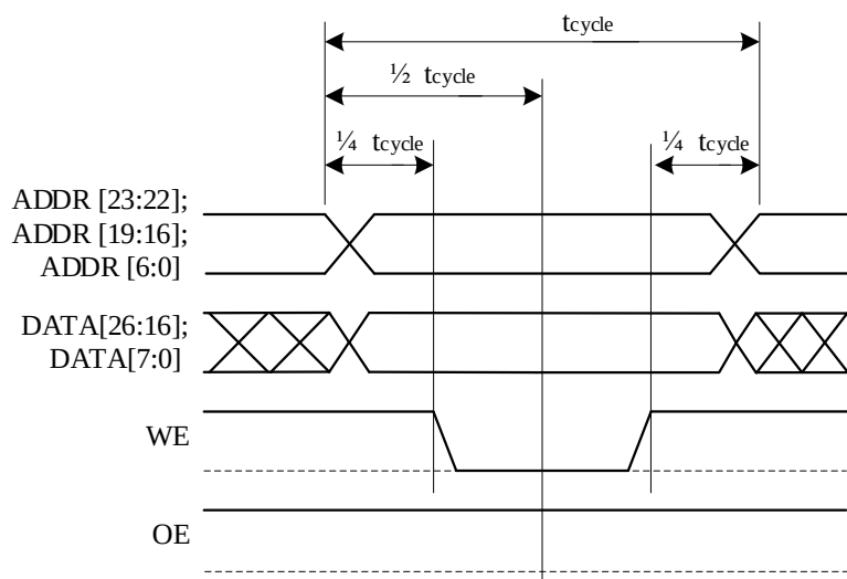
Рисунок 32 – Диаграмма записи контроллера внешней системной шины
