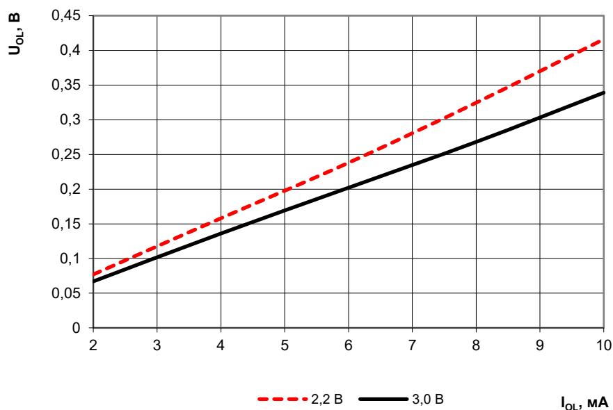
Рисунок 145 – Зависимость выходного напряжения низкого уровня от выходного тока низкого уровня при напряжении питания 2,2 и 3,0 В
