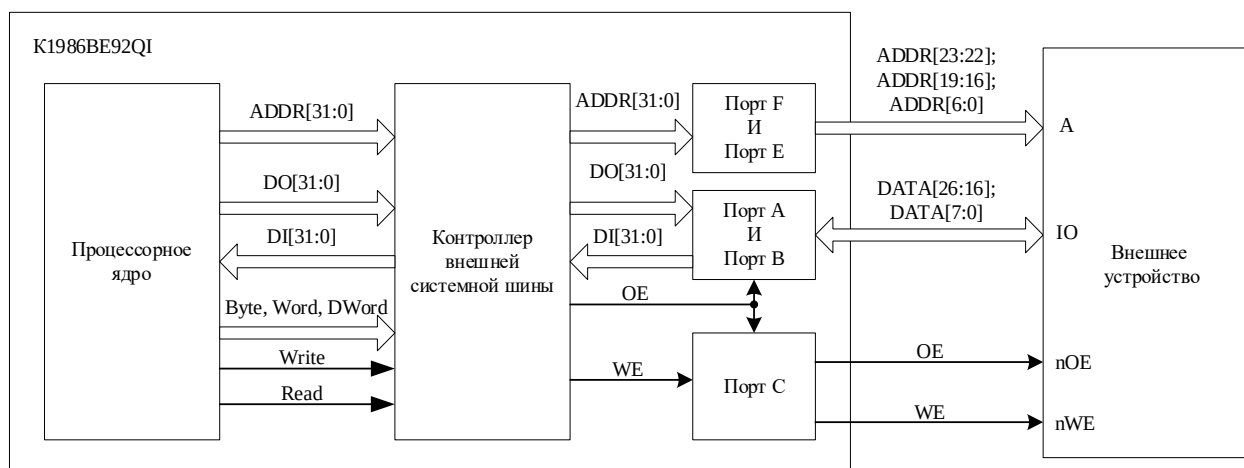
Рисунок 31 – Обмен по внешней системной шине
