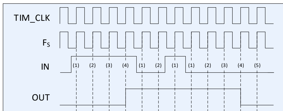
Рисунок 81 – Диаграмма работы фильтра, F_S = TIM\_CLK , N = 4
