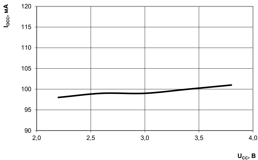
Рисунок 140 – Зависимость динамического тока потребления от напряжения питания
