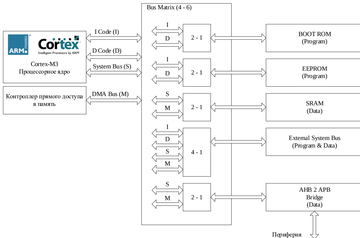
Рисунок 8 – Структурная схема организации памяти
