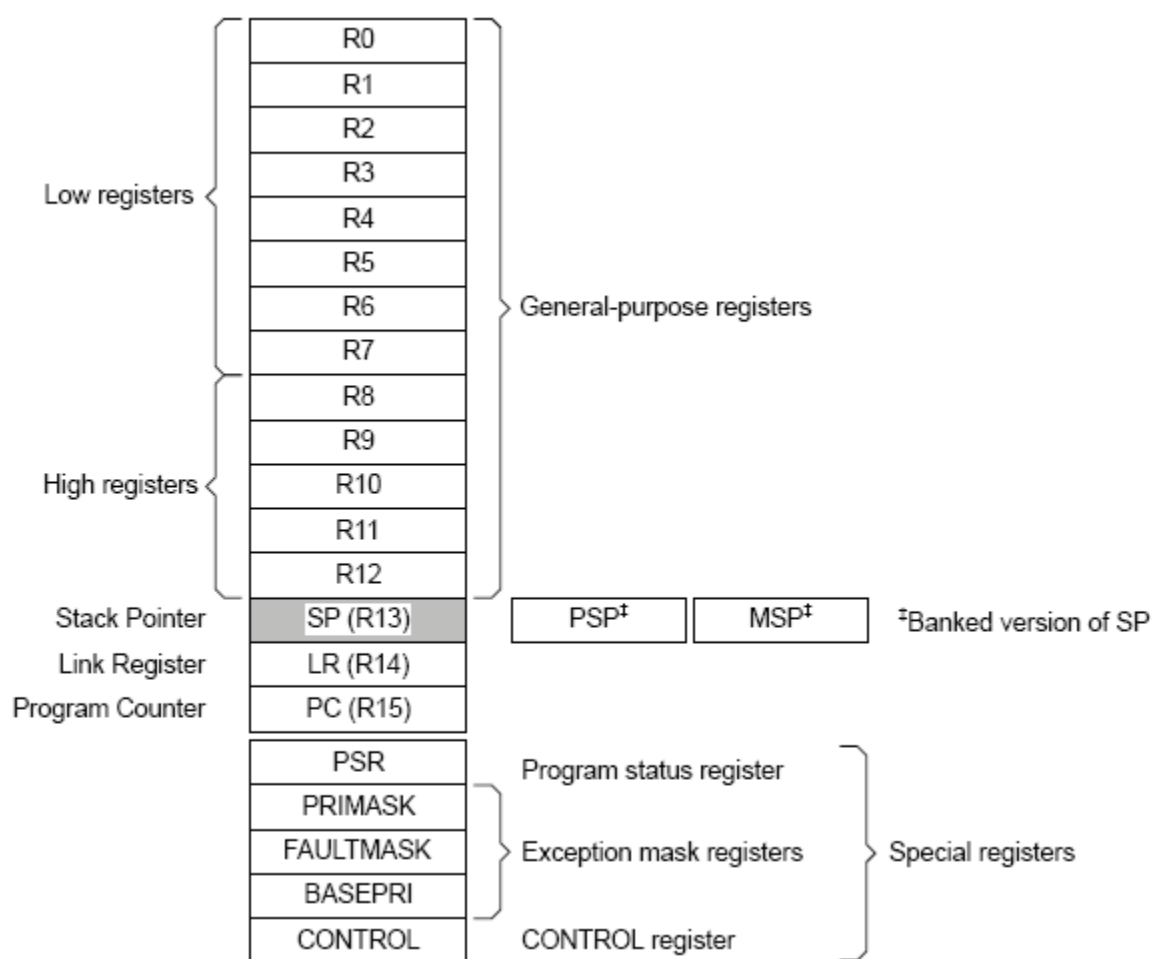
Рисунок 19 – Регистры ядра
