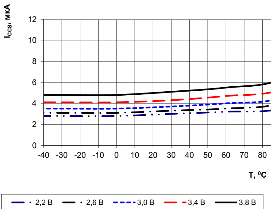
Рисунок 141 – Зависимость статического тока потребления в режиме покоя (регулятор напряжения выключен) от температуры при разном напряжении
