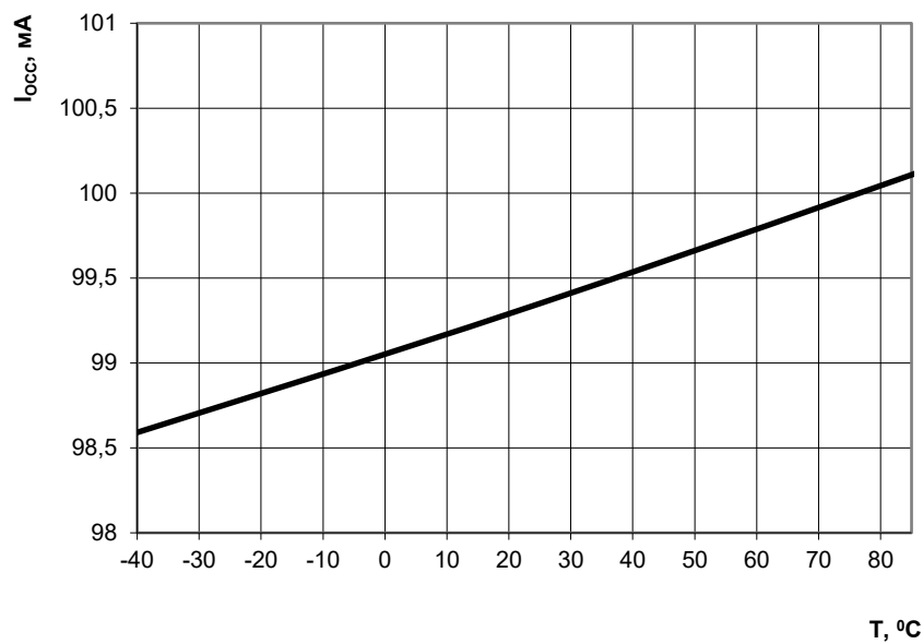
Рисунок 139 – Зависимость динамического тока потребления от температуры при: f_C = 80 МГц
