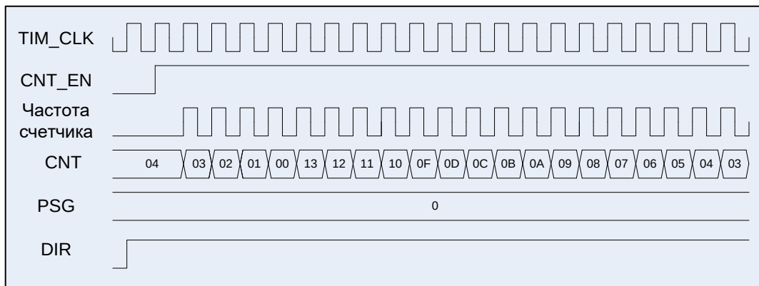
Рисунок 59 – Диаграммы работы таймера, счет обратный от 0x13 до 0, стартовое значение 0x04
