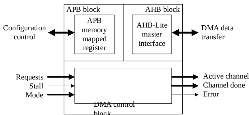
Рисунок 118 – Структурная схема контроллера
