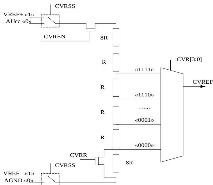
Рисунок 91 – Структура блока формирования CVREF
