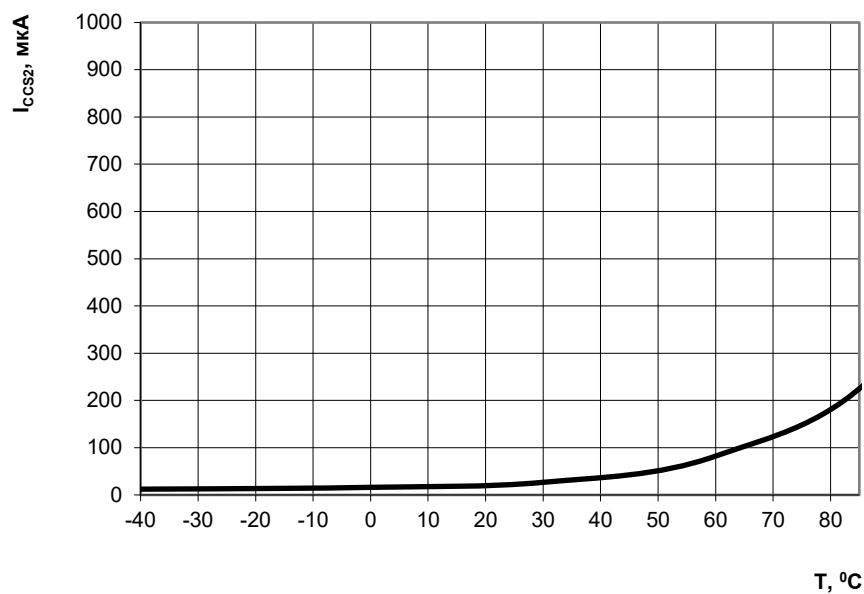
Рисунок 143 – Зависимость статического тока потребления в режиме покоя (регулятор напряжения включен) от температуры
