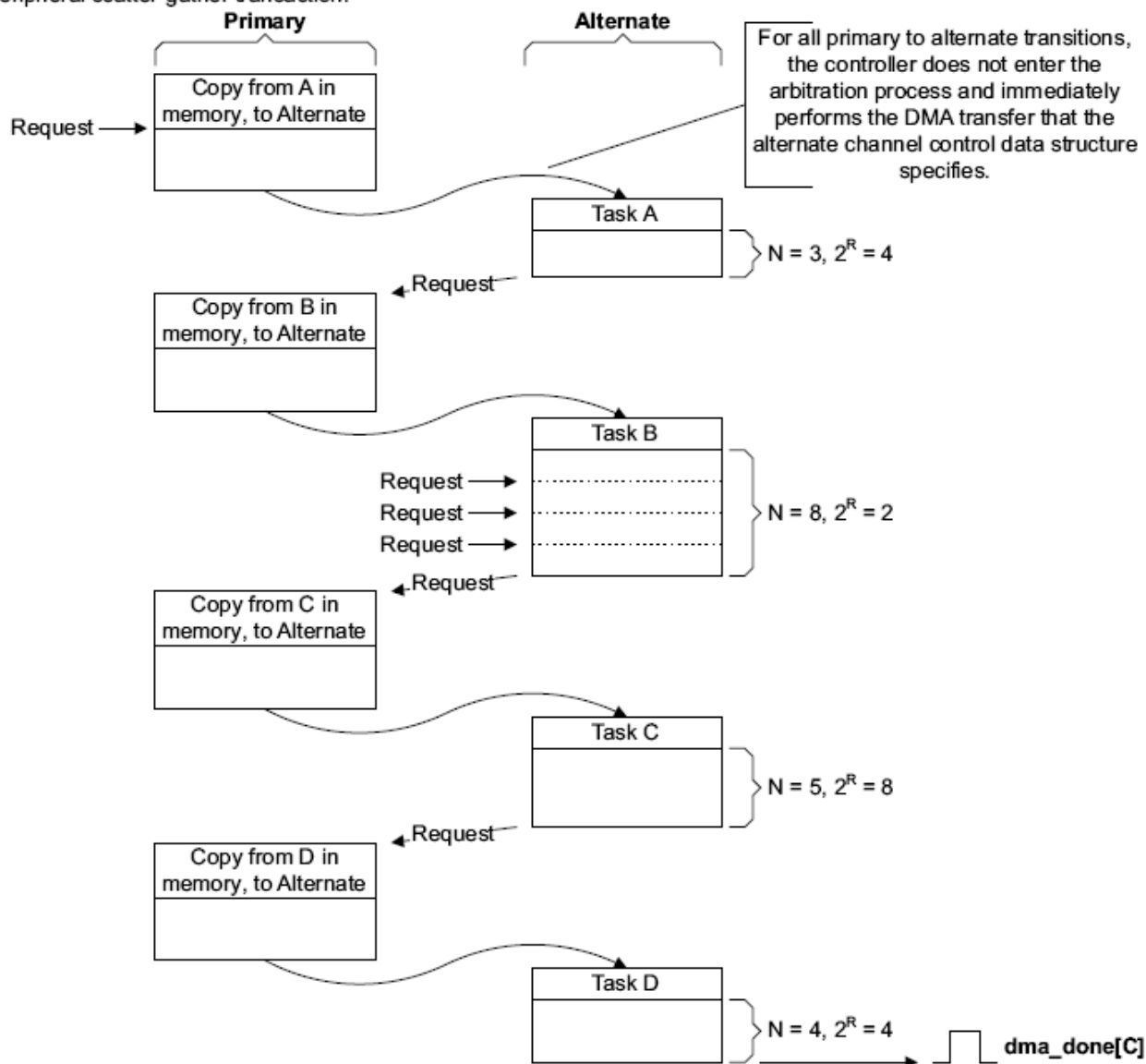
Рисунок 127 – Пример работы DMA в режиме с «Исполнением с изменением конфигурации»
