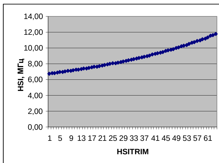
Рисунок 29 – Зависимость частоты HSI от значения HSITRIM
