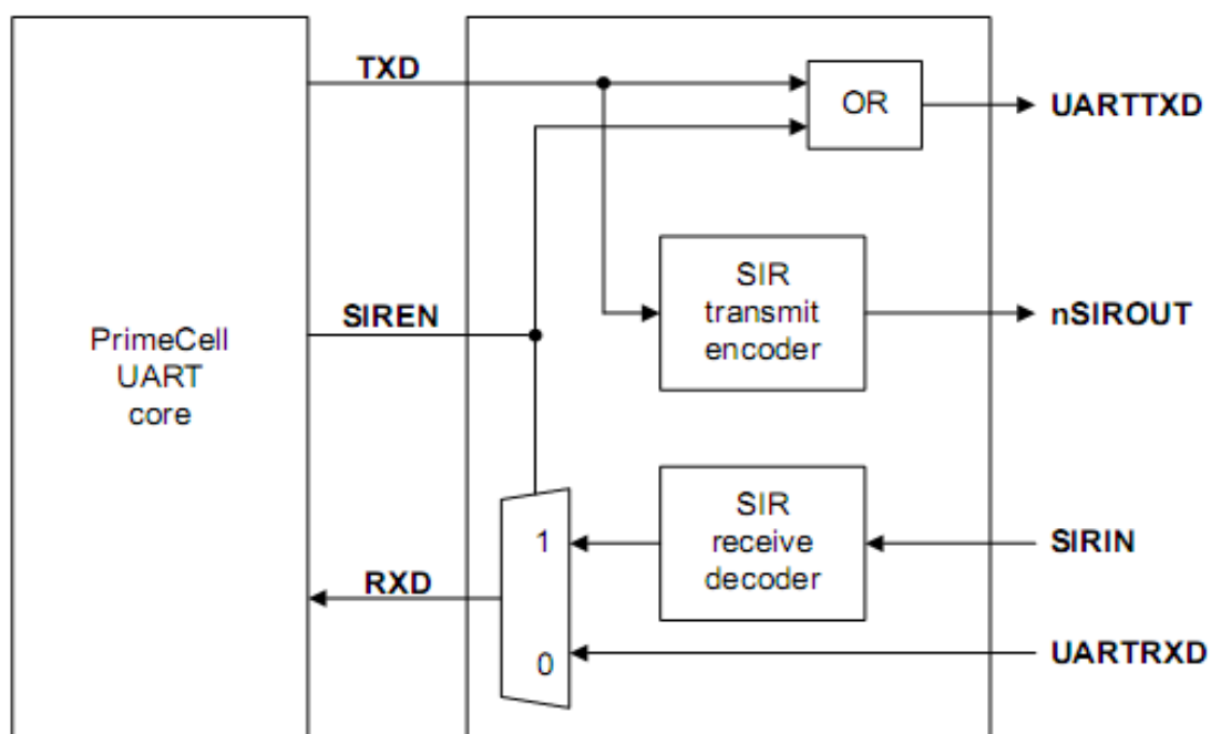
Рисунок 112 – Структурная схема кодека IrDA
