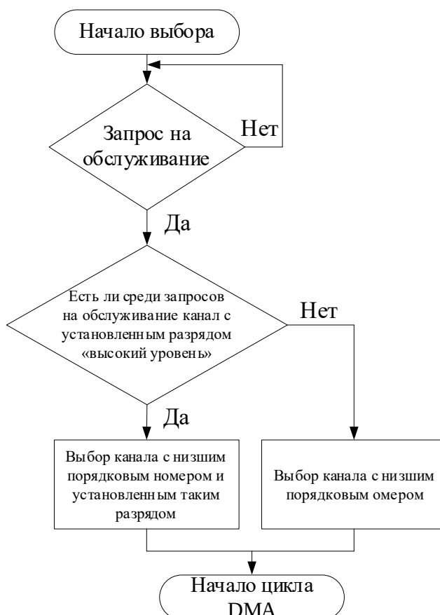
Рисунок 124 – Алгоритм выбора следующего канала для обслуживания
