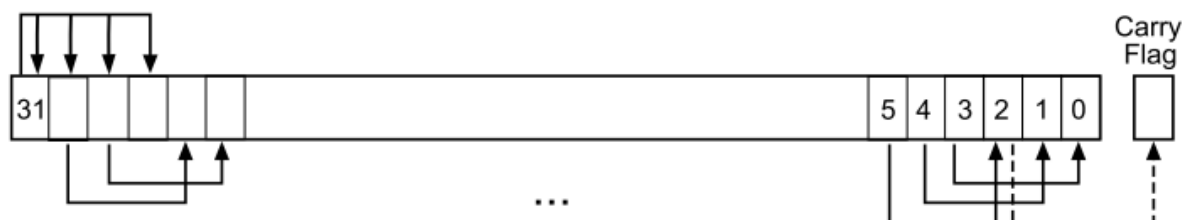
Рисунок 20 – Инструкция ASR # 3
