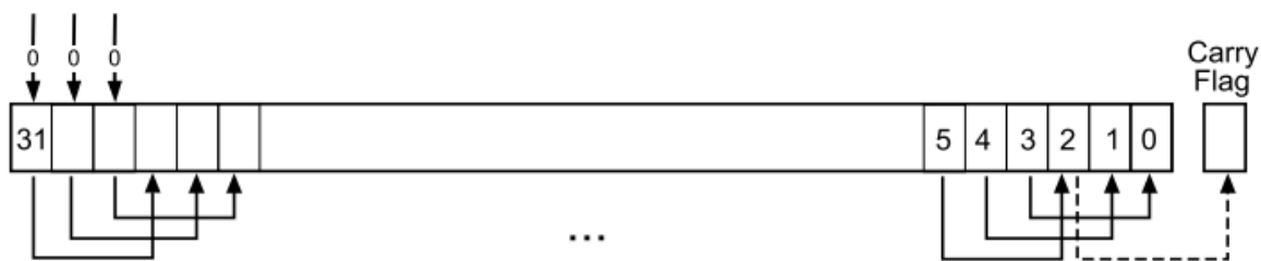
Рисунок 21 – Инструкция LSR # 3
