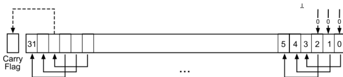
Рисунок 22 – Инструкция LSL # 3
