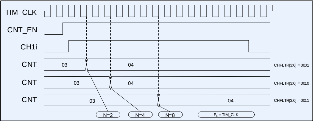
Рисунок 76 – Диаграмма внешнего тактирования с разными вариантами фильтра
