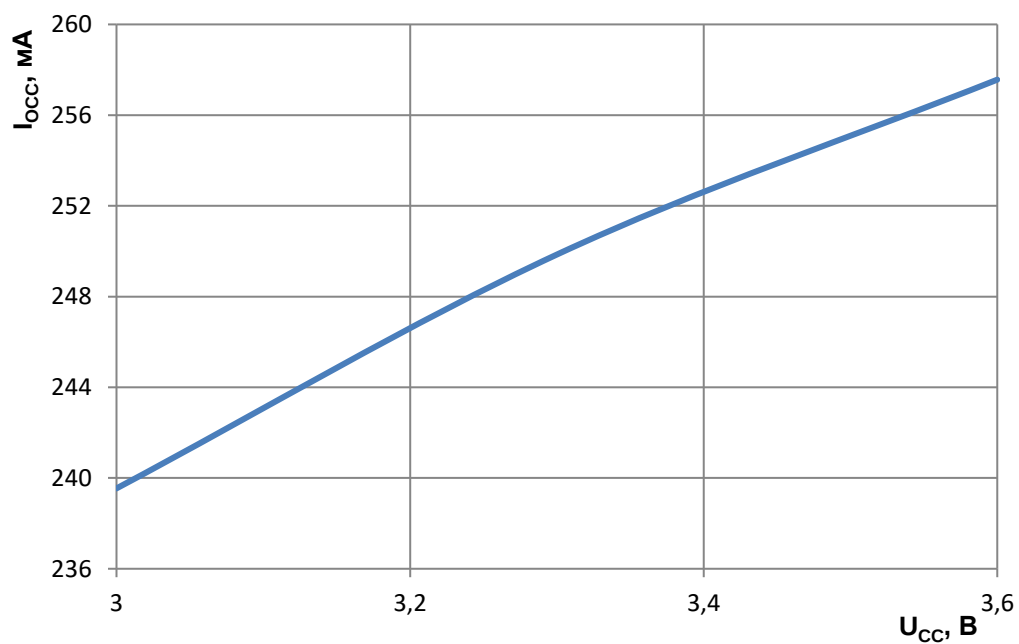
Рисунок 145 – Зависимость динамического тока потребления от напряжения питания
