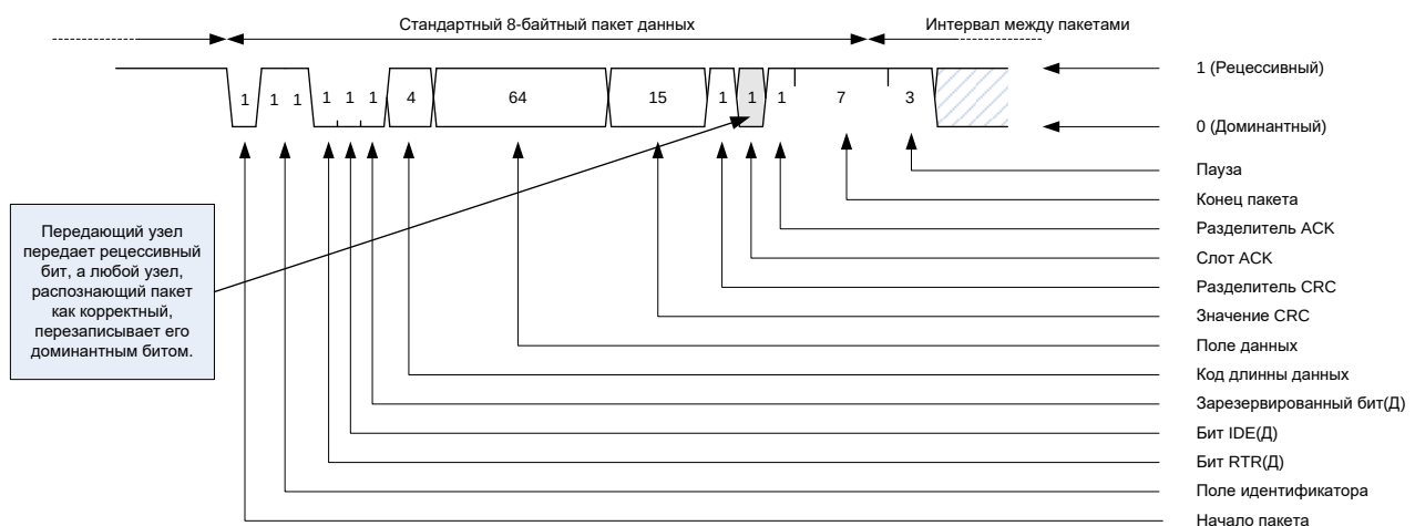
Рисунок 50 – Контроль подтверждения
