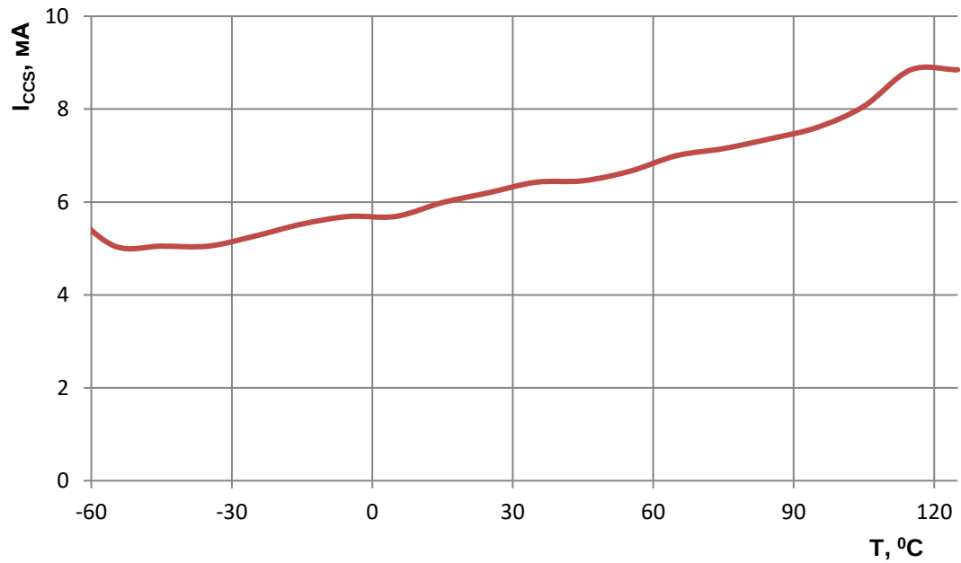
Рисунок 146 – Зависимость статического тока потребления в режиме покоя (регулятор напряжения выключен) от температуры при напряжении U_{CC}=3.6V
