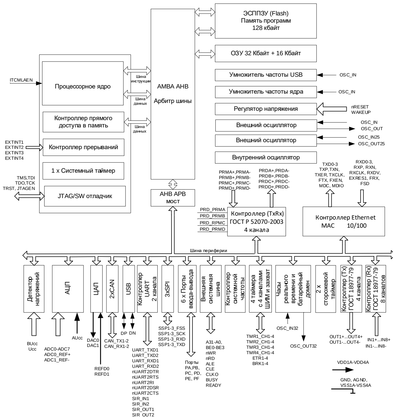
Рисунок 1 – Структурная блок-схема микросхемы
