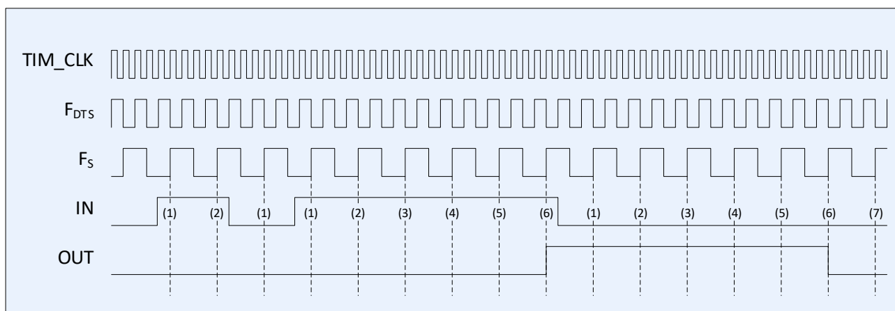
Рисунок 88 – Диаграмма работы фильтра, F_S = F_{DTS}/2 , N = 6
