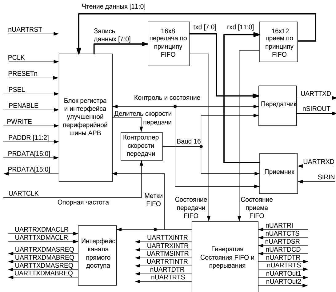
Рисунок 114 – Блок-схема универсального асинхронного приемопередатчика (UART)
