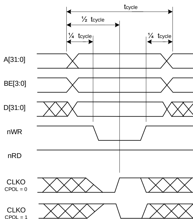
Рисунок 28 – Диаграмма записи
