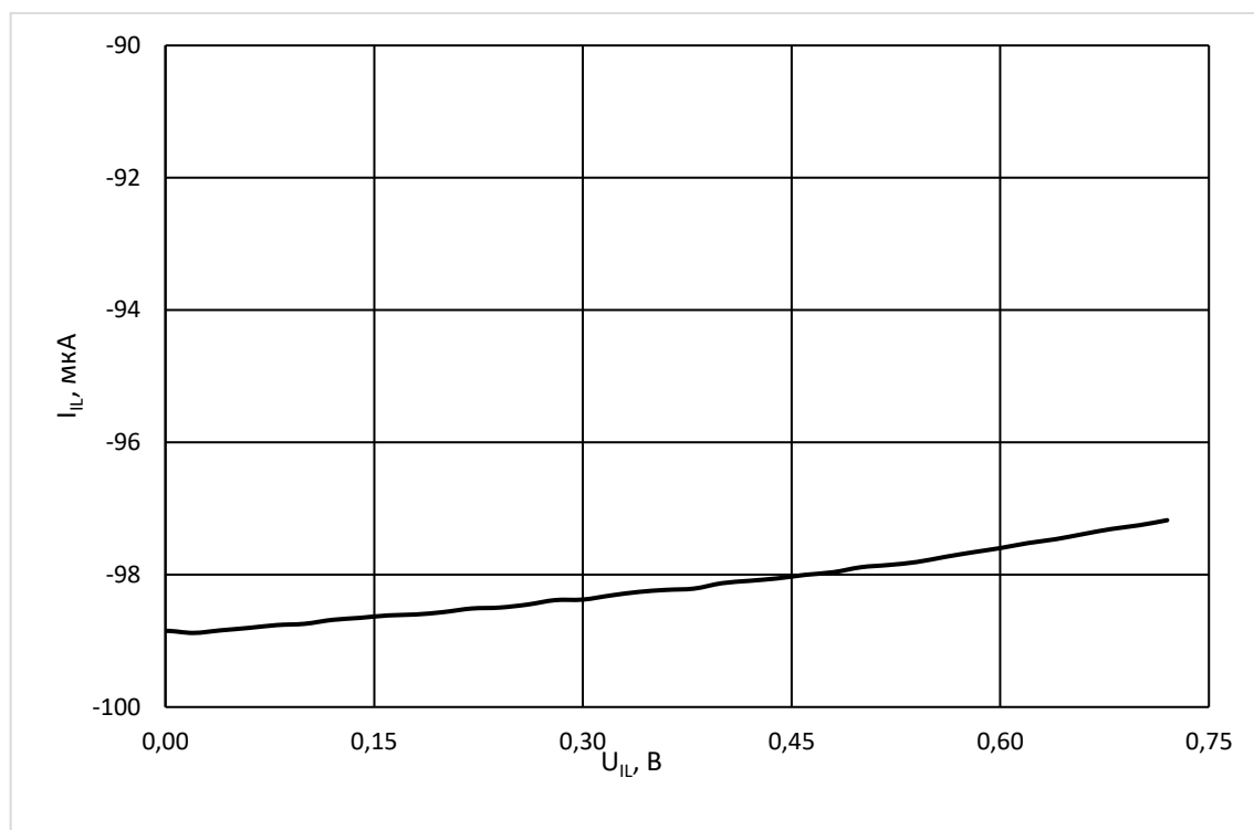
Рисунок 49 – Зависимость входного тока низкого уровня I_{IL} от входного напряжения низкого уровня U_{IL} при U_{CC} = 3,6 В, T = 25 °С, U_{IH} = U_{CC}
