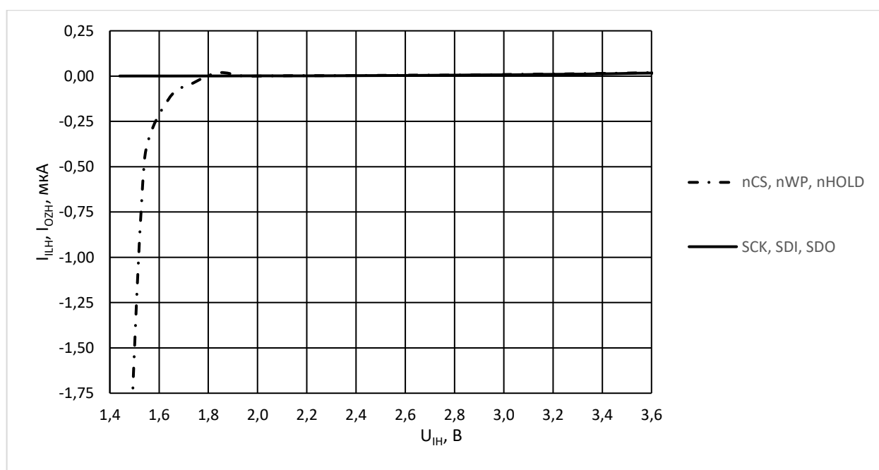
Рисунок 46 – Зависимость тока утечки высокого уровня на входе I_{IH} , выходного тока высокого уровня в состоянии «Выключено» I_{OZH} от входного напряжения высокого уровня U_{IH} при U_{CC} = 1,8 В, U_{IL} = 0 В, T = 25 °С
