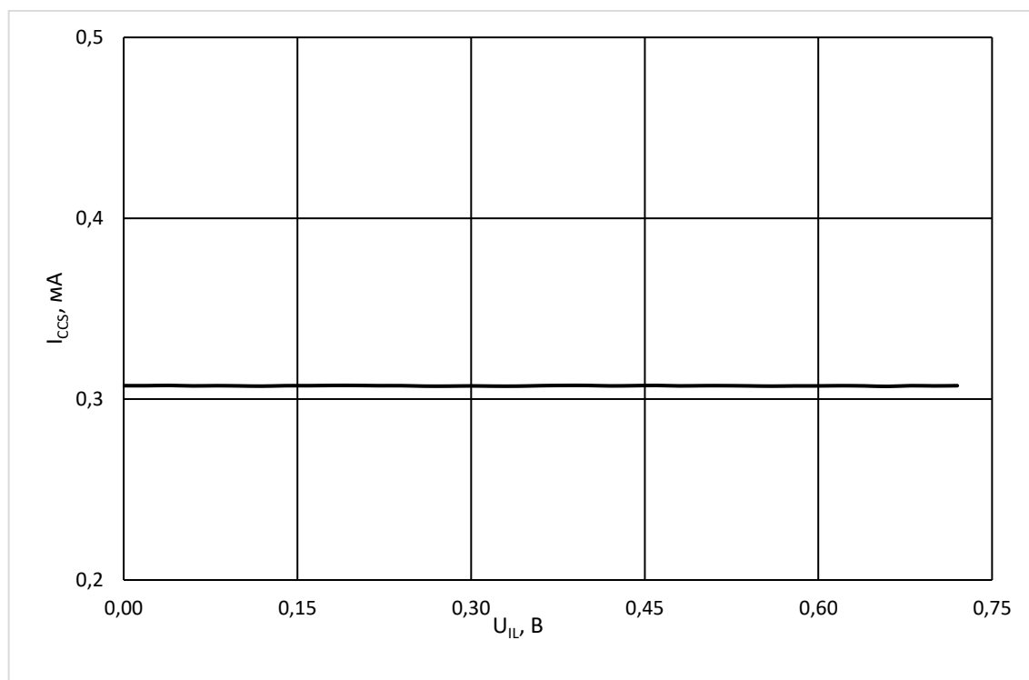
Рисунок 53 – Зависимость тока потребления в режиме хранения I_{CCS} от входного напряжения низкого уровня U_{IL} при U_{CC} = 3,6 В, U_{IH} = U_{CC} , U_{nCE} = U_{CC} , U_{nWP} = U_{nHOLD} = Z , f_{C(SCK)} = 0 МГц, T = 25 °C
