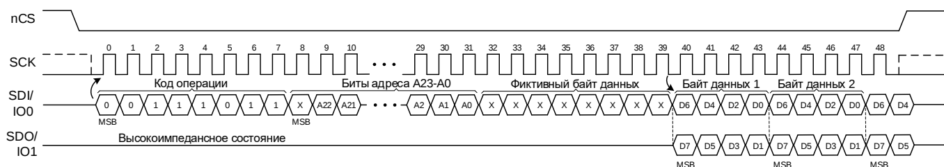
Рисунок 7 – Операция чтения с кодом 3Bh
