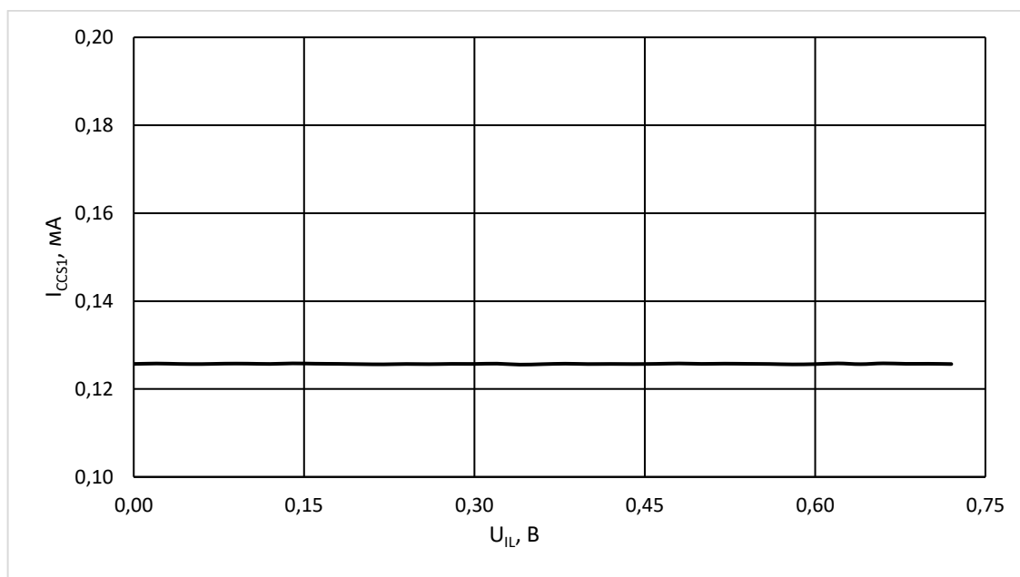
Рисунок 57 – Зависимость тока в режиме пониженного энергопотребления I_{CCS1} от входного напряжения низкого уровня U_{IL} при U_{CC} = 3,6 В, U_{IH} = U_{CC} , U_{nCE} = U_{CC} , U_{nWP} = U_{nHOLD} = Z , f_{C(SCK)} = 0 МГц, T = 25 °С
