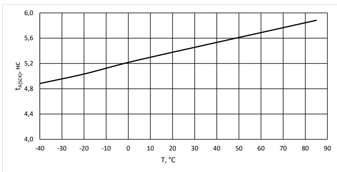
Рисунок 62 – Зависимость времени выборки данных по спаду сигнала SCK t_{A(SCK)} от температуры T при U_{CC} = 1,8\text{ В} , f_{C(SCK)} = 25\text{ МГц} , U_{IL} = 0\text{ В} , U_{IH} = U_{CC}
