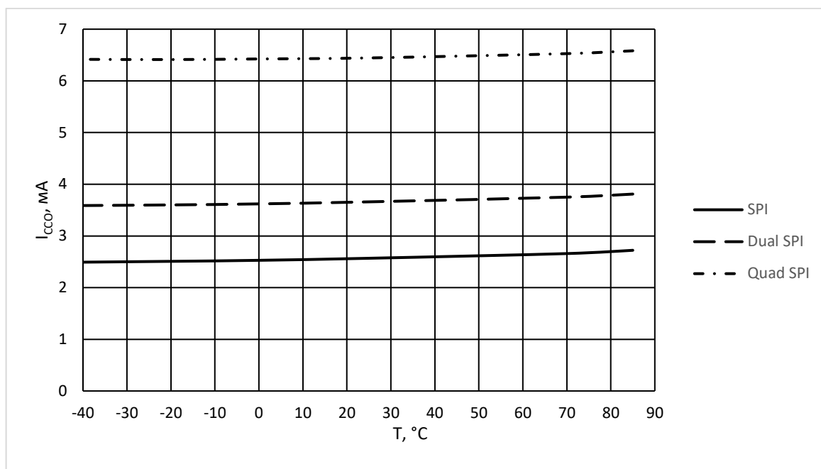
Рисунок 59 – Зависимость динамического тока потребления I_{CCO} при чтении в режимах SPI, Dual SPI и Quad SPI от температуры T при U_{CC} = 3,6 В, f_{C(SCK)} = 100 МГц, U_{IL} = 0 В, U_{IH} = U_{CC}
