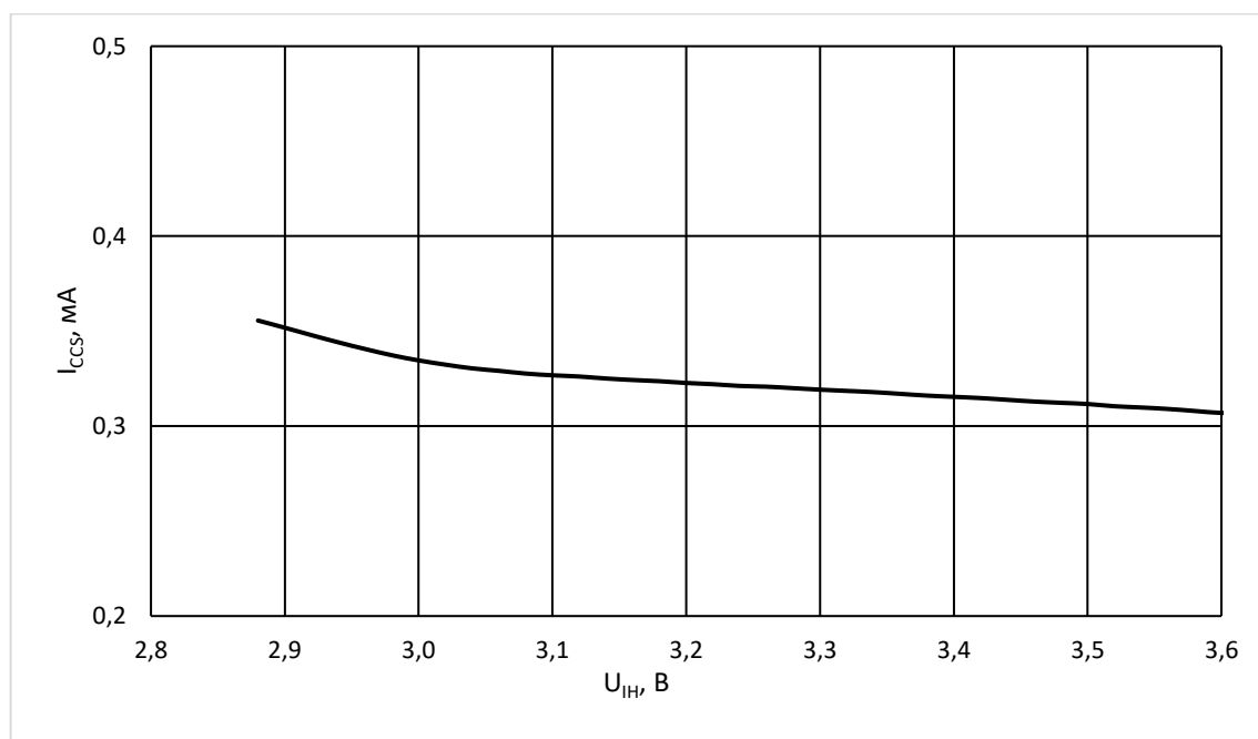
Рисунок 52 – Зависимость тока потребления в режиме хранения I_{CCS} от входного напряжения высокого уровня U_{IH} при U_{CC} = 3,6 В, U_{IL} = 0 В, U_{nCE} = U_{IH} , U_{nWP} = U_{nHOLD} = Z , f_{C(SCK)} = 0 МГц, T = 25 °C
