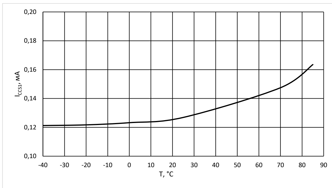
Рисунок 55 – Зависимость тока в режиме пониженного энергопотребления I_{CCS1} от температуры T при U_{CC} = 3,6 В, U_{IL} = 0 В, U_{IH} = U_{CC} , U_{nCS} = U_{CC} , U_{nWP} = U_{nHOLD} = Z , f_{C(SCK)} = 0 МГц
