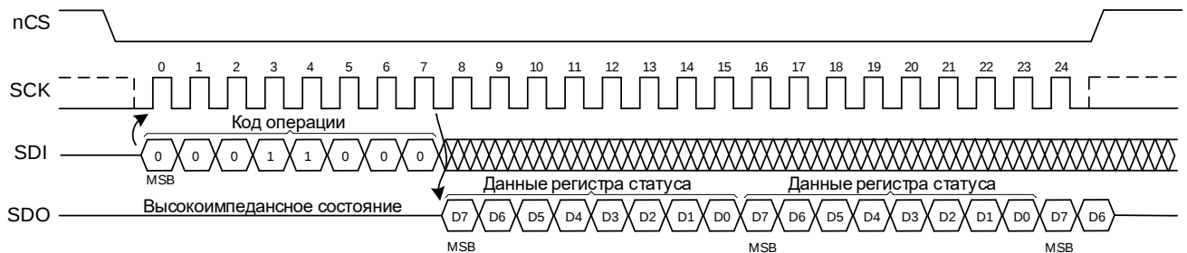
Рисунок 24 – Операция чтения регистра статуса помехоустойчивого кодирования
