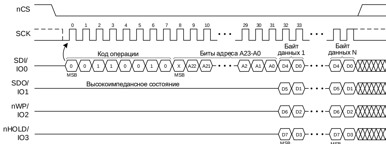
Рисунок 11 – Операция программирования с кодом 32h
