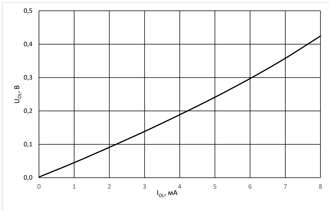
Рисунок 41 – Зависимость выходного напряжения низкого уровня U_{OL} от тока нагрузки I_{OL} при U_{CC} = 1,8 В, T = 25 °С
