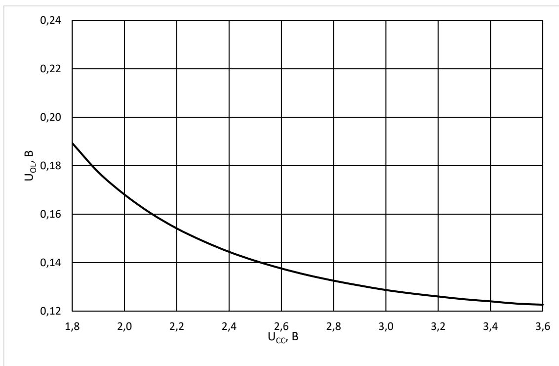
Рисунок 39 – Зависимость выходного напряжения низкого уровня U_{OL} от напряжения питания U_{CC} при T = 25\text{ }^{\circ}\text{C} и I_{OL} = 4\text{ мА}
