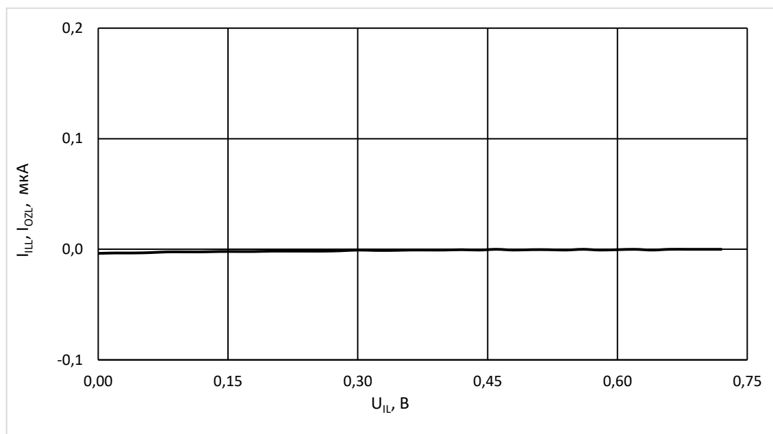
Рисунок 45 – Зависимость тока утечки низкого уровня на входе I_{IL} , выходного тока низкого уровня в состоянии «Выключено» I_{OZL} от входного напряжения низкого уровня U_{IL} при U_{CC} = 3,6 В, T = 25 °С, U_{IH} = U_{CC}
