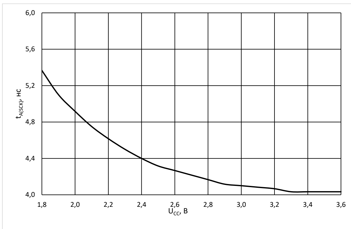
Рисунок 61 – Зависимость времени выборки данных по спаду сигнала SCK t_{A(SCK)} от напряжения питания U_{CC} при T = 25\text{ }^{\circ}\text{C} , f_{C(SCK)} = 25\text{ МГц} , U_{IL} = 0\text{ В} , U_{IH} = U_{CC}
