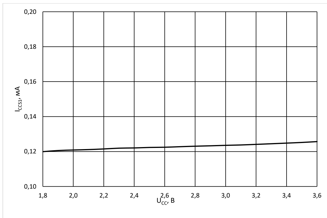
Рисунок 54 – Зависимость тока в режиме пониженного энергопотребления I_{CCS1} от напряжения питания U_{CC} при T = 25 °C, U_{IL} = 0 В, U_{IH} = U_{CC} , U_{nCS} = U_{CC} , U_{nWP} = U_{nHOLD} = Z , f_{C(SCK)} = 0 МГц
