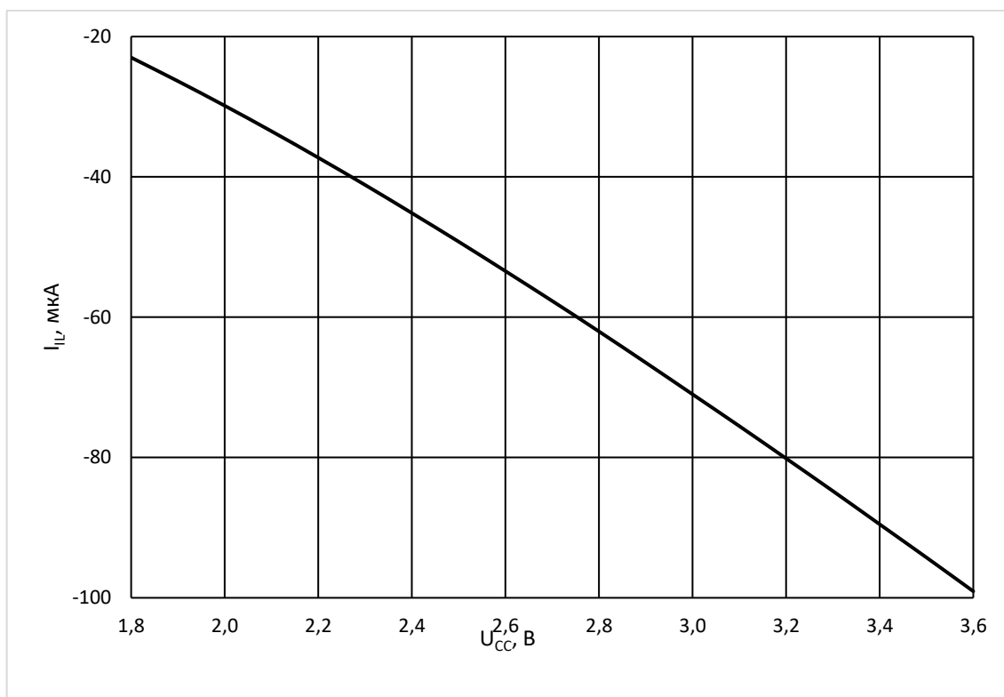
Рисунок 47 – Зависимость входного тока низкого уровня I_{IL} от напряжения питания U_{CC} при T = 25\text{ °C} , U_{IL} = 0\text{ В} , U_{IH} = U_{CC}
