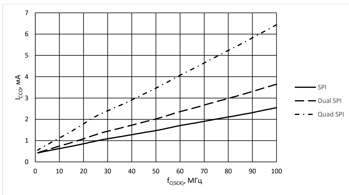
Рисунок 60 – Зависимость динамического тока потребления I_{CCO} при чтении в режимах SPI, Dual SPI и Quad SPI от частоты тактового сигнала SPI интерфейса f_{C(SCK)} при U_{CC} = 3,6 В, U_{IL} = 0 В, U_{IH} = U_{CC} и T = 25 °C
