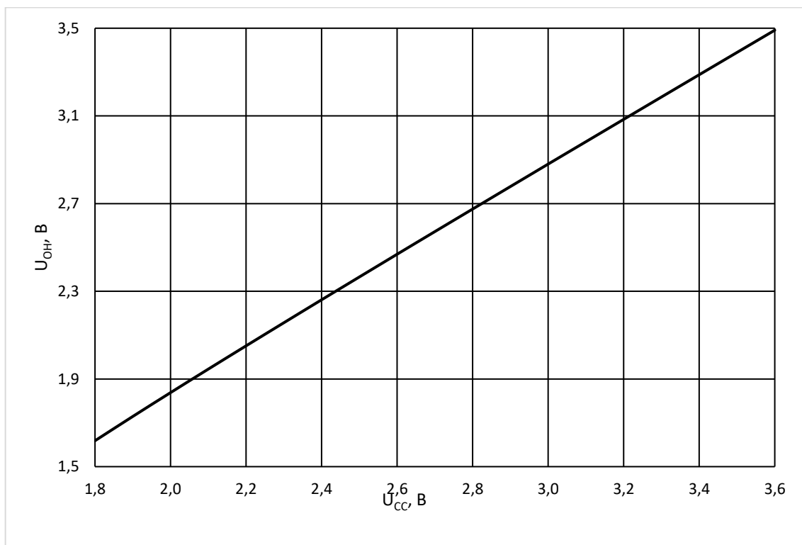
Рисунок 42 – Зависимость выходного напряжения высокого уровня U_{OH} от напряжения питания U_{CC} при T = 25 °С и I_{OH} = -4 мА
