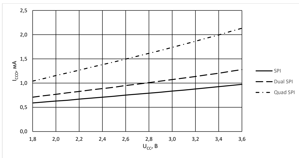
Рисунок 58 – Зависимость динамического тока потребления I_{CCO} при чтении в режимах SPI, Dual SPI и Quad SPI от напряжения питания U_{CC} при T = 25 °С, U_{IL} = 0 В, U_{IH} = U_{CC} , f_{C(SCK)} = 25 МГц
