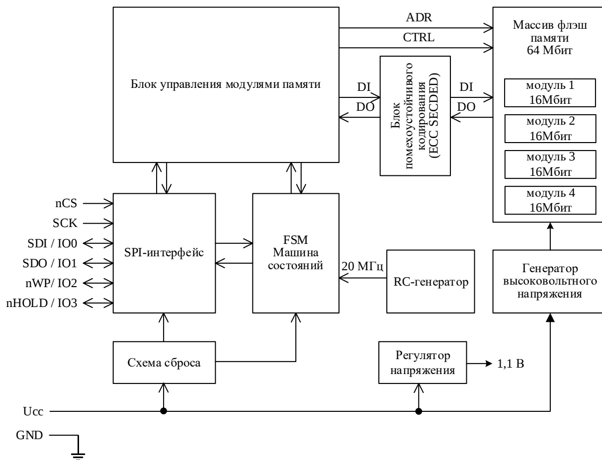
Рисунок 1 – Структурная блок-схема
