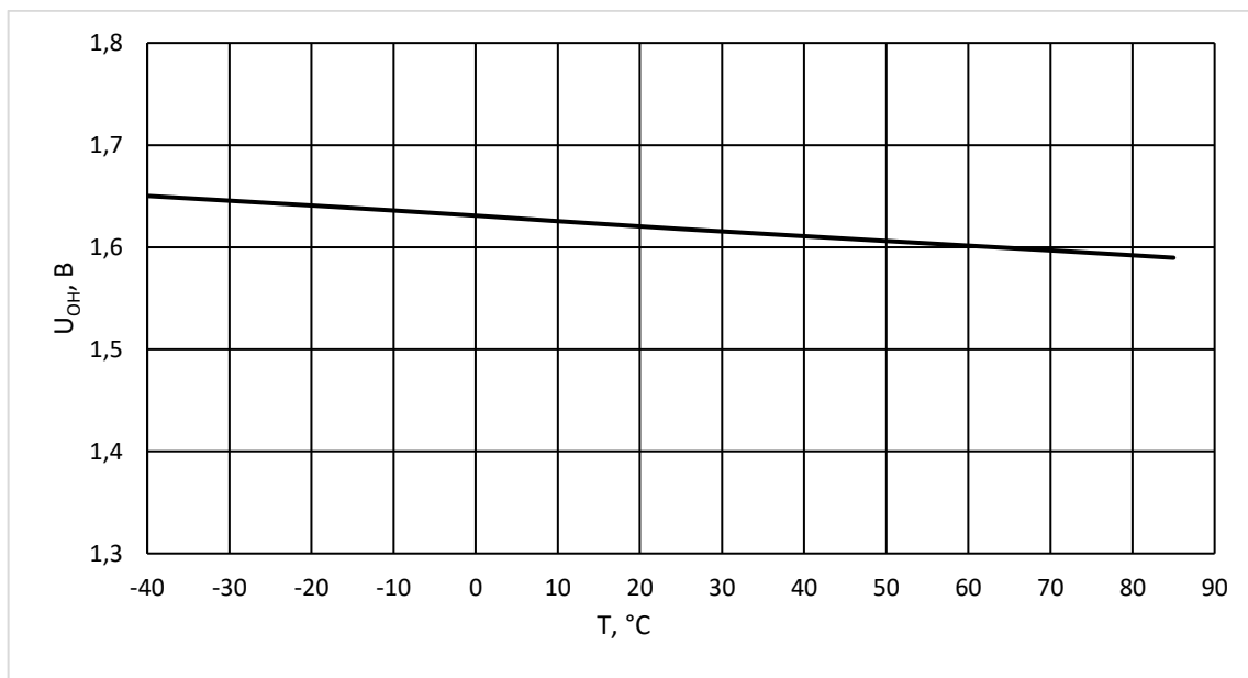
Рисунок 43 – Зависимость выходного напряжения высокого уровня U_{OH} от температуры T при U_{CC} = 1,8 В и I_{OH} = -4 мА
