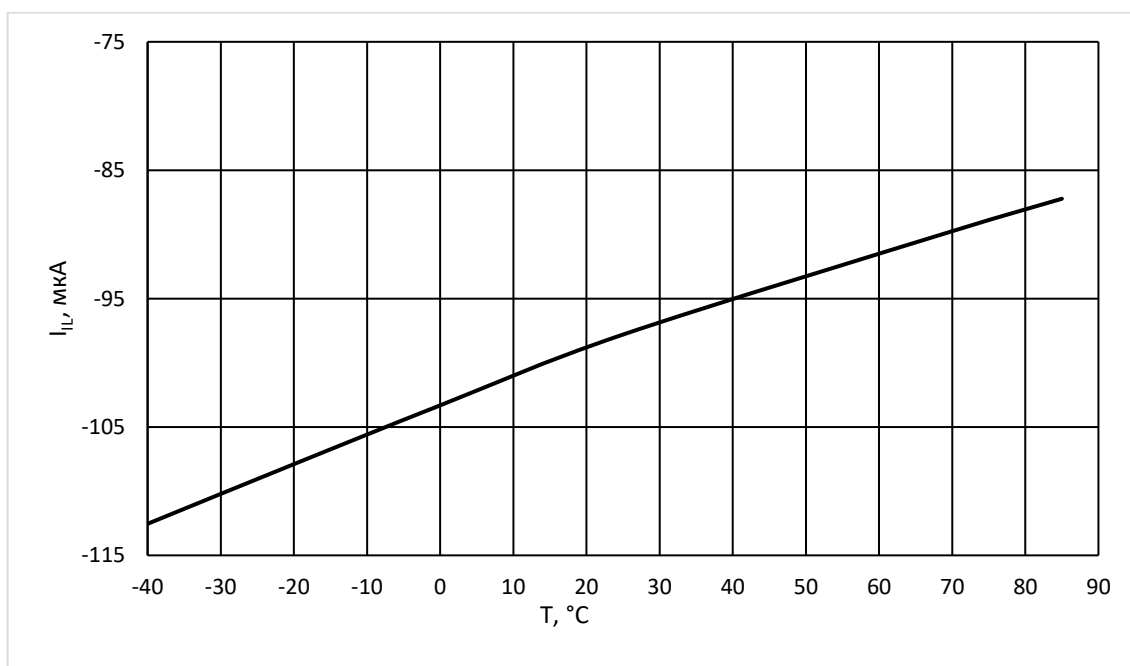
Рисунок 48 – Зависимость входного тока низкого уровня I_{IL} от температуры T при U_{CC} = 3,6\text{ В} , U_{IL} = 0\text{ В} , U_{IH} = U_{CC}
