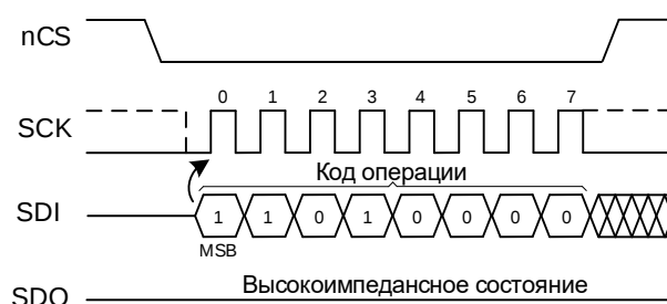
Рисунок 16 – Операция возобновления программирования/стирания
