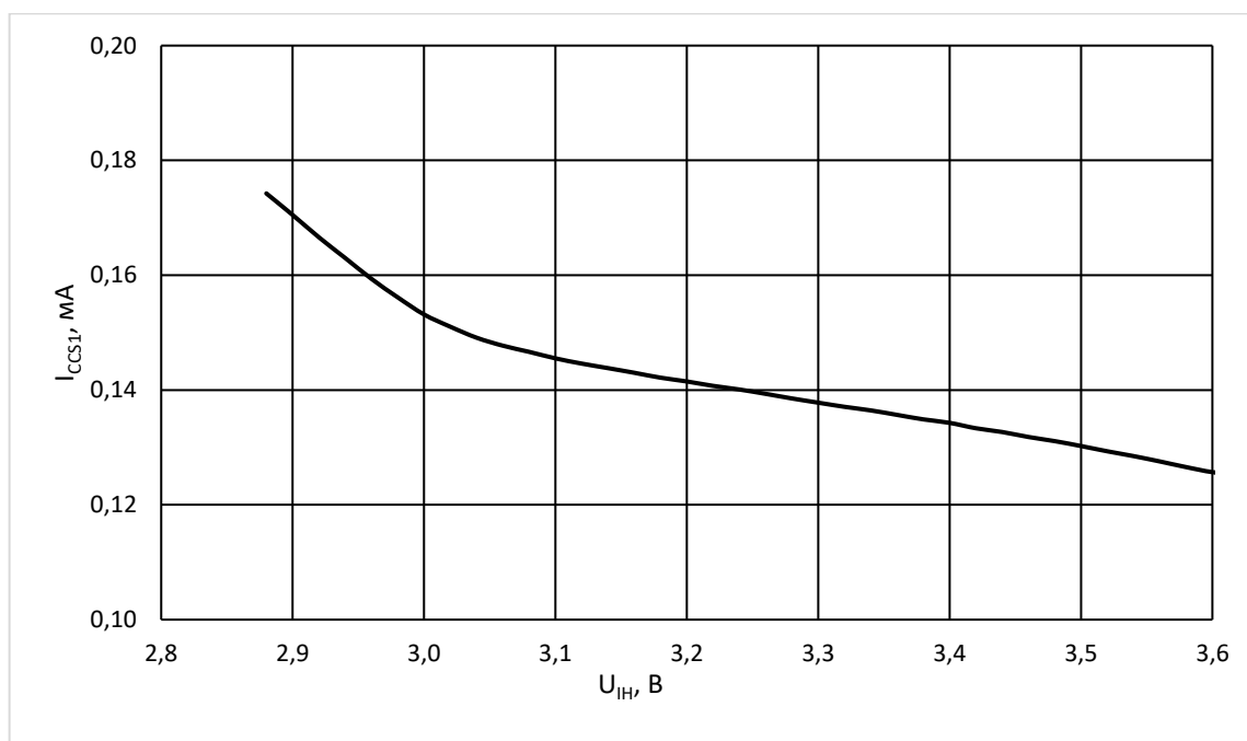
Рисунок 56 – Зависимость тока в режиме пониженного энергопотребления I_{CCS1} от входного напряжения высокого уровня U_{IH} при U_{CC} = 3,6 В, U_{IL} = 0 В, U_{nCE} = U_{IH} , U_{nWP} = U_{nHOLD} = Z , f_{C(SCK)} = 0 МГц, T = 25 °C
