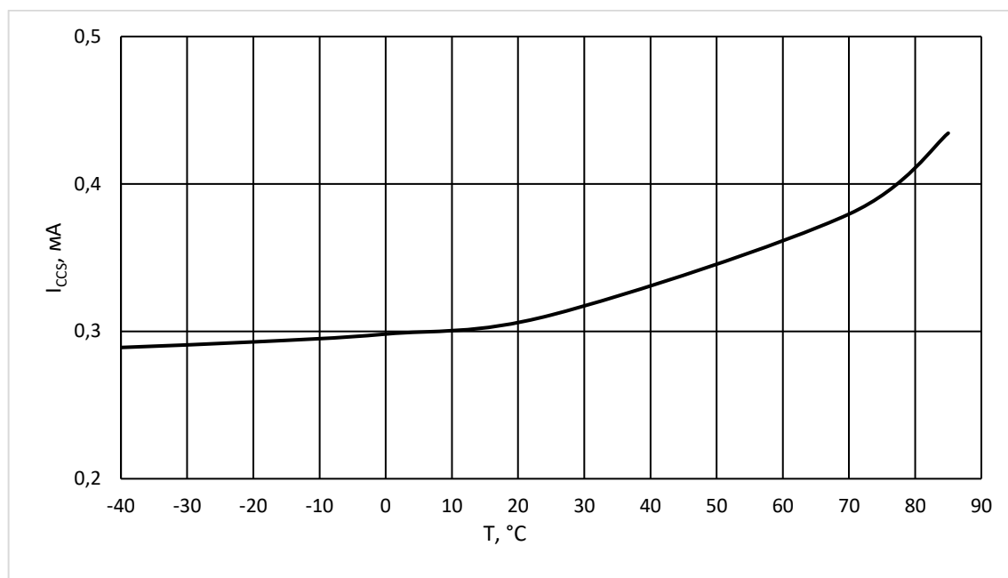
Рисунок 51 – Зависимость тока потребления в режиме хранения I_{CCS} от температуры T при U_{CC} = 3,6 В, U_{IL} = 0 В, U_{IH} = U_{CC} , U_{nCS} = U_{CC} , U_{nWP} = U_{nHOLD} = Z , f_{C(SCK)} = 0 МГц
