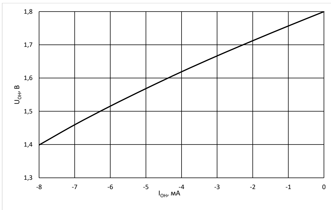
Рисунок 44 – Зависимость выходного напряжения высокого уровня U_{OH} от тока нагрузки I_{OH} при U_{CC} = 1,8 В, T = 25 °C
