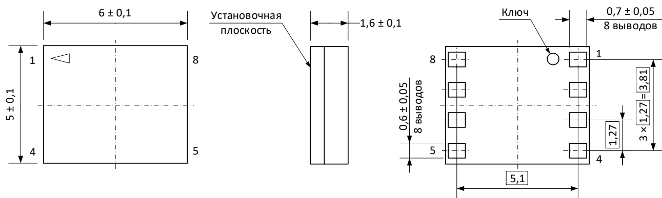
Рисунок 63 – Микросхема в корпусе DFN8 5×6×1,6 (1,27)
