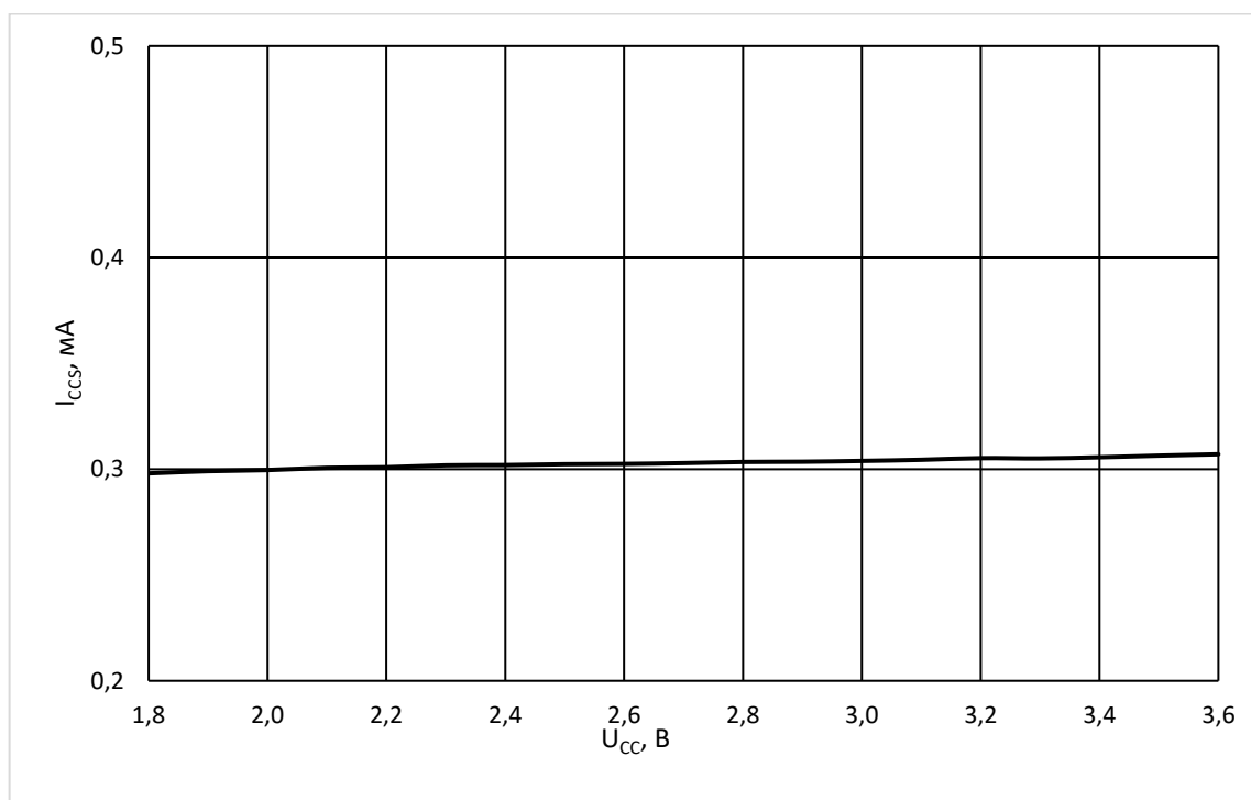
Рисунок 50 – Зависимость тока потребления в режиме хранения I_{CCS} от напряжения питания U_{CC} при T = 25 °С, U_{IL} = 0 В, U_{IH} = U_{CC} , U_{nCS} = U_{CC} , U_{nWP} = U_{nHOLD} = Z , f_{C(SCK)} = 0 МГц
