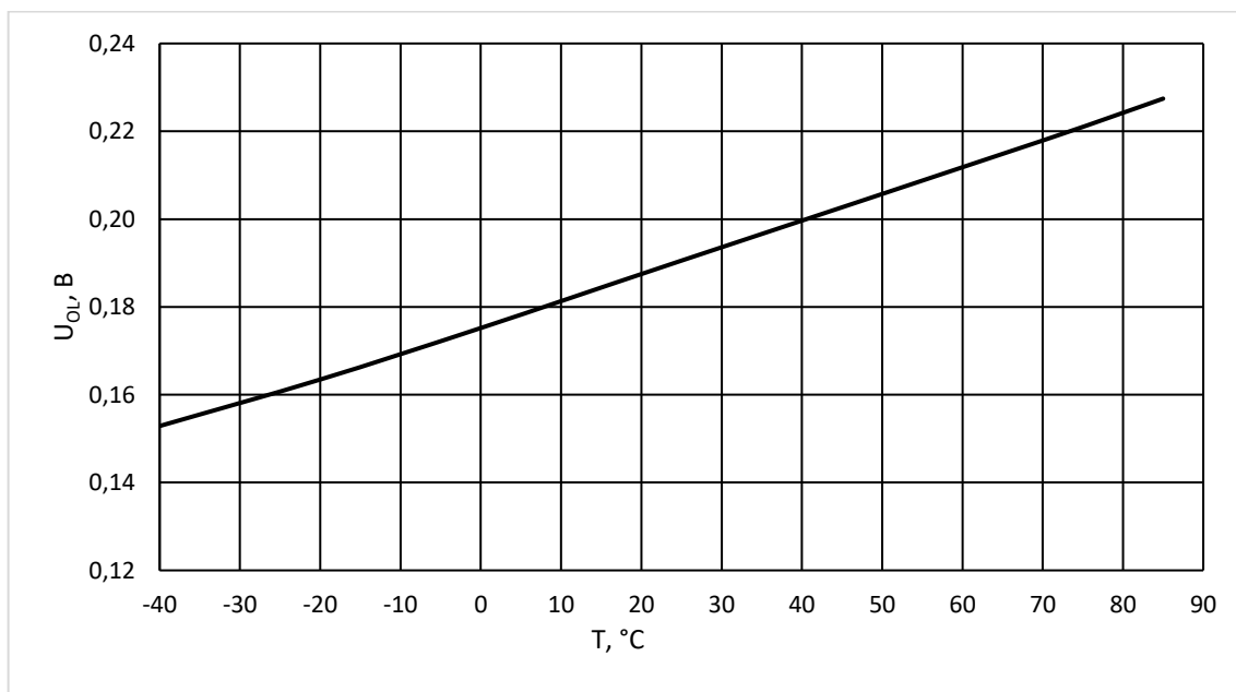
Рисунок 40 – Зависимость выходного напряжения низкого уровня U_{OL} от температуры T при U_{CC} = 1,8\text{ В} и I_{OL} = 4\text{ мА}
