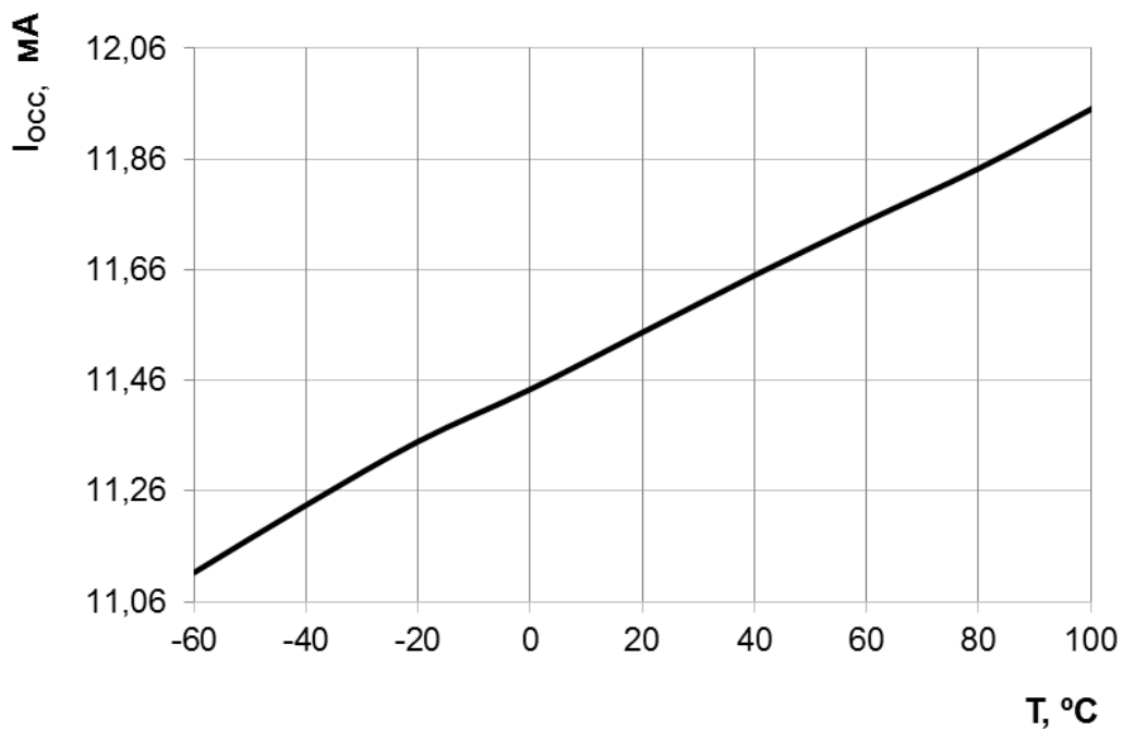
Рисунок 130 – Зависимость динамического тока потребления I_{\text{осс}} аналоговых блоков от температуры при U_{\text{CC}} = 1,32 \text{ В} , U_{\text{CCIO}} = U_{\text{CCA}} = 3,6 \text{ В}
