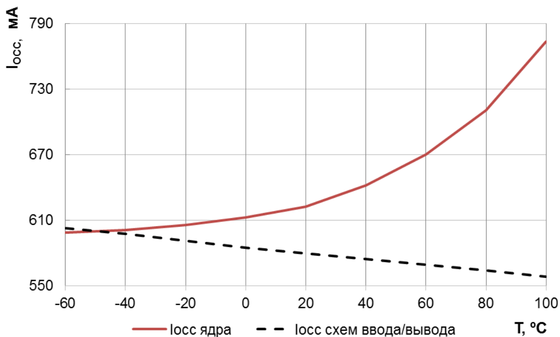
Рисунок 129 – Зависимость динамического тока потребления I_{\text{осс}} ядра и схем ввода/вывода от температуры при U_{\text{CC}} = 1,32 \text{ В} , U_{\text{CCIO}} = U_{\text{CCA}} = 3,6 \text{ В} , f_c = 230 \text{ МГц}
