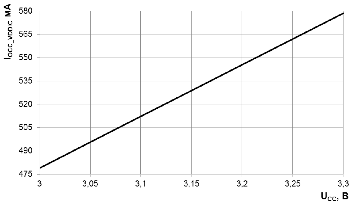
Рисунок 131 – Зависимость динамического тока потребления I OCC схем ввода/вывода от напряжения питания при f c = 230 МГц, T = 25 °C
