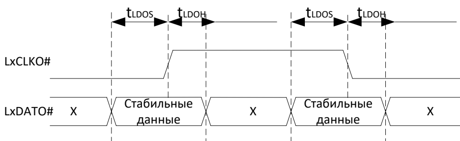
Рисунок 85 – Временная диаграмма выходных данных порта связи
