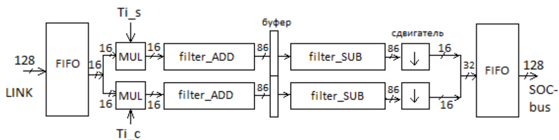
Рисунок 114 – Структура модуля в режиме DOWN
