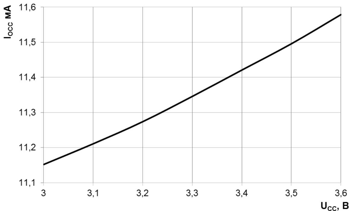
Рисунок 132 – Зависимость динамического тока потребления I OCC аналоговых блоков от напряжения питания при f c = 230 МГц, T = 25 °C
