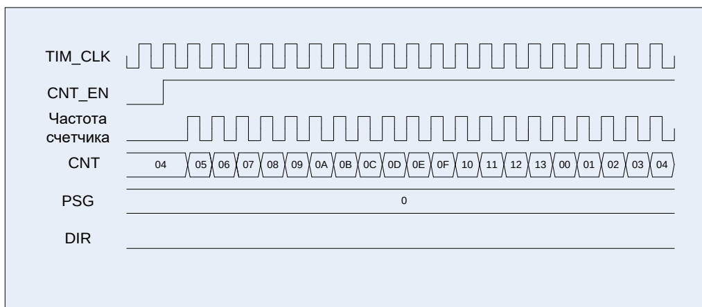
Рисунок 20 – Диаграммы работы таймера, счет вверх от 0 до 0x0013, стартовое значение 0x0004
