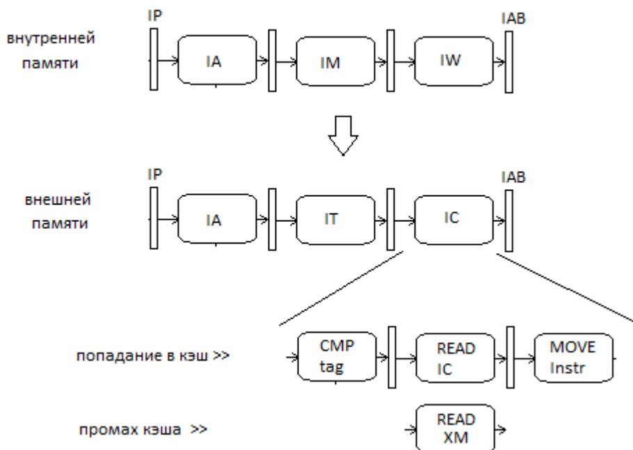
Рисунок 12 – Конвейер выборки команд из внешней памяти
