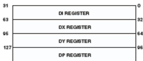
Рисунок 51 – Регистры блока управления передачей
