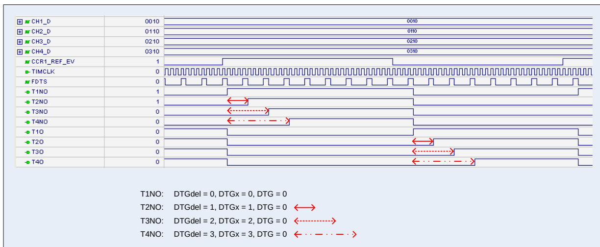
Рисунок 42 – Диаграмма работы схемы DTG
