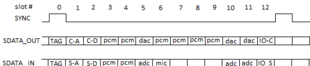
Рисунок 97 – Структура фрейма
