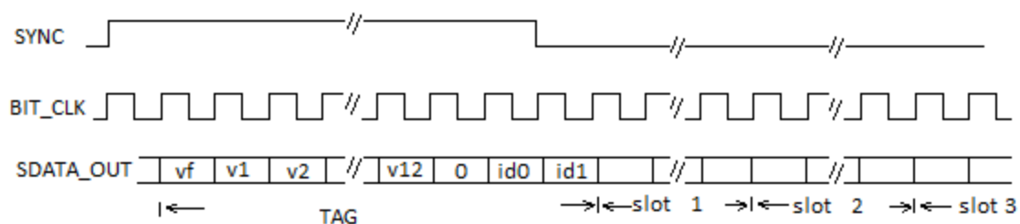
Рисунок 98 – Структура тэга
