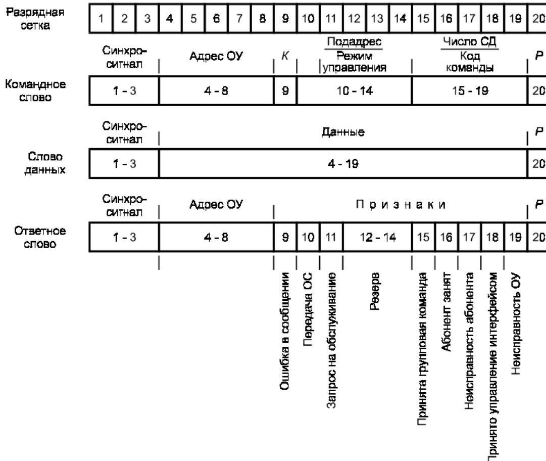
Рисунок 110 – Форматы слов
