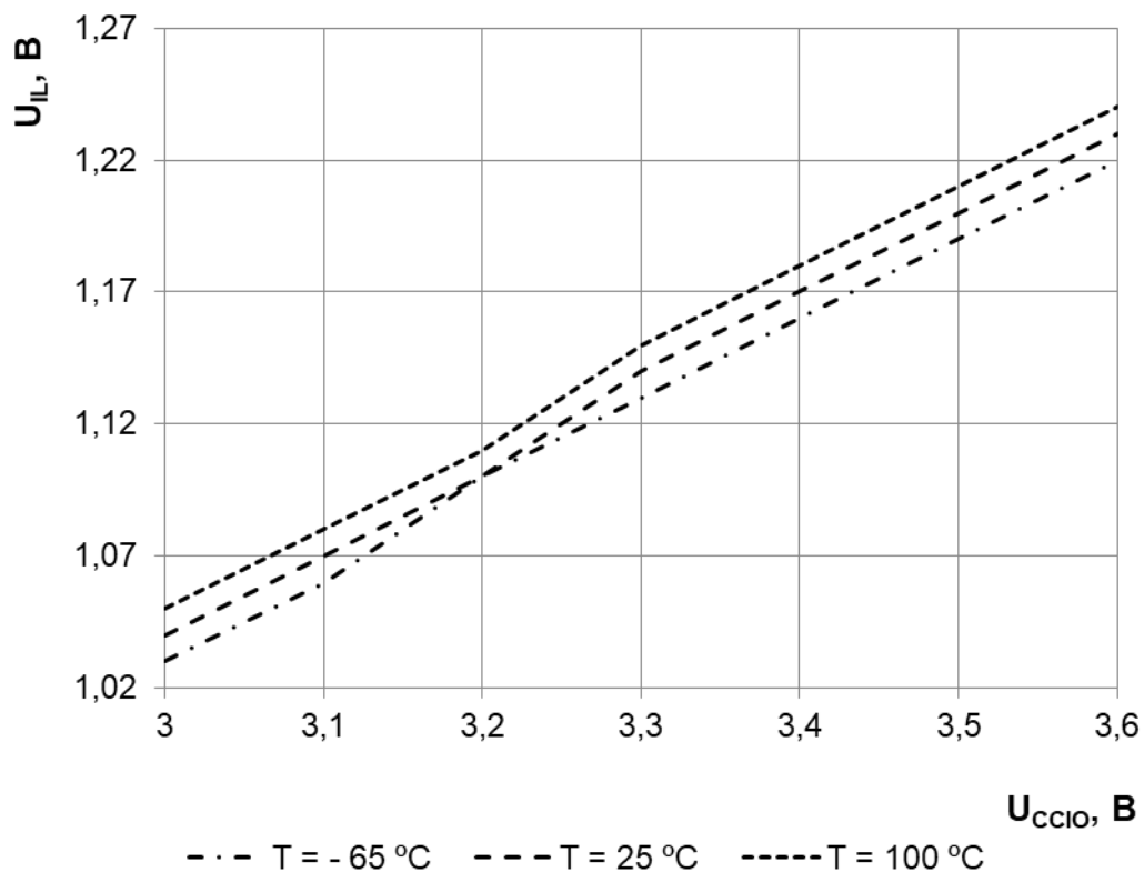
Рисунок 137 – Зависимость входного напряжения низкого уровня U_{IL} от напряжения питания схем ввода/вывода U_{CCIO} при U_{CC} = 1,08 \text{ В}
