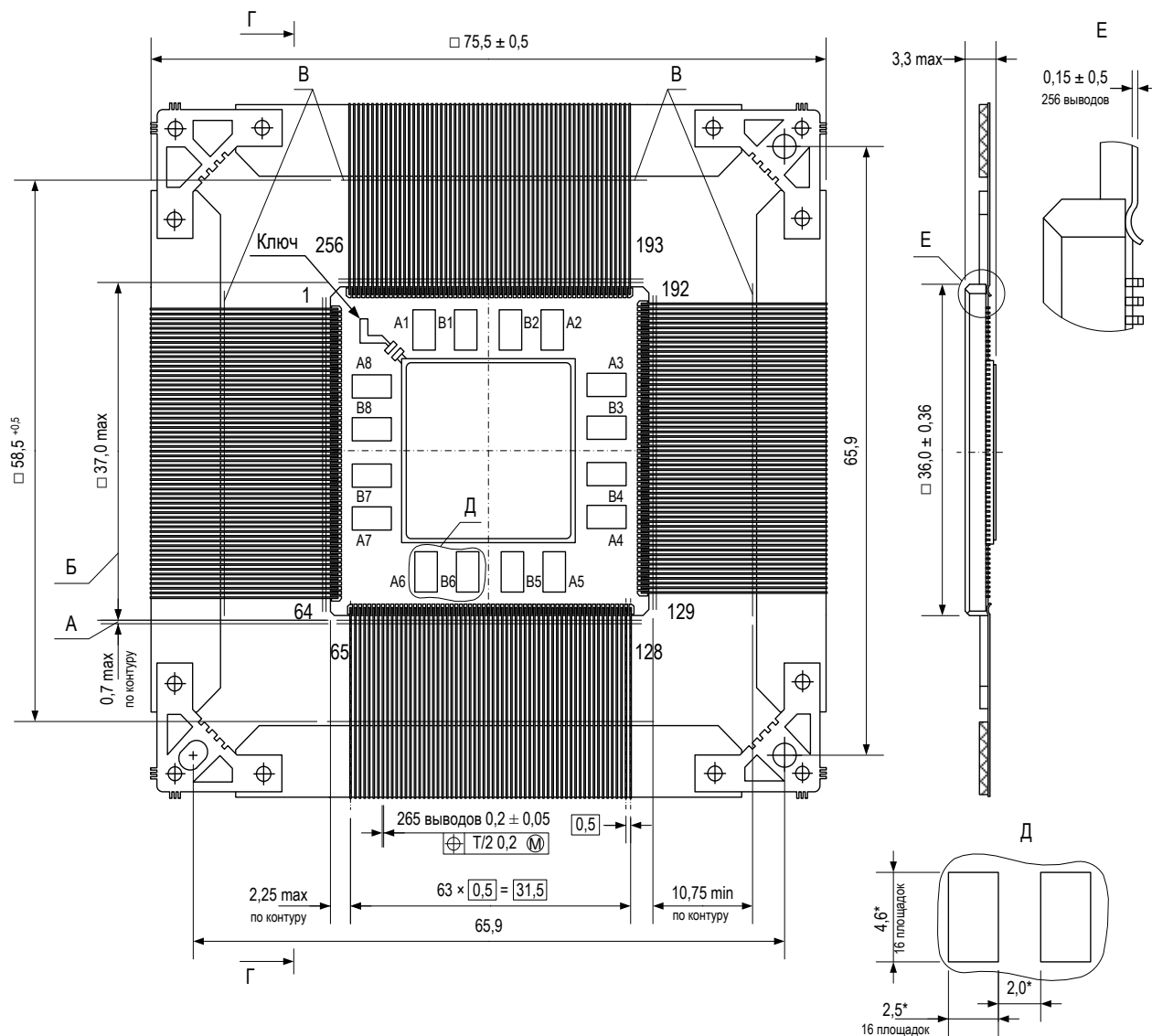
Рисунок 138 – Микросхема в корпусе 4244.256-3
