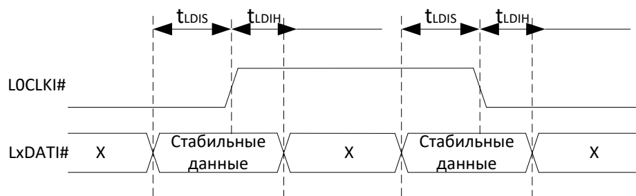
Рисунок 83 – Временная диаграмма входных данных порта связи при тактировании от L0CLKI#
