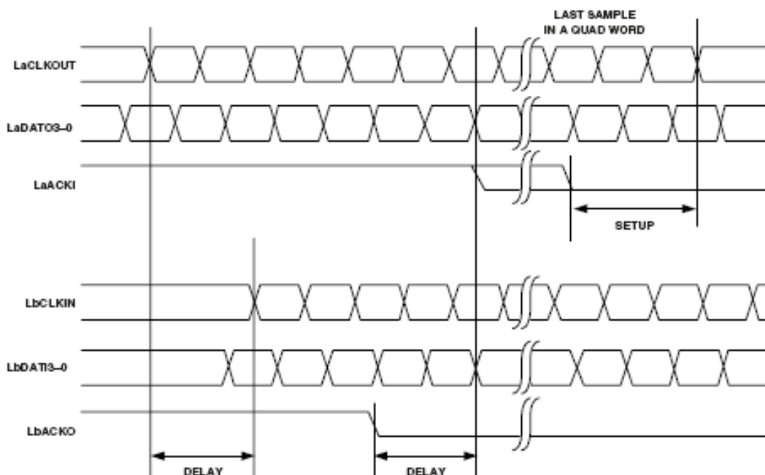
Рисунок 82 – Порт связи “а” передает порту связи “b” с задержкой
