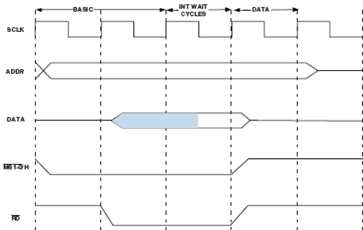
Рисунок 59 – Медленный протокол. Чтение с циклами ожидания
