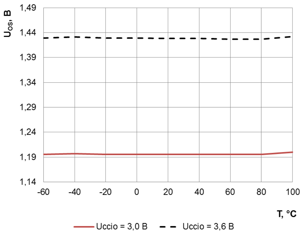
Рисунок 128 – Зависимость синфазного выходного напряжения LINK портов U_{Os} от температуры при R_L=100 Ом
