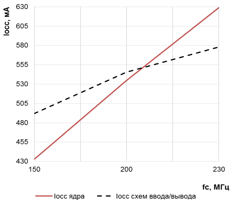
Рисунок 134 – Зависимость динамического тока потребления I_{oss} ядра и схем ввода/вывода от тактовой частоты процессора f_c при U_{CC} = 1,32 \text{ В} , U_{CCIO} = U_{CCA} = 3,6 \text{ В} , T = 25 \text{ °C}
