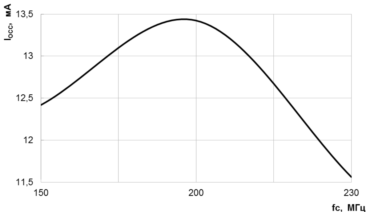
Рисунок 135 – Зависимость динамического тока потребления аналоговых блоков I_{occ} от тактовой частоты процессора f_c при U_{cc} = 1,32 В, U_{ccio} = U_{cca} = 3,6 В, T = 25 °С
