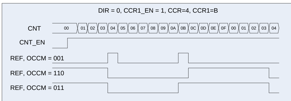
Рисунок 43 – Диаграмма работы схемы в режиме ШИМ, CCR1_EN = 1
