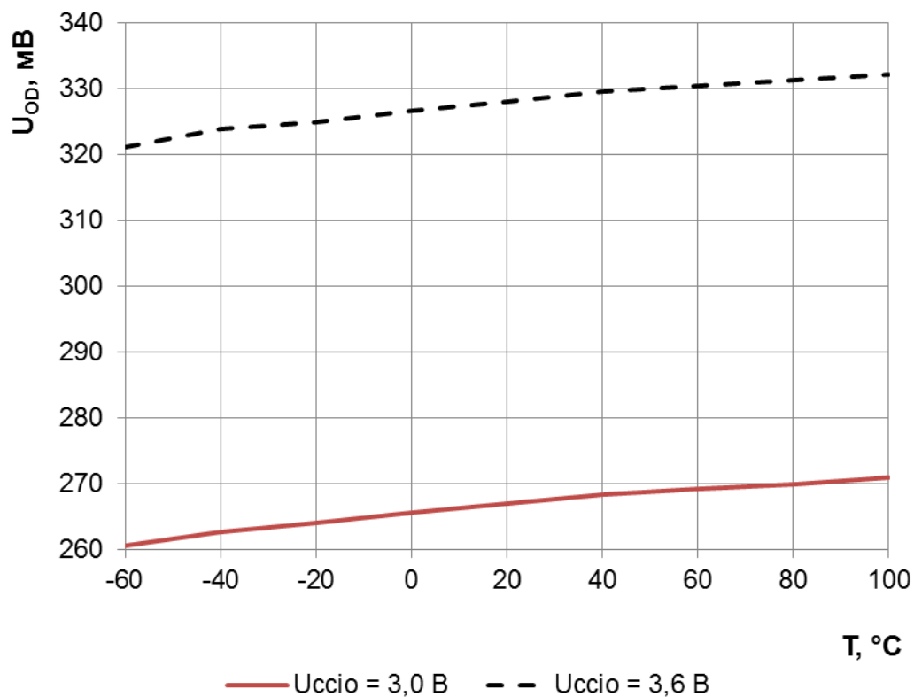
Рисунок 127 – Зависимость дифференциального выходного напряжения LINK-портов U_{OD} от температуры при R_L=100 Ом
