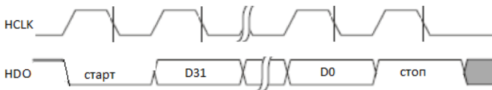
Рисунок 68 – Передача информации контроллером интерфейса
