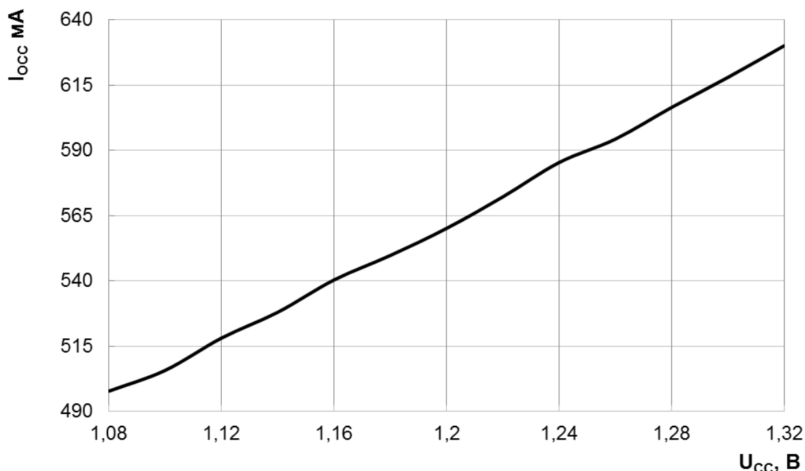
Рисунок 133 – Зависимость динамического тока потребления I_{oss} ядра от напряжения питания при f_c = 230 \text{ МГц} , T = 25 \text{ °C}
