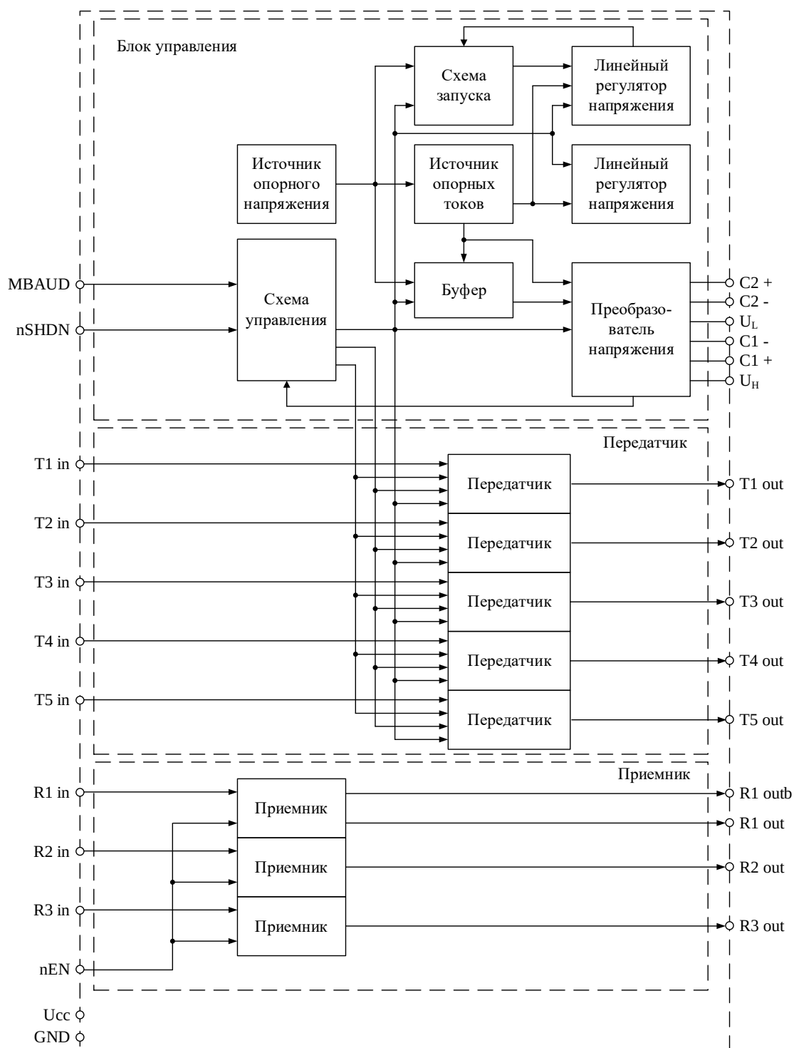
Рисунок 1 – Структурная блок-схема
