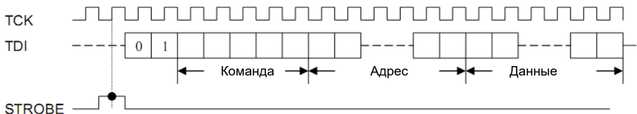
Рисунок 9 – Режим командного цикла
