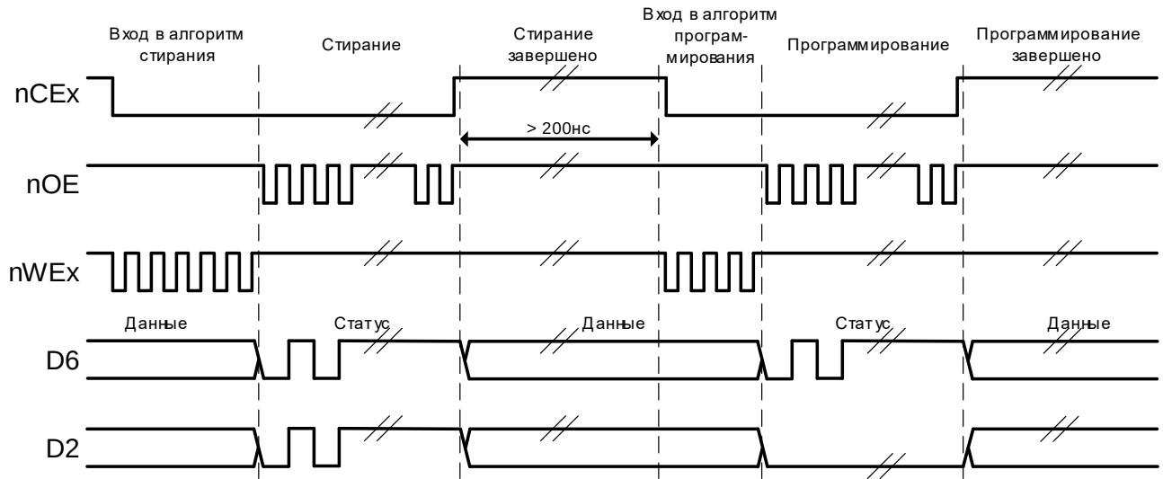
Рисунок 36 – Временная диаграмма переключения статусных бит
