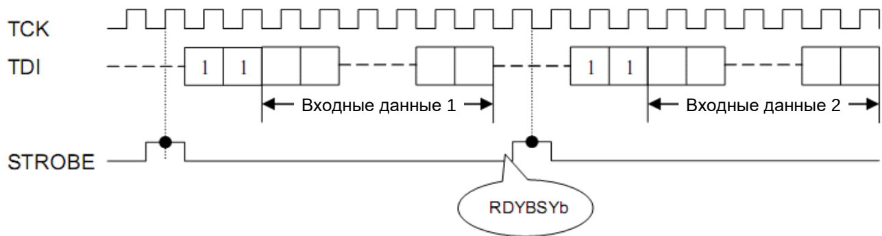
Рисунок 12 – Повтор цикла записи
