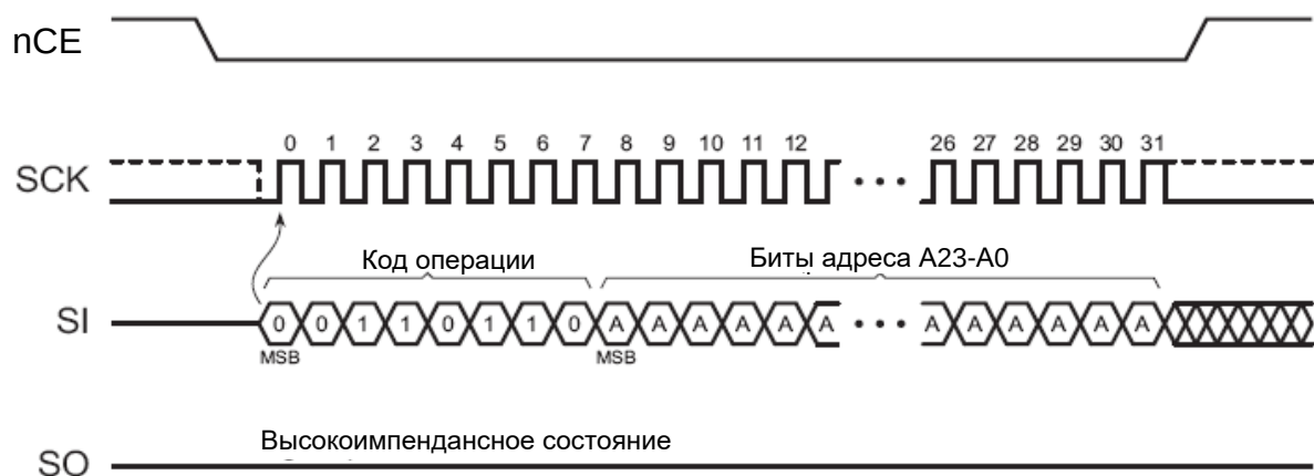
Рисунок 21 – Операция установки защиты сектора
