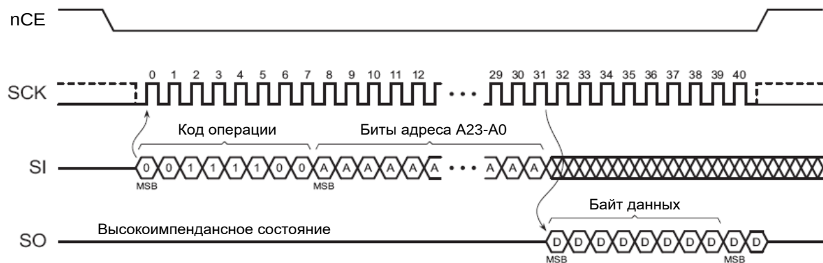
Рисунок 23 – Операция чтения регистра защиты сектора
