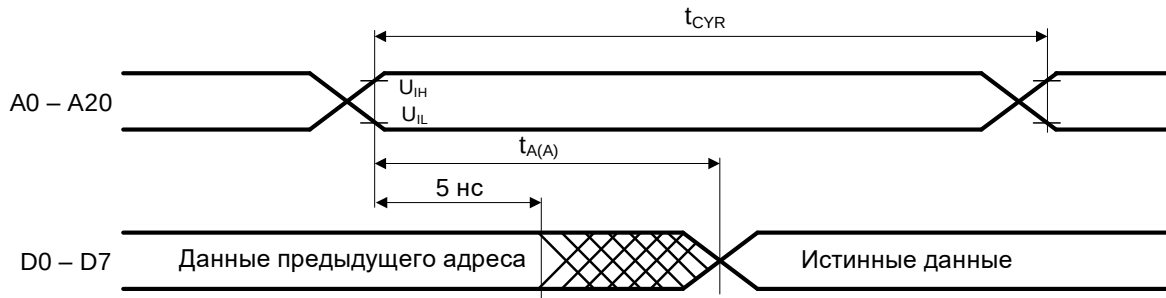
Рисунок 31 – Временная диаграмма цикла чтения по адресу
