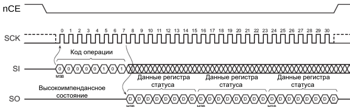
Рисунок 24 – Операция чтения регистра статуса
