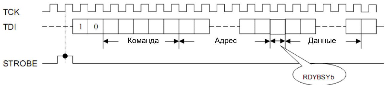
Рисунок 10 – Режим цикла чтения
