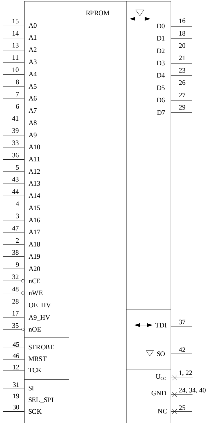
Рисунок 2 – Условное графическое обозначение
