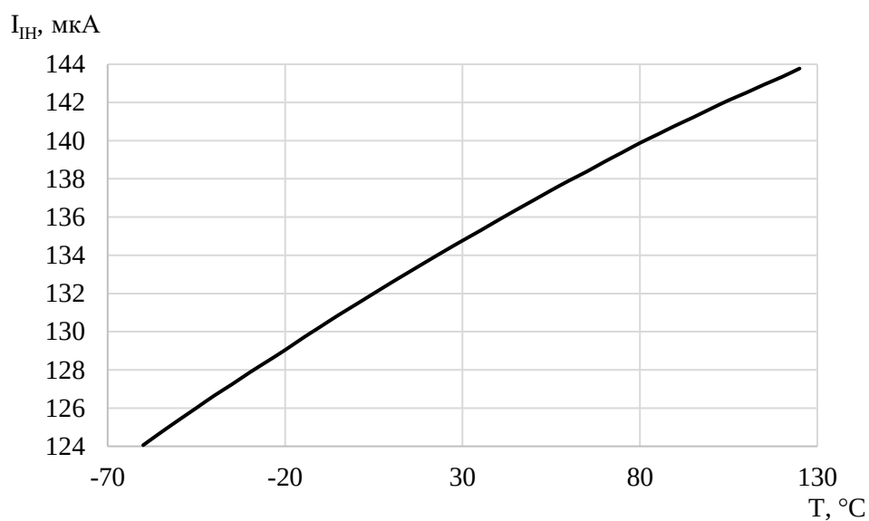
Рисунок 48 – Зависимость тока высокого уровня по входу SCK от температуры при U_{\text{СС}} = 3,6 В, U_{\text{ИЛ}} = 0 В, U_{\text{ИН}} = 5,5 В
