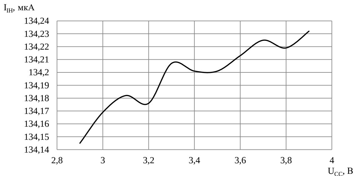
Рисунок 47 – Зависимость тока высокого уровня по входу SCK от напряжения питания при U_{\text{ИЛ}} = 0 В, U_{\text{ИН}} = 5,5 В, T = 25 °С
