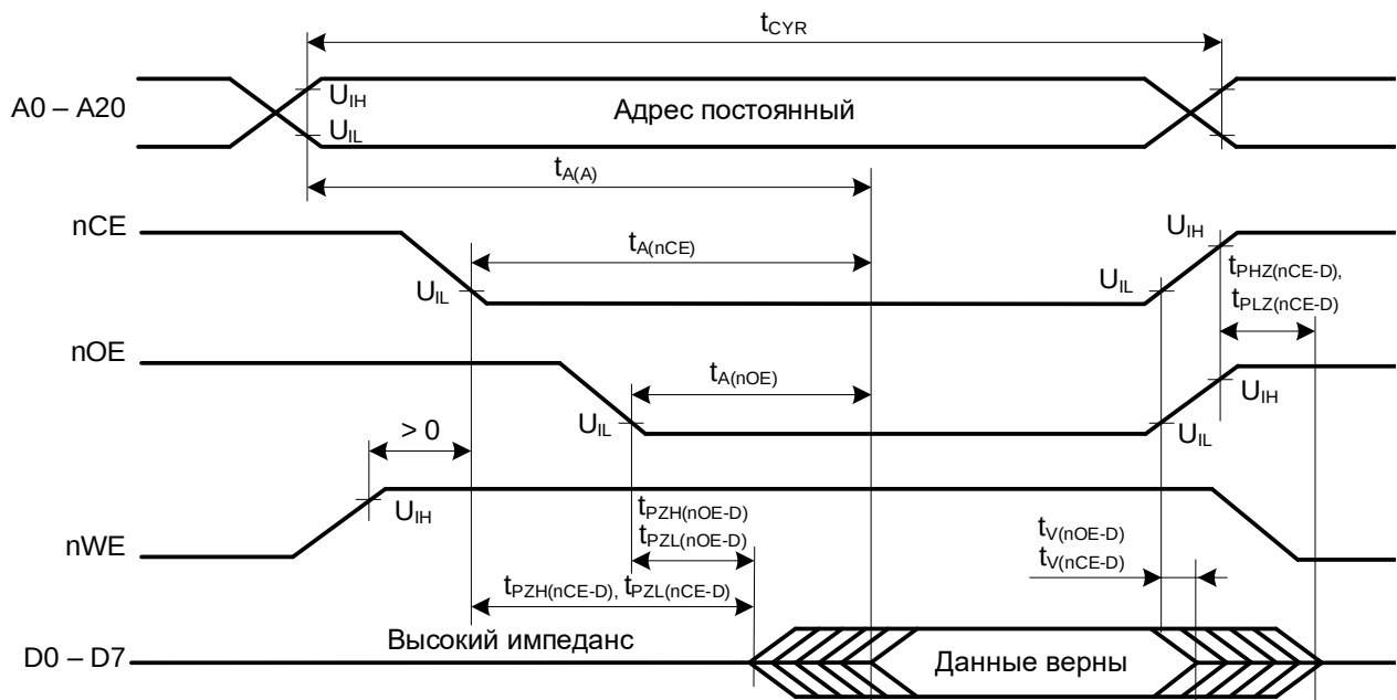
Рисунок 32 – Временная диаграмма цикла чтения управление по nOE, nCE
