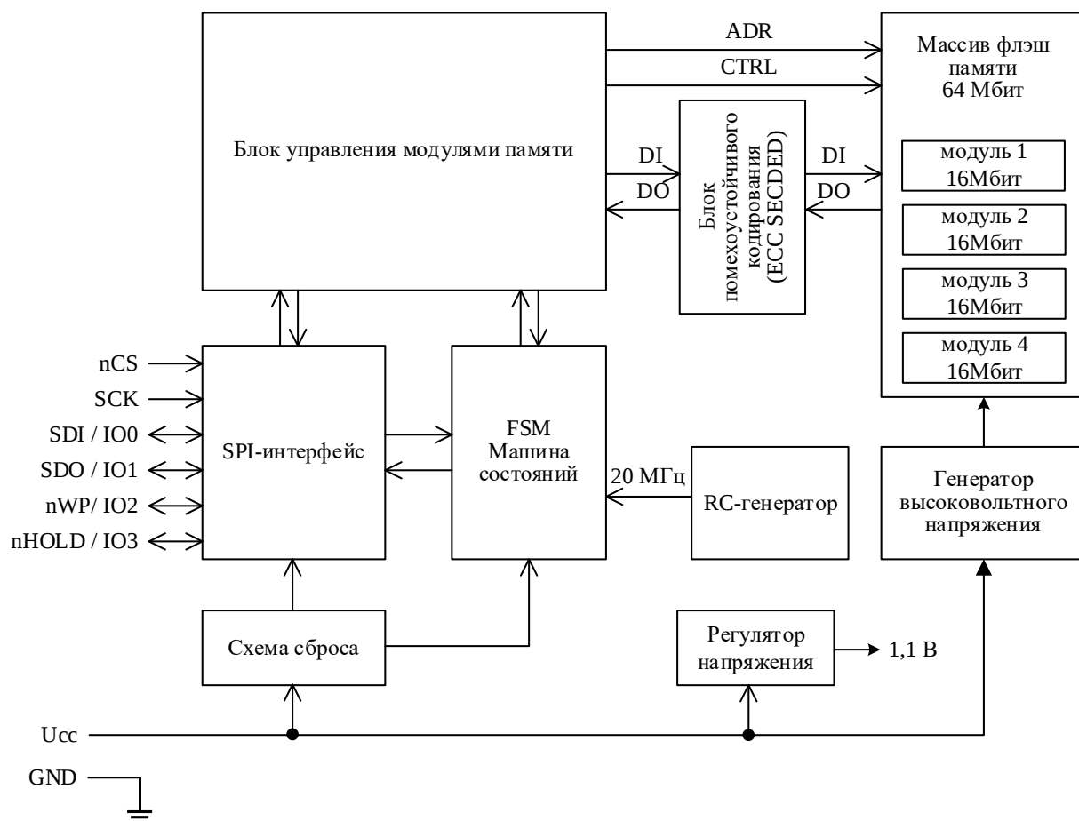
Рисунок 1 – Структурная блок-схема
