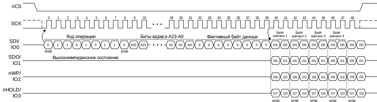
Рисунок 8 – Операция чтения с кодом 6Bh
