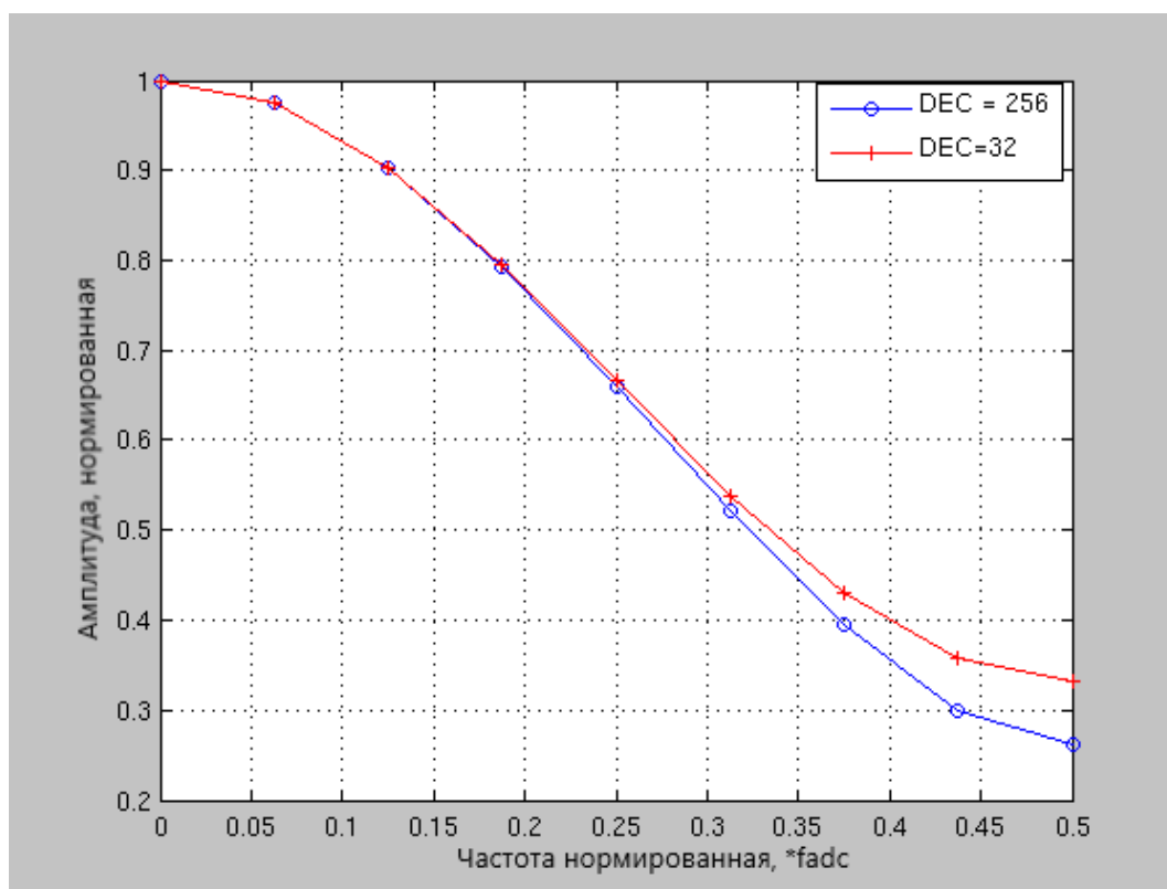
Рисунок 4 – АЧХ цифрового фильтра
