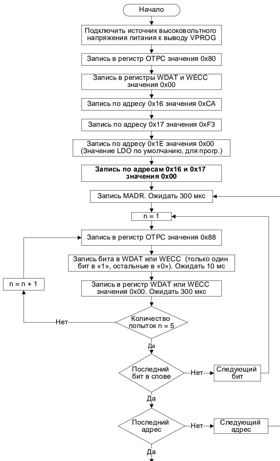
Рисунок 6 – Алгоритм программирования памяти ОТР
