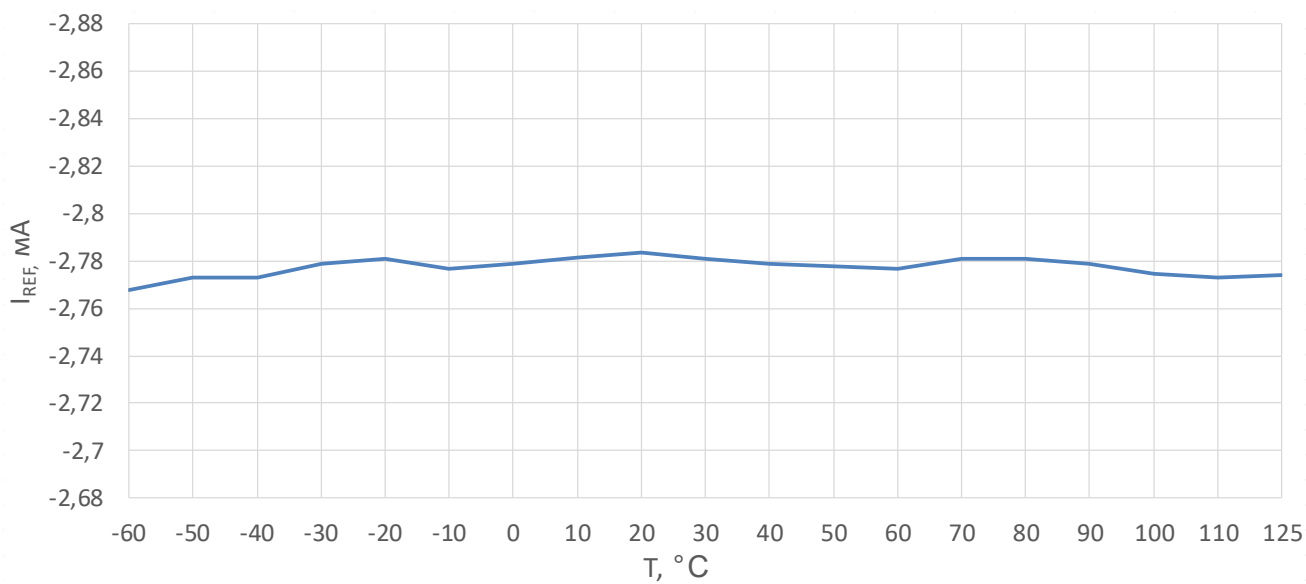
Рисунок 13 – Зависимость выходного опорного тока от температуры среды при U_{CC} = 5,5 В, U_{REF} = 4,5 В
