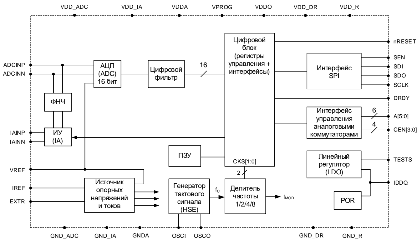
Рисунок 1 – Структурная блок-схема микросхемы
