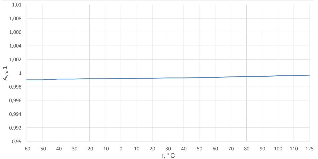
Рисунок 15 – Зависимость коэффициента усиления дифференциального сигнала ИУ по напряжению от температуры среды при U_{CC} = 5,5\text{ В} , U_{IAINN} = 0\text{ В} , I_{AS}[1:0] = 00
