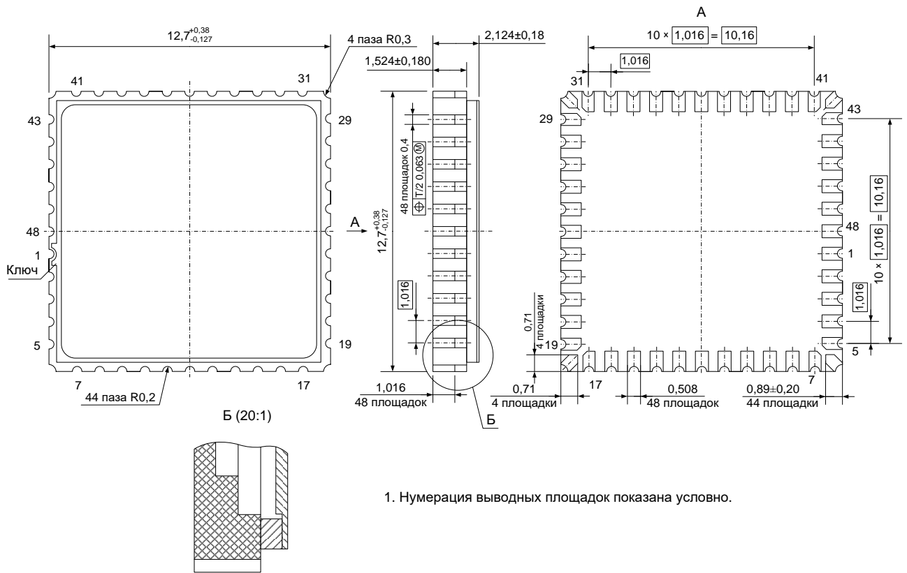
Рисунок 19 – Микросхема в корпусе 5142.48-А
