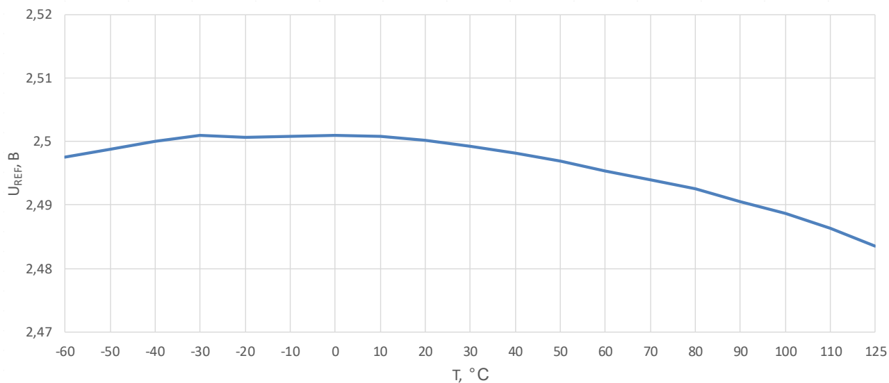
Рисунок 10 – Зависимость выходного опорного напряжения от температуры среды при U_{CC} = 5,5 В
