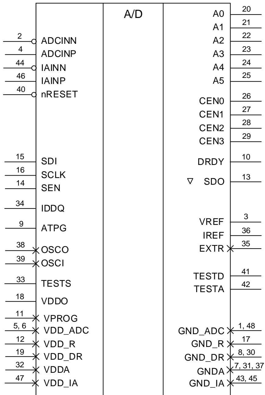
Рисунок 2 – Условное графическое обозначение микросхемы
