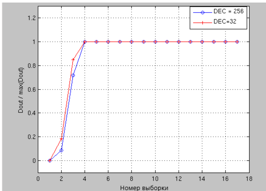
Рисунок 5 – Переходная характеристика – отношение цифрового кода на выходе к максимальному значению цифрового кода (D out /max(D out )) в зависимости от номера выборки
