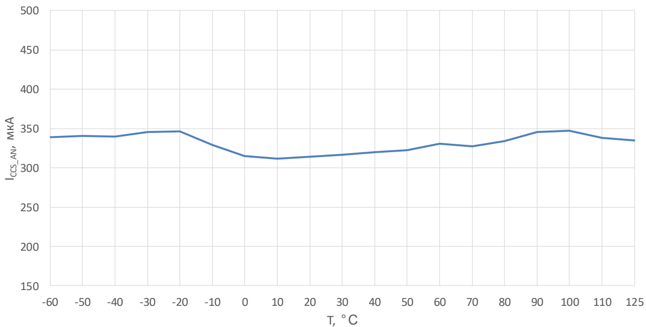
Рисунок 11 – Зависимость статического тока потребления в режиме пониженного энергопотребления от температуры среды при U_{CC} = 5,5 В
