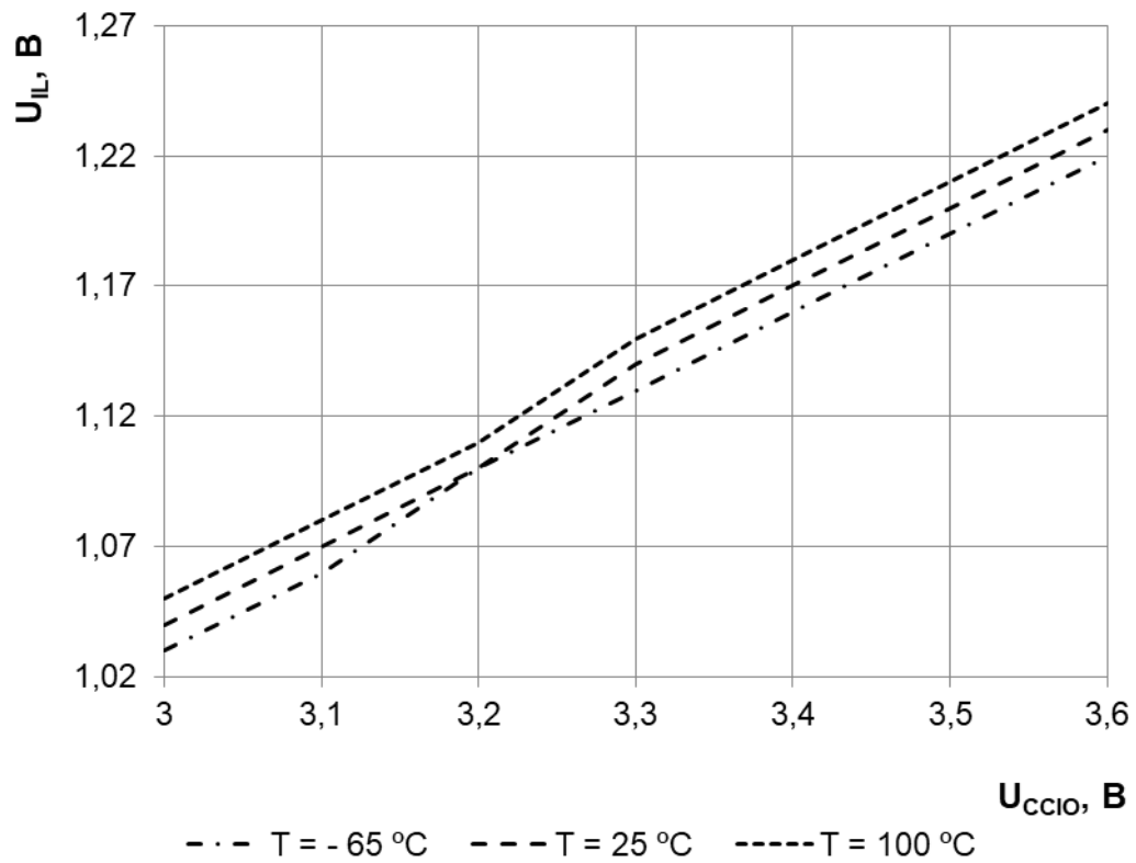
Рисунок 187 – Зависимость входного напряжения низкого уровня U_{IL} от напряжения питания схем ввода/вывода U_{CCIU} при U_{CC} = 1,08\text{ В}
