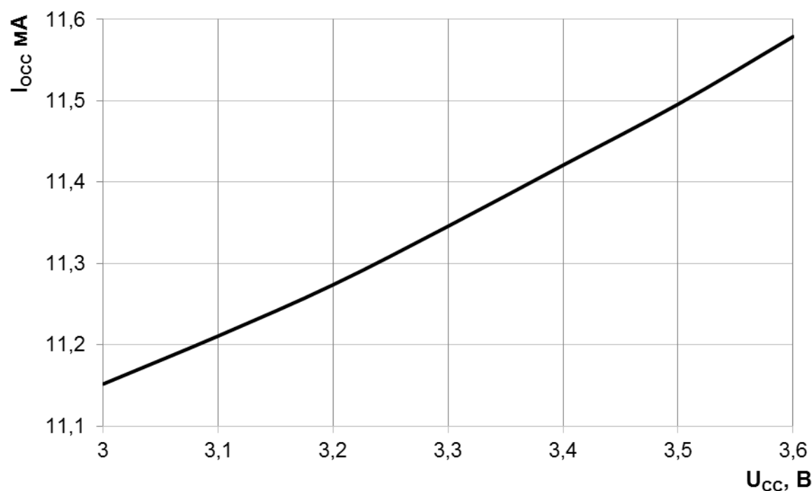
Рисунок 182 – Зависимость динамического тока потребления I OSS аналоговых блоков от напряжения питания при f C = 230 МГц, T = 25 °C
