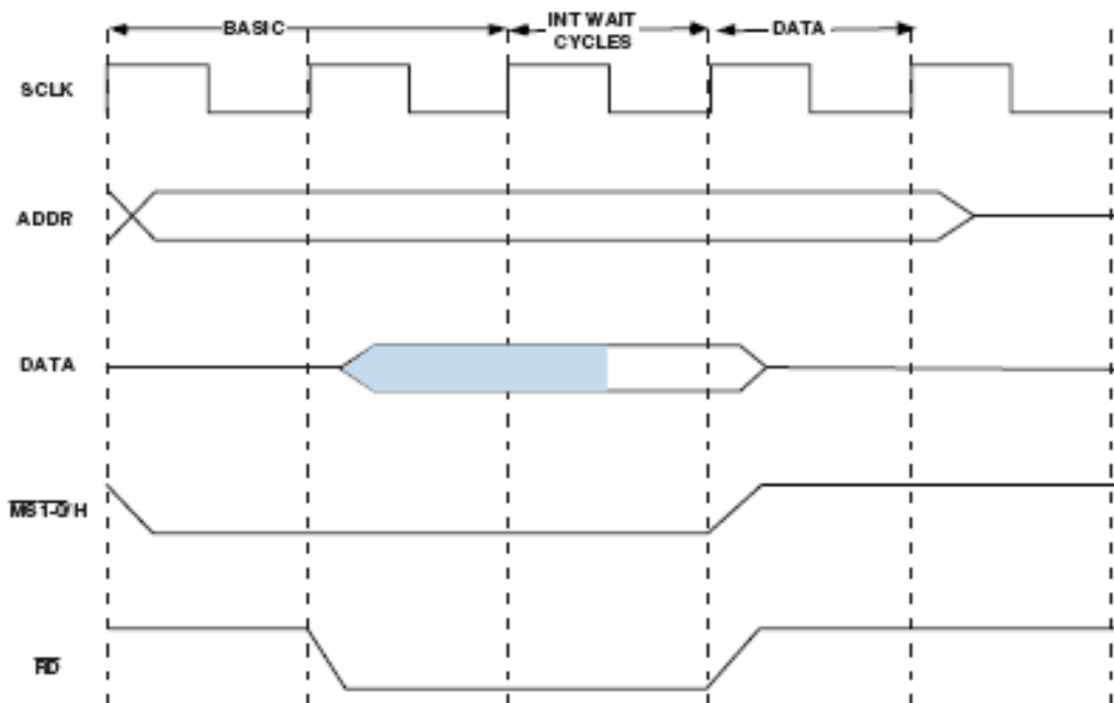
Рисунок 60 – Медленный протокол. Чтение с циклами ожидания
