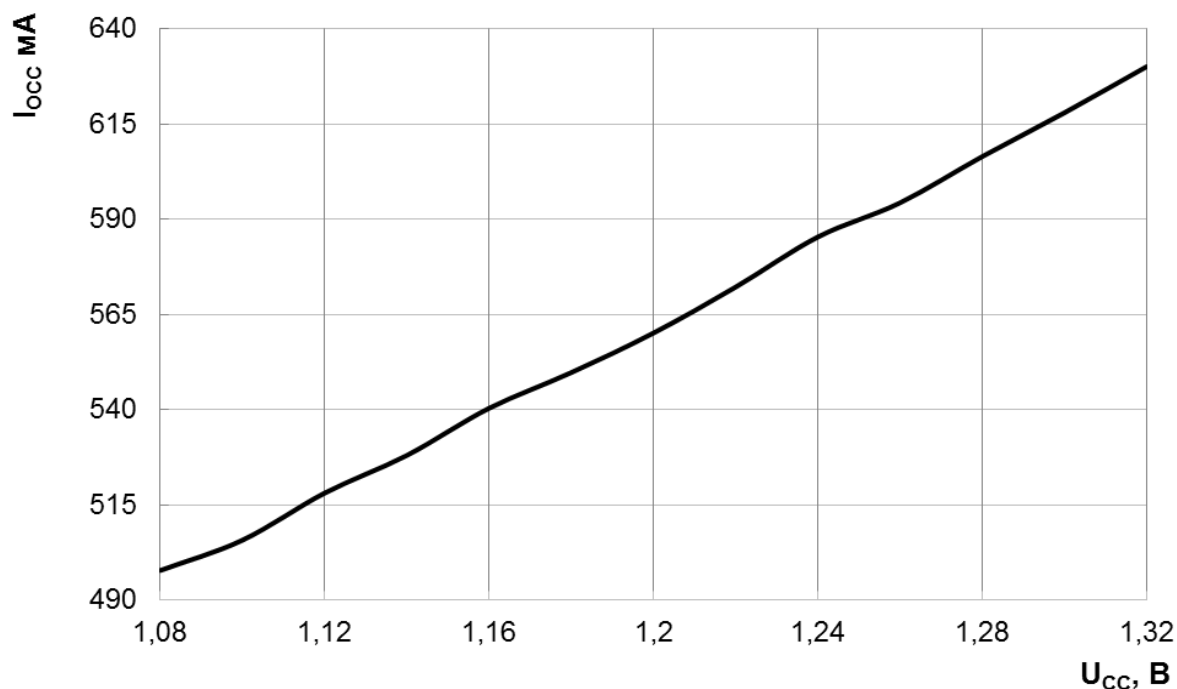
Рисунок 183 – Зависимость динамического тока потребления I_{OCC} ядра от напряжения питания при f_C = 230 \text{ МГц} , T = 25 \text{ }^\circ\text{C}
