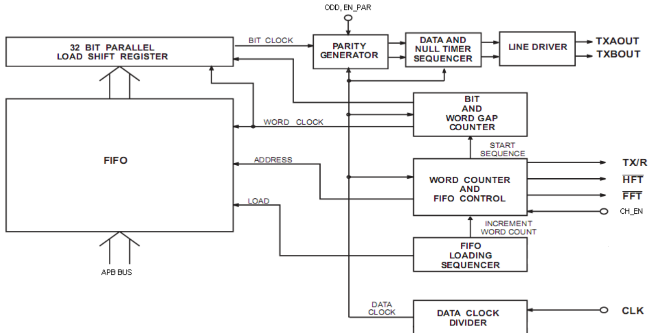
Рисунок 145 – Структурная схема канала передачи
