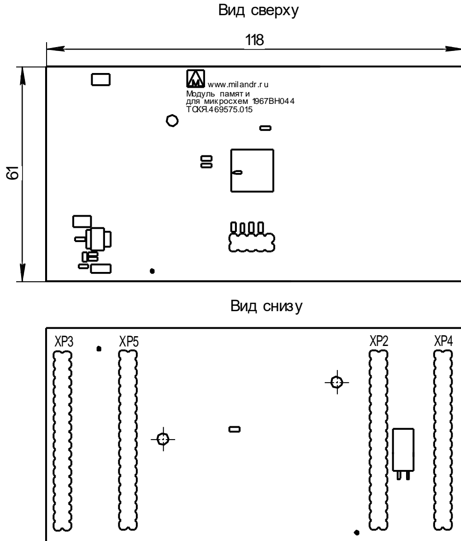
Рисунок 9 – Модуль памяти
