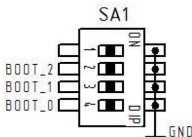
Рисунок 8 – Переключатель SA1 модуля процессора
